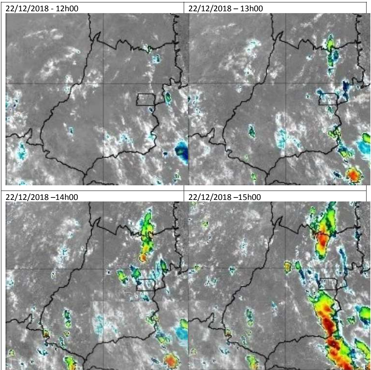
Figura 3 – Imagens realçadas do satélite GOES-16 entre as 12h00 do dia 22 e 05h00 do dia 23 de dezembro de 2018.
