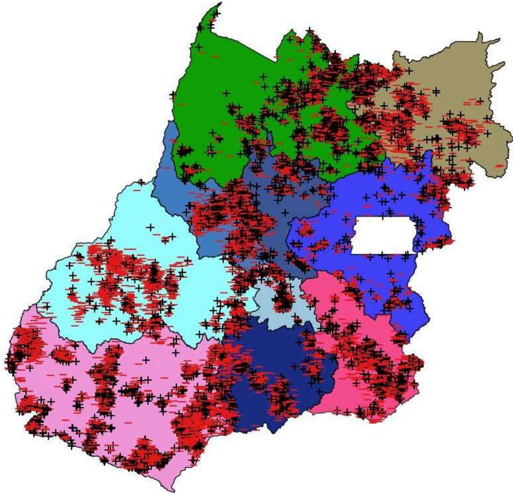
Figura 2 – Descargas atmosféricas (raios) nuvem-solo (em preto) e nuvem-nuvem (em vermelho) detectadas pelo sistema Earth Networks entre 12h00 do dia 22 e as 07h00 do dia 23 de dezembro de 2018 sobre a área de concessão da ENEL DISTRIBUIÇÃO GOIÁS.
