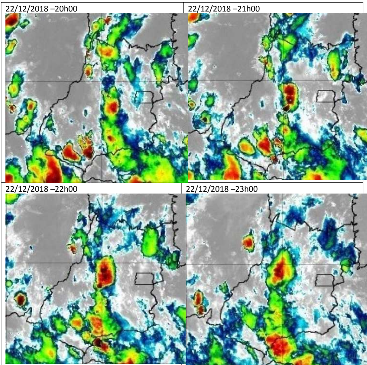
Figura 3 (continuação) – Imagens realçadas do satélite GOES-16 entre as 12h00 do dia 22 e 05h00 do dia 23 de dezembro de 2018.
