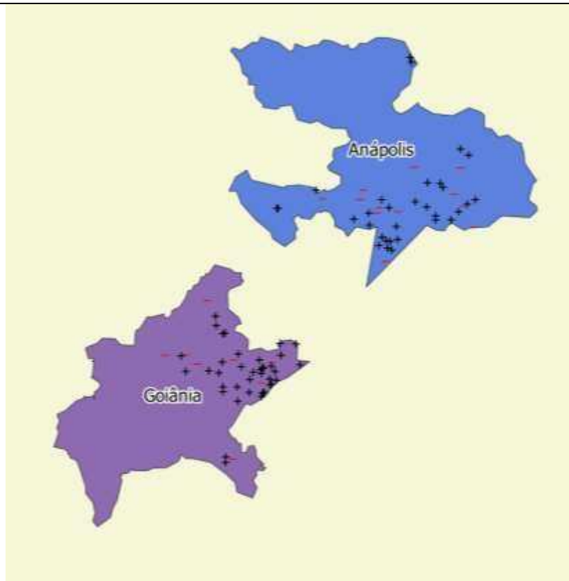
Figura 2 – Descargas atmosféricas (raios) nuvem-solo (em preto) e nuvem-nuvem (em vermelho) detectadas pelo sistema Earth Networks entre 14h35 e 17h05 do dia 18 de outubro de 2018 sobre os municípios de Goiânia e Anápolis.
