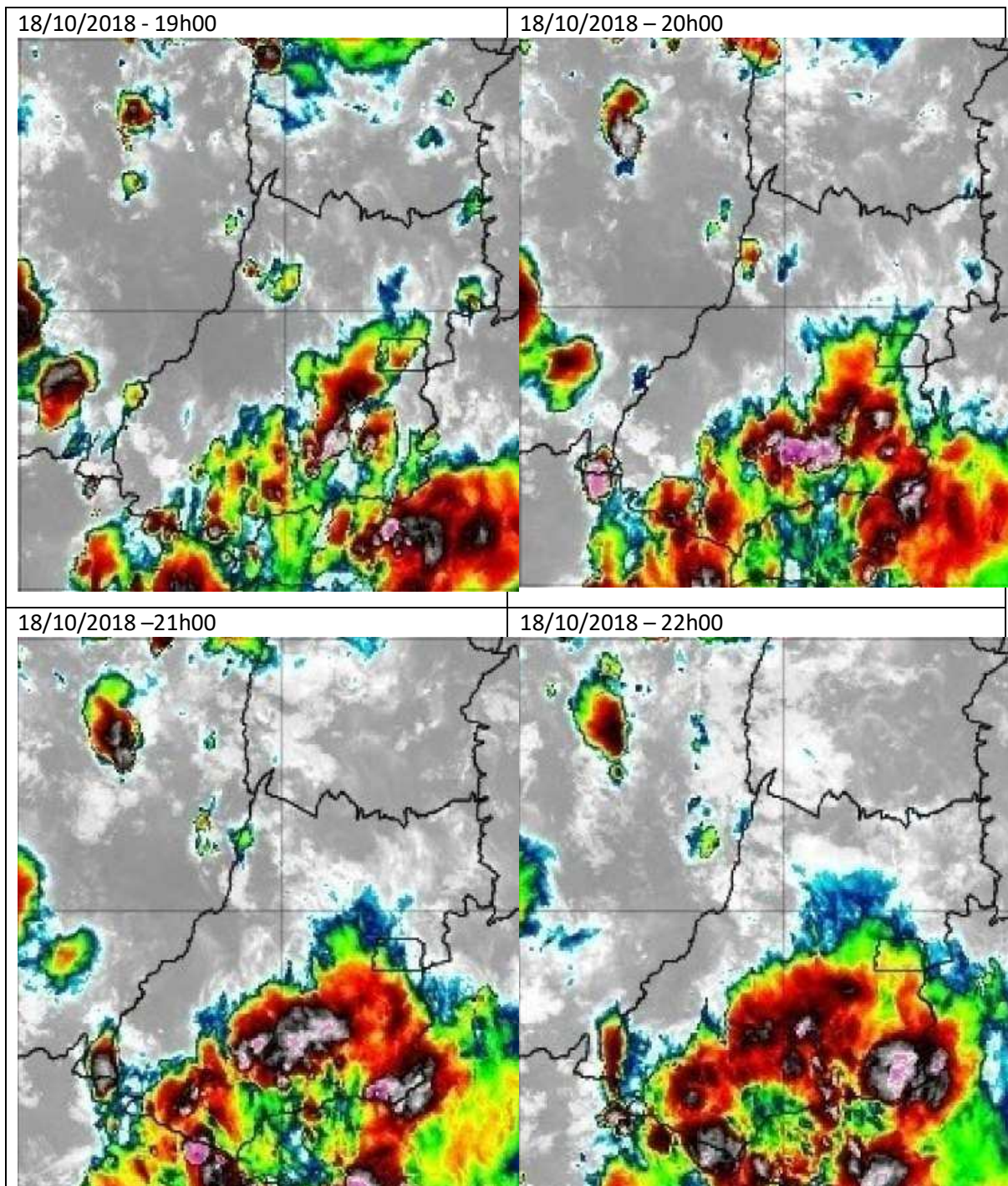
Figura 3 – Imagens realçadas do satélite GOES-16 entre as 19h00 do dia 18 e as 15h00 do dia 19 de outubro de 2018.
