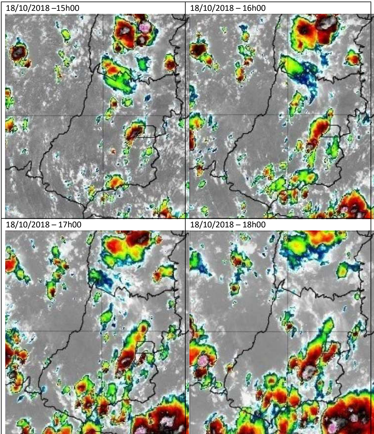
Figura 3 (continuação) – Imagens realçadas do satélite GOES-16 entre as 13h00 e 20h00 do dia 18 de outubro de 2018.
