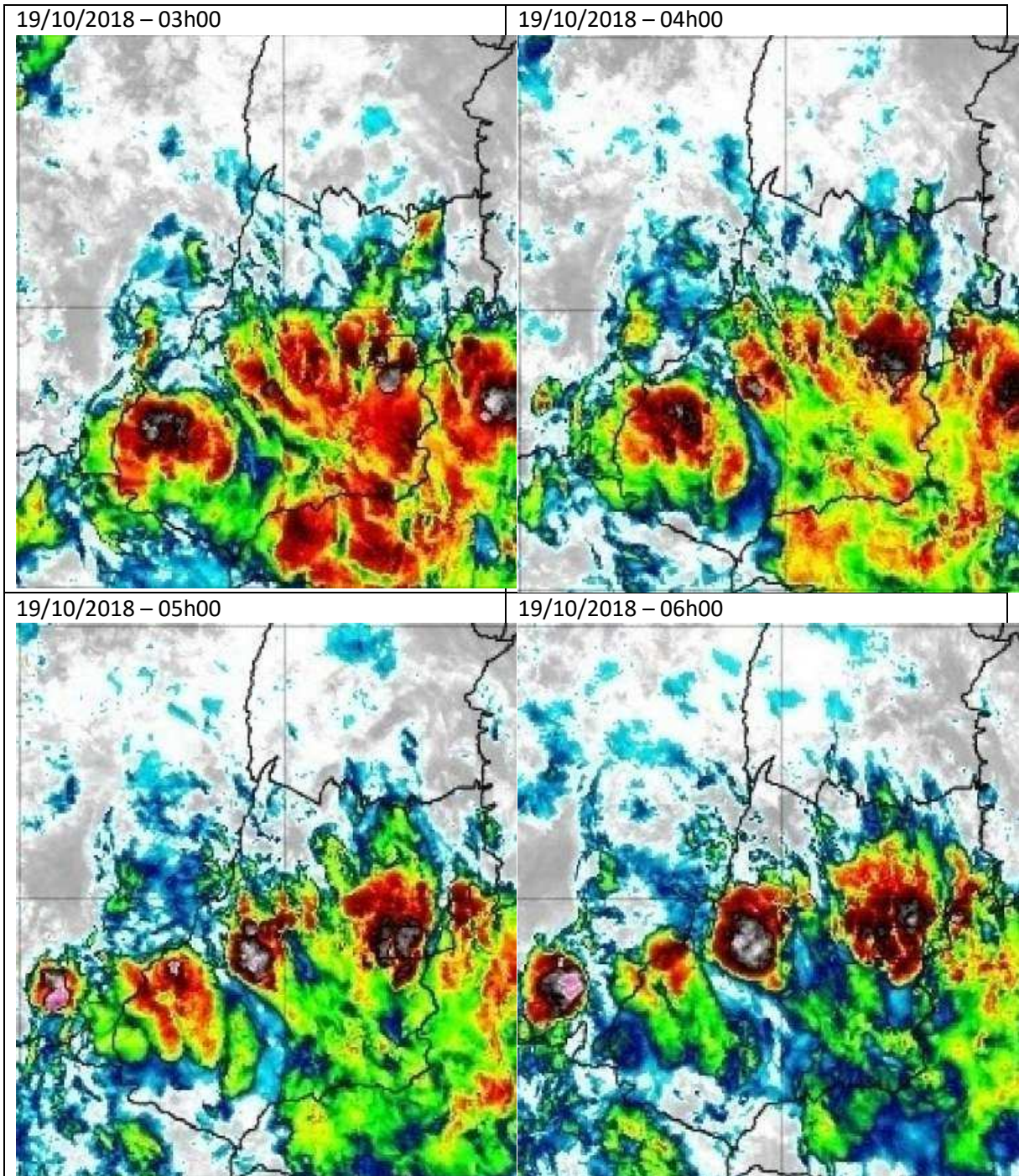
Figura 3 (continuação) – Imagens realçadas do satélite GOES-16 entre as 19h00 do dia 18 e as 15h00 do dia 19 de outubro de 2018.
