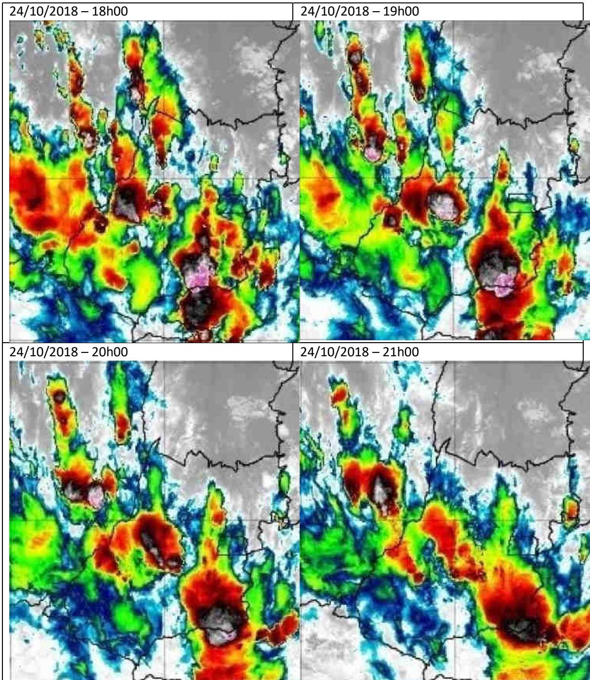
Figura 3 (continuação) – Imagens realçadas do satélite GOES-16 entre as 10h00 do dia 24 e as 01h00 do dia 25 de outubro de 2018.
