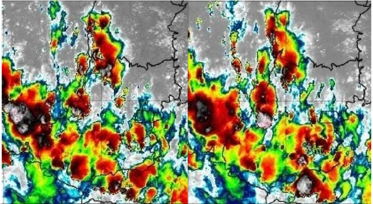
Figura 3 (continuação) – Imagens realçadas do satélite GOES-16 entre as 10h00 do dia 24 e as 01h00 do dia 25 de outubro de 2018.
