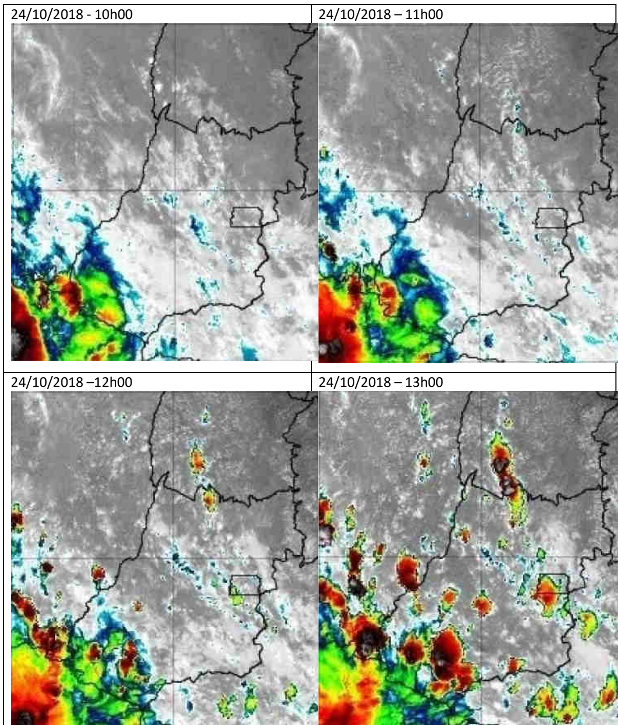
Figura 3 – Imagens realçadas do satélite GOES-16 entre as 10h00 do dia 24 e as 01h00 do dia 25 de outubro de 2018.
