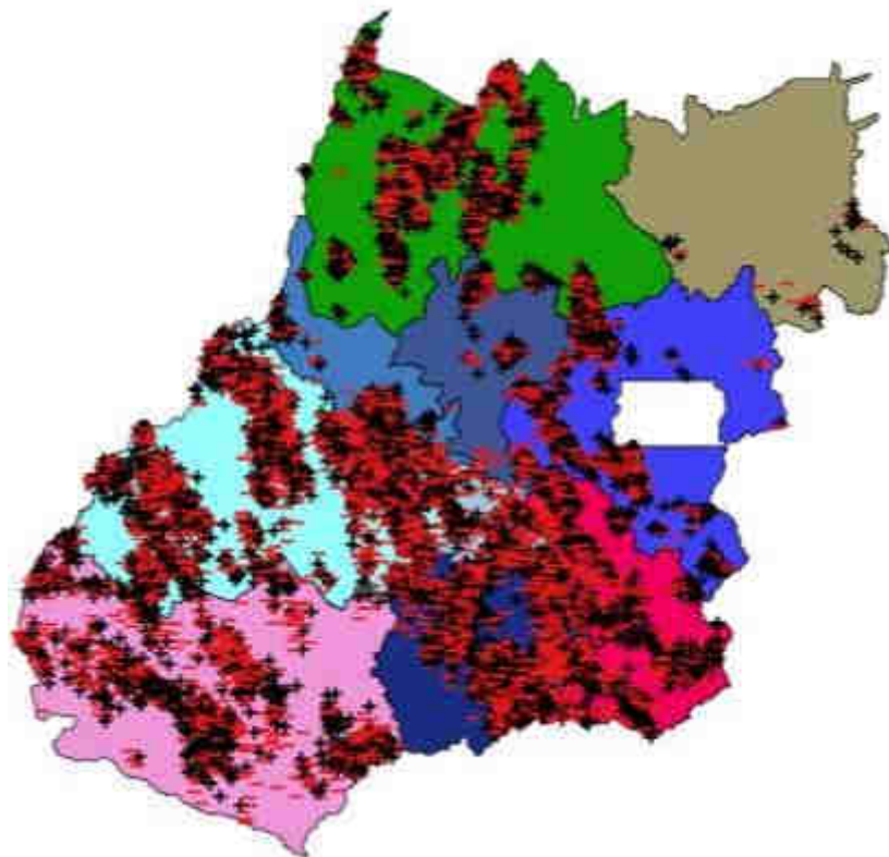
Figura 2 – Descargas atmosféricas (raios) nuvem-solo (em preto) e nuvem-nuvem (em vermelho) detectadas pelo sistema Earth Networks entre 20h00 do dia 18 e as 12h00 do dia 19 de outubro de 2018 sobre a área de concessão da CELG Distribuição.
