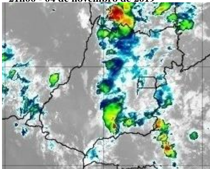
Figura 7 –Imagens realçadas do satélite GOES-16 das 21h00 do dia 04 de novembro de 2019. FONTE: Cptec/INPE.
