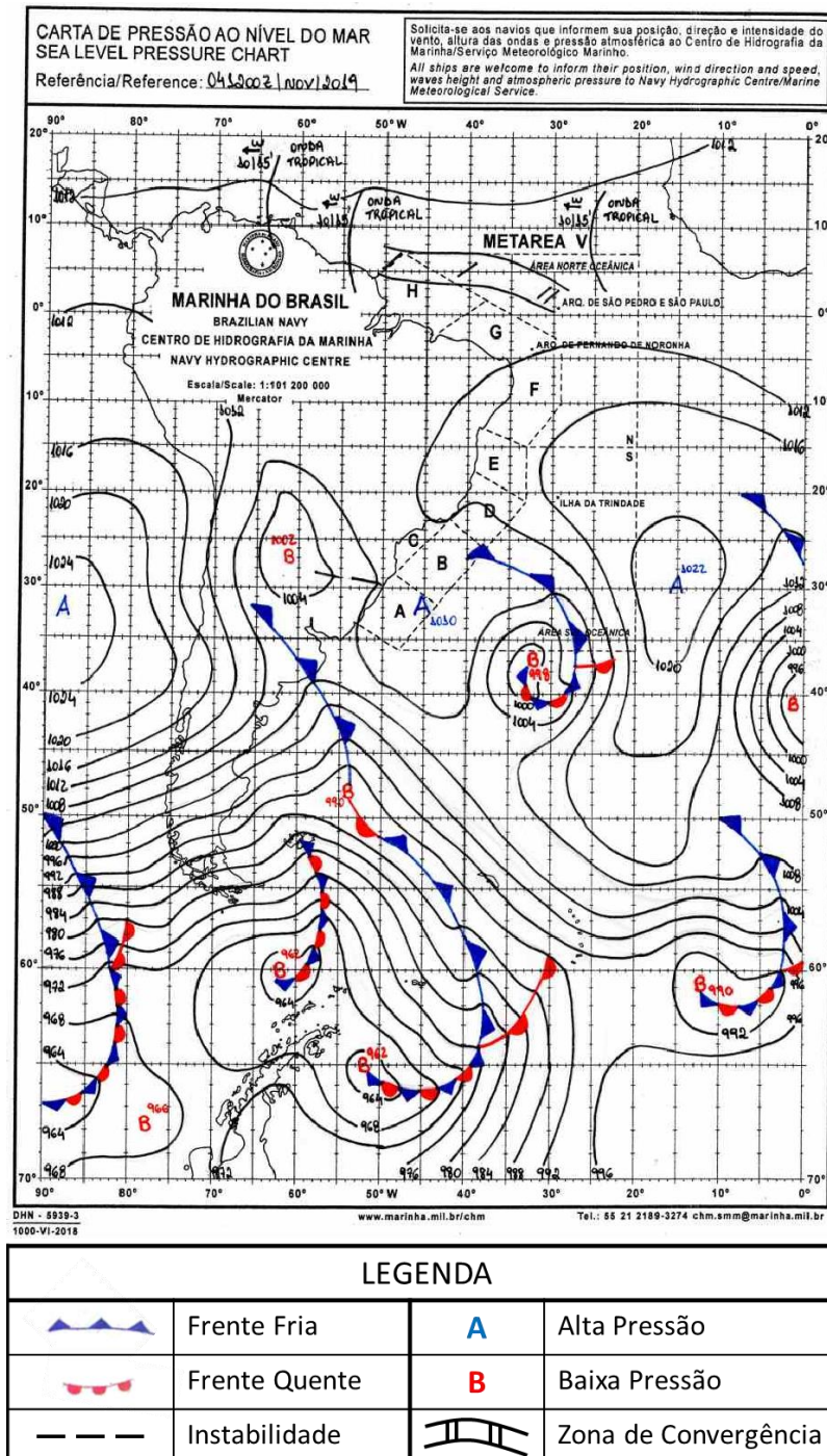
Figura A1 - Carta sinótica da Marinha do Brasil para as 1200Z do dia 04 de novembro de 2019 (0900 do dia 04 de novembro de 2019, hora local).
