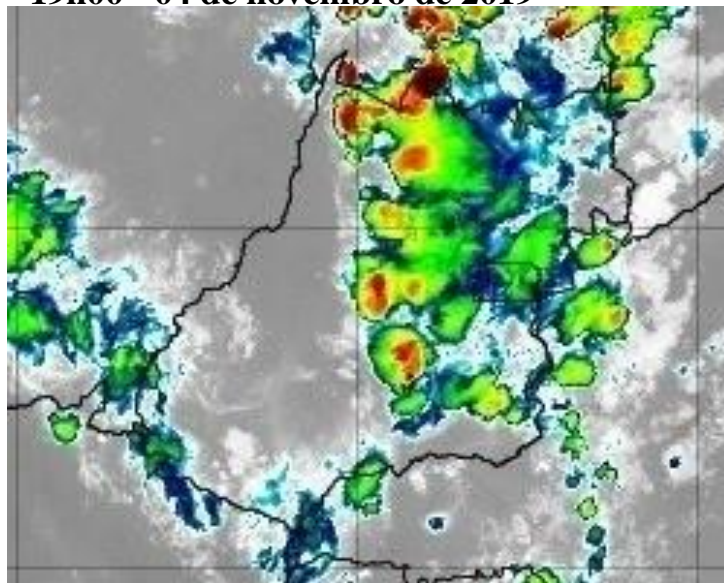
Figura 6 –Imagens realçadas do satélite GOES-16 das 19h00 do dia 04 de novembro de 2019. FONTE: Cptec/INPE.
