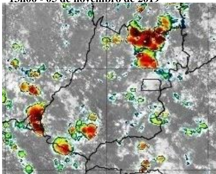
Figura 3 –Imagens realçadas do satélite GOES-16 das 13h00 do dia 05 de novembro de 2019. FONTE: Cptec/INPE.
