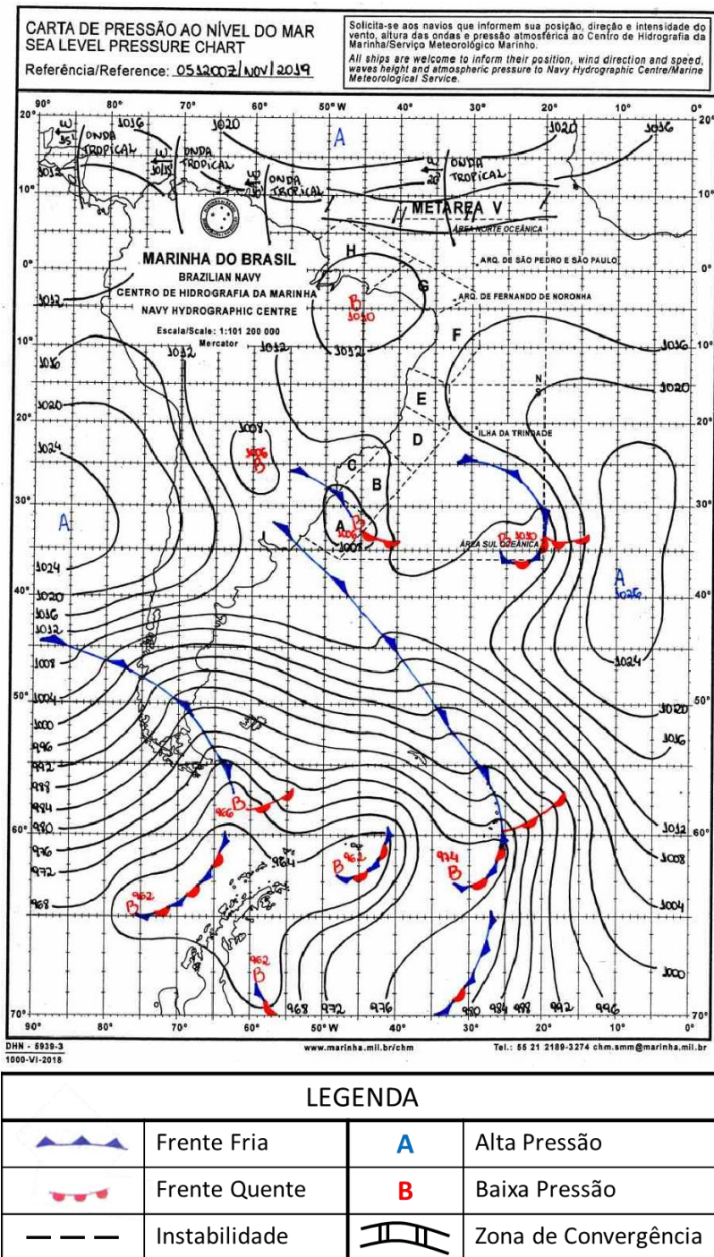
Figura A1 - Carta sinótica da Marinha do Brasil para as 1200Z do dia 05 de novembro de 2019 (09h00 do dia 05 de novembro de 2019, hora local).
