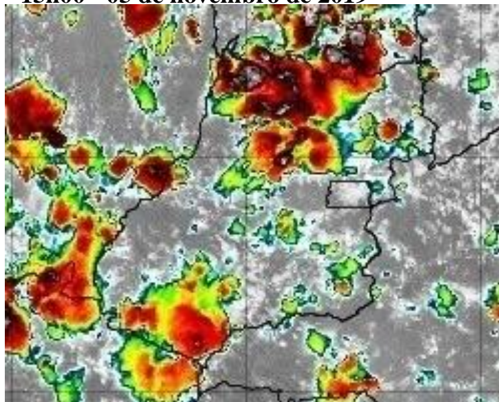
Figura 4 –Imagens realçadas do satélite GOES-16 das 15h00 do dia 05 de novembro de 2019. FONTE: Cptec/INPE.
