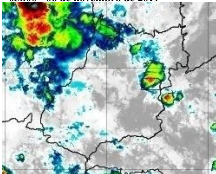
Figura 10 –Imagens realçadas do satélite GOES-16 das 03h00 do dia 06 de novembro de 2019. FONTE: Cptec/INPE.
