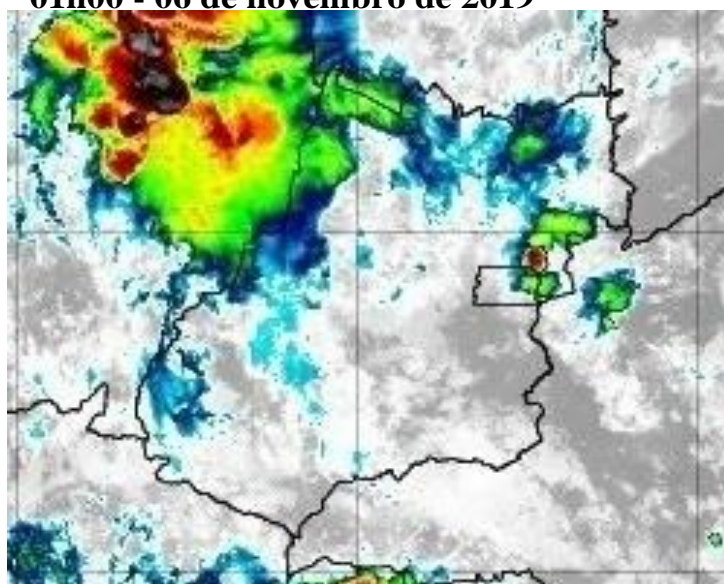
Figura 9 –Imagens realçadas do satélite GOES-16 das 01h00 do dia 06 de novembro de 2019. FONTE: Cptec/INPE.
