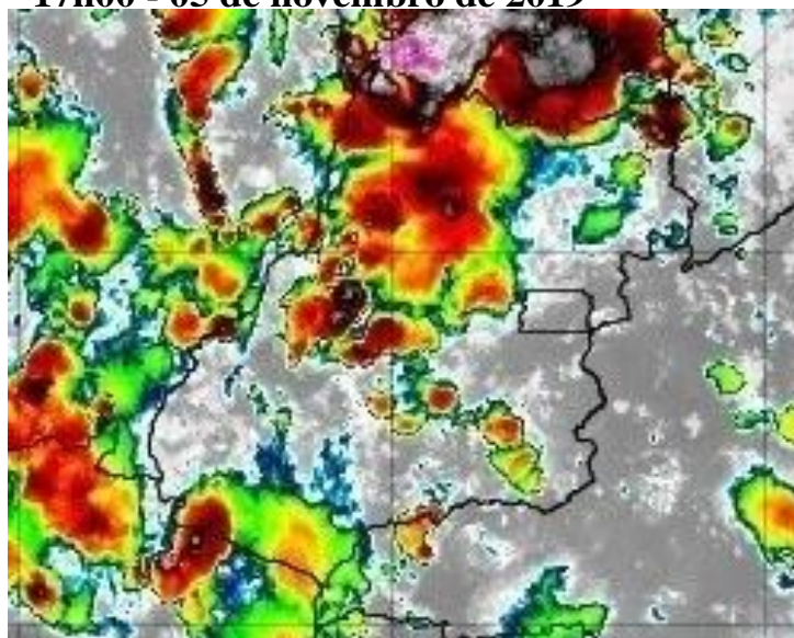
Figura 5 –Imagens realçadas do satélite GOES-16 das 17h00 do dia 05 de novembro de 2019. FONTE: Cptec/INPE.
