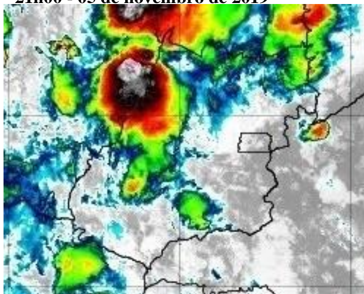
Figura 7 –Imagens realçadas do satélite GOES-16 das 21h00 do dia 05 de novembro de 2019. FONTE: Cptec/INPE.
