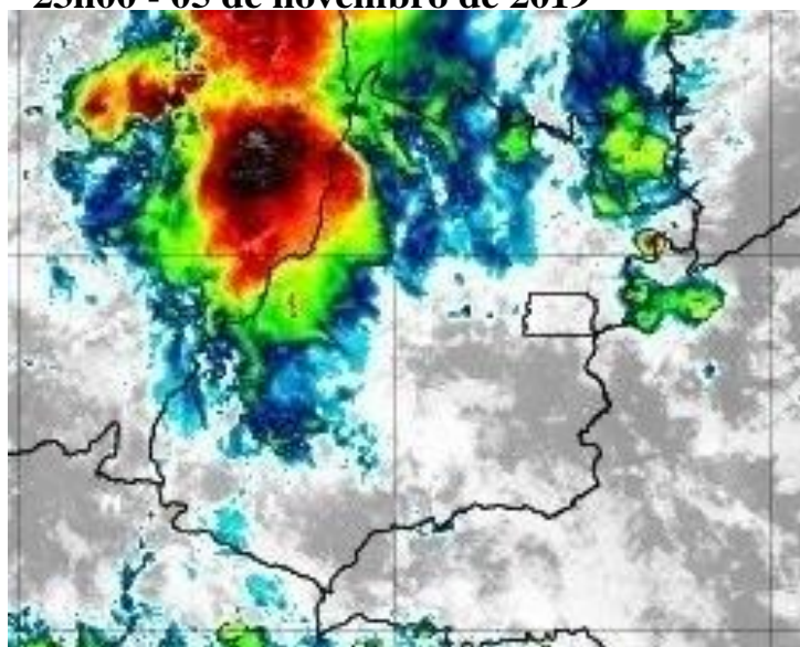
Figura 8 –Imagens realçadas do satélite GOES-16 das 23h00 do dia 05 de novembro de 2019. FONTE: Cptec/INPE.
