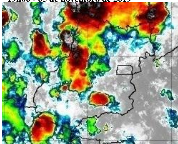
Figura 6 –Imagens realçadas do satélite GOES-16 das 19h00 do dia 05 de novembro de 2019. FONTE: Cptec/INPE.
