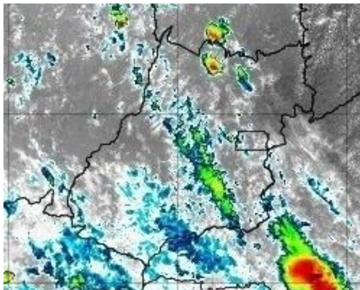
Figura 27 –Imagens realçadas do satélite GOES-16 das 13h00 do dia 08 de novembro de 2019. FONTE: Cptec/INPE.
