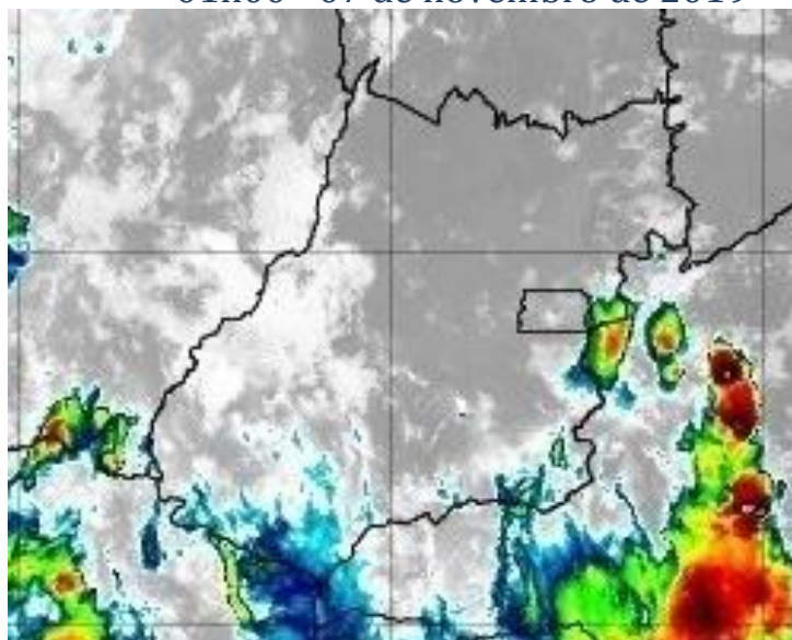
Figura 9 –Imagens realçadas do satélite GOES-16 das 01h00 do dia 07 de novembro de 2019. FONTE: Cptec/INPE.
