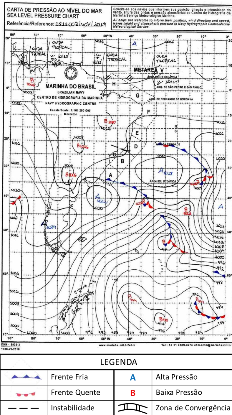
Figura A3 - Carta sinótica da Marinha do Brasil para as 1200Z do dia 08 de novembro de 2019 (09h00 do dia 08 de novembro de 2019, hora local).
