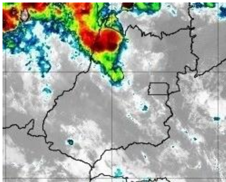
Figura 32 –Imagens realçadas do satélite GOES-16 das 23h00 do dia 08 de novembro de 2019. FONTE: Cptec/INPE.
