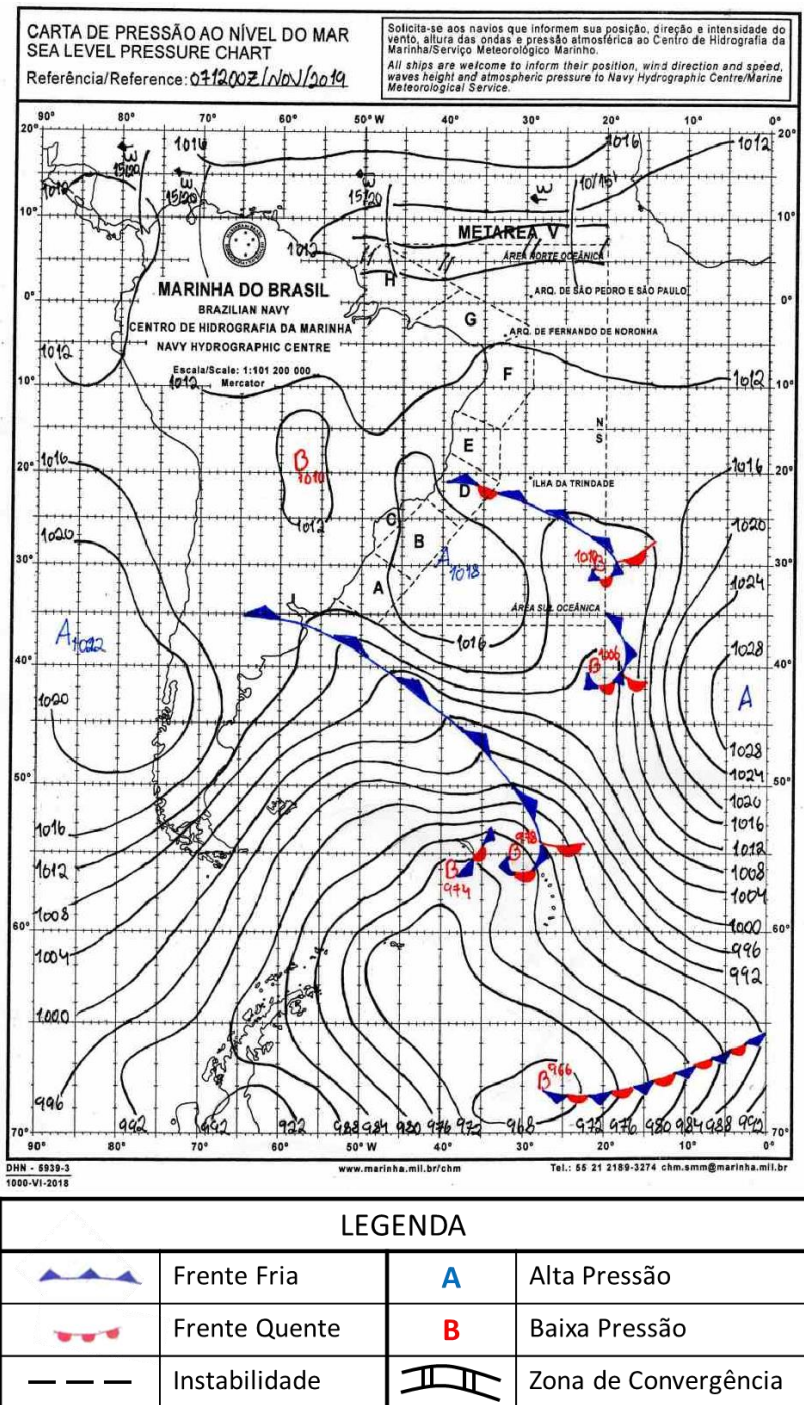
Figura A2 - Carta sinótica da Marinha do Brasil para as 1200Z do dia 07 de novembro de 2019 (09h00 do dia 07 de novembro de 2019, hora local).
