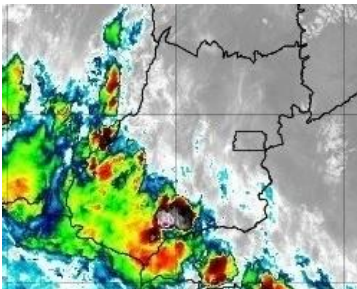
Figura 20 –Imagens realçadas do satélite GOES-16 das 23h00 do dia 07 de novembro de 2019. FONTE: Cptec/INPE.
