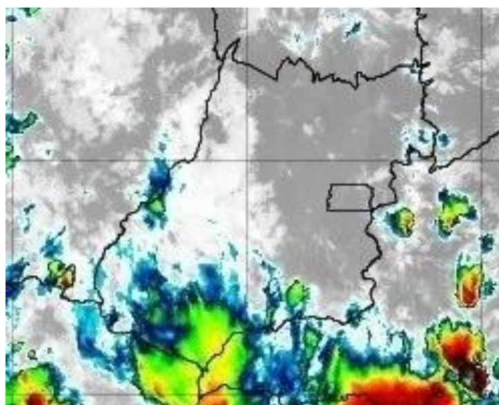
Figura 8 –Imagens realçadas do satélite GOES-16 das 23h00 do dia 06 de novembro de 2019. FONTE: Cptec/INPE.
