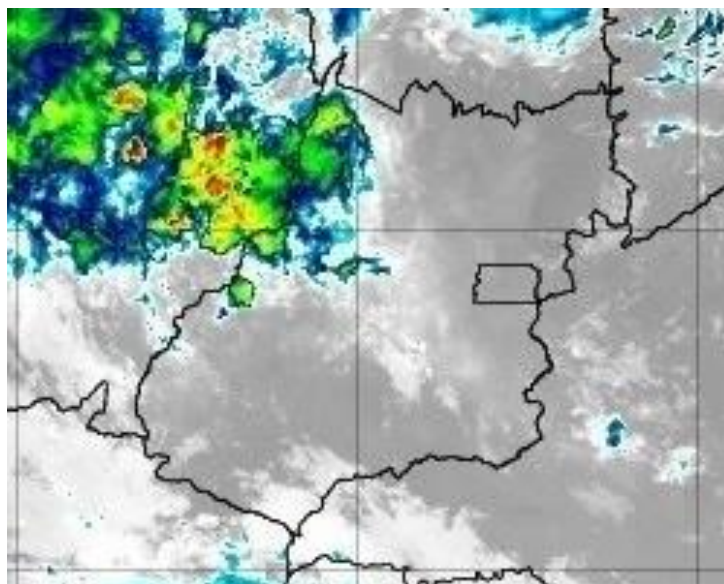
Figura 35 –Imagens realçadas do satélite GOES-16 das 05h00 do dia 09 de novembro de 2019. FONTE: Cptec/INPE.
