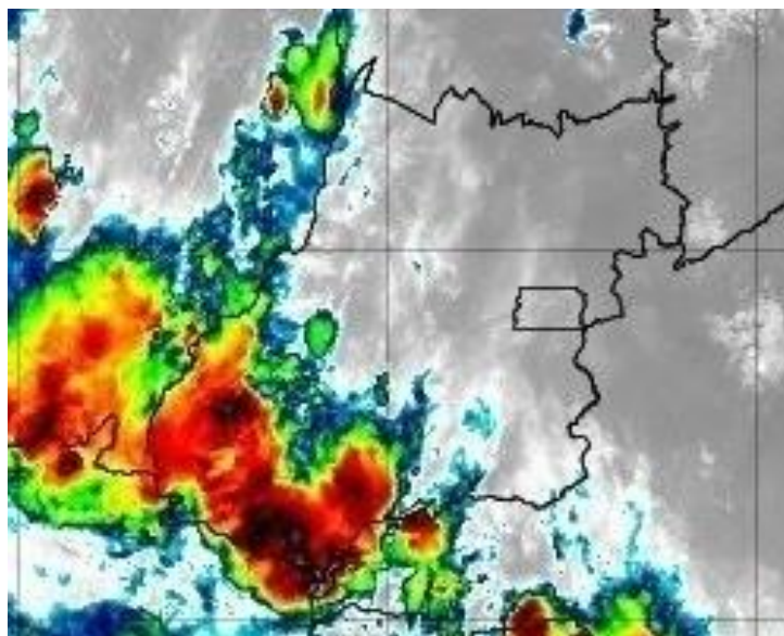
Figura 19 –Imagens realçadas do satélite GOES-16 das 21h00 do dia 07 de novembro de 2019. FONTE: Cptec/INPE.
