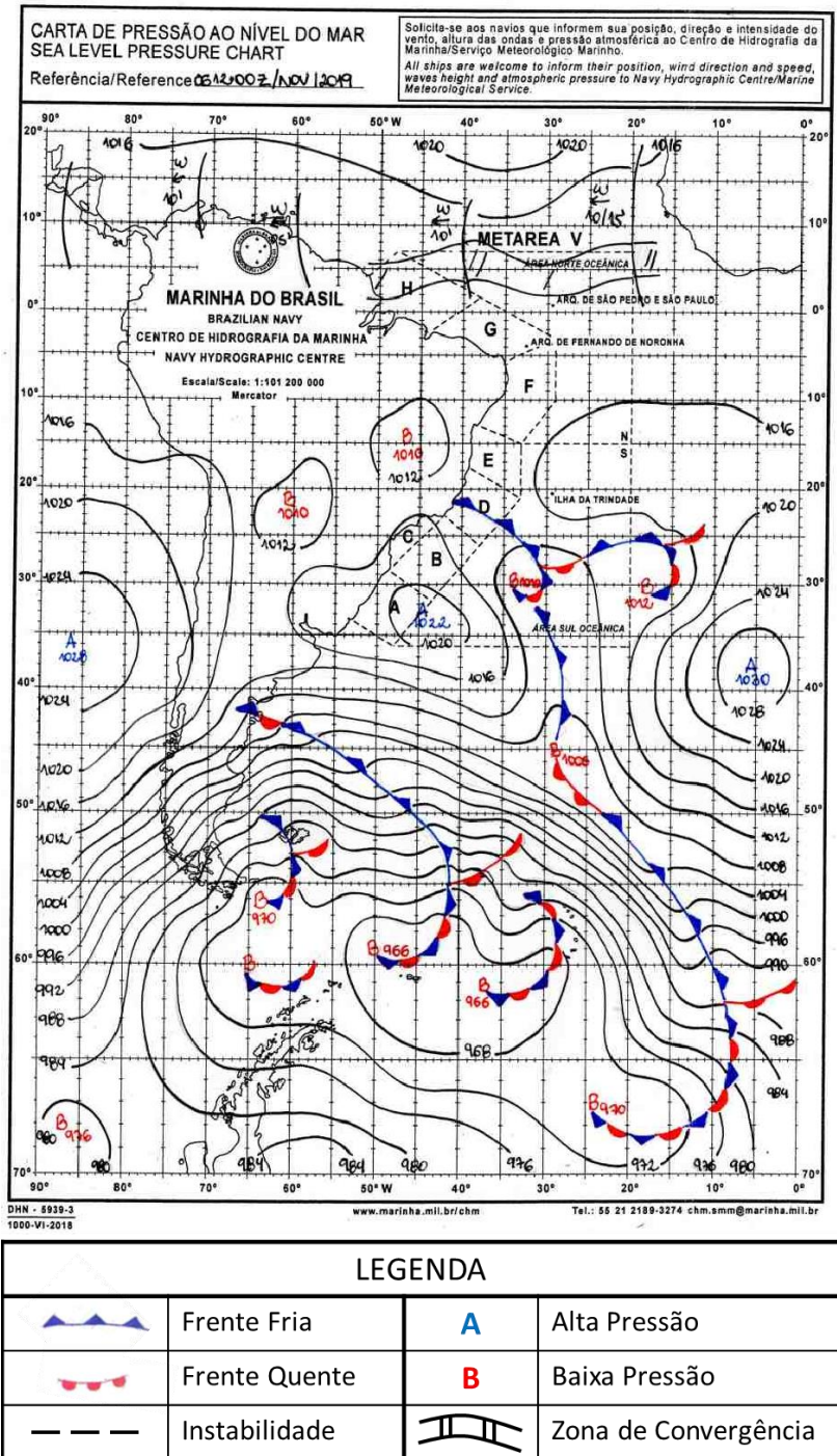
Figura A1 - Carta sinótica da Marinha do Brasil para as 1200Z do dia 06 de novembro de 2019 (09h00 do dia 06 de novembro de 2019, hora local).
