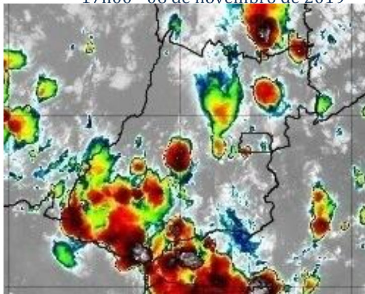
Figura 5 –Imagens realçadas do satélite GOES-16 das 17h00 do dia 06 de novembro de 2019. FONTE: Cptec/INPE.
