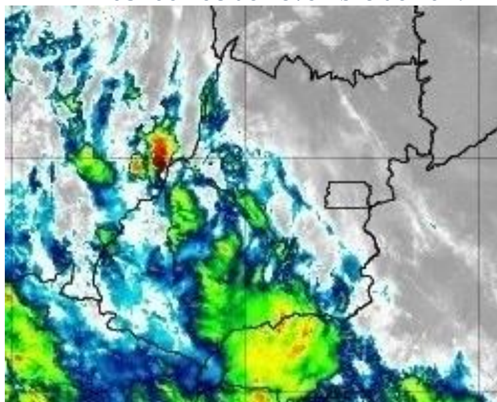
Figura 23 –Imagens realçadas do satélite GOES-16 das 05h00 do dia 08 de novembro de 2019. FONTE: Cptec/INPE.
