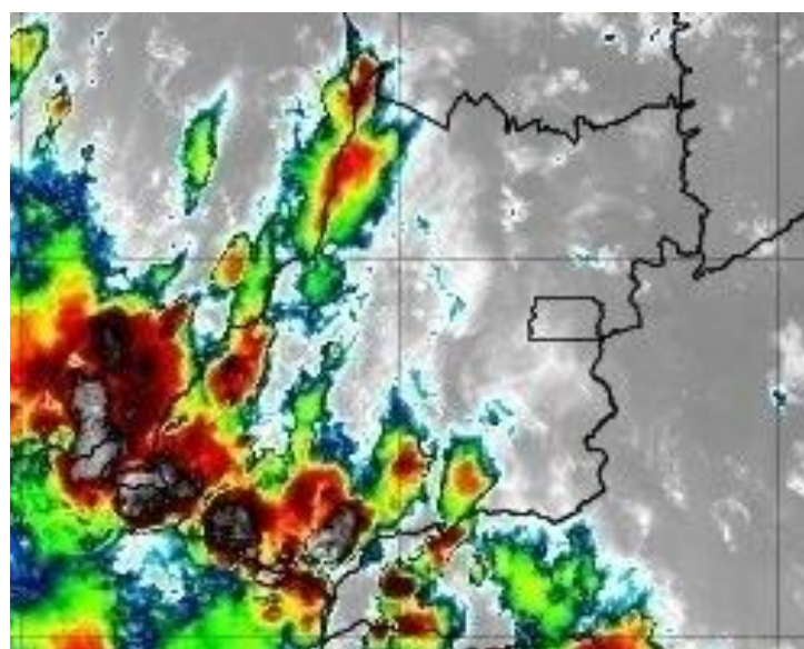
Figura 18 –Imagens realçadas do satélite GOES-16 das 19h00 do dia 07 de novembro de 2019. FONTE: Cptec/INPE.
