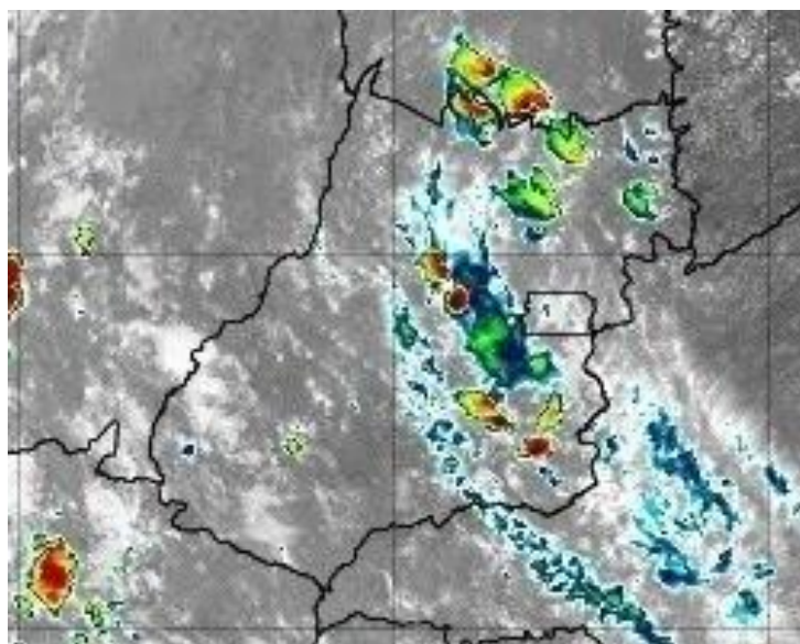
Figura 15 –Imagens realçadas do satélite GOES-16 das 13h00 do dia 07 de novembro de 2019. FONTE: Cptec/INPE.
