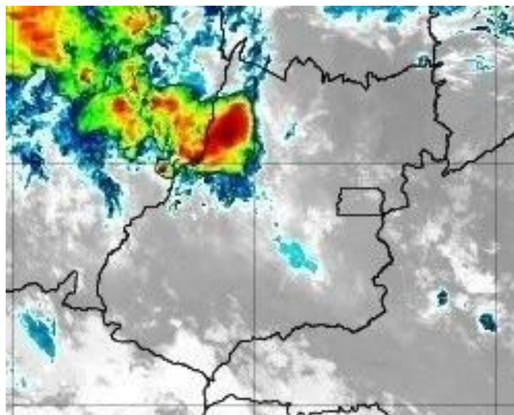
Figura 34 –Imagens realçadas do satélite GOES-16 das 03h00 do dia 09 de novembro de 2019. FONTE: Cptec/INPE.
