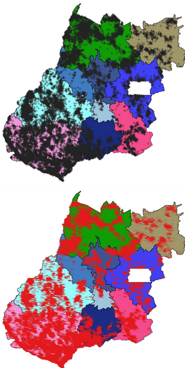
Figura 2 –Descargas atmosféricas nuvem-solo (em preto) e nuvem-nuvem (em vermelho) detectadas pelo sistema Earth Networks entre 10h00 do dia 06 e 05h00 do dia 09 de novembro de 2019 sobre a área de concessão da CELG Distribuição.
