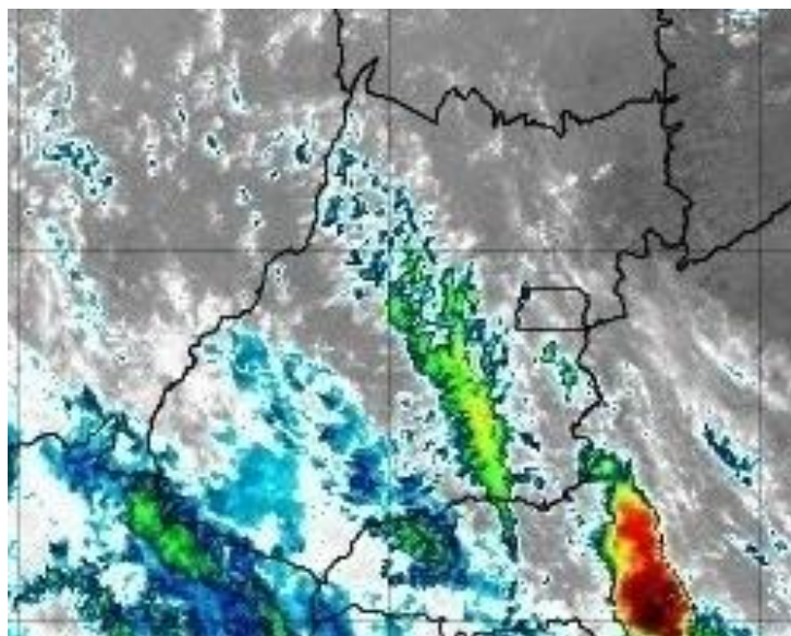
Figura 26 –Imagens realçadas do satélite GOES-16 das 11h00 do dia 08 de novembro de 2019. FONTE: Cptec/INPE.
