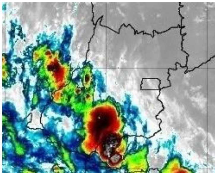
Figura 21 –Imagens realçadas do satélite GOES-16 das 01h00 do dia 08 de novembro de 2019. FONTE: Cptec/INPE.
