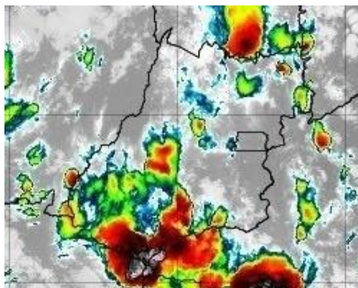
Figura 6 –Imagens realçadas do satélite GOES-16 das 19h00 do dia 06 de novembro de 2019. FONTE: Cptec/INPE.
