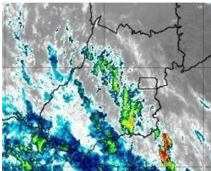
Figura 25 –Imagens realçadas do satélite GOES-16 das 09h00 do dia 08 de novembro de 2019. FONTE: Cptec/INPE.
