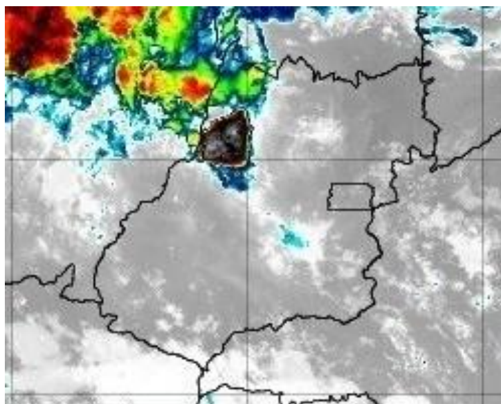
Figura 33 –Imagens realçadas do satélite GOES-16 das 01h00 do dia 09 de novembro de 2019. FONTE: Cptec/INPE.
