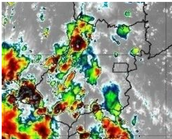
Figura 17 –Imagens realçadas do satélite GOES-16 das 17h00 do dia 07 de novembro de 2019. FONTE: Cptec/INPE.
