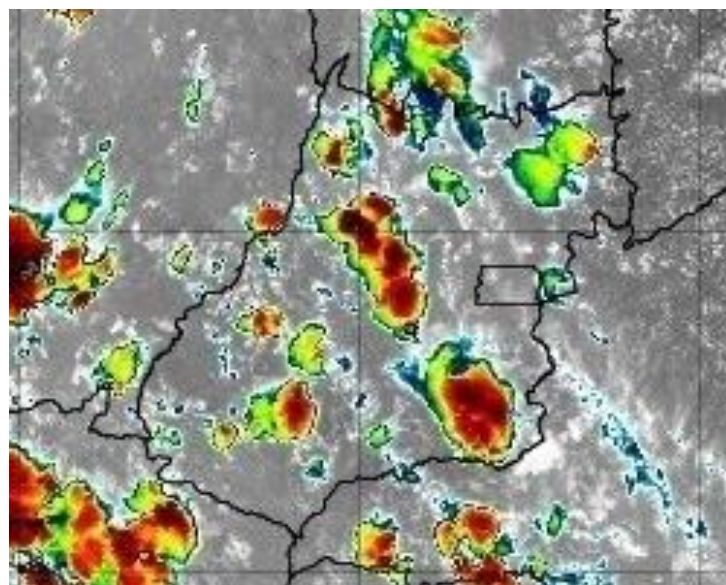
Figura 16 –Imagens realçadas do satélite GOES-16 das 15h00 do dia 07 de novembro de 2019. FONTE: Cptec/INPE.
