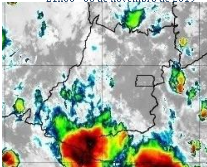
Figura 7 –Imagens realçadas do satélite GOES-16 das 21h00 do dia 06 de novembro de 2019. FONTE: Cptec/INPE.
