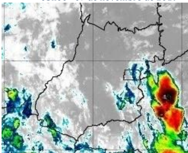
Figura 10 –Imagens realçadas do satélite GOES-16 das 03h00 do dia 07 de novembro de 2019. FONTE: Cptec/INPE.
