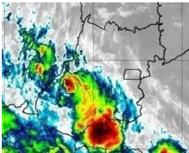
Figura 22 –Imagens realçadas do satélite GOES-16 das 03h00 do dia 08 de novembro de 2019. FONTE: Cptec/INPE.
