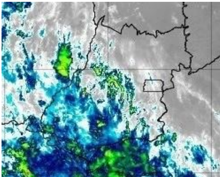
Figura 24 –Imagens realçadas do satélite GOES-16 das 07h00 do dia 08 de novembro de 2019. FONTE: Cptec/INPE.
