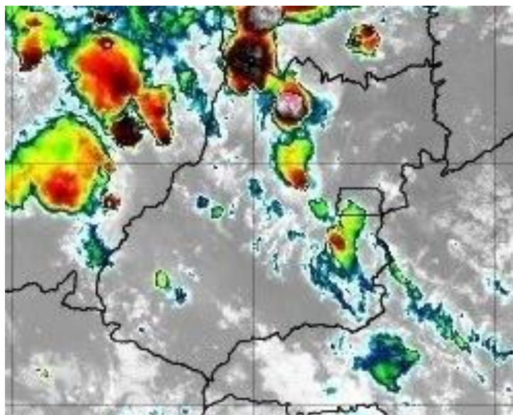
Figura 30 –Imagens realçadas do satélite GOES-16 das 19h00 do dia 08 de novembro de 2019. FONTE: Cptec/INPE.
