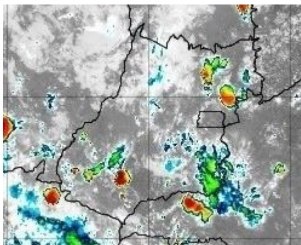
Figura 3 –Imagens realçadas do satélite GOES-16 das 13h00 do dia 06 de novembro de 2019. FONTE: Cptec/INPE.
