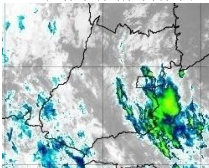
Figura 12 –Imagens realçadas do satélite GOES-16 das 07h00 do dia 07 de novembro de 2019. FONTE: Cptec/INPE.
