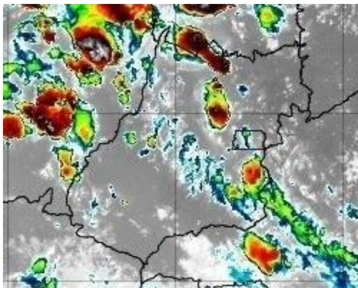
Figura 29 –Imagens realçadas do satélite GOES-16 das 17h00 do dia 08 de novembro de 2019. FONTE: Cptec/INPE.
