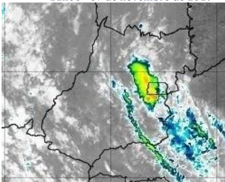
Figura 14 –Imagens realçadas do satélite GOES-16 das 11h00 do dia 07 de novembro de 2019. FONTE: Cptec/INPE.
