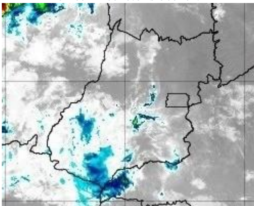
Figura 13 – Imagens realçadas do satélite GOES-16 das 07h00 do dia 12 de novembro de 2019. FONTE: Cptec/INPE.
