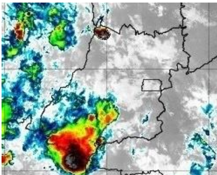
Figura 9 – Imagens realçadas do satélite GOES-16 das 23h00 do dia 11 de novembro de 2019. FONTE: Cptec/INPE.
