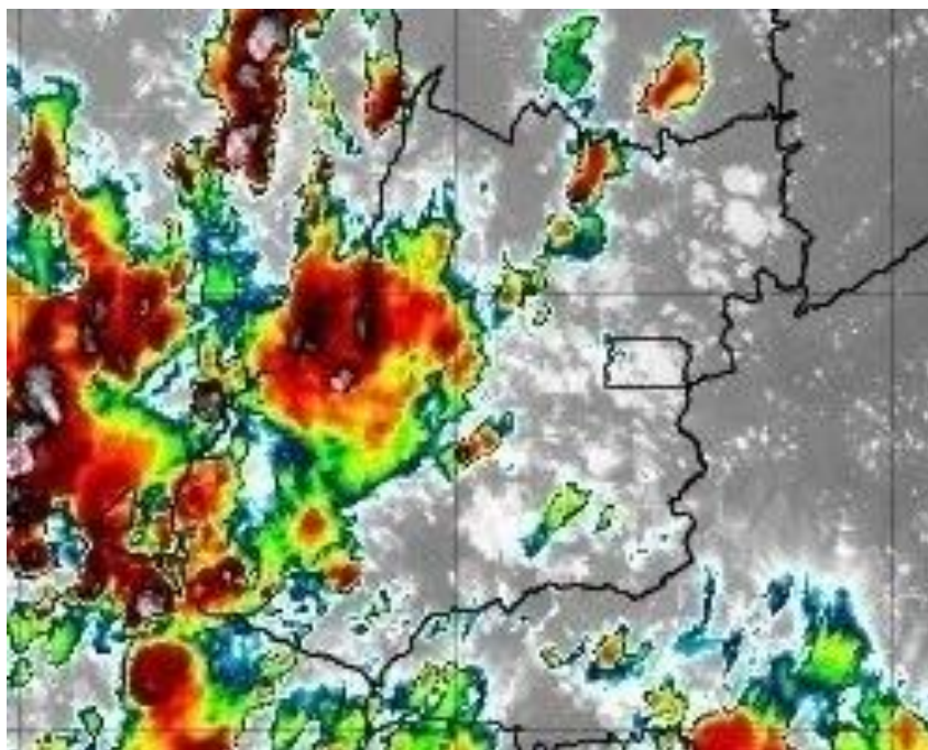
Figura 6 – Imagens realçadas do satélite GOES-16 das 17h00 do dia 11 de novembro de 2019. FONTE: Cptec/INPE.
