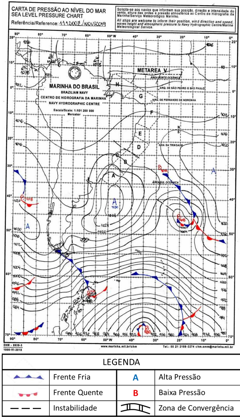
Figura A1 - Carta sinótica da Marinha do Brasil para as 1200Z do dia 11 de novembro de 2019 (09h00 do dia 11 de novembro de 2019, hora local).
