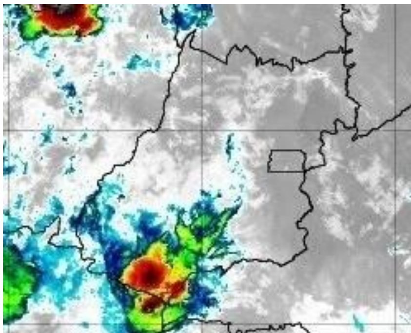
Figura 11 – Imagens realçadas do satélite GOES-16 das 03h00 do dia 12 de novembro de 2019. FONTE: Cptec/INPE.
