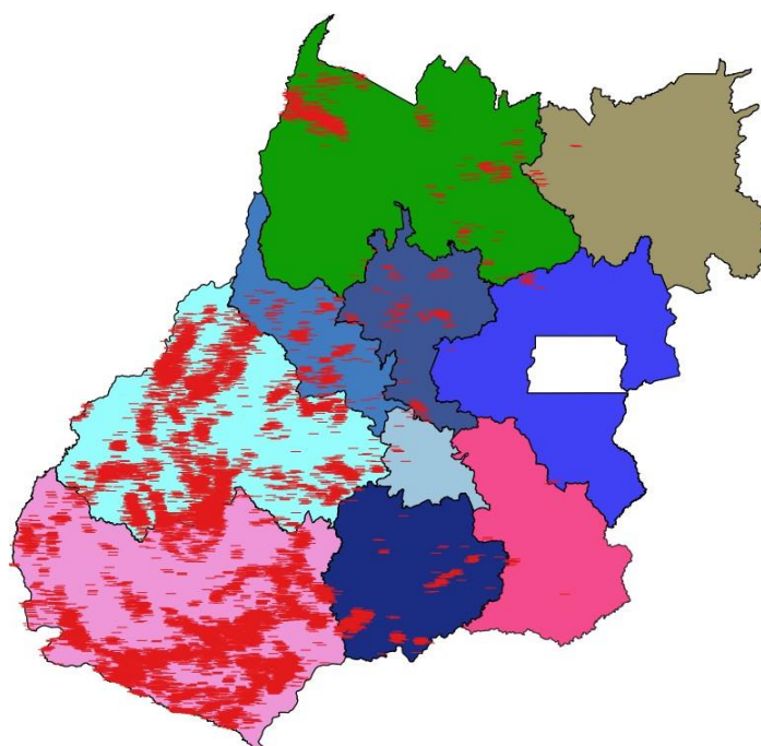
Figura 3 – Descargas atmosféricas nuvem-nuvem (em vermelho) detectadas pelo sistema Earth Networks entre 10h30 do dia 11 e as 03h00 do dia 12 de novembro de 2019 sobre a área de concessão da CELG Distribuição.
