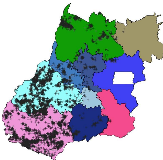
Figura 2 – Descargas atmosféricas nuvem-solo (em preto) detectadas pelo sistema Earth Networks entre 10h30 do dia 11 e as 03h00 do dia 12 de novembro de 2019 sobre a área de concessão da CELG Distribuição.
