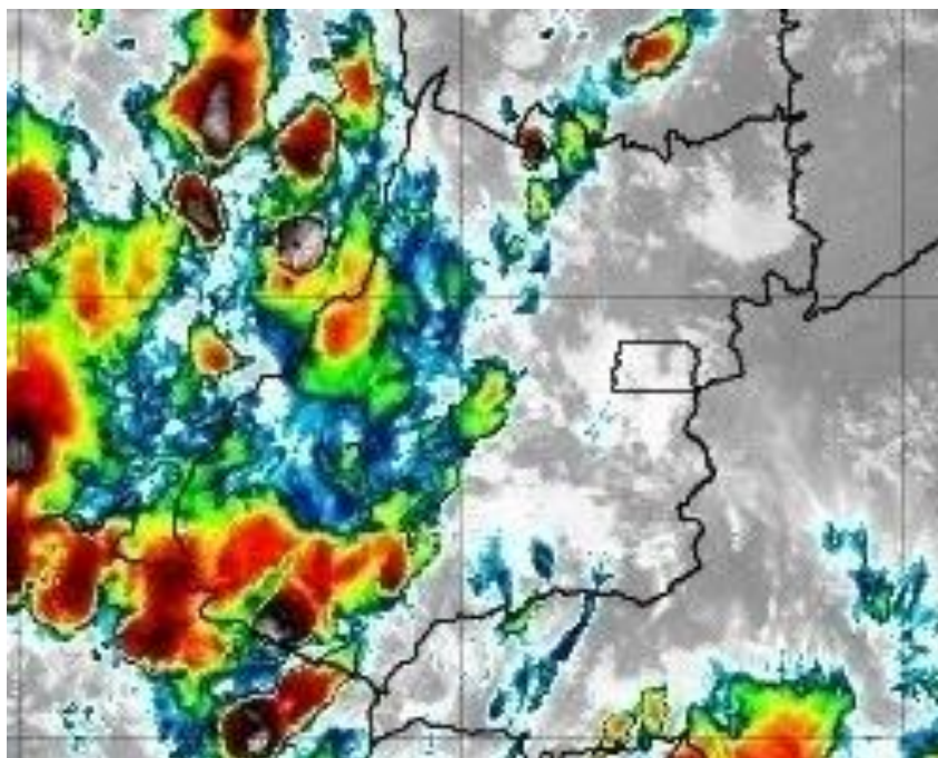
Figura 7 – Imagens realçadas do satélite GOES-16 das 19h00 do dia 11 de novembro de 2019. FONTE: Cptec/INPE.
