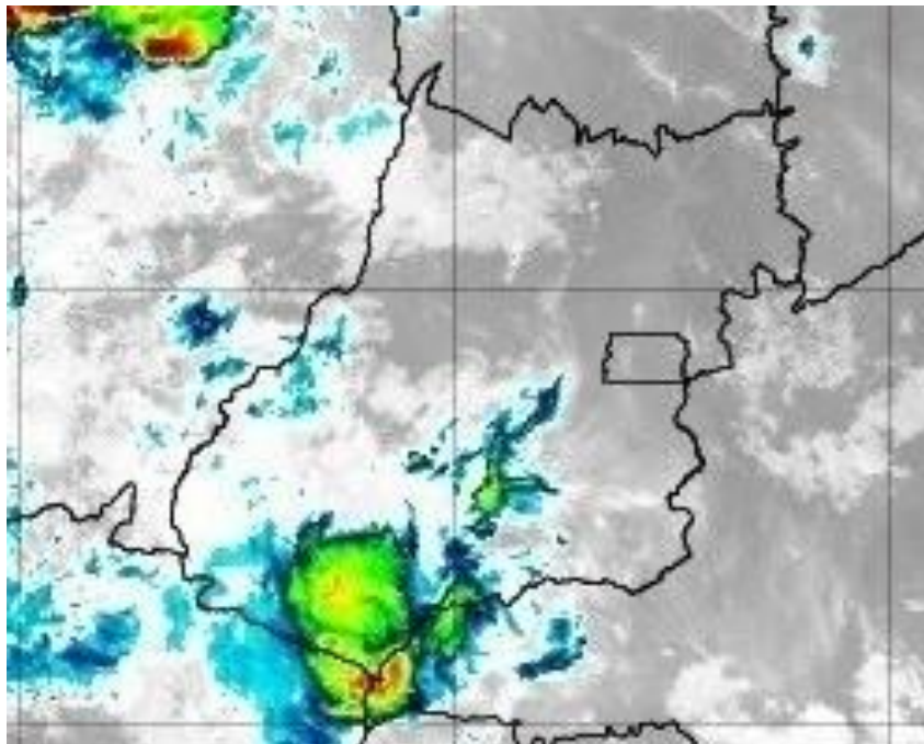
Figura 12 – Imagens realçadas do satélite GOES-16 das 05h00 do dia 12 de novembro de 2019. FONTE: Cptec/INPE.
