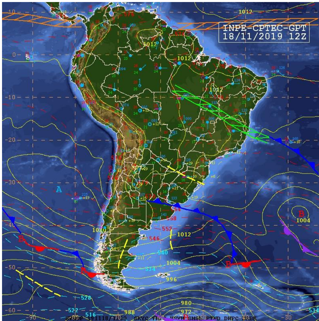
Figura A5 - Carta sinótica da Marinha do Brasil para as 1200Z do dia 18 de novembro de 2019 (09h00 do dia 18 de novembro de 2019, hora local). FONTE:CPTEC).
