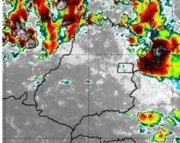
Figura 18 –Imagens realçadas do satélite GOES-16 das 17h00 do dia 16 de novembro de 2019. FONTE: Cptec/INPE.
