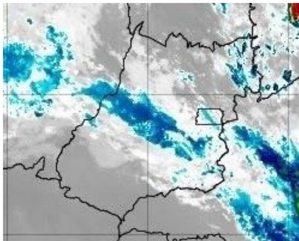
Figura 15 –Imagens realçadas do satélite GOES-16 das 05h00 do dia 16 de novembro de 2019. FONTE: Cptec/INPE.
