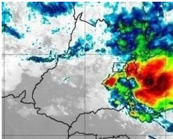
Figura 29 –Imagens realçadas do satélite GOES-16 das 05h00 do dia 18 de novembro de 2019. FONTE: Cptec/INPE.
