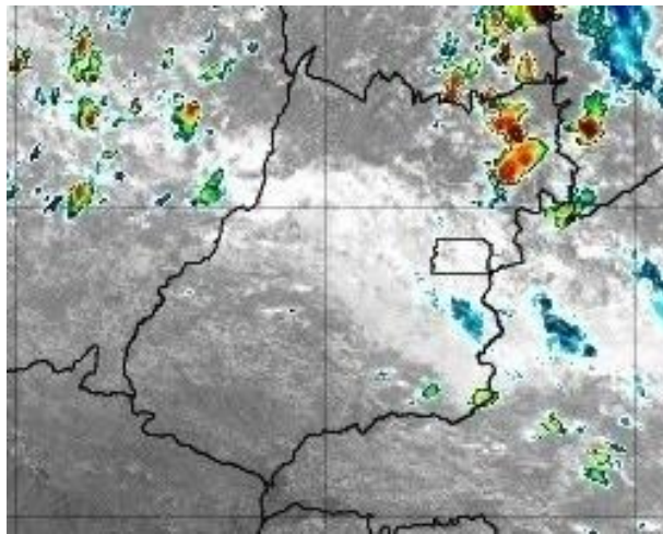
Figura 17 –Imagens realçadas do satélite GOES-16 das 13h00 do dia 16 de novembro de 2019. FONTE: Cptec/INPE.
