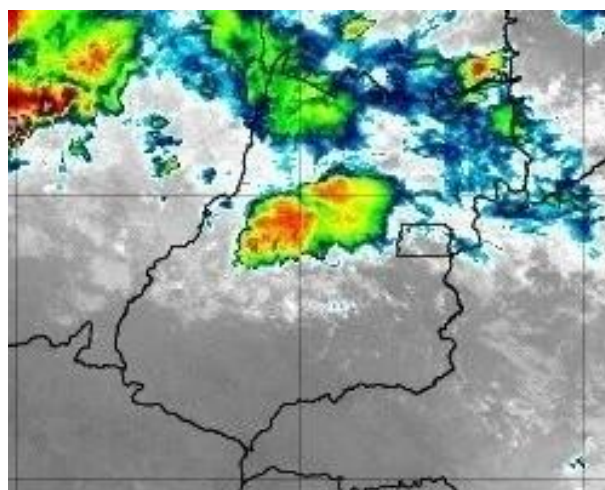
Figura 23 –Imagens realçadas do satélite GOES-16 das 09h00 do dia 17 de novembro de 2019. FONTE: Cptec/INPE.
