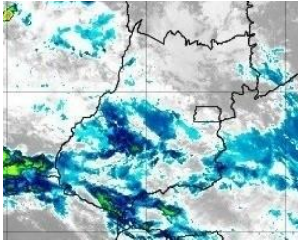
Figura 36 –Imagens realçadas do satélite GOES-16 das 05h00 do dia 19 de novembro de 2019. FONTE: Cptec/INPE.
