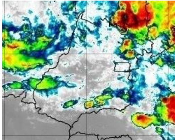
Figura 26 –Imagens realçadas do satélite GOES-16 das 21h00 do dia 17 de novembro de 2019. FONTE: Cptec/INPE.
