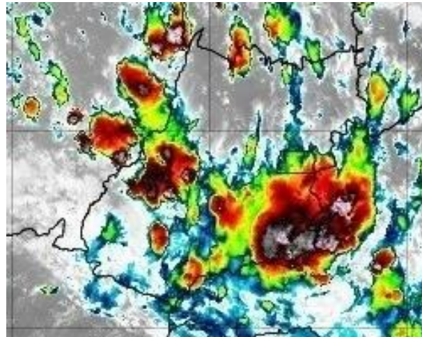
Figura 11 –Imagens realçadas do satélite GOES-16 das 17h00 do dia 15 de novembro de 2019. FONTE: Cptec/INPE.
