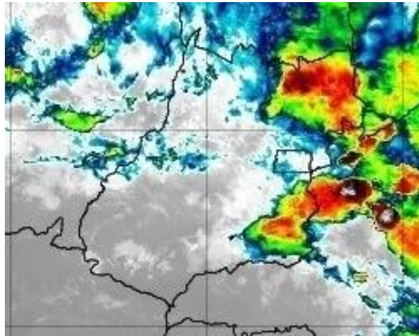
Figura 27 –Imagens realçadas do satélite GOES-16 das 01h00 do dia 18 de novembro de 2019. FONTE: Cptec/INPE.
