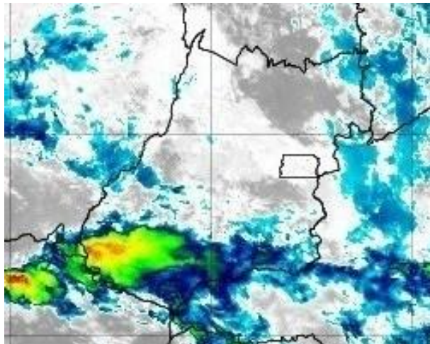
Figura 35 –Imagens realçadas do satélite GOES-16 das 01h00 do dia 19 de novembro de 2019. FONTE: Cptec/INPE.
