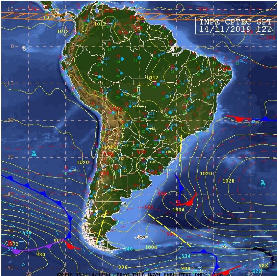
Figura A1 - Carta sinótica para as 1200Z do dia 14 de novembro de 2019 (09h00 do dia 14 de novembro de 2019, hora local. FONTE:CPTEC).
