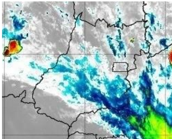
Figura 13 –Imagens realçadas do satélite GOES-16 das 01h00 do dia 16 de novembro de 2019. FONTE: Cptec/INPE.
