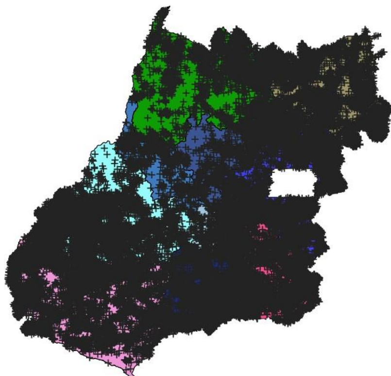
Figura 2 – Descargas atmosféricas nuvem-solo (em preto) detectadas pelo sistema Earth Networks entre 06h30 do dia 14 e 02h30 do dia 21 de novembro de 2019 sobre a área de concessão da CELG Distribuição.
