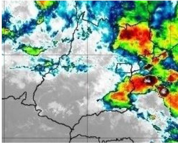
Figura 28 –Imagens realçadas do satélite GOES-16 das 01h00 do dia 18 de novembro de 2019. FONTE: Cptec/INPE.
