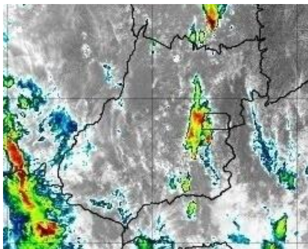
Figura 4 –Imagens realçadas do satélite GOES-16 das 13h00 do dia 14 de novembro de 2019. FONTE: Cptec/INPE.
