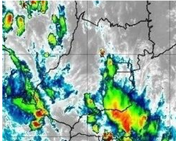
Figura 6 –Imagens realçadas do satélite GOES-16 das 21h00 do dia 14 de novembro de 2019. FONTE: Cptec/INPE.
