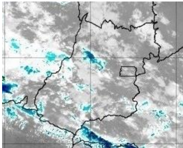
Figura 37 –Imagens realçadas do satélite GOES-16 das 09h00 do dia 19 de novembro de 2019. FONTE: Cptec/INPE.
