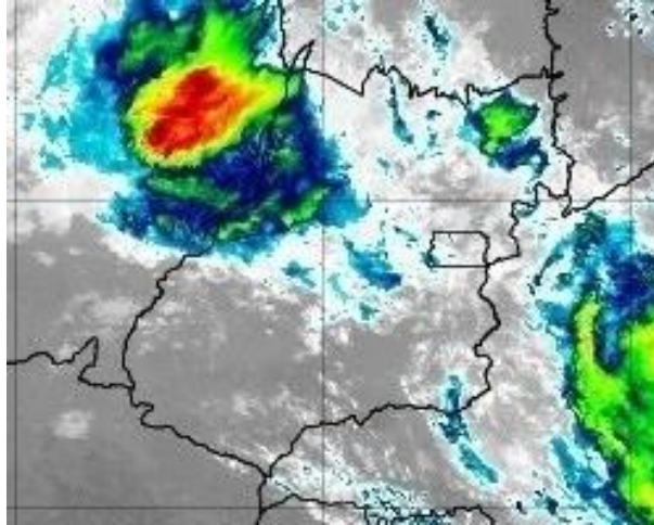
Figura 44 –Imagens realçadas do satélite GOES-16 das 09h00 do dia 20 de novembro de 2019. FONTE: Cptec/INPE.
