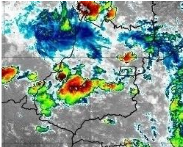
Figura 45 –Imagens realçadas do satélite GOES-16 das 13h00 do dia 20 de novembro de 2019. FONTE: Cptec/INPE.
