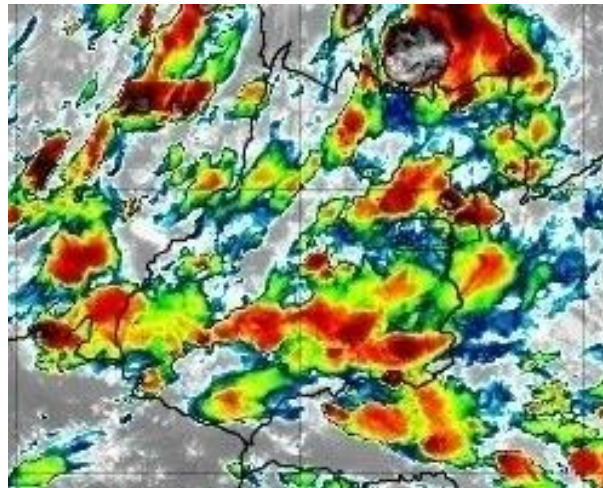
Figura 39 –Imagens realçadas do satélite GOES-16 das 17h00 do dia 19 de novembro de 2019. FONTE: Cptec/INPE.
