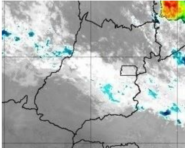
Figura 16 –Imagens realçadas do satélite GOES-16 das 09h00 do dia 16 de novembro de 2019. FONTE: Cptec/INPE.
