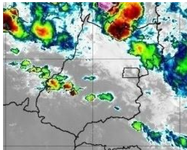
Figura 19 –Imagens realçadas do satélite GOES-16 das 21h00 do dia 16 de novembro de 2019. FONTE: Cptec/INPE.
