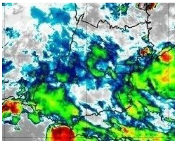
Figura 47 –Imagens realçadas do satélite GOES-16 das 21h00 do dia 20 de novembro de 2019. FONTE: Cptec/INPE.
