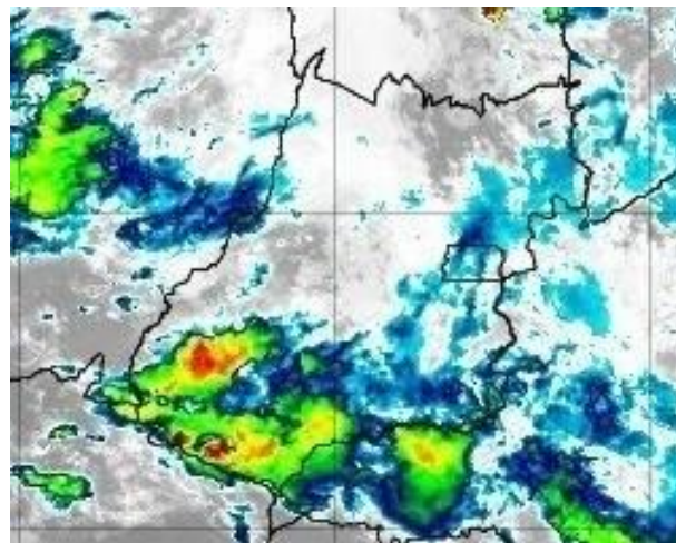
Figura 33 –Imagens realçadas do satélite GOES-16 das 21h00 do dia 18 de novembro de 2019. FONTE: Cptec/INPE.
