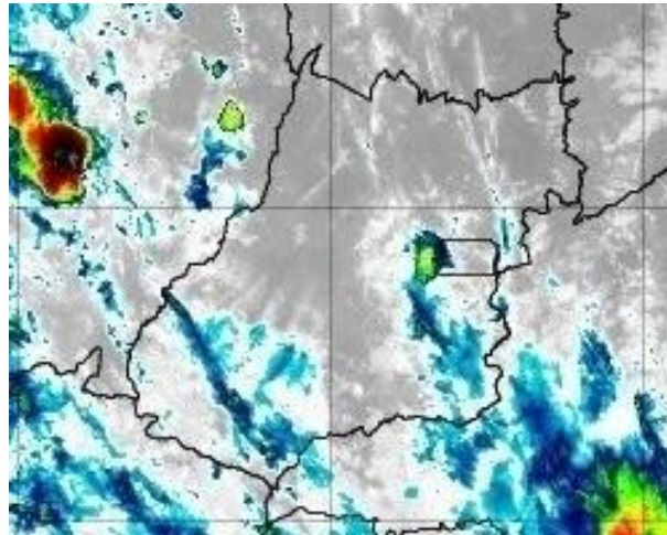
Figura 7 –Imagens realçadas do satélite GOES-16 das 01h00 do dia 15 de novembro de 2019. FONTE: Cptec/INPE.
