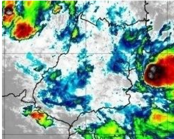
Figura 42 –Imagens realçadas do satélite GOES-16 das 01h00 do dia 20 de novembro de 2019. FONTE: Cptec/INPE.
