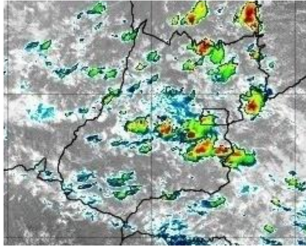
Figura 38 –Imagens realçadas do satélite GOES-16 das 13h00 do dia 19 de novembro de 2019. FONTE: Cptec/INPE.
