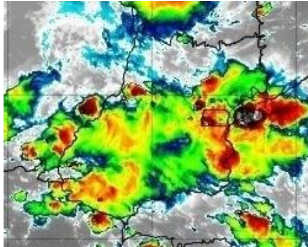
Figura 46 –Imagens realçadas do satélite GOES-16 das 17h00 do dia 20 de novembro de 2019. FONTE: Cptec/INPE.
