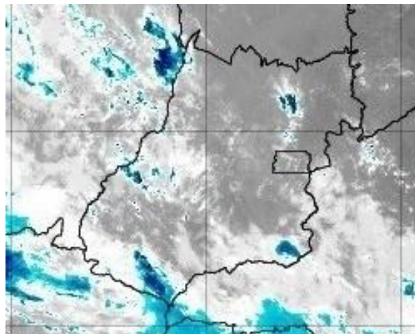
Figura 9 –Imagens realçadas do satélite GOES-16 das 09h00 do dia 15 de novembro de 2019. FONTE: Cptec/INPE.
