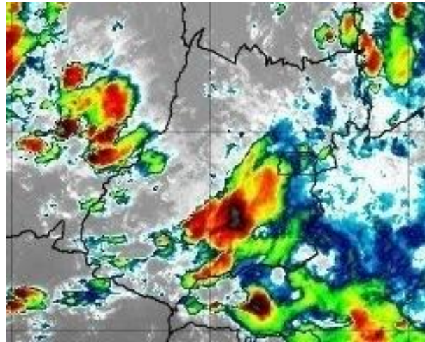
Figura 32 –Imagens realçadas do satélite GOES-16 das 17h00 do dia 18 de novembro de 2019. FONTE: Cptec/INPE.
