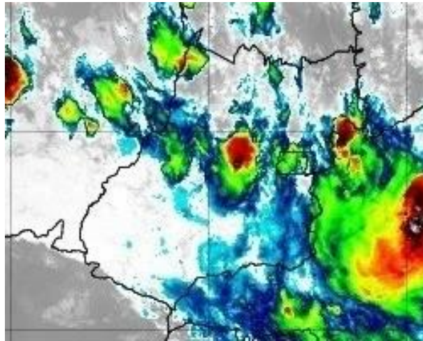
Figura 12 –Imagens realçadas do satélite GOES-16 das 21h00 do dia 15 de novembro de 2019. FONTE: Cptec/INPE.
