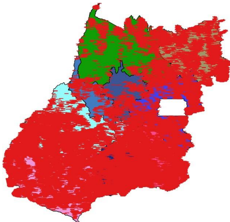
Figura 3 –Descargas atmosféricas nuvem-nuvem (em vermelho) detectadas pelo sistema Earth Networks entre 06h30 do dia 14 e 02h30 do dia 21 de novembro de 2019 sobre a área de concessão da CELG Distribuição.
