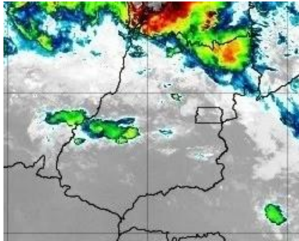
Figura 20 –Imagens realçadas do satélite GOES-16 das 01h00 do dia 17 de novembro de 2019. FONTE: Cptec/INPE.
