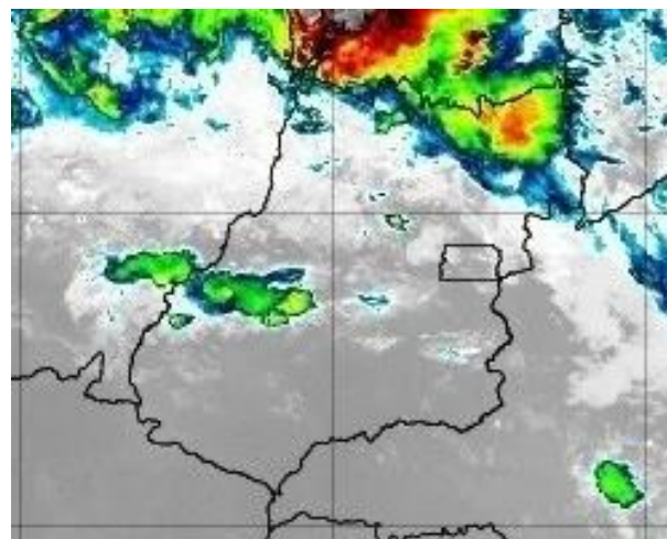
Figura 21 –Imagens realçadas do satélite GOES-16 das 01h00 do dia 17 de novembro de 2019. FONTE: Cptec/INPE.
