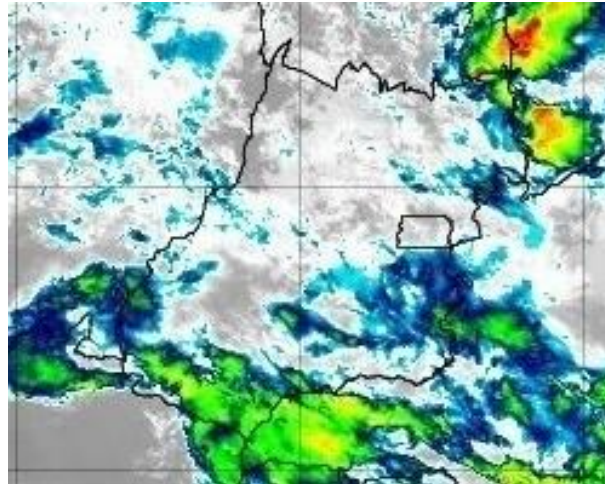
Figura 48 –Imagens realçadas do satélite GOES-16 das 01h00 do dia 21 de novembro de 2019. FONTE: Cptec/INPE.
