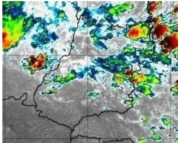
Figura 24 –Imagens realçadas do satélite GOES-16 das 13h00 do dia 17 de novembro de 2019. FONTE: Cptec/INPE.
