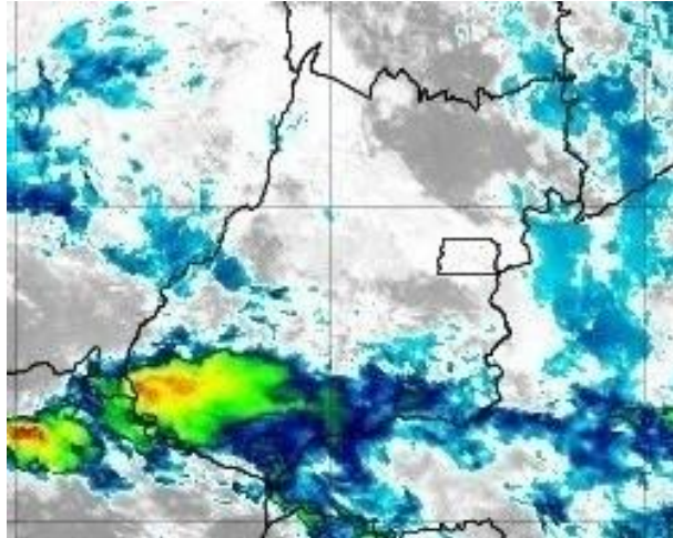
Figura 34 –Imagens realçadas do satélite GOES-16 das 01h00 do dia 19 de novembro de 2019. FONTE: Cptec/INPE.
