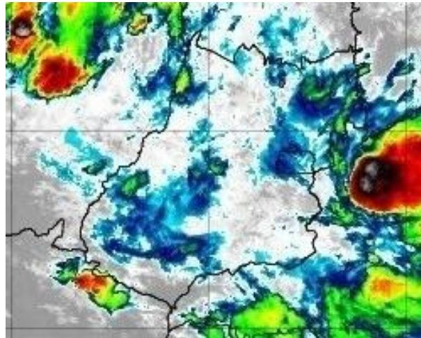
Figura 41 –Imagens realçadas do satélite GOES-16 das 01h00 do dia 20 de novembro de 2019. FONTE: Cptec/INPE.
