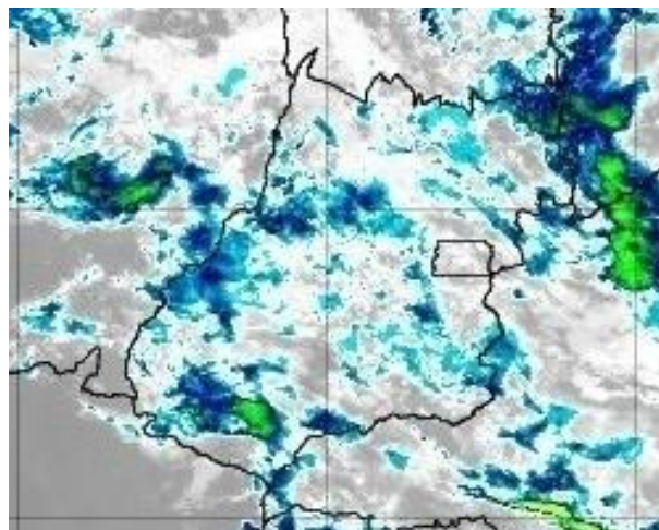
Figura 49 –Imagens realçadas do satélite GOES-16 das 05h00 do dia 21 de novembro de 2019. FONTE: Cptec/INPE.
