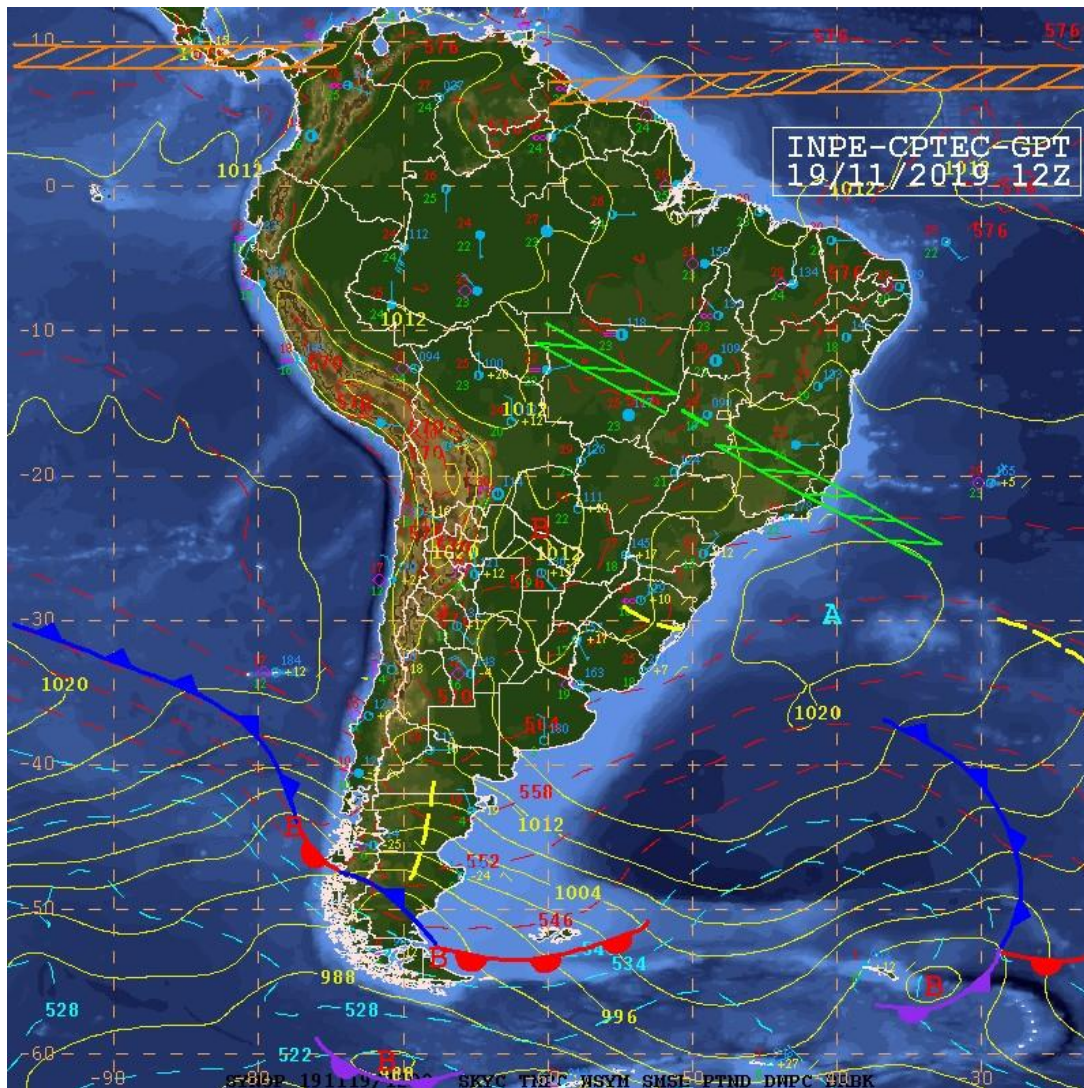
Figura A6 - Carta sinótica da Marinha do Brasil para as 1200Z do dia 19 de novembro de 2019 (09h00 do dia 19 de novembro de 2019, hora local). FONTE:CPTEC).
