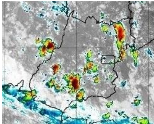
Figura 10 –Imagens realçadas do satélite GOES-16 das 13h00 do dia 15 de novembro de 2019. FONTE: Cptec/INPE.
