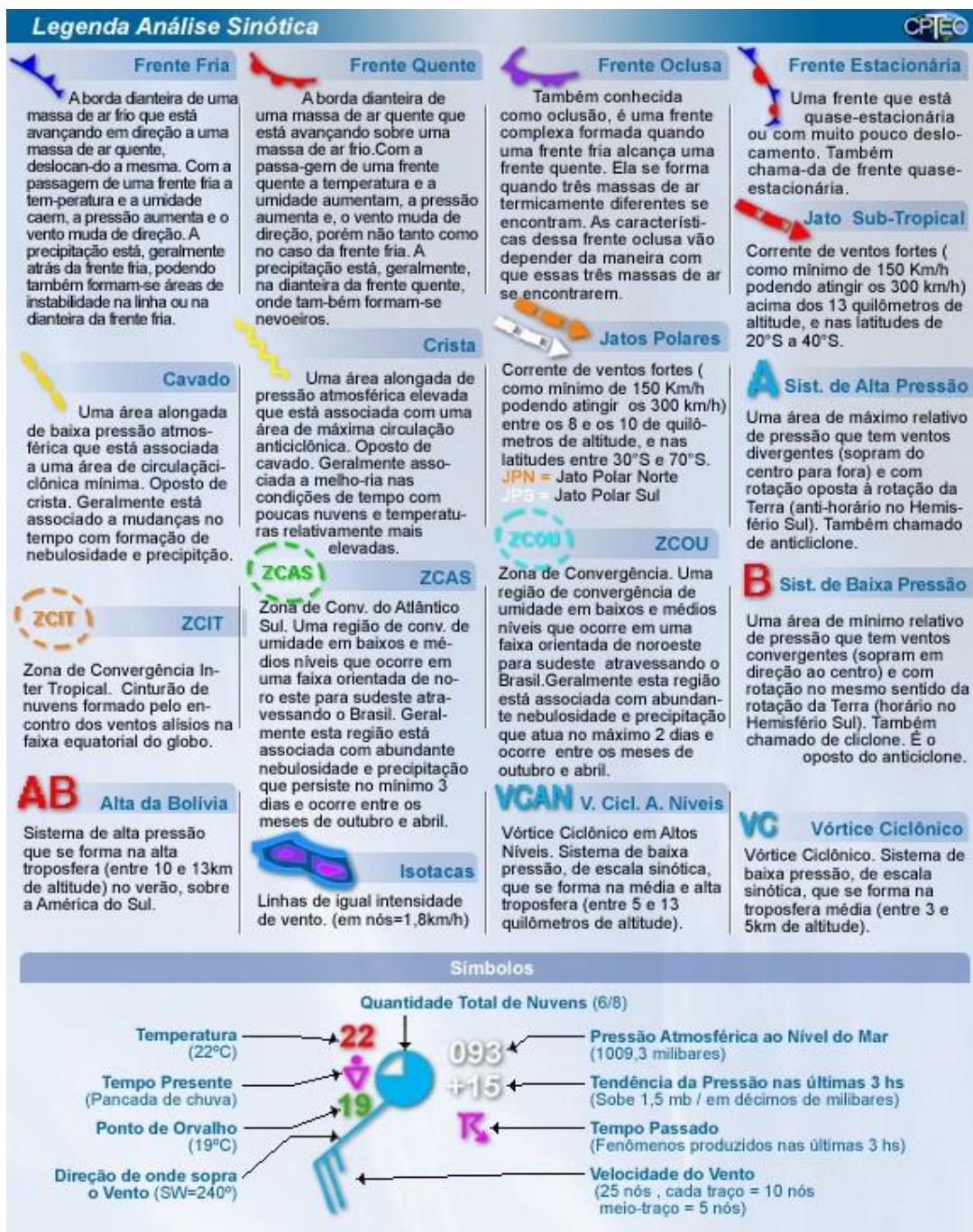
Figura A8 - Legenda das cartas sinóticas apresentadas acima. FONTE:CPTEC
