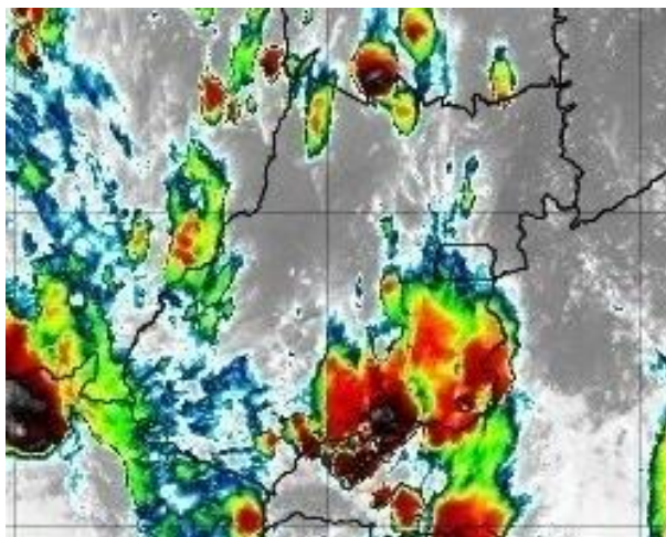
Figura 5 –Imagens realçadas do satélite GOES-16 das 17h00 do dia 14 de novembro de 2019. FONTE: Cptec/INPE.
