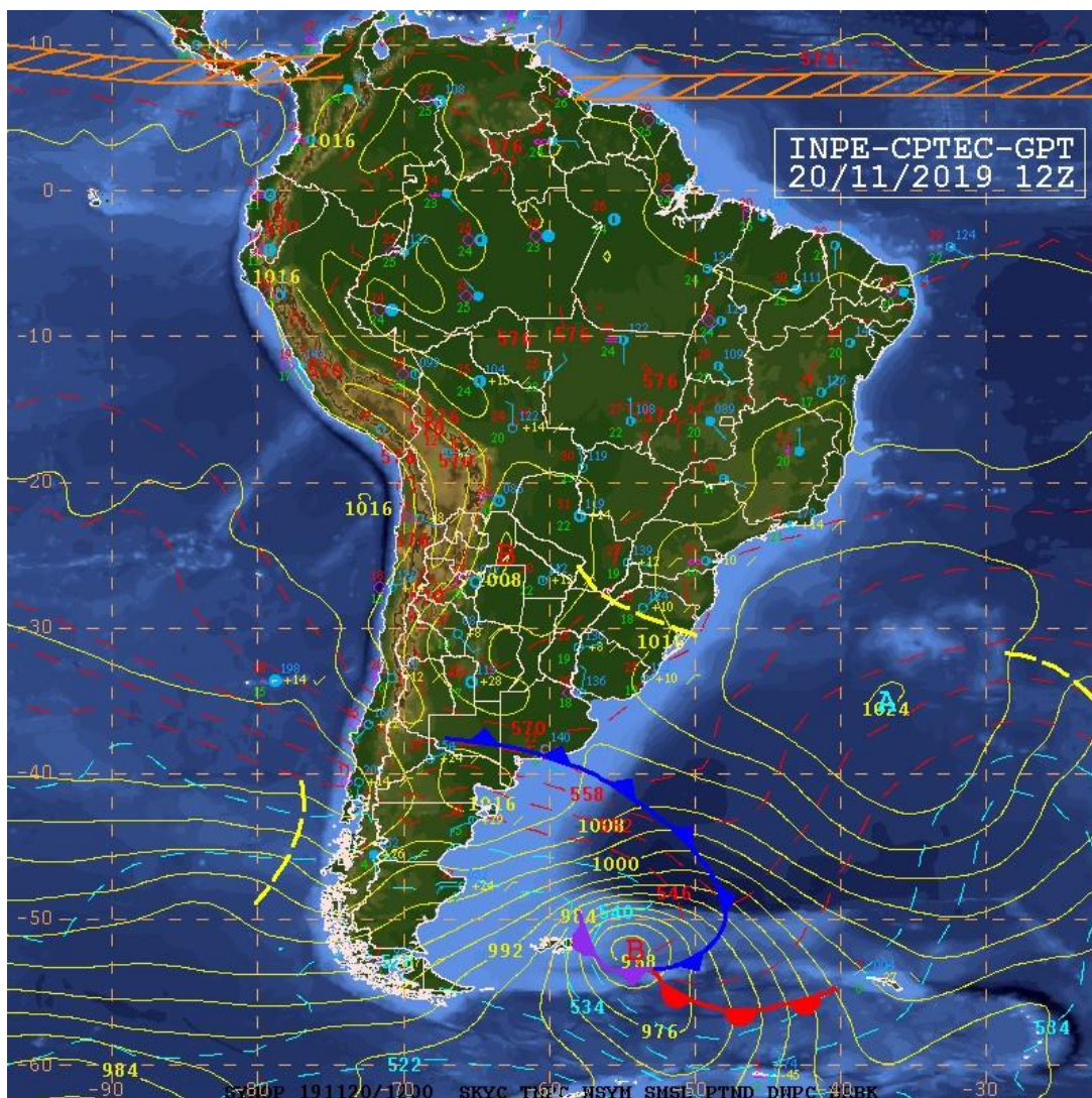
Figura A7 - Carta sinótica da Marinha do Brasil para as 1200Z do dia 20 de novembro de 2019 (09h00 do dia 20 de novembro de 2019, hora local. FONTE:CPTEC).
