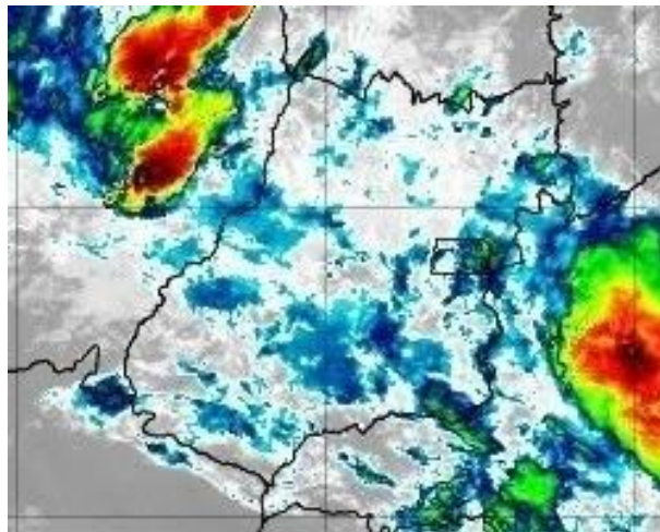
Figura 43 –Imagens realçadas do satélite GOES-16 das 05h00 do dia 20 de novembro de 2019. FONTE: Cptec/INPE.
