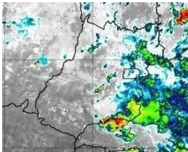
Figura 31 –Imagens realçadas do satélite GOES-16 das 13h00 do dia 18 de novembro de 2019. FONTE: Cptec/INPE.
