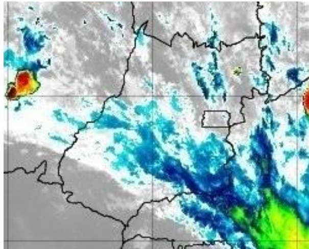
Figura 14 –Imagens realçadas do satélite GOES-16 das 01h00 do dia 16 de novembro de 2019. FONTE: Cptec/INPE.
