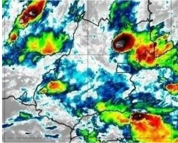
Figura 40 –Imagens realçadas do satélite GOES-16 das 21h00 do dia 19 de novembro de 2019. FONTE: Cptec/INPE.
