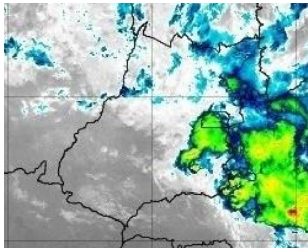
Figura 30 –Imagens realçadas do satélite GOES-16 das 09h00 do dia 18 de novembro de 2019. FONTE: Cptec/INPE.
