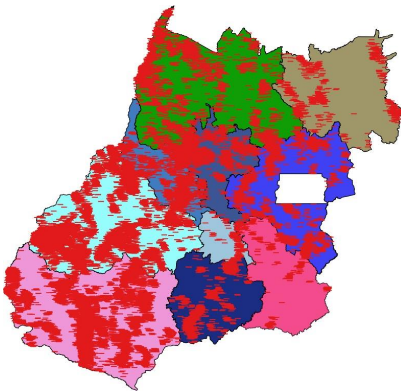
Figura 3 –Descargas atmosféricas nuvem-nuvem (em vermelho) detectadas pelo sistema Earth Networks entre 10h00 do dia 25 e 04h30 do dia 26 de novembro de 2019 sobre a área de concessão da CELG Distribuição.
