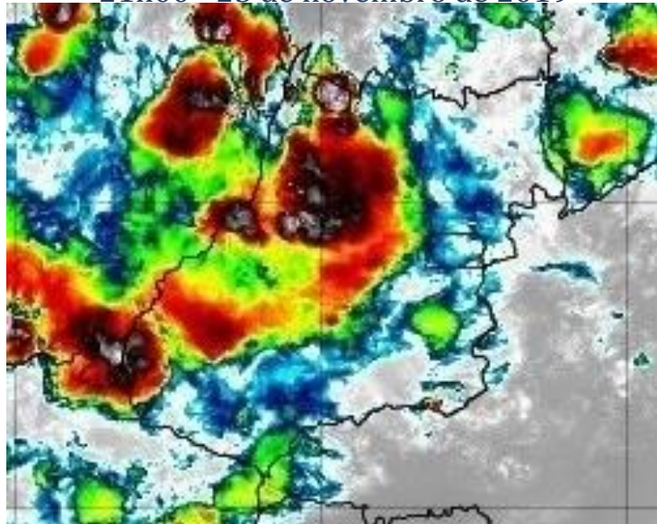
Figura 8 –Imagens realçadas do satélite GOES-16 das 21h00 do dia 25 de novembro de 2019. FONTE: Cptec/INPE.
