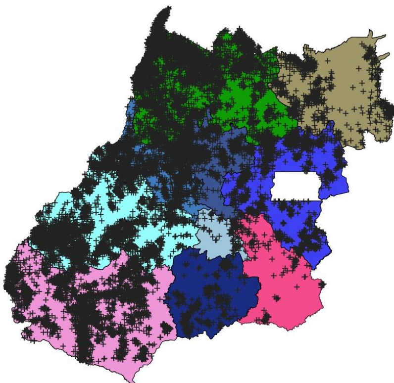
Figura 2 –Descargas atmosféricas nuvem-solo (em preto) detectadas pelo sistema Earth Networks entre 10h00 do dia 25 e 04h30 do dia 26 de novembro de 2019 sobre a área de concessão da CELG Distribuição.
