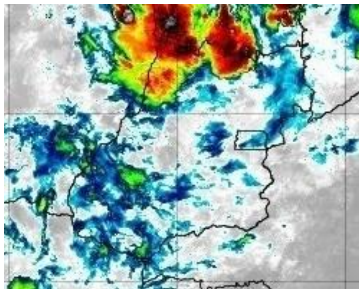
Figura 11 –Imagens realçadas do satélite GOES-16 das 03h00 do dia 26 de novembro de 2019. FONTE: Cptec/INPE.
