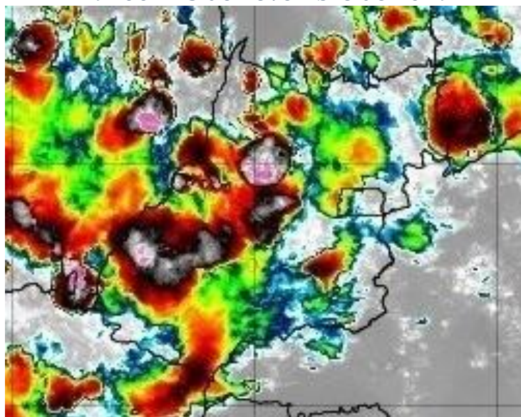
Figura 7 –Imagens realçadas do satélite GOES-16 das 19h00 do dia 25 de novembro de 2019. FONTE: Cptec/INPE.
