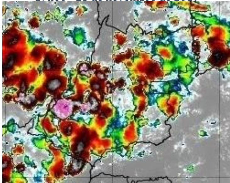
Figura 6 –Imagens realçadas do satélite GOES-16 das 17h00 do dia 25 de novembro de 2019. FONTE: Cptec/INPE.
