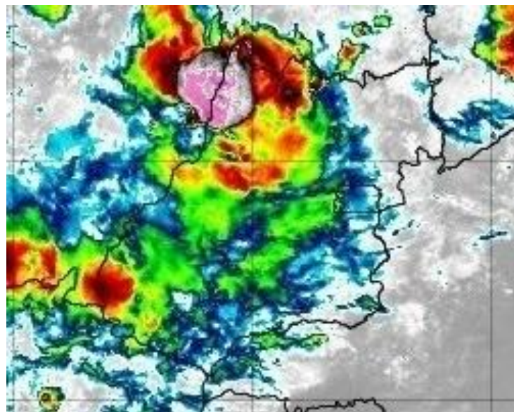
Figura 9 –Imagens realçadas do satélite GOES-16 das 23h00 do dia 25 de novembro de 2019. FONTE: Cptec/INPE.
