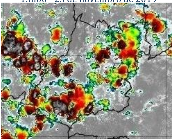
Figura 5 –Imagens realçadas do satélite GOES-16 das 15h00 do dia 25 de novembro de 2019. FONTE: Cptec/INPE.
