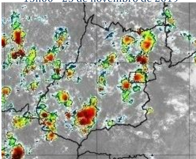
Figura 4 –Imagens realçadas do satélite GOES-16 das 13h00 do dia 25 de novembro de 2019. FONTE: Cptec/INPE.
