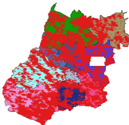
Figura 3 –Descargas atmosféricas nuvem-nuvem (em vermelho) detectadas pelo sistema Earth Networks entre 09h50 do dia 27 de novembro e 03h00 do dia 01 de dezembro de 2019 sobre a área de concessão da CELG Distribuição.
