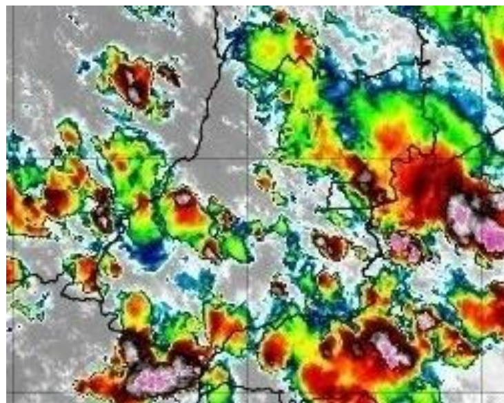
Figura 17 –Imagens realçadas do satélite GOES-16 das 17h00 do dia 29 de novembro de 2019. FONTE: Cptec/INPE.
