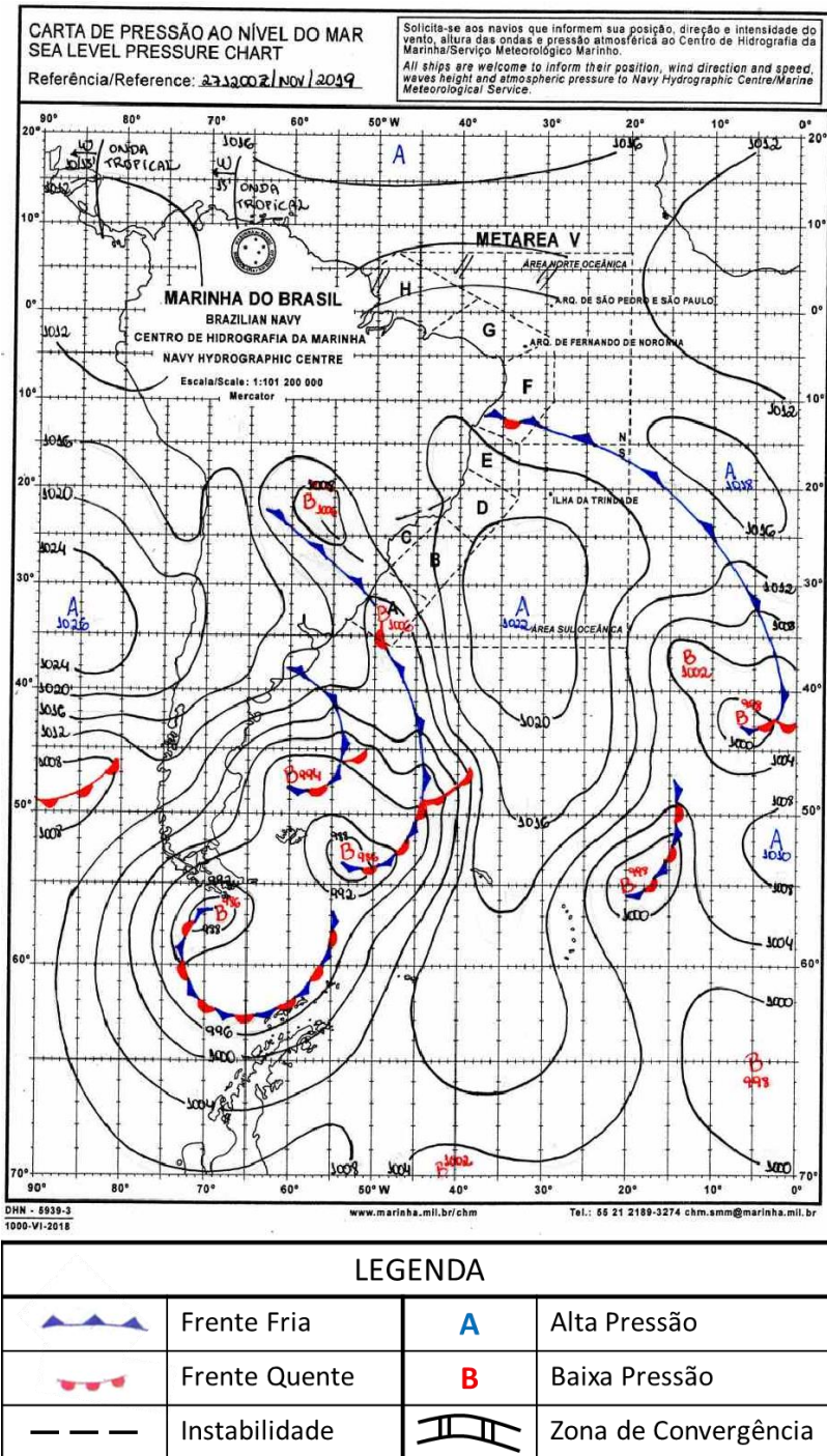
Figura A1 - Carta sinótica para as 1200Z do dia 27 de novembro de 2019 (09h00 do dia 27 de novembro de 2019, hora local. FONTE: Marinha do Brasil).
