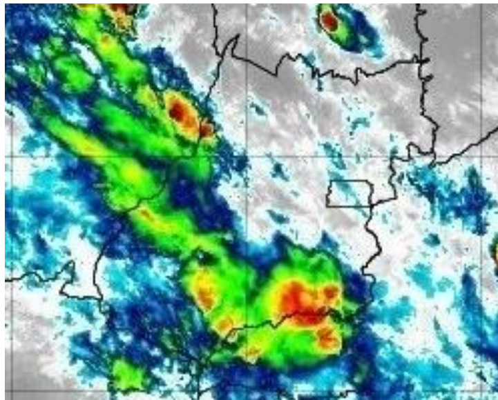
Figura 25 –Imagens realçadas do satélite GOES-16 das 01h00 do dia 01 de dezembro de 2019. FONTE: Cptec/INPE.
