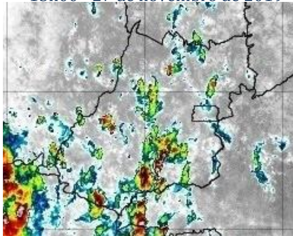
Figura 4 –Imagens realçadas do satélite GOES-16 das 13h00 do dia 27 de novembro de 2019. FONTE: Cptec/INPE.
