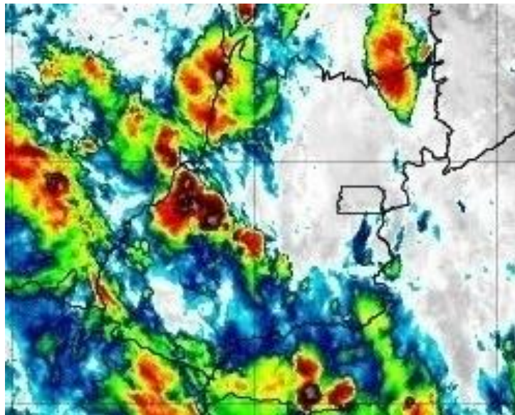
Figura 7 –Imagens realçadas do satélite GOES-16 das 01h00 do dia 28 de novembro de 2019. FONTE: Cptec/INPE.
