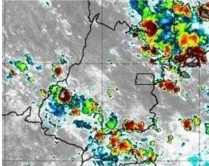
Figura 16 –Imagens realçadas do satélite GOES-16 das 13h00 do dia 29 de novembro de 2019. FONTE: Cptec/INPE.
