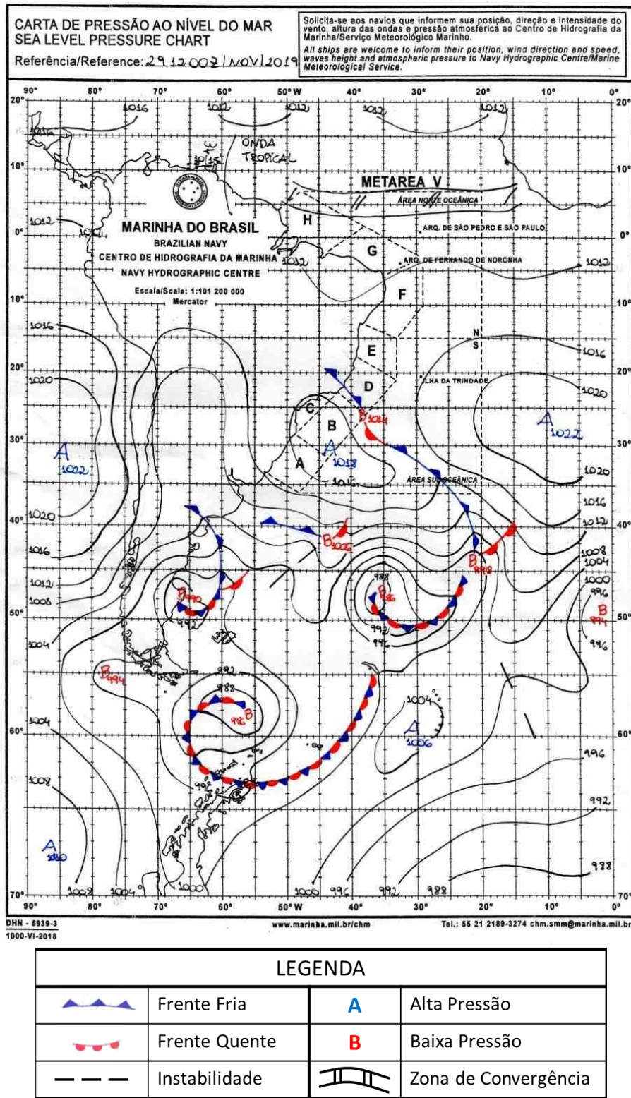
Figura A5 - Carta sinótica para as 1200Z do dia 29 de novembro de 2019 (09h00 do dia 29 de novembro de 2019, hora local. FONTE: Marinha do Brasil).
