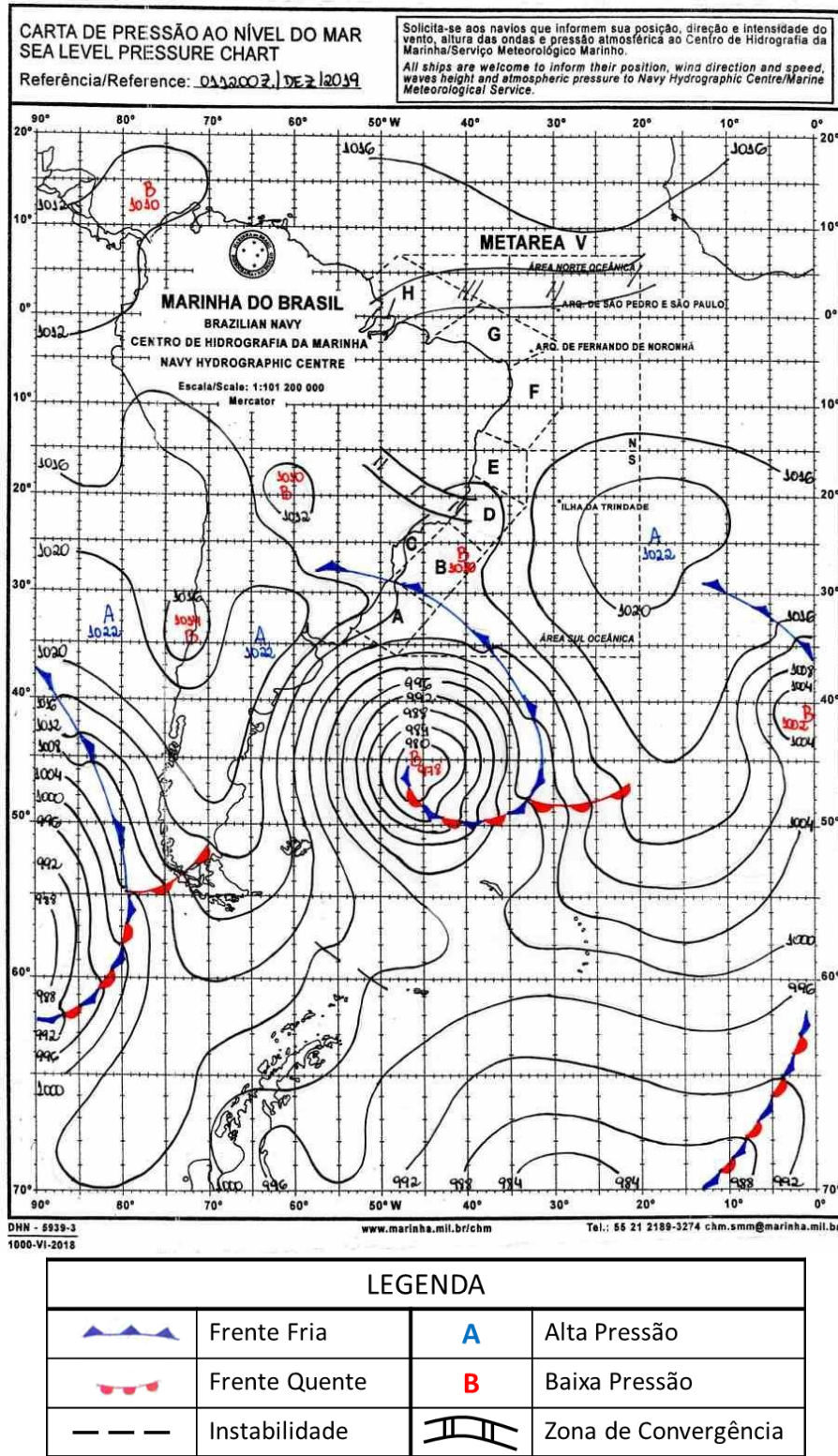
Figura A7 - Carta sinótica para as 1200Z do dia 01 de dezembro de 2019 (09h00 do dia 01 de dezembro de 2019, hora local. FONTE: Marinha do Brasil).
