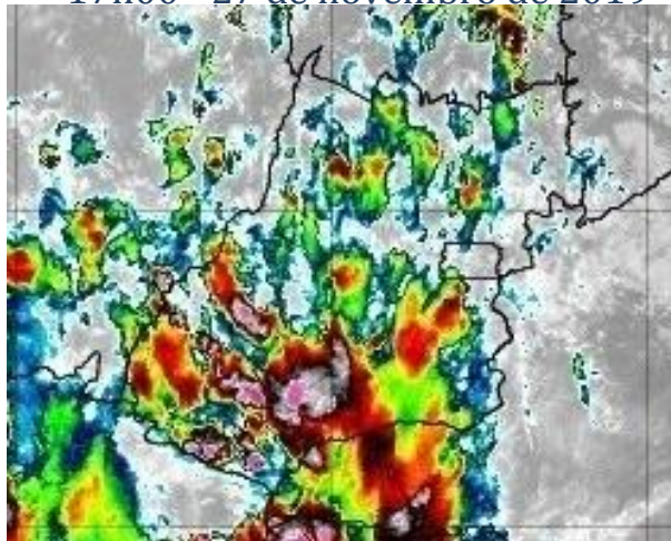
Figura 5 –Imagens realçadas do satélite GOES-16 das 17h00 do dia 27 de novembro de 2019. FONTE: Cptec/INPE.
