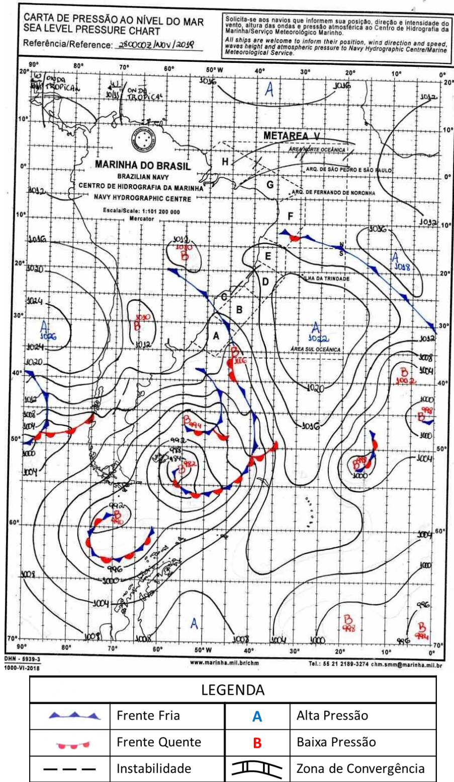
Figura A2 - Carta sinótica da Marinha do Brasil para as 0000Z do dia 28 de novembro de 2019 (21h00 do dia 27 de novembro de 2019, hora local). FONTE: Marinha do Brasil).
