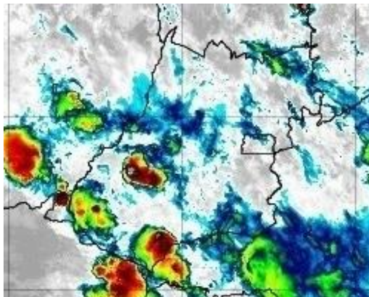
Figura 13 –Imagens realçadas do satélite GOES-16 das 01h00 do dia 29 de novembro de 2019. FONTE: Cptec/INPE.
