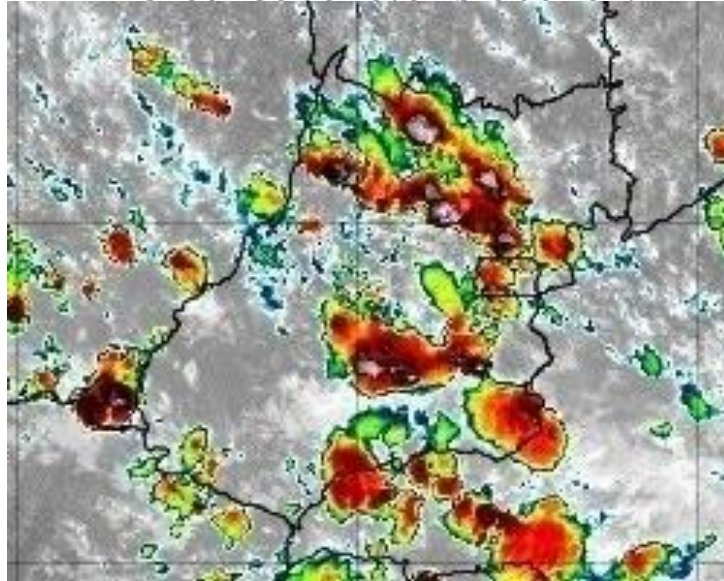
Figura 22 –Imagens realçadas do satélite GOES-16 das 13h00 do dia 30 de novembro de 2019. FONTE: Cptec/INPE.
