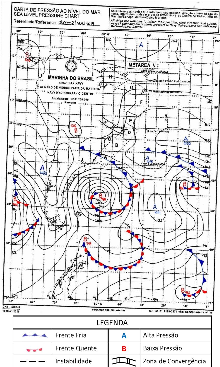
Figura A8 - Carta sinótica da Marinha do Brasil para as 0000Z do dia 01 de dezembro de 2019 (21h00 do dia 30 de novembro de 2019, hora local). FONTE: Marinha do Brasil).
