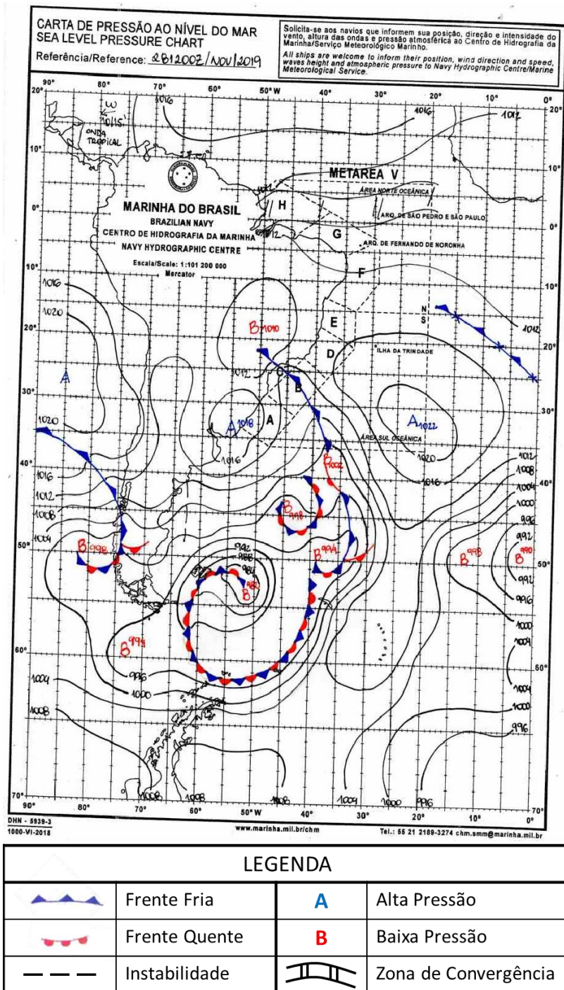
Figura A3 - Carta sinótica para as 1200Z do dia 28 de novembro de 2019 (09h00 do dia 28 de novembro de 2019, hora local. FONTE: Marinha do Brasil).
