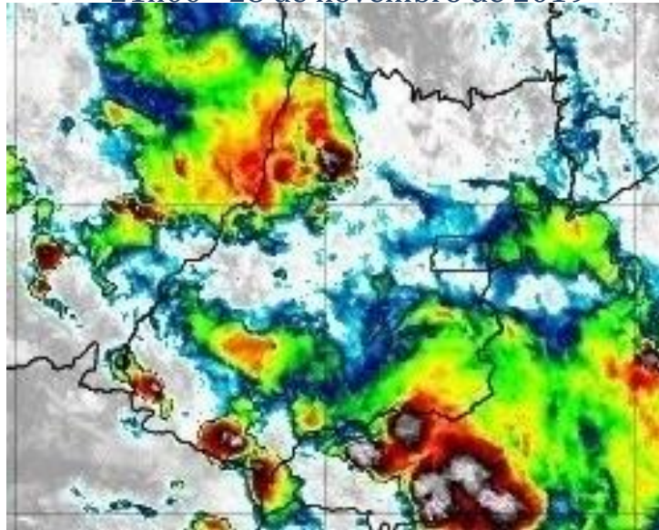
Figura 12 –Imagens realçadas do satélite GOES-16 das 21h00 do dia 28 de novembro de 2019. FONTE: Cptec/INPE.
