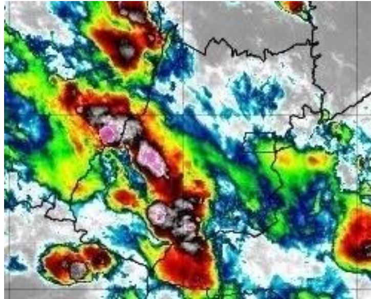
Figura 24 –Imagens realçadas do satélite GOES-16 das 21h00 do dia 30 de novembro de 2019. FONTE: Cptec/INPE.
