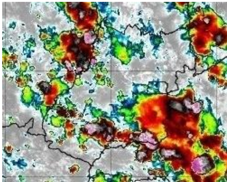
Figura 11 –Imagens realçadas do satélite GOES-16 das 17h00 do dia 28 de novembro de 2019. FONTE: Cptec/INPE.
