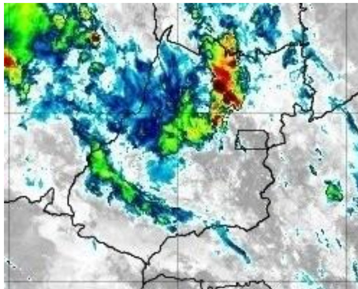
Figura 9 –Imagens realçadas do satélite GOES-16 das 09h00 do dia 28 de novembro de 2019. FONTE: Cptec/INPE.
