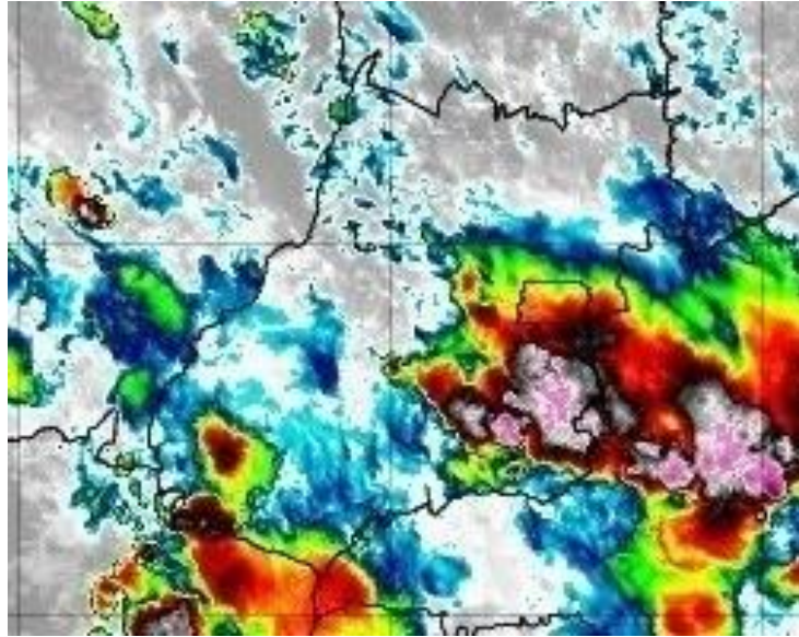
Figura 18 –Imagens realçadas do satélite GOES-16 das 21h00 do dia 29 de novembro de 2019. FONTE: Cptec/INPE.
