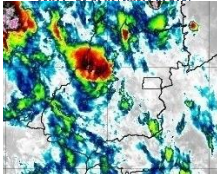
Figura 8 –Imagens realçadas do satélite GOES-16 das 05h00 do dia 28 de novembro de 2019. FONTE: Cptec/INPE.
