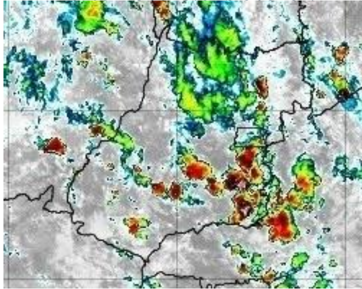
Figura 10 –Imagens realçadas do satélite GOES-16 das 13h00 do dia 28 de novembro de 2019. FONTE: Cptec/INPE.
