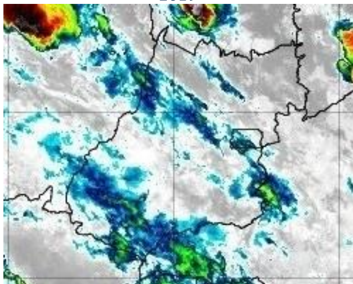
Figura 26 –Imagens realçadas do satélite GOES-16 das 05h00 do dia 01 de dezembro de 2019. FONTE: Cptec/INPE.
