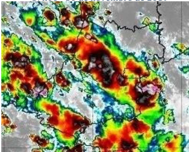
Figura 23 –Imagens realçadas do satélite GOES-16 das 17h00 do dia 30 de novembro de 2019. FONTE: Cptec/INPE.
