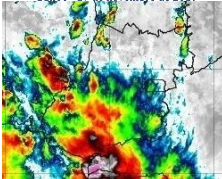
Figura 6 –Imagens realçadas do satélite GOES-16 das 21h00 do dia 27 de novembro de 2019. FONTE: Cptec/INPE.
