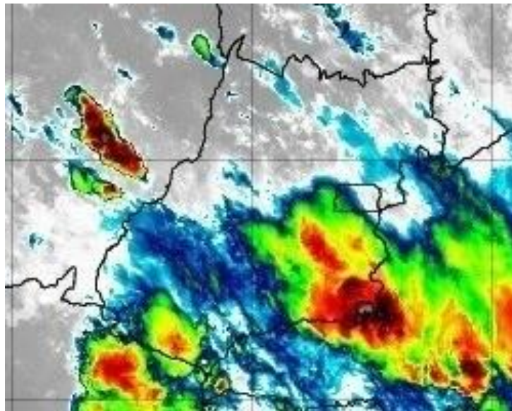
Figura 19 –Imagens realçadas do satélite GOES-16 das 01h00 do dia 30 de novembro de 2019. FONTE: Cptec/INPE.
