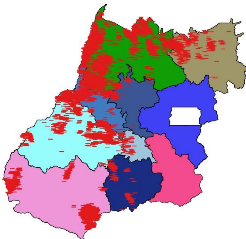
Figura 3 – Descargas atmosféricas nuvem-nuvem (em vermelho) detectadas pelo sistema Earth Networks entre 13h00 do dia 12 e as 02h30 do dia 14 de novembro de 2019 sobre a área de concessão da CELG Distribuição.
