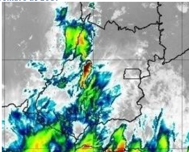
Figura 19 – Imagens realçadas do satélite GOES-16 das 21h00 do dia 13 de novembro de 2019. FONTE: Cptec/INPE.
