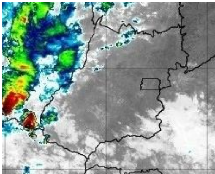
Figura 14 – Imagens realçadas do satélite GOES-16 das 11h00 do dia 13 de novembro de 2019. FONTE: Cptec/INPE.
