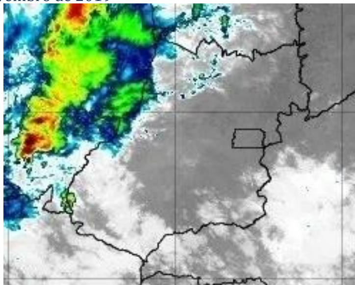
Figura 13 – Imagens realçadas do satélite GOES-16 das 09h00 do dia 13 de novembro de 2019. FONTE: Cptec/INPE.
