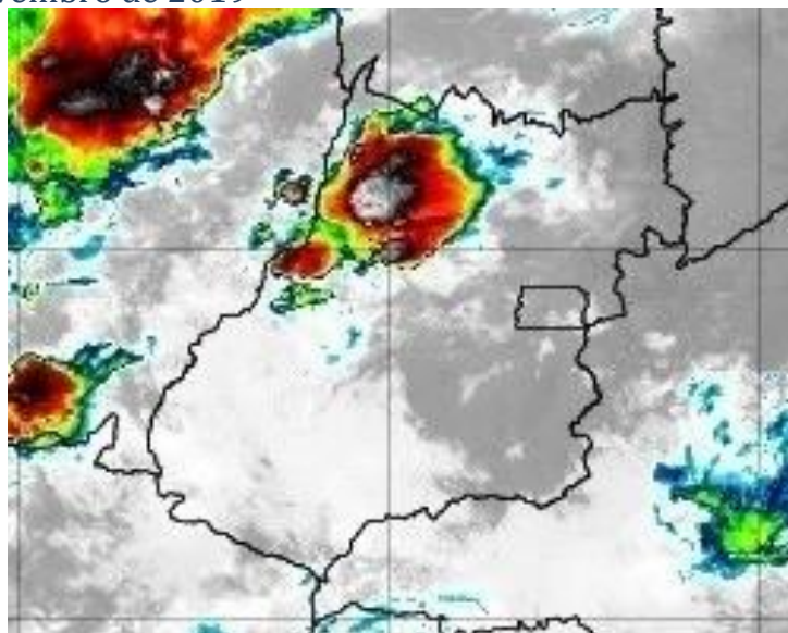
Figura 9 – Imagens realçadas do satélite GOES-16 das 01h00 do dia 13 de novembro de 2019. FONTE: Cptec/INPE.
