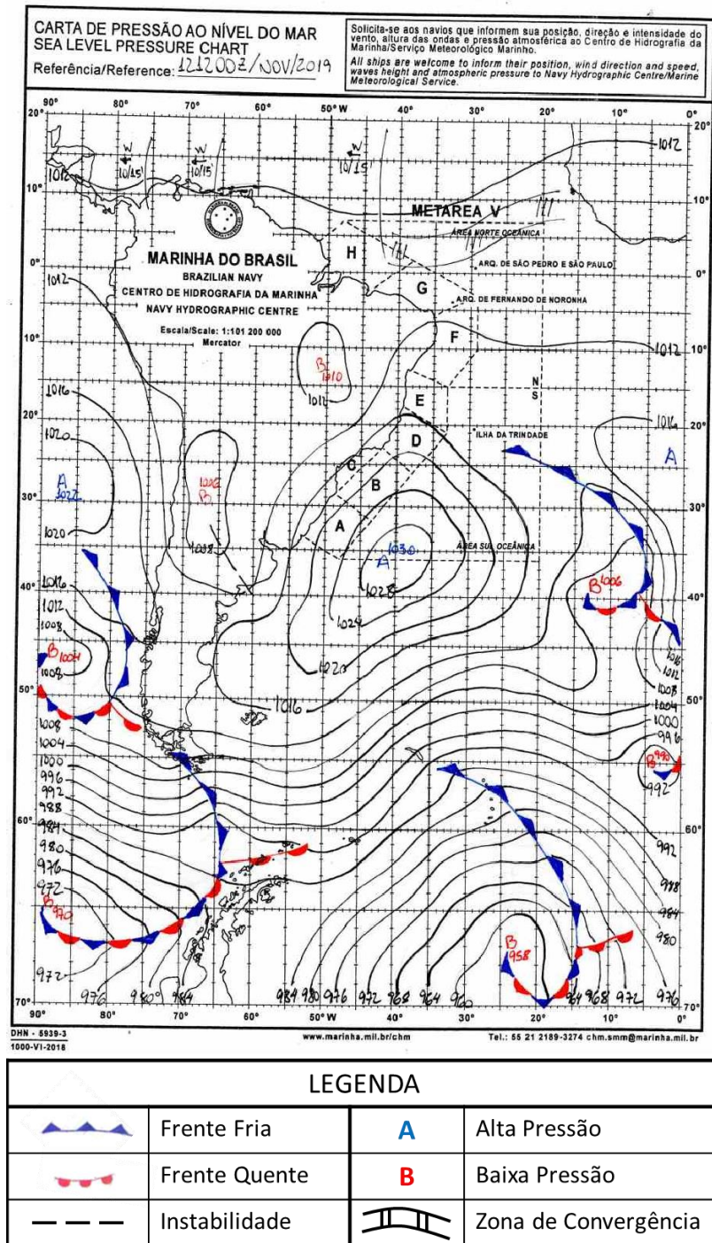
Figura A1 - Carta sinótica da Marinha do Brasil para as 1200Z do dia 12 de novembro de 2019 (09h00 do dia 12 de novembro de 2019, hora local).
