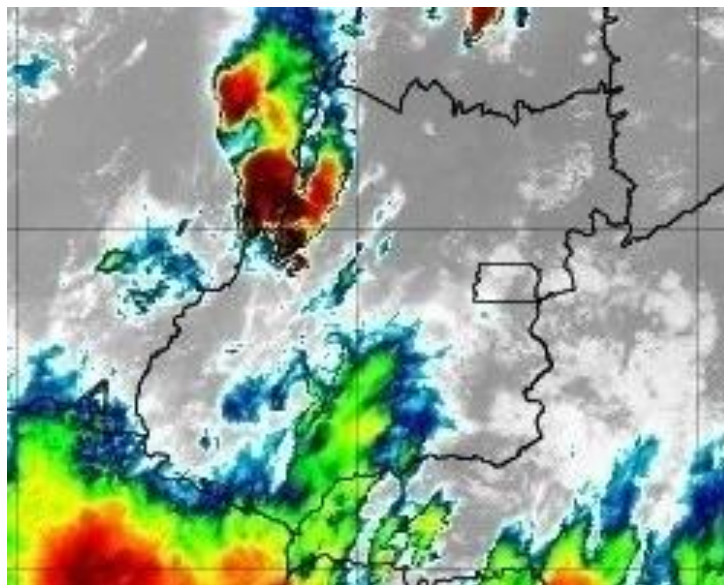
Figura 18 – Imagens realçadas do satélite GOES-16 das 19h00 do dia 13 de novembro de 2019. FONTE: Cptec/INPE.
