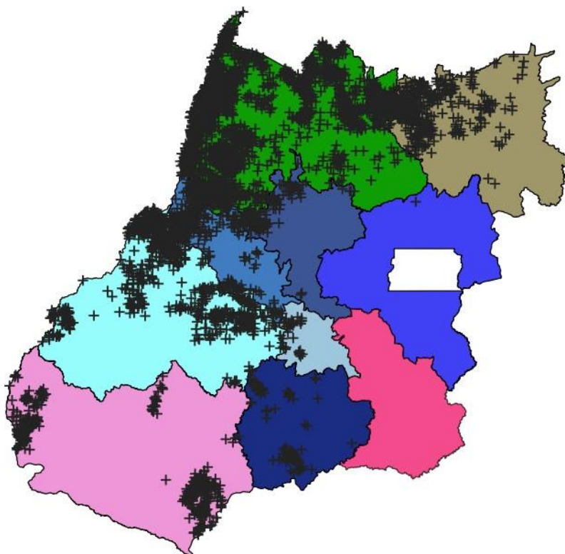
Figura 2 – Descargas atmosféricas nuvem-solo (em preto) detectadas pelo sistema Earth Networks entre 13h00 do dia 12 e as 02h30 do dia 14 de novembro de 2019 sobre a área de concessão da CELG Distribuição.
