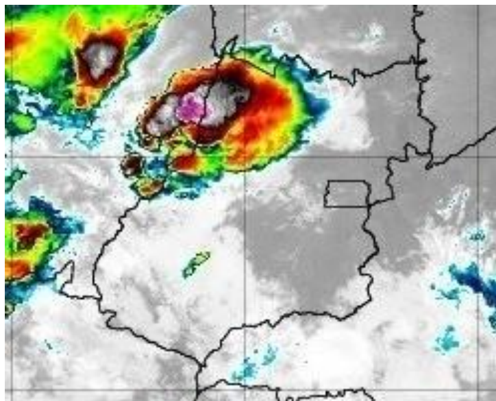
Figura 10 – Imagens realçadas do satélite GOES-16 das 03h00 do dia 13 de novembro de 2019. FONTE: Cptec/INPE.
