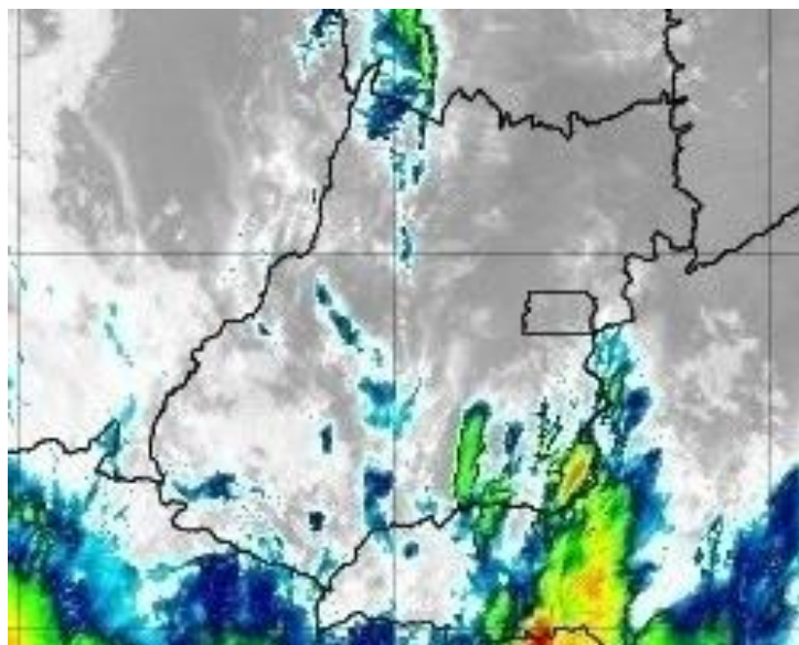
Figura 22 – Imagens realçadas do satélite GOES-16 das 03h00 do dia 14 de novembro de 2019. FONTE: Cptec/INPE.
