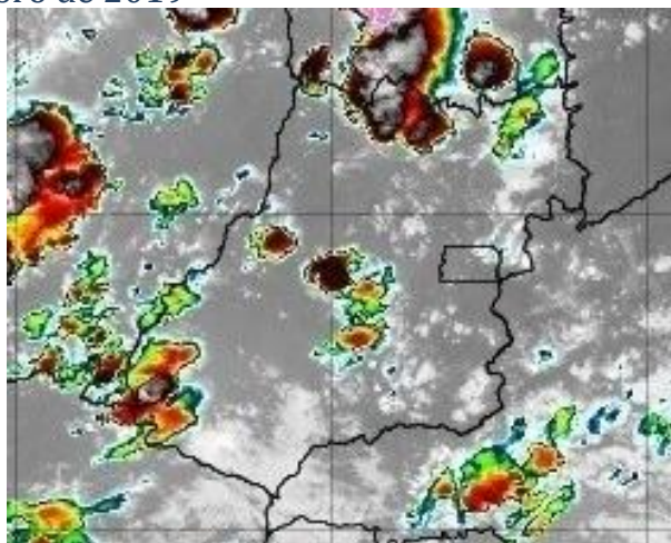
Figura 5 – Imagens realçadas do satélite GOES-16 das 17h00 do dia 12 de novembro de 2019. FONTE: Cptec/INPE.
