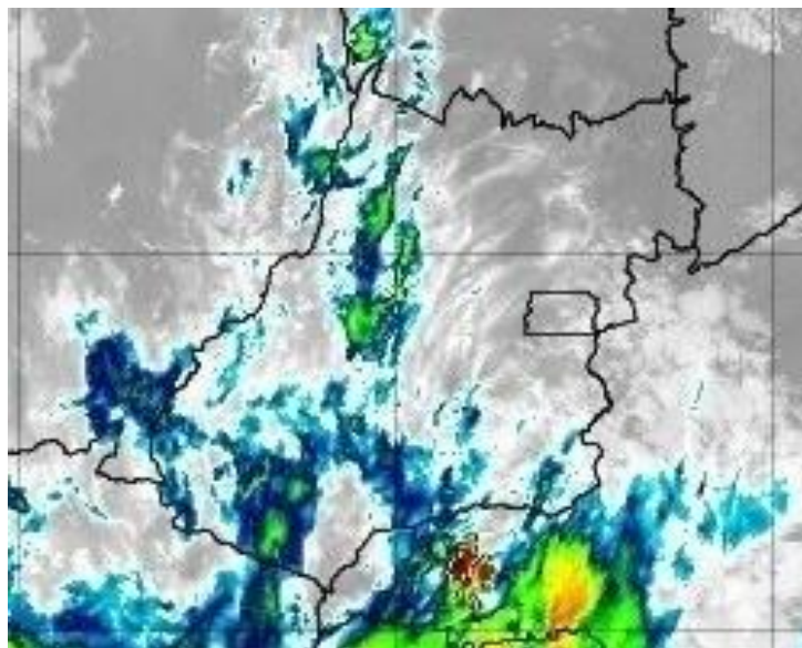
Figura 20 – Imagens realçadas do satélite GOES-16 das 23h00 do dia 13 de novembro de 2019. FONTE: Cptec/INPE.
