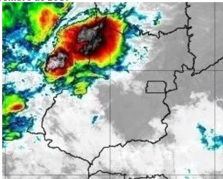
Figura 11 – Imagens realçadas do satélite GOES-16 das 05h00 do dia 13 de novembro de 2019. FONTE: Cptec/INPE.
