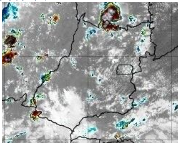
Figura 4 – Imagens realçadas do satélite GOES-16 das 15h00 do dia 12 de novembro de 2019. FONTE: Cptec/INPE.
