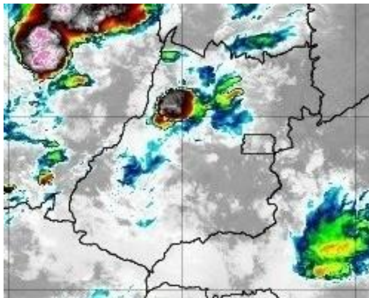
Figura 8 – Imagens realçadas do satélite GOES-16 das 23h00 do dia 12 de novembro de 2019. FONTE: Cptec/INPE.
