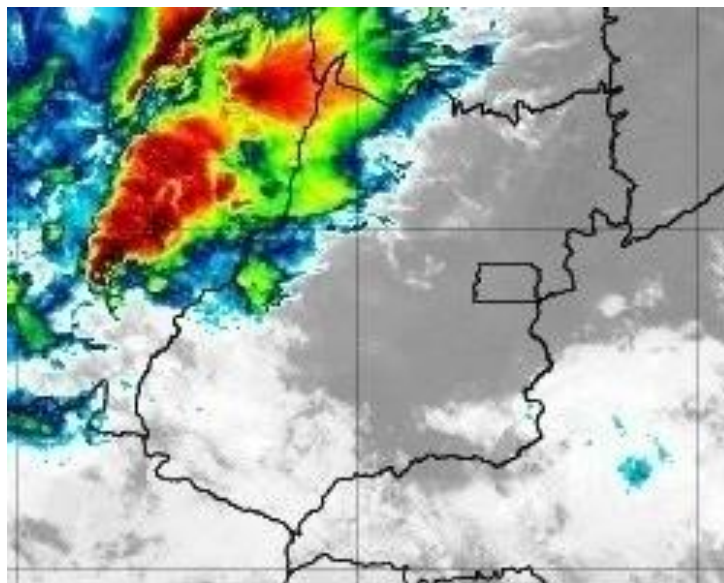
Figura 12 – Imagens realçadas do satélite GOES-16 das 07h00 do dia 13 de novembro de 2019. FONTE: Cptec/INPE.
