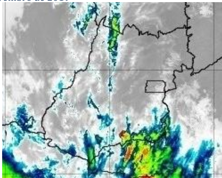
Figura 21 – Imagens realçadas do satélite GOES-16 das 01h00 do dia 14 de novembro de 2019. FONTE: Cptec/INPE.
