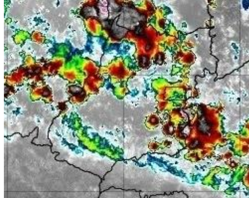
Figura 18 – Imagens realçadas do satélite GOES-16 das 15h00 do dia 07 de dezembro de 2019. FONTE: Cptec/INPE.
