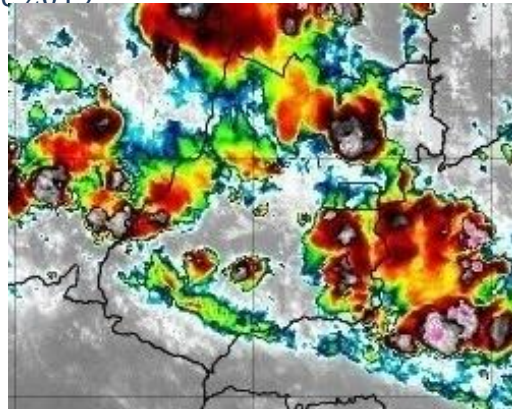
Figura 19 – Imagens realçadas do satélite GOES-16 das 17h00 do dia 07 de dezembro de 2019. FONTE: Cptec/INPE.
