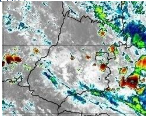
Figura 29 – Imagens realçadas do satélite GOES-16 das 13h00 do dia 08 de dezembro de 2019. FONTE: Cptec/INPE.
