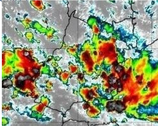
Figura 31 – Imagens realçadas do satélite GOES-16 das 17h00 do dia 08 de dezembro de 2019. FONTE: Cptec/INPE.
