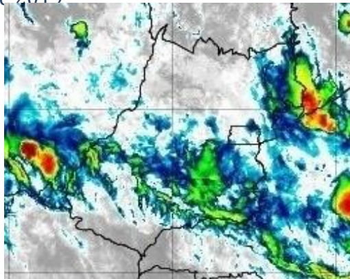
Figura 23 – Imagens realçadas do satélite GOES-16 das 01h00 do dia 08 de dezembro de 2019. FONTE: Cptec/INPE.
