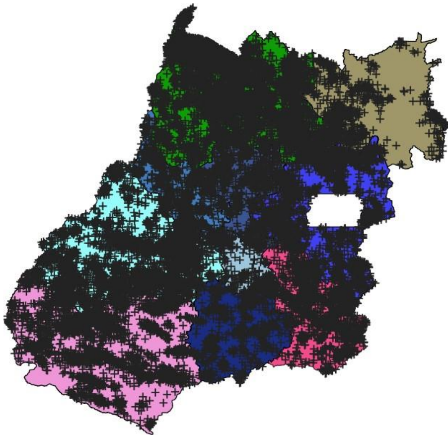
Figura 2 – Descargas atmosféricas nuvem-solo (em preto) detectadas pelo sistema Earth Networks entre 07h30 do dia 06 e 08h30 do dia 09 de dezembro de 2019 sobre a área de concessão da CELG Distribuição.
