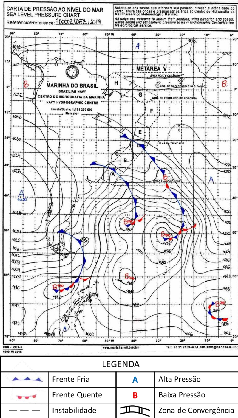
Figura A1 - Carta sinótica da Marinha do Brasil para as 0000Z do dia 07 de dezembro de 2019 (21h00 do dia 06 de dezembro de 2019, hora local. FONTE: Marinha do Brasil).
