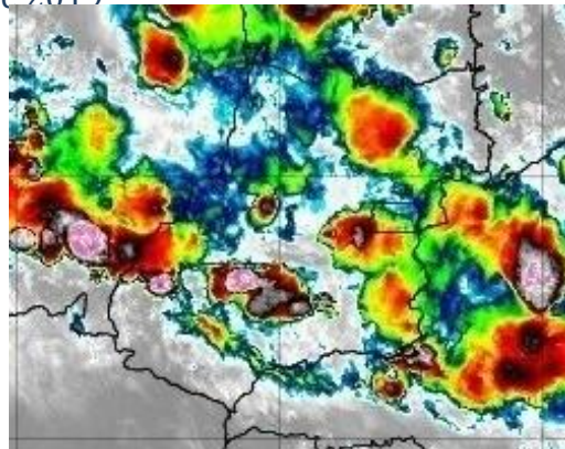
Figura 20 – Imagens realçadas do satélite GOES-16 das 19h00 do dia 07 de dezembro de 2019. FONTE: Cptec/INPE.
