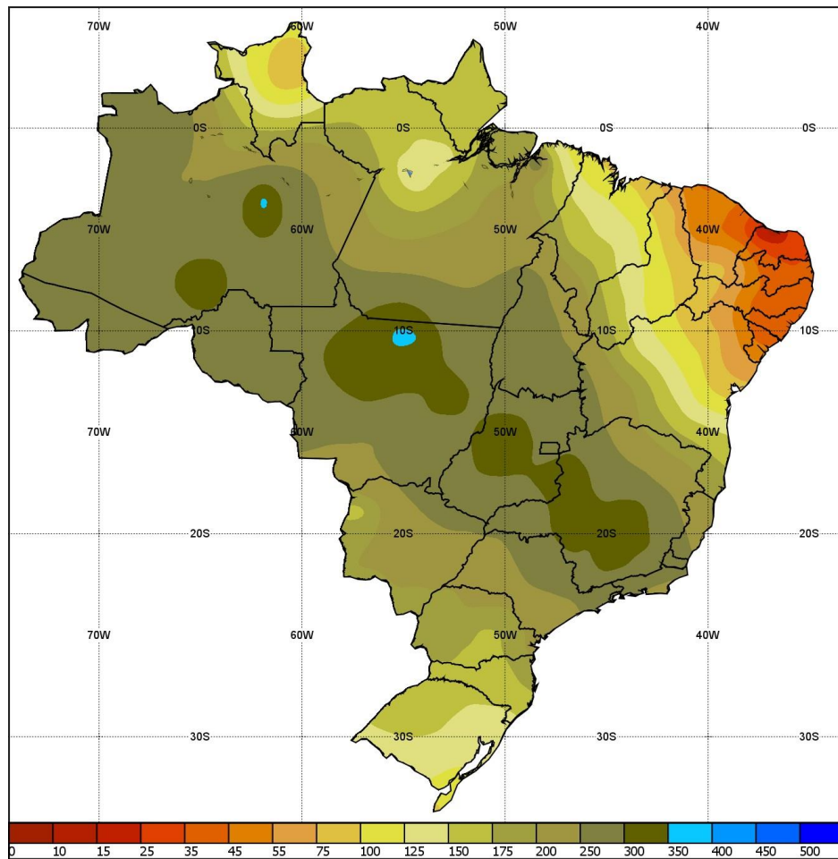
Figura A6 - Média climatológica (1981-2010) de precipitação acumulada para o mês de dezembro. Fonte: INMET).
