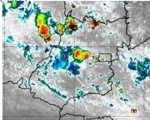
Figura 16 – Imagens realçadas do satélite GOES-16 das 11h00 do dia 07 de dezembro de 2019. FONTE: Cptec/INPE.
