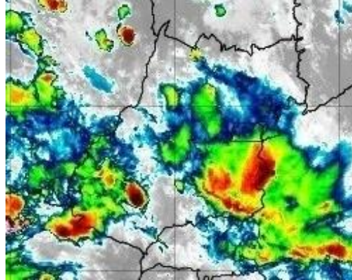
Figura 33 – Imagens realçadas do satélite GOES-16 das 21h00 do dia 08 de dezembro de 2019. FONTE: Cptec/INPE.
