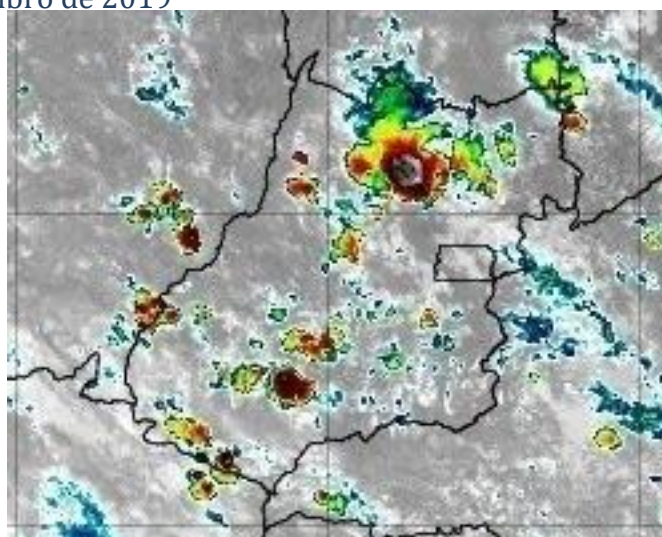
Figura 5 – Imagens realçadas do satélite GOES-16 das 13h00 do dia 06 de dezembro de 2019. FONTE: Cptec/INPE.
