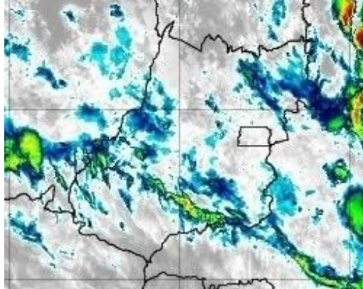
Figura 24 – Imagens realçadas do satélite GOES-16 das 03h00 do dia 08 de dezembro de 2019. FONTE: Cptec/INPE.
