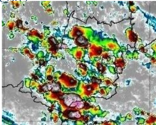
Figura 7 – Imagens realçadas do satélite GOES-16 das 17h00 do dia 06 de dezembro de 2019. FONTE: Cptec/INPE.
