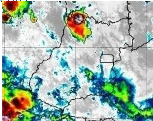
Figura 35 – Imagens realçadas do satélite GOES-16 das 01h00 do dia 09 de dezembro de 2019. FONTE: Cptec/INPE.
