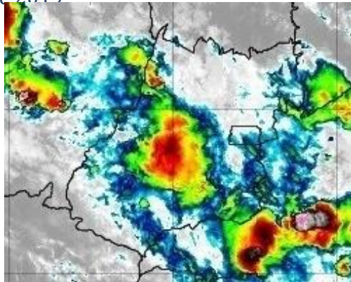
Figura 10 – Imagens realçadas do satélite GOES-16 das 23h00 do dia 06 de dezembro de 2019. FONTE: Cptec/INPE.
