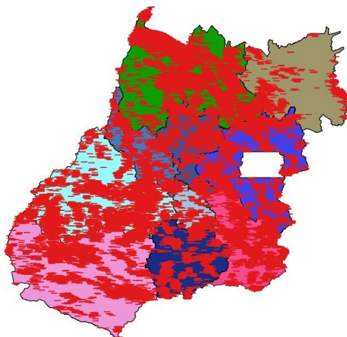
Figura 3 – Descargas atmosféricas nuvem-nuvem (em vermelho) detectadas pelo sistema Earth Networks entre 07h30 do dia 06 e 08h30 do dia 09 de dezembro de 2019 sobre a área de concessão da CELG Distribuição.
