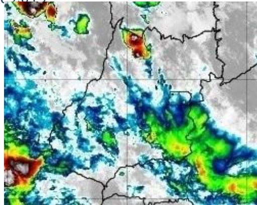
Figura 34 – Imagens realçadas do satélite GOES-16 das 23h00 do dia 08 de dezembro de 2019. FONTE: Cptec/INPE.
