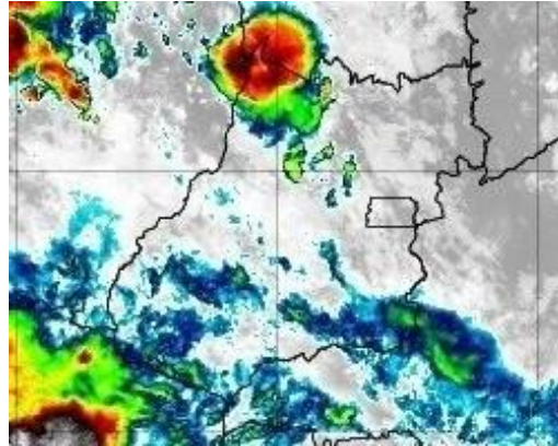
Figura 36 – Imagens realçadas do satélite GOES-16 das 03h00 do dia 09 de dezembro de 2019. FONTE: Cptec/INPE.
