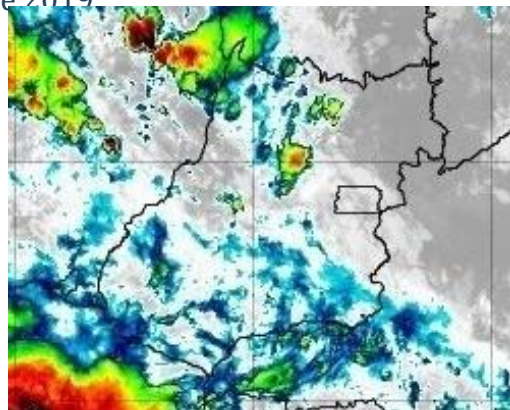
Figura 37 – Imagens realçadas do satélite GOES-16 das 05h00 do dia 09 de dezembro de 2019. FONTE: Cptec/INPE.
