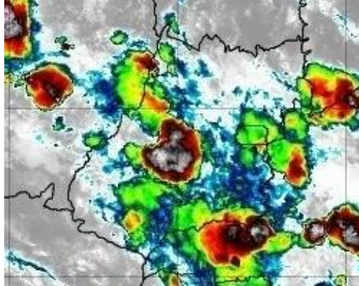
Figura 9 – Imagens realçadas do satélite GOES-16 das 21h00 do dia 06 de dezembro de 2019. FONTE: Cptec/INPE.
