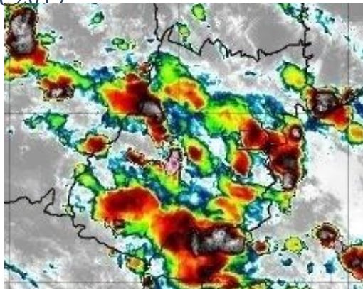
Figura 8 – Imagens realçadas do satélite GOES-16 das 19h00 do dia 06 de dezembro de 2019. FONTE: Cptec/INPE.
