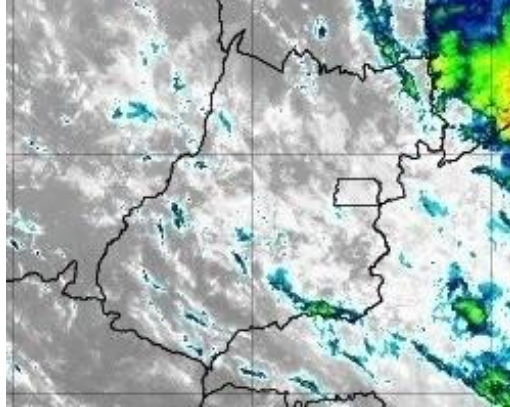
Figura 27 – Imagens realçadas do satélite GOES-16 das 09h00 do dia 08 de dezembro de 2019. FONTE: Cptec/INPE.
