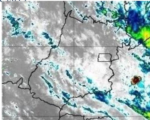
Figura 28 – Imagens realçadas do satélite GOES-16 das 11h00 do dia 08 de dezembro de 2019. FONTE: Cptec/INPE.
