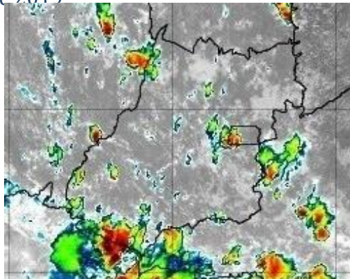
Figura 17 – Imagens realçadas do satélite GOES-16 das 13h00 do dia 11 de dezembro de 2019. FONTE: Cptec/INPE.
