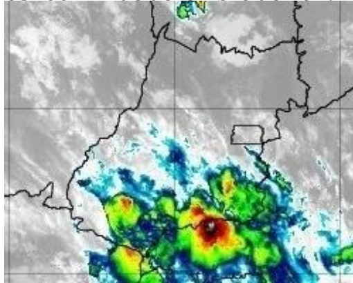
Figura 21 – Imagens realçadas do satélite GOES-16 das 05h00 do dia 12 de dezembro de 2019. FONTE: Cptec/INPE.
