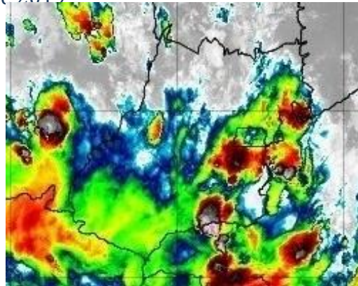
Figura 7 – Imagens realçadas do satélite GOES-16 das 21h00 do dia 09 de dezembro de 2019. FONTE: Cptec/INPE.
