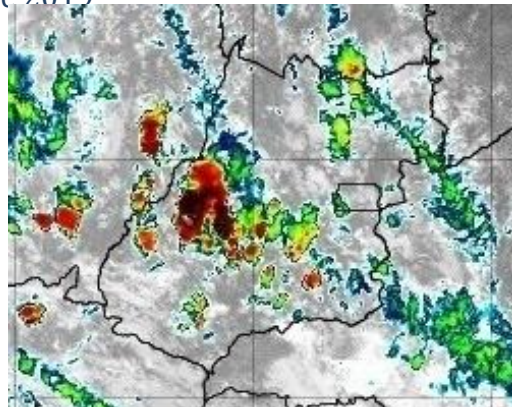
Figura 11 – Imagens realçadas do satélite GOES-16 das 13h00 do dia 10 de dezembro de 2019. FONTE: Cptec/INPE.
