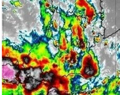
Figura 6 – Imagens realçadas do satélite GOES-16 das 17h00 do dia 09 de dezembro de 2019. FONTE: Cptec/INPE.
