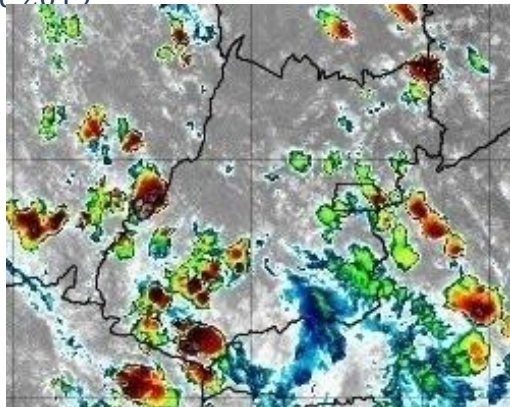
Figura 23 – Imagens realçadas do satélite GOES-16 das 13h00 do dia 12 de dezembro de 2019. FONTE: Cptec/INPE.
