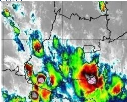
Figura 19 – Imagens realçadas do satélite GOES-16 das 21h00 do dia 11 de dezembro de 2019. FONTE: Cptec/INPE.
