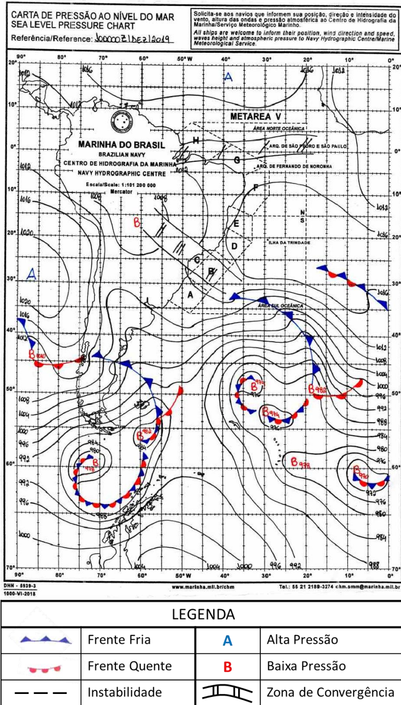
Figura A1 - Carta sinótica da Marinha do Brasil para as 0000Z do dia 10 de dezembro de 2019 (21h00 do dia 09 de dezembro de 2019, hora local. FONTE: Marinha do Brasil).
