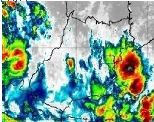
Figura 8 – Imagens realçadas do satélite GOES-16 das 01h00 do dia 10 de dezembro de 2019. FONTE: Cptec/INPE.
