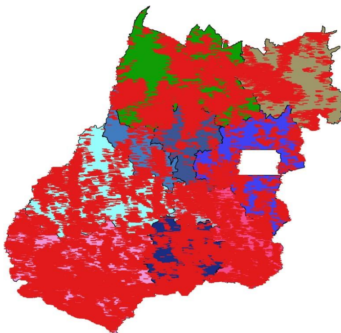
Figura 3 – Descargas atmosféricas nuvem-nuvem (em vermelho) detectadas pelo sistema Earth Networks entre 09h00 do dia 09 e 08h00 do dia 13 de dezembro de 2019 sobre a área de concessão da CELG Distribuição.
