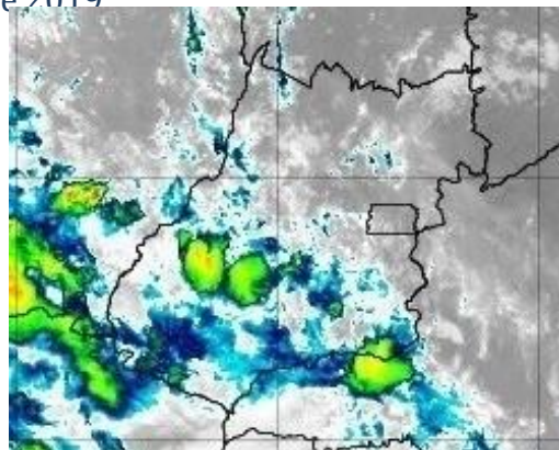
Figura 28 – Imagens realçadas do satélite GOES-16 das 09h00 do dia 13 de dezembro de 2019. FONTE: Cptec/INPE.
