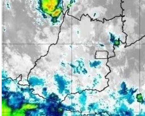
Figura 15 – Imagens realçadas do satélite GOES-16 das 05h00 do dia 11 de dezembro de 2019. FONTE: Cptec/INPE.
