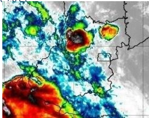
Figura 26 – Imagens realçadas do satélite GOES-16 das 01h00 do dia 13 de dezembro de 2019. FONTE: Cptec/INPE.
