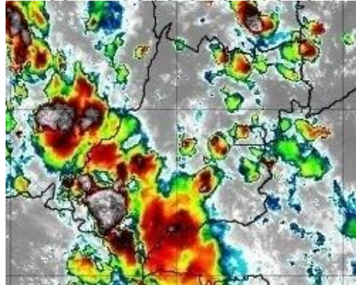
Figura 24 – Imagens realçadas do satélite GOES-16 das 17h00 do dia 12 de dezembro de 2019. FONTE: Cptec/INPE.
