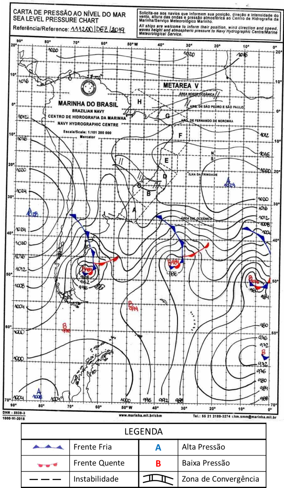
Figura A4 - Carta sinótica da Marinha do Brasil para as 1200Z do dia 11 de dezembro de 2019 (0900 do dia 11 de dezembro de 2019, hora local). FONTE: Marinha do Brasil).
