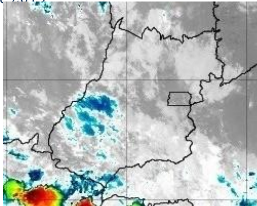
Figura 16 – Imagens realçadas do satélite GOES-16 das 09h00 do dia 11 de dezembro de 2019. FONTE: Cptec/INPE.
