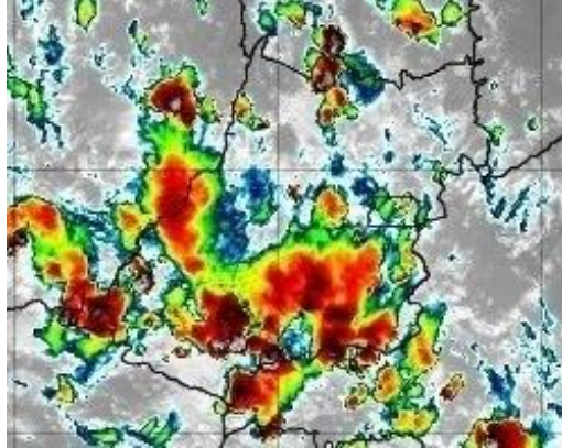
Figura 12 – Imagens realçadas do satélite GOES-16 das 17h00 do dia 10 de dezembro de 2019. FONTE: Cptec/INPE.
