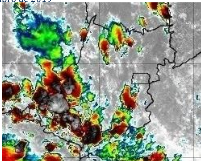
Figura 5 – Imagens realçadas do satélite GOES-16 das 13h00 do dia 09 de dezembro de 2019. FONTE: Cptec/INPE.
