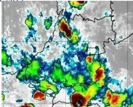
Figura 13 – Imagens realçadas do satélite GOES-16 das 21h00 do dia 10 de dezembro de 2019. FONTE: Cptec/INPE.
