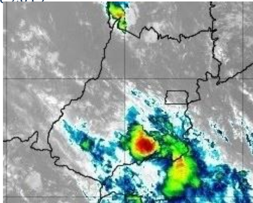
Figura 22 – Imagens realçadas do satélite GOES-16 das 09h00 do dia 12 de dezembro de 2019. FONTE: Cptec/INPE.
