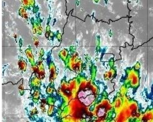
Figura 18 – Imagens realçadas do satélite GOES-16 das 17h00 do dia 11 de dezembro de 2019. FONTE: Cptec/INPE.
