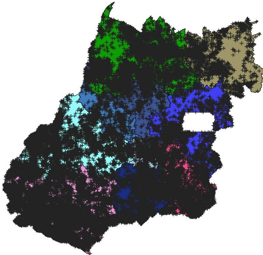
Figura 2 – Descargas atmosféricas nuvem-solo (em preto) detectadas pelo sistema Earth Networks entre 09h00 do dia 09 e 08h00 do dia 13 de dezembro de 2019 sobre a área de concessão da CELG Distribuição.
