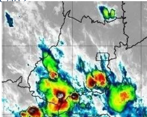
Figura 20 – Imagens realçadas do satélite GOES-16 das 01h00 do dia 12 de dezembro de 2019. FONTE: Cptec/INPE.
