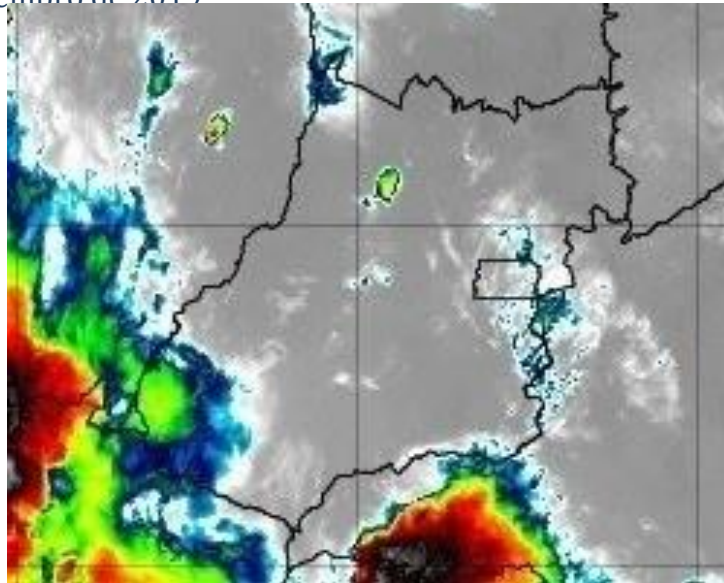
Figura 21 – Imagens realçadas do satélite GOES-16 das 21h00 do dia 14 de dezembro de 2019. FONTE: Cptec/INPE.
