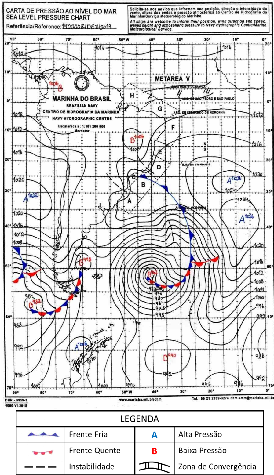
Figura A2 - Carta sinótica da Marinha do Brasil para as 0000Z do dia 14 de dezembro de 2019 (21h00 do dia 13 de dezembro de 2019, hora local). FONTE: Marinha do Brasil).
