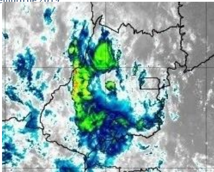
Figura 15 – Imagens realçadas do satélite GOES-16 das 09h00 do dia 14 de dezembro de 2019. FONTE: Cptec/INPE.
