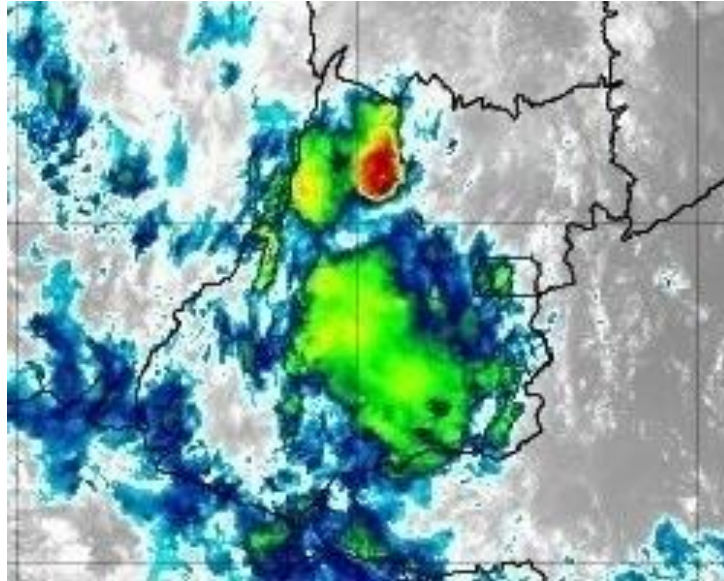
Figura 14 – Imagens realçadas do satélite GOES-16 das 07h00 do dia 14 de dezembro de 2019. FONTE: Cptec/INPE.
