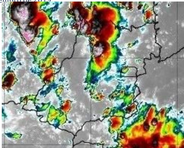
Figura 7 – Imagens realçadas do satélite GOES-16 das 17h00 do dia 13 de dezembro de 2019. FONTE: Cptec/INPE.
