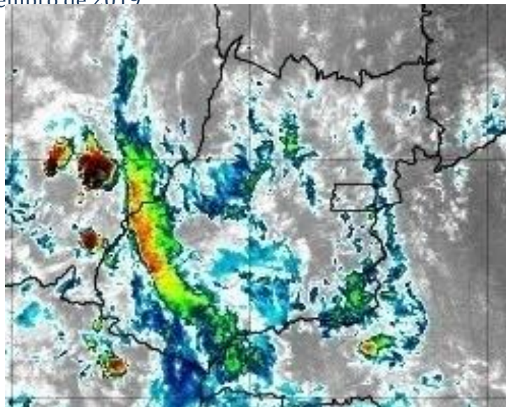
Figura 17 – Imagens realçadas do satélite GOES-16 das 13h00 do dia 14 de dezembro de 2019. FONTE: Cptec/INPE.
