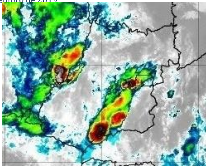
Figura 11 – Imagens realçadas do satélite GOES-16 das 01h00 do dia 14 de dezembro de 2019. FONTE: Cptec/INPE.
