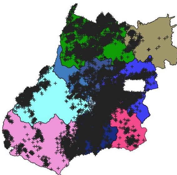
Figura 2 – Descargas atmosféricas nuvem-solo (em preto) detectadas pelo sistema Earth Networks entre 09h00 do dia 13 e 16h40 do dia 14 de dezembro de 2019 sobre a área de concessão da CELG Distribuição.
