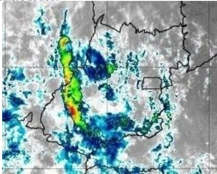
Figura 16 – Imagens realçadas do satélite GOES-16 das 11h00 do dia 14 de dezembro de 2019. FONTE: Cptec/INPE.
