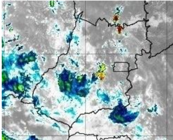
Figura 4 – Imagens realçadas do satélite GOES-16 das 13h00 do dia 13 de dezembro de 2019. FONTE: Cptec/INPE.
