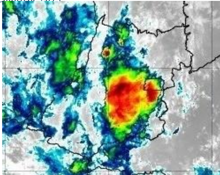
Figura 13 – Imagens realçadas do satélite GOES-16 das 05h00 do dia 14 de dezembro de 2019. FONTE: Cptec/INPE.
