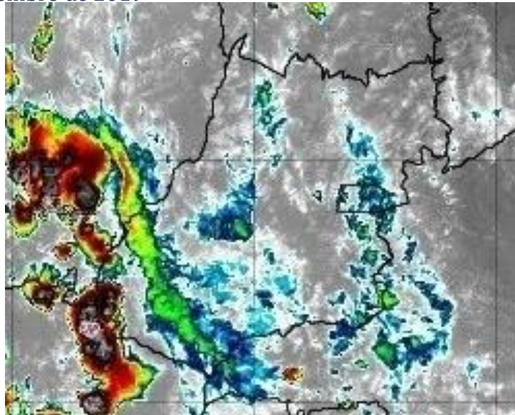
Figura 18 – Imagens realçadas do satélite GOES-16 das 15h00 do dia 14 de dezembro de 2019. FONTE: Cptec/INPE.
