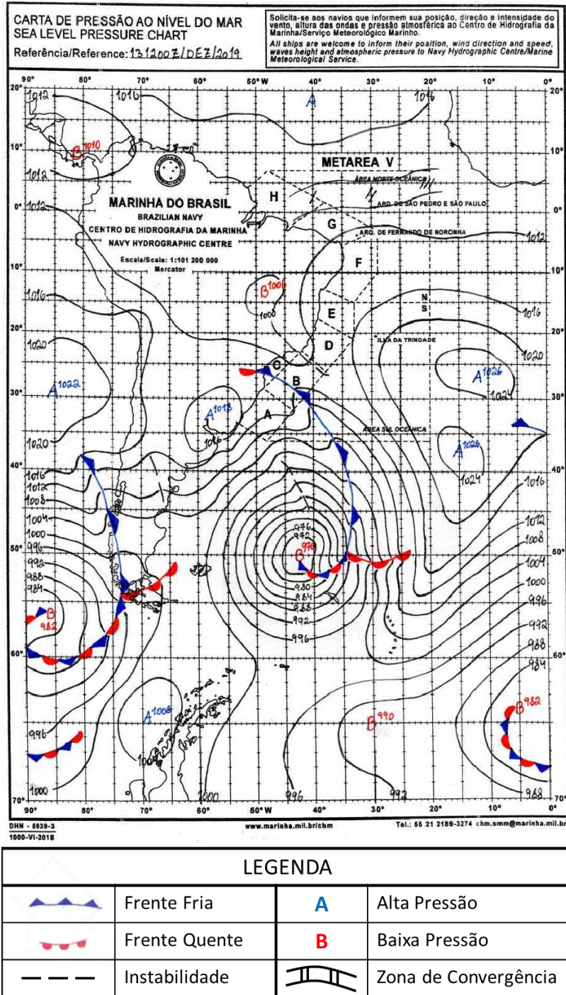
Figura A1 - Carta sinótica para as 1200Z do dia 13 de dezembro de 2019 (09h00 do dia 13 de dezembro de 2019, hora local. FONTE: Marinha do Brasil).
