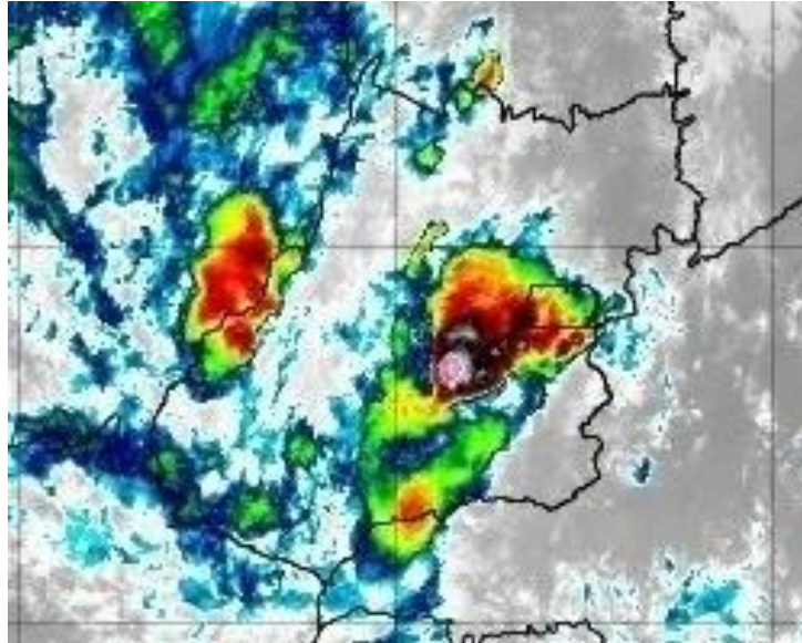
Figura 12 – Imagens realçadas do satélite GOES-16 das 03h00 do dia 14 de dezembro de 2019. FONTE: Cptec/INPE.
