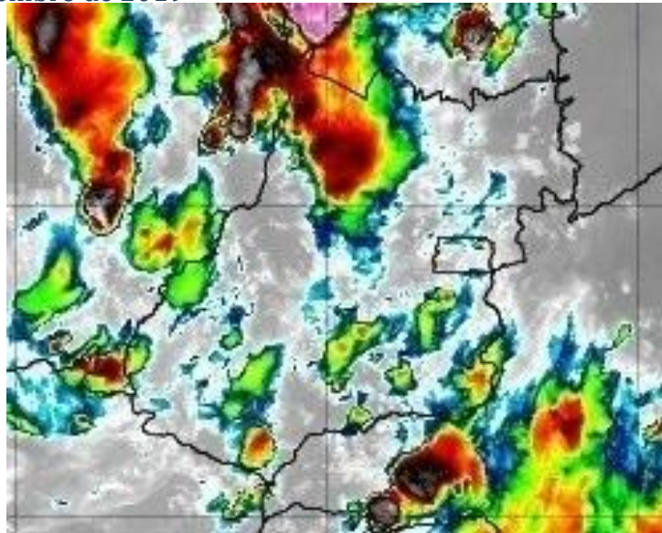
Figura 8 – Imagens realçadas do satélite GOES-16 das 19h00 do dia 13 de dezembro de 2019. FONTE: Cptec/INPE.
