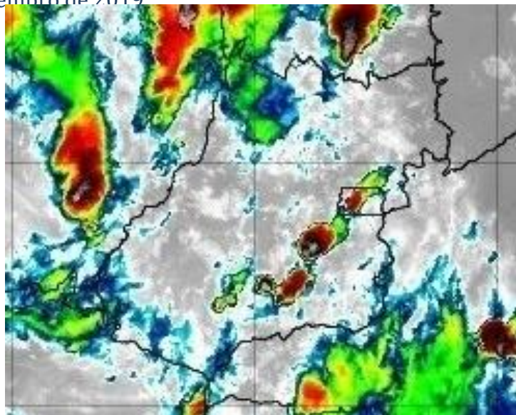
Figura 9 – Imagens realçadas do satélite GOES-16 das 21h00 do dia 13 de dezembro de 2019. FONTE: Cptec/INPE.
