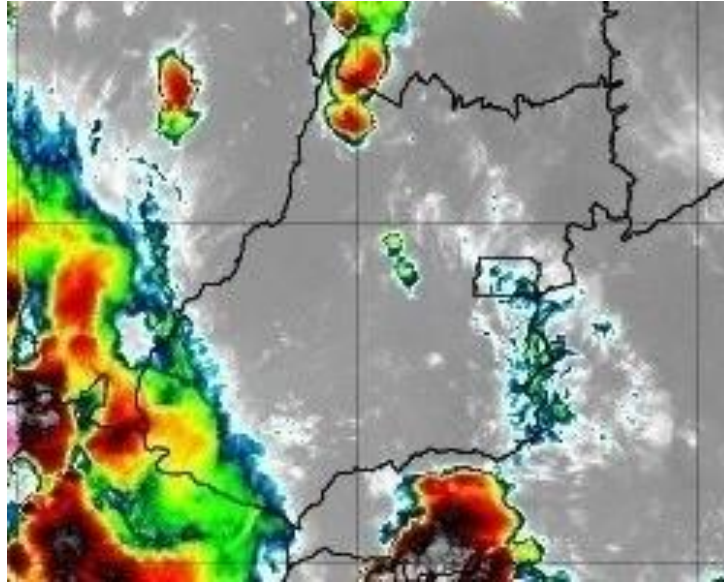
Figura 20 – Imagens realçadas do satélite GOES-16 das 19h00 do dia 14 de dezembro de 2019. FONTE: Cptec/INPE.
