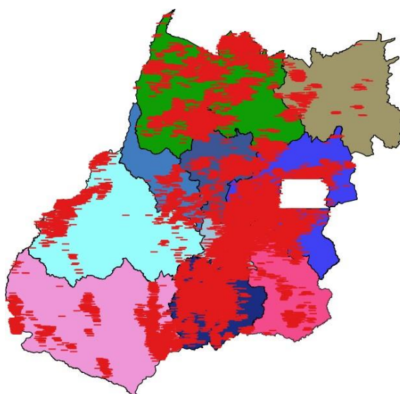
Figura 3 – Descargas atmosféricas nuvem-nuvem (em vermelho) detectadas pelo sistema Earth Networks entre 09h00 do dia 13 e 16h40 do dia 14 de dezembro de 2019 sobre a área de concessão da CELG Distribuição.
