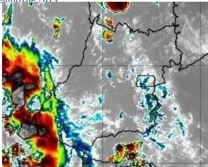
Figura 19 – Imagens realçadas do satélite GOES-16 das 17h00 do dia 14 de dezembro de 2019. FONTE: Cptec/INPE.
