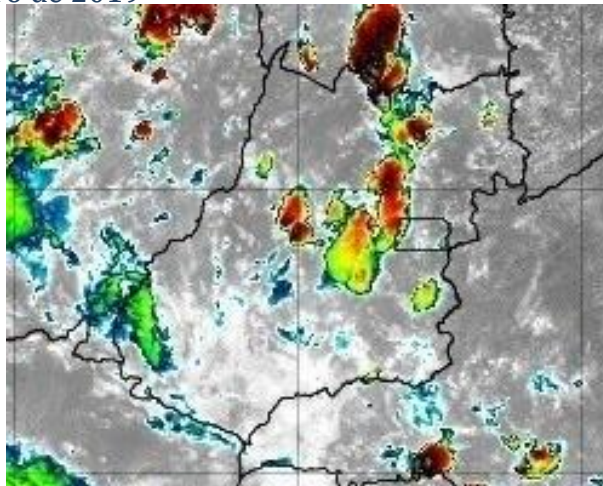
Figura 5 – Imagens realçadas do satélite GOES-16 das 13h00 do dia 13 de dezembro de 2019. FONTE: Cptec/INPE.
