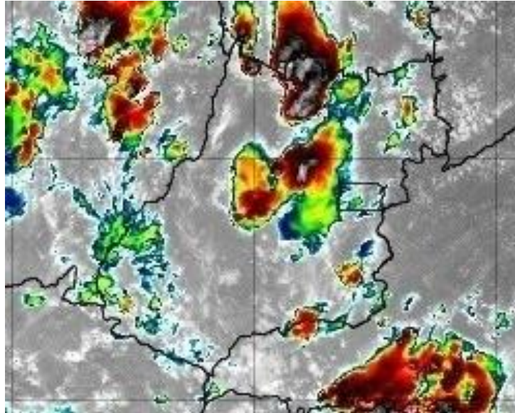
Figura 6 – Imagens realçadas do satélite GOES-16 das 15h00 do dia 13 de dezembro de 2019. FONTE: Cptec/INPE.
