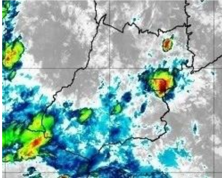
Figura 10 – Imagens realçadas do satélite GOES-16 das 01h00 do dia 19 de dezembro de 2019. FONTE: Cptec/INPE.
