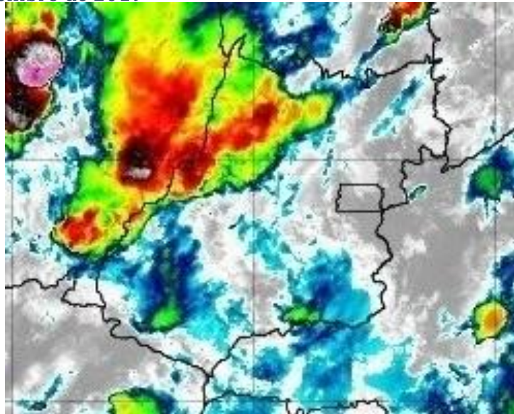
Figura 20 – Imagens realçadas do satélite GOES-16 das 21h00 do dia 19 de dezembro de 2019. FONTE: Cptec/INPE.
