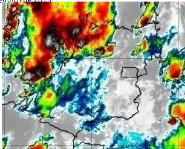
Figura 19 – Imagens realçadas do satélite GOES-16 das 19h00 do dia 19 de dezembro de 2019. FONTE: Cptec/INPE.
