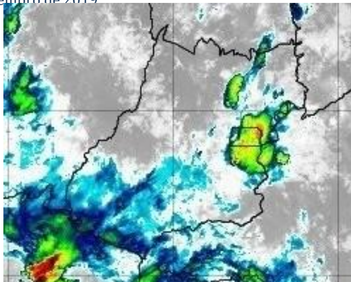
Figura 11 – Imagens realçadas do satélite GOES-16 das 03h00 do dia 19 de dezembro de 2019. FONTE: Cptec/INPE.
