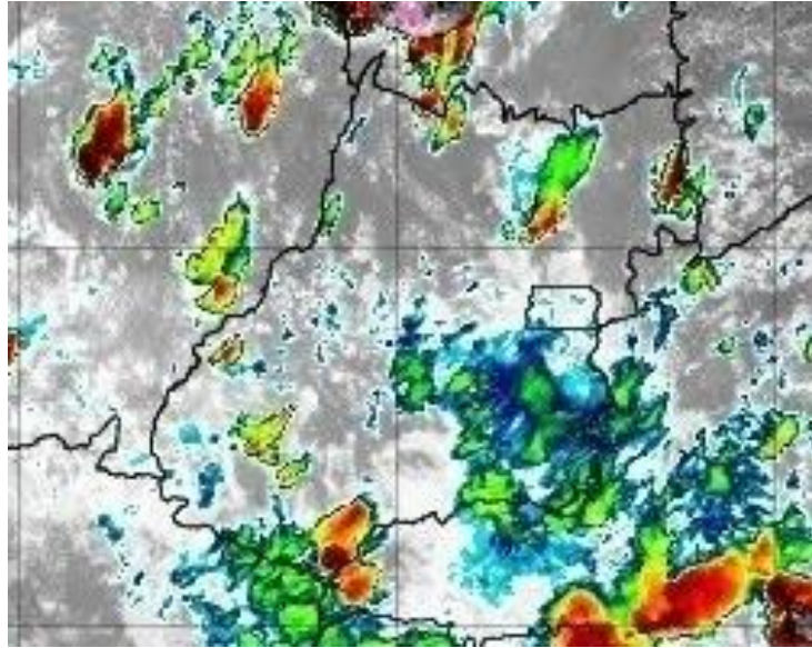
Figura 16 – Imagens realçadas do satélite GOES-16 das 13h00 do dia 19 de dezembro de 2019. FONTE: Cptec/INPE.
