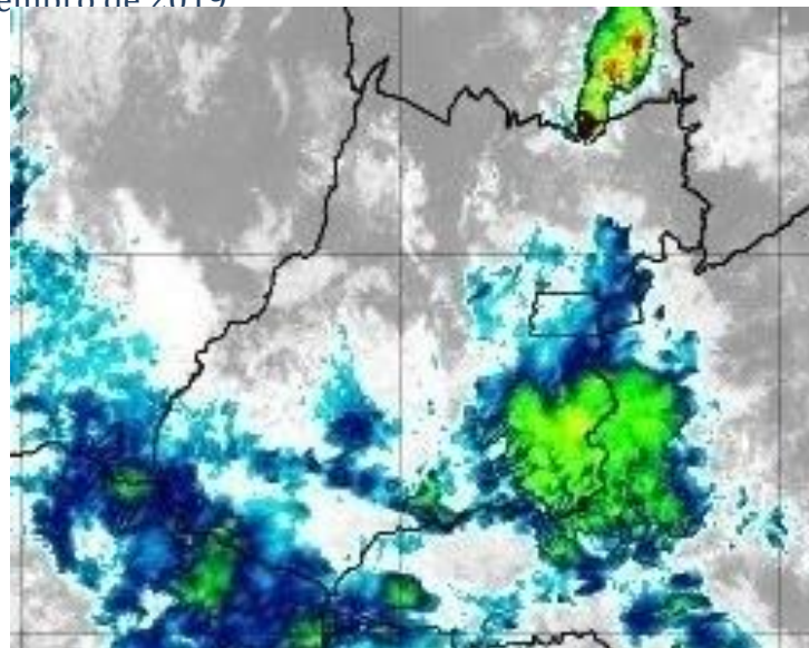
Figura 13 – Imagens realçadas do satélite GOES-16 das 07h00 do dia 19 de dezembro de 2019. FONTE: Cptec/INPE.
