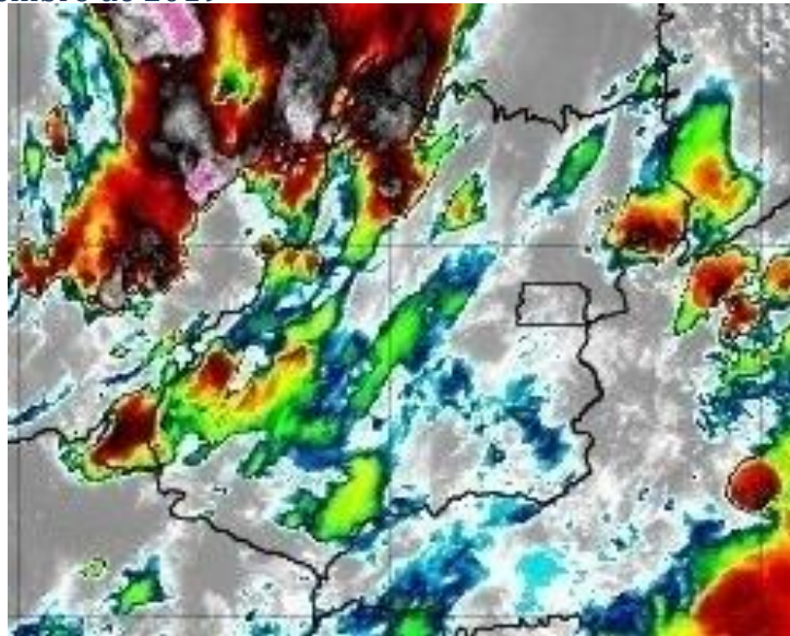
Figura 18 – Imagens realçadas do satélite GOES-16 das 17h00 do dia 19 de dezembro de 2019. FONTE: Cptec/INPE.
