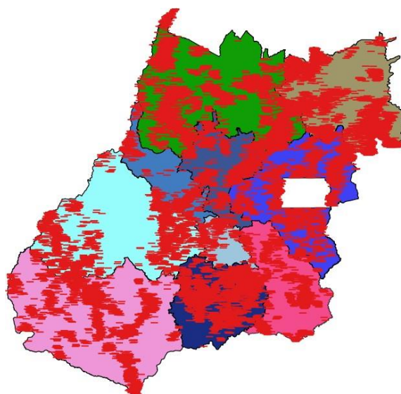
Figura 3 – Descargas atmosféricas nuvem-nuvem (em vermelho) detectadas pelo sistema Earth Networks entre 11h00 do dia 18 e 01h00 do dia 20 de dezembro de 2019 sobre a área de concessão da CELG Distribuição.
