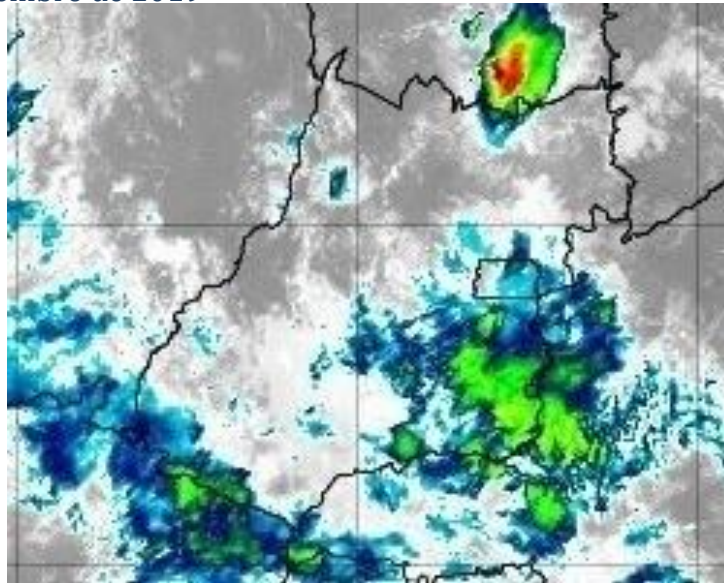
Figura 14 – Imagens realçadas do satélite GOES-16 das 09h00 do dia 19 de dezembro de 2019. FONTE: Cptec/INPE.
