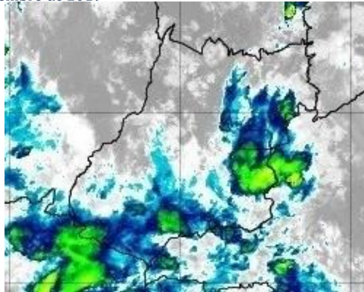
Figura 12 – Imagens realçadas do satélite GOES-16 das 05h00 do dia 19 de dezembro de 2019. FONTE: Cptec/INPE.
