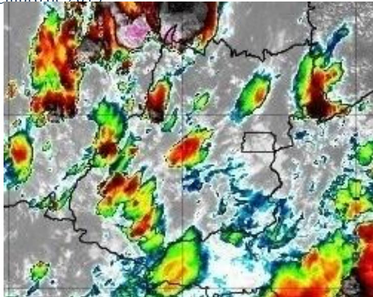
Figura 17 – Imagens realçadas do satélite GOES-16 das 15h00 do dia 19 de dezembro de 2019. FONTE: Cptec/INPE.
