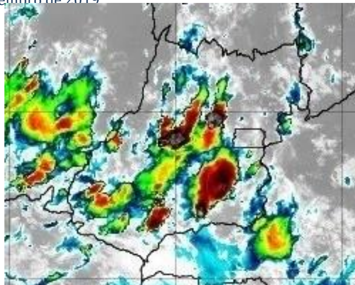
Figura 7 – Imagens realçadas do satélite GOES-16 das 19h00 do dia 18 de dezembro de 2019. FONTE: Cptec/INPE.
