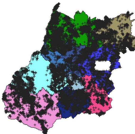
Figura 2 – Descargas atmosféricas nuvem-solo (em preto) detectadas pelo sistema Earth Networks entre 11h00 do dia 18 e 01h00 do dia 20 de dezembro de 2019 sobre a área de concessão da CELG Distribuição.
