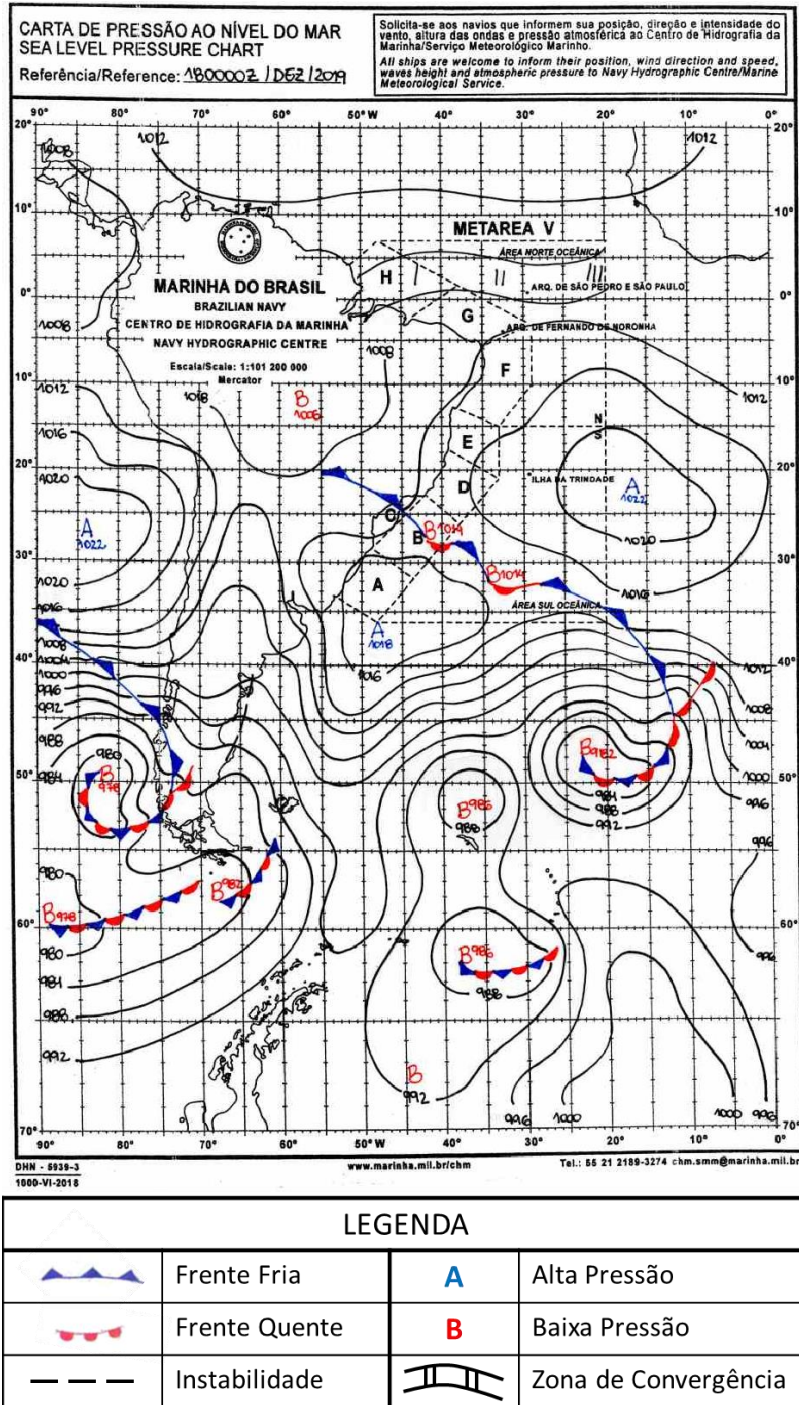
Figura A1 - Carta sinótica para as 0000Z do dia 18 de dezembro de 2019 (21h00 do dia 17 de dezembro de 2019, hora local. FONTE: Marinha do Brasil).
