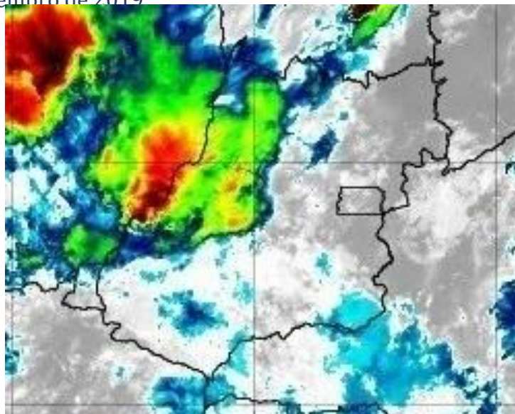
Figura 21 – Imagens realçadas do satélite GOES-16 das 23h00 do dia 19 de dezembro de 2019. FONTE: Cptec/INPE.
