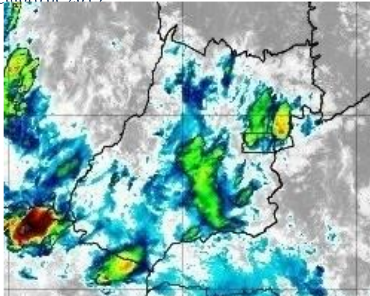
Figura 9 – Imagens realçadas do satélite GOES-16 das 23h00 do dia 18 de dezembro de 2019. FONTE: Cptec/INPE.
