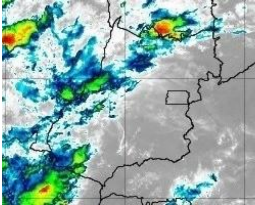
Figura 8 – Imagens realçadas do satélite GOES-16 das 23h00 do dia 27 de dezembro de 2019. FONTE: Cptec/INPE.
