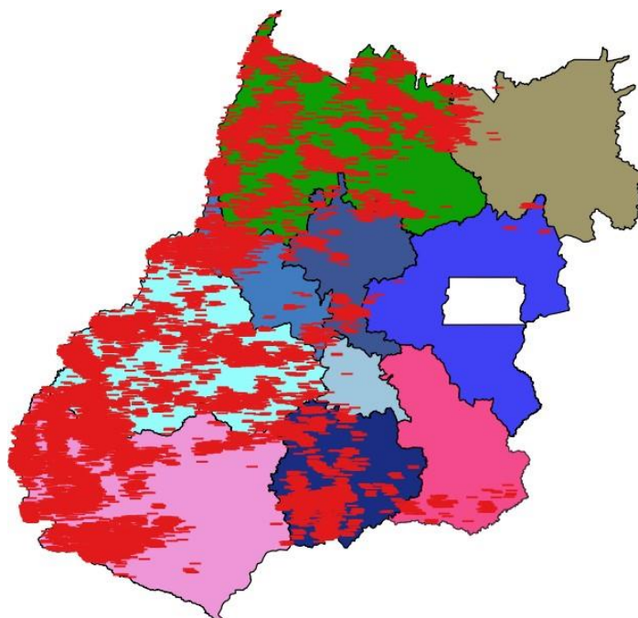
Figura 3 – Descargas atmosféricas nuvem-nuvem (em vermelho) detectadas pelo sistema Earth Networks entre 10h30 do dia 27 e as 04h00 do dia 28 de dezembro de 2019 sobre a área de concessão da CELG Distribuição.
