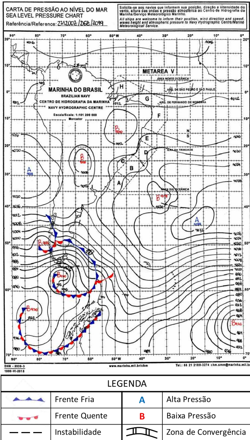
Figura A1 - Carta sinótica da Marinha do Brasil para as 1200Z do dia 27 de dezembro de 2019 (09h00 do dia 27 de dezembro de 2019, hora local). FONTE: Marinha do Brasil).
