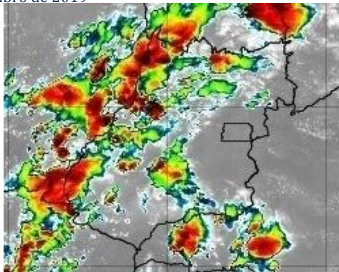
Figura 5 – Imagens realçadas do satélite GOES-16 das 17h00 do dia 27 de dezembro de 2019. FONTE: Cptec/INPE.
