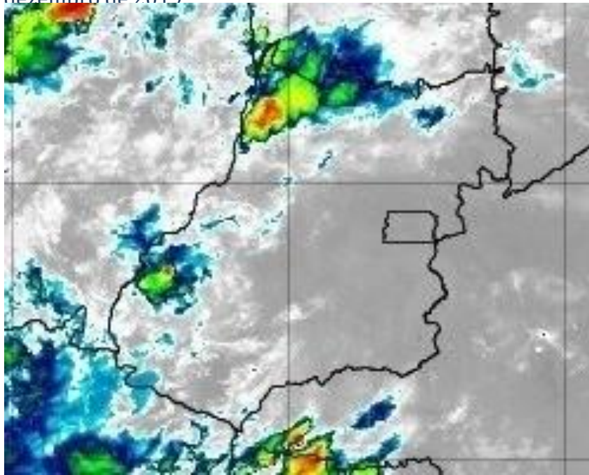
Figura 10 – Imagens realçadas do satélite GOES-16 das 03h00 do dia 28 de dezembro de 2019. FONTE: Cptec/INPE.
