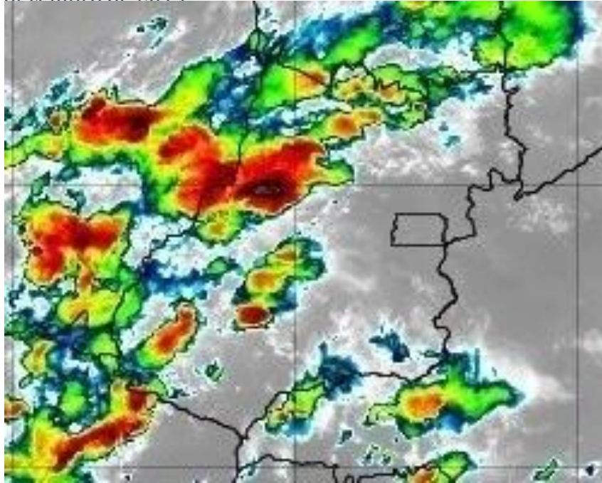
Figura 6 – Imagens realçadas do satélite GOES-16 das 19h00 do dia 27 de dezembro de 2019. FONTE: Cptec/INPE.
