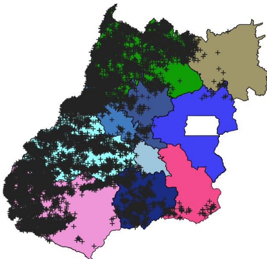
Figura 2 – Descargas atmosféricas nuvem-solo (em preto) detectadas pelo sistema Earth Networks entre 10h30 do dia 27 e as 04h00 do dia 28 de dezembro de 2019 sobre a área de concessão da CELG Distribuição.
