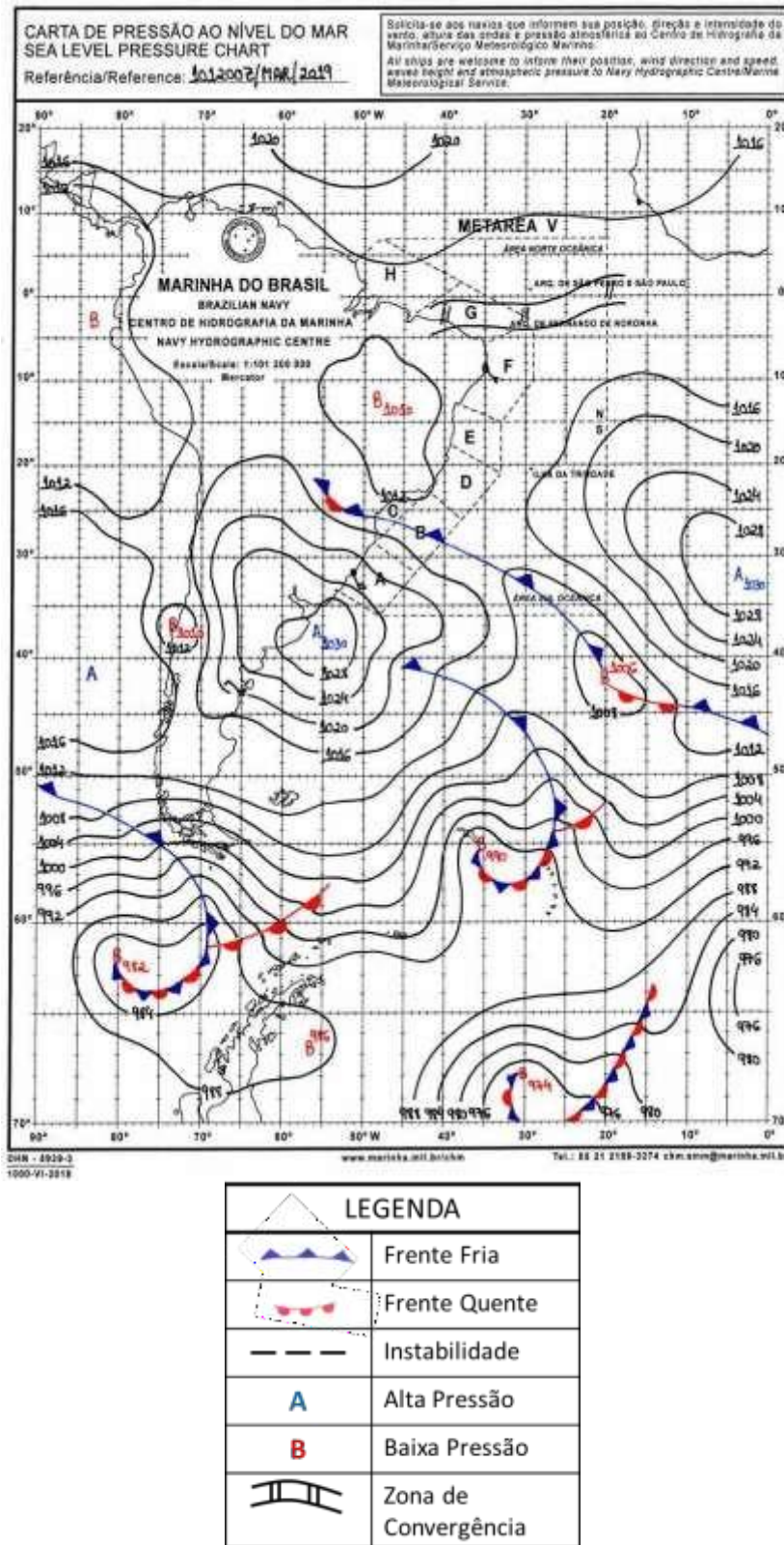
Figura A1 – Carta sinótica da Marinha do Brasil para as 1200Z do dia 10 de março de 2019 (09h00 do dia 10 de março de 2019, hora local).
