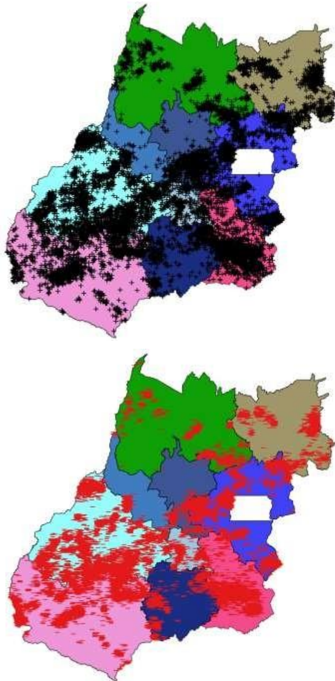
Figura 2 – Descargas atmosféricas nuvem-solo (em preto) e nuvem-nuvem (em vermelho) detectadas pelo sistema Earth Networks entre 10h55 do dia 10 e 08h00 do dia 11 de março de 2019 sobre a área de concessão da Enel Distribuição Goiás.
