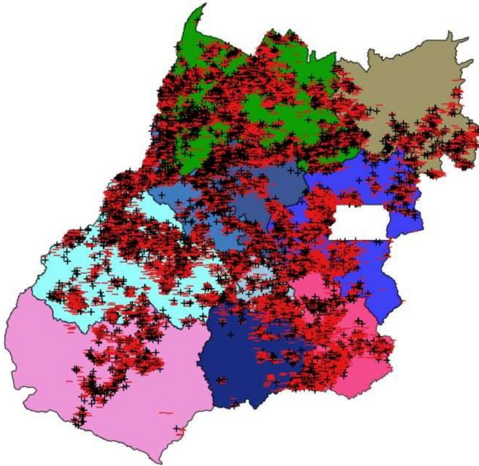
Figura 2 – Descargas atmosféricas nuvem-solo (em preto) e nuvem-nuvem (em vermelho) detectadas pelo sistema Earth Networks entre 10h00 do dia 12 e 04h00 do dia 13 de janeiro de 2019 sobre a área de concessão da ENEL DISTRIBUIÇÃO GOIÁS.
