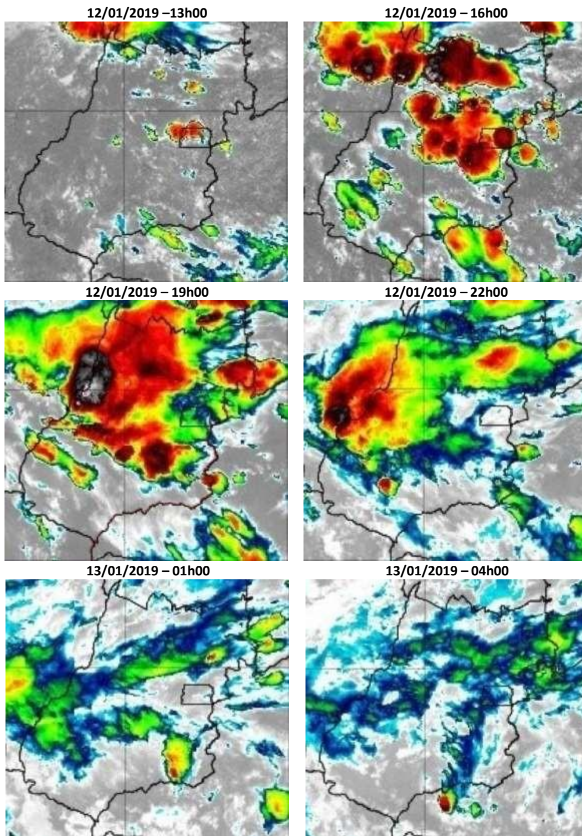
Figura 3 – Imagens realçadas do satélite GOES-16 entre as 13h00 do dia 12 e 04h00 do dia 13 de janeiro de 2019.
