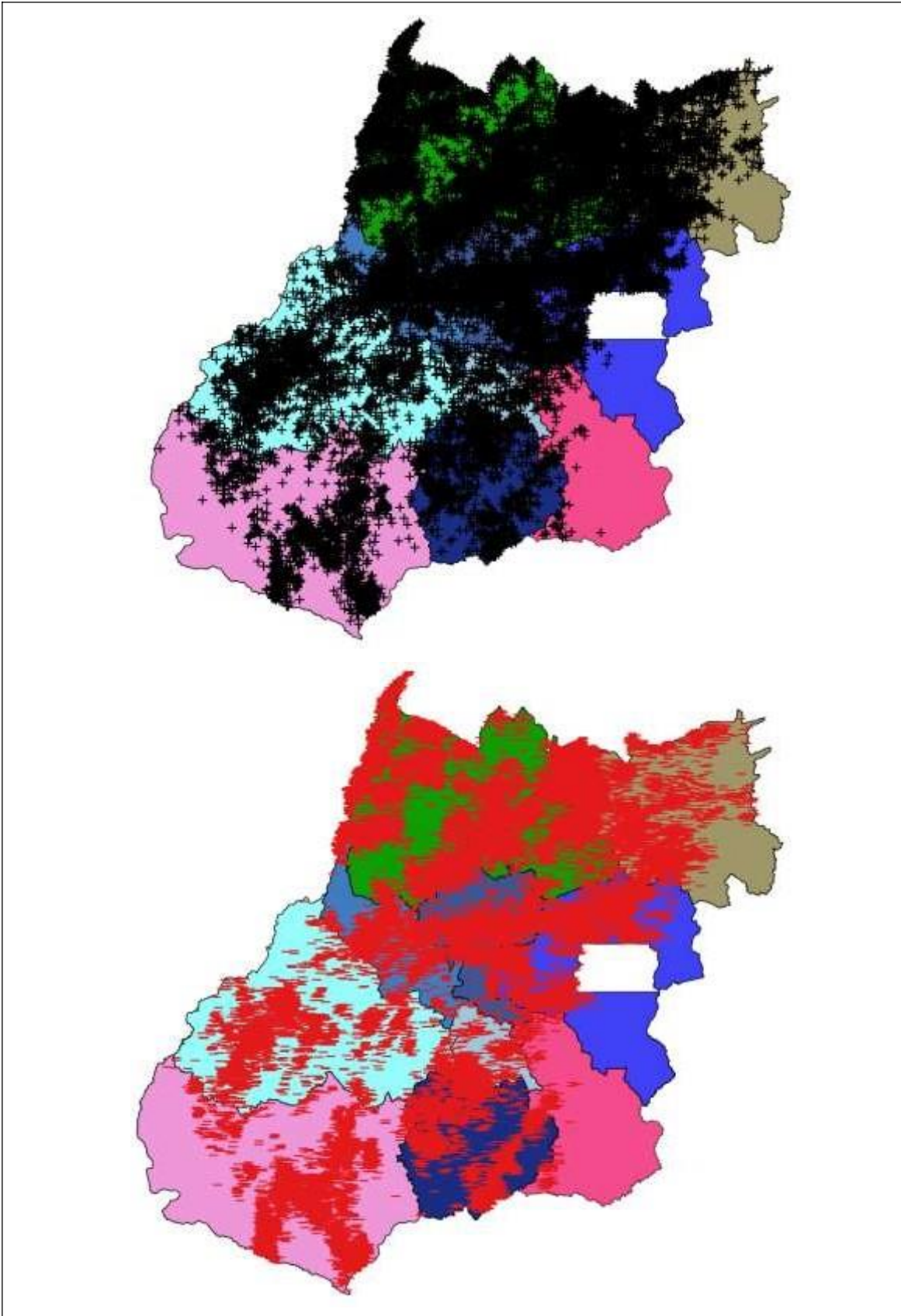
Figura 2 – Descargas atmosféricas nuvem-solo (em preto) e nuvem-nuvem (em vermelho) detectadas pelo sistema Earth Networks entre 10h50 do dia 22 e 10h00 do dia 23 de fevereiro de 2019 sobre a área de concessão da CELG Distribuição.
