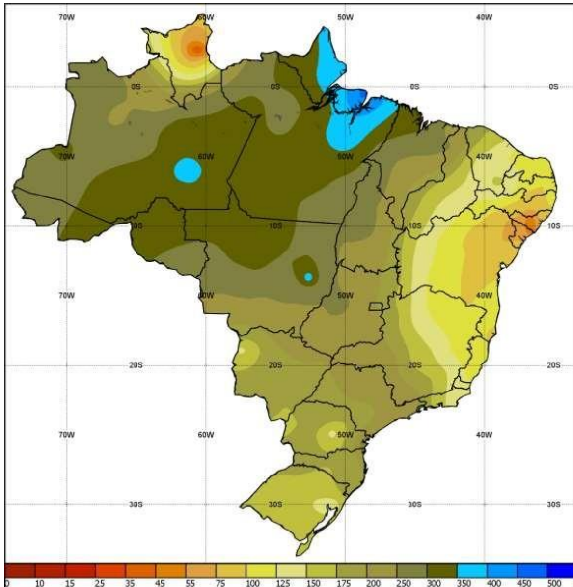
Figura A3 – Média climatológica (1981-2010) de precipitação acumulada para o mês de fevereiro.
