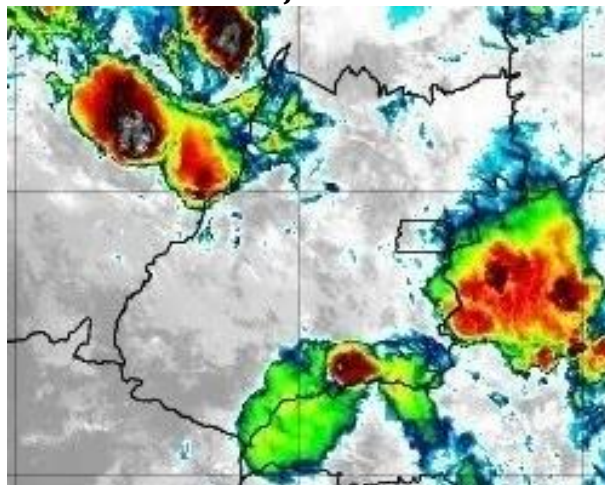
Figura 13 – Imagens realçadas do satélite GOES-16 das 01h00 do dia 04 de janeiro de 2020. FONTE: Cptec/INPE.
