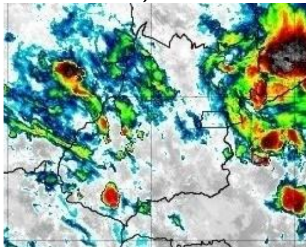
Figura 31 – Imagens realçadas do satélite GOES-16 das 03h00 do dia 07 de janeiro de 2020. FONTE: Cptec/INPE.
