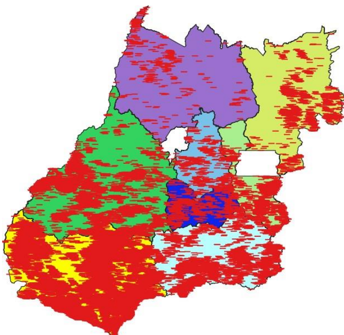
Figura 3 – Descargas atmosféricas nuvem-nuvem (em vermelho) detectadas pelo sistema Earth Networks entre 09h30 do dia 02 e 08h00 do dia 07 de janeiro de 2020 sobre a área de concessão da CELG Distribuição.
