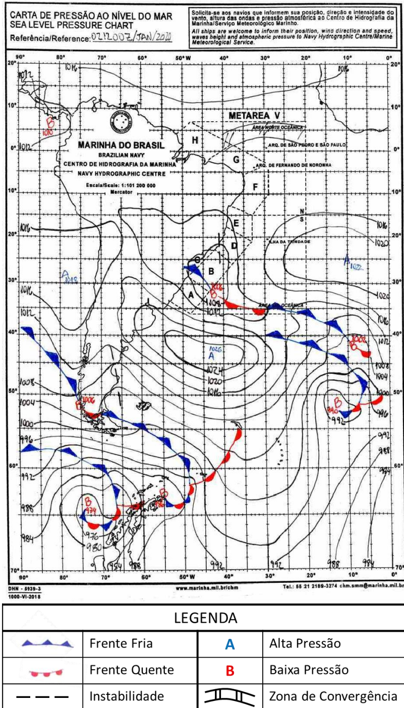
Figura A1 - Carta sinótica para as 1200Z do dia 02 de janeiro de 2020 (0900 do dia 02 de janeiro de 2020 hora local. FONTE: Marinha do Brasil).
