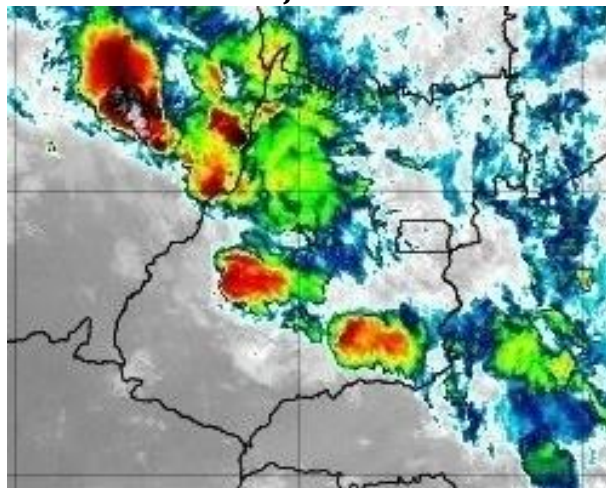
Figura 15 – Imagens realçadas do satélite GOES-16 das 09h00 do dia 04 de janeiro de 2020. FONTE: Cptec/INPE.
