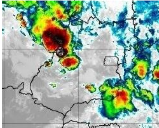
Figura 14 – Imagens realçadas do satélite GOES-16 das 05h00 do dia 04 de janeiro de 2020. FONTE: Cptec/INPE.
