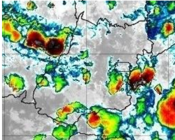
Figura 12 – Imagens realçadas do satélite GOES-16 das 21h00 do dia 03 de janeiro de 2020. FONTE: Cptec/INPE.
