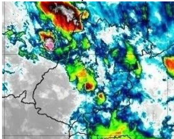
Figura 7 – Imagens realçadas do satélite GOES-16 das 01h00 do dia 03 de janeiro de 2020. FONTE: Cptec/INPE.
