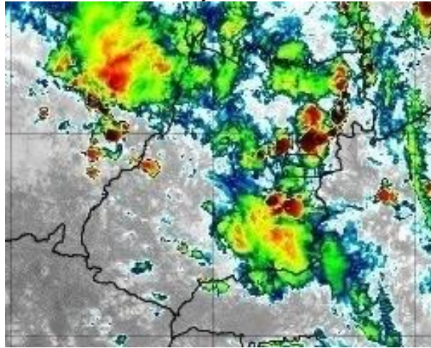
Figura 16 – Imagens realçadas do satélite GOES-16 das 13h00 do dia 04 de janeiro de 2020. FONTE: Cptec/INPE.
