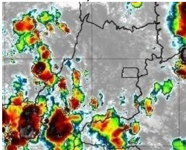
Figura 29 – Imagens realçadas do satélite GOES-16 das 17h00 do dia 06 de janeiro de 2020. FONTE: Cptec/INPE.
