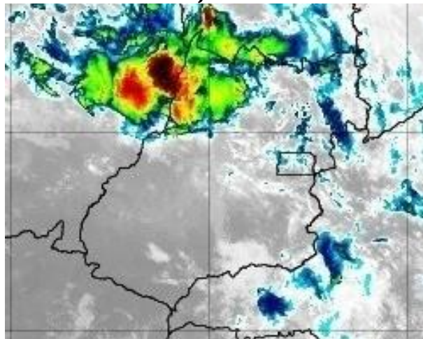
Figura 9 – Imagens realçadas do satélite GOES-16 das 09h00 do dia 03 de janeiro de 2020. FONTE: Cptec/INPE.
