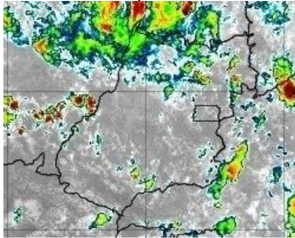
Figura 10 – Imagens realçadas do satélite GOES-16 das 13h00 do dia 03 de janeiro de 2020. FONTE: Cptec/INPE.
