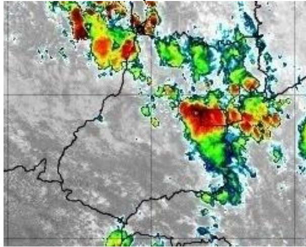
Figura 22 – Imagens realçadas do satélite GOES-16 das 13h00 do dia 05 de janeiro de 2020. FONTE: Cptec/INPE.
