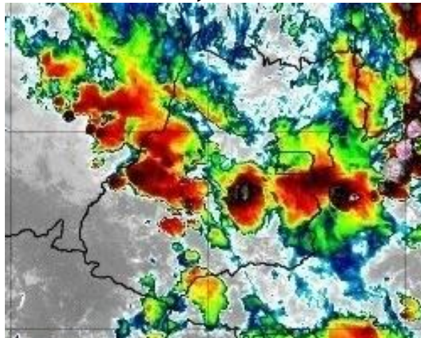
Figura 17 – Imagens realçadas do satélite GOES-16 das 17h00 do dia 04 de janeiro de 2020. FONTE: Cptec/INPE.
