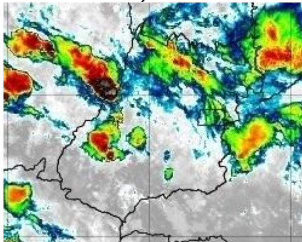
Figura 32 – Imagens realçadas do satélite GOES-16 das 07h00 do dia 07 de janeiro de 2020. FONTE: Cptec/INPE.
