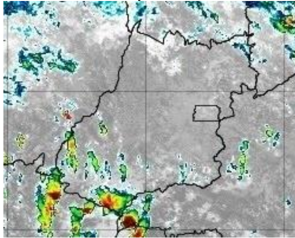
Figura 28 – Imagens realçadas do satélite GOES-16 das 13h00 do dia 06 de janeiro de 2020. FONTE: Cptec/INPE.
