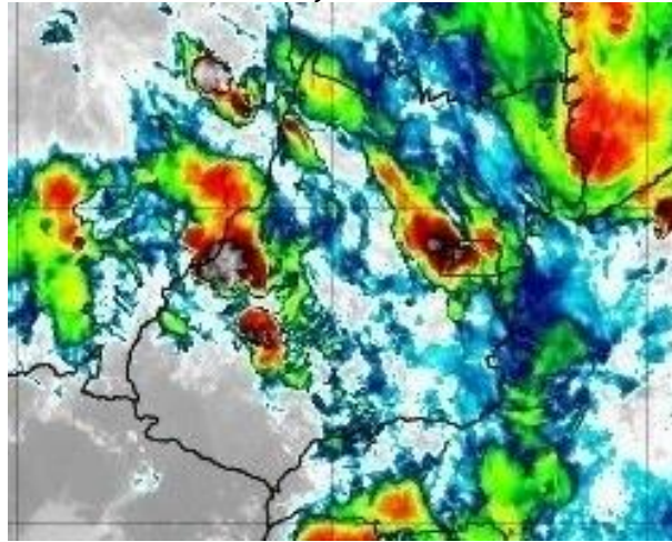
Figura 6 – Imagens realçadas do satélite GOES-16 das 21h00 do dia 02 de janeiro de 2020. FONTE: Cptec/INPE.
