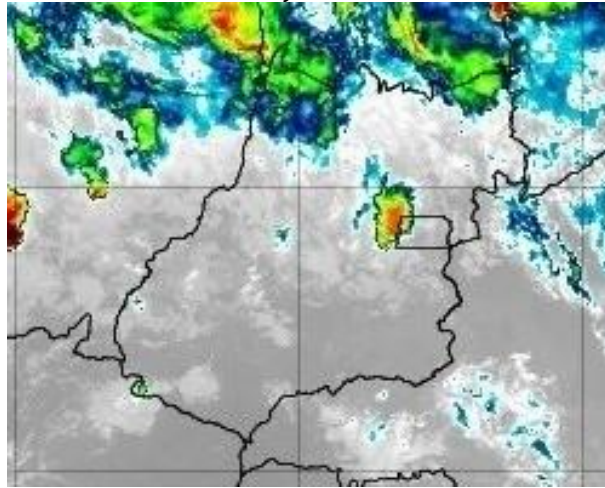
Figura 26 – Imagens realçadas do satélite GOES-16 das 05h00 do dia 06 de janeiro de 2020. FONTE: Cptec/INPE.
