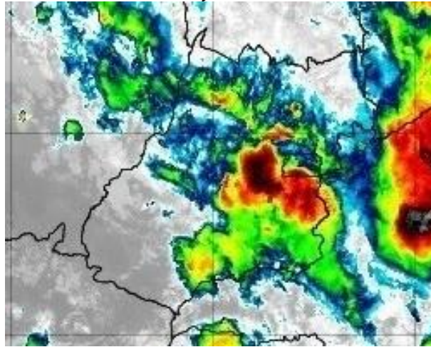
Figura 18 – Imagens realçadas do satélite GOES-16 das 21h00 do dia 04 de janeiro de 2020. FONTE: Cptec/INPE.
