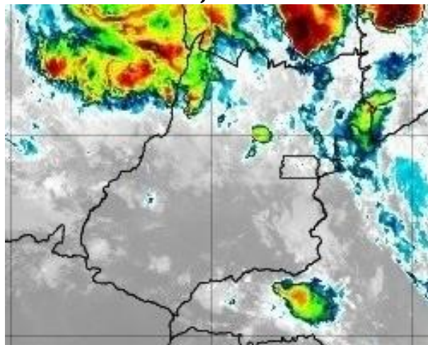
Figura 25 – Imagens realçadas do satélite GOES-16 das 01h00 do dia 06 de janeiro de 2020. FONTE: Cptec/INPE.
