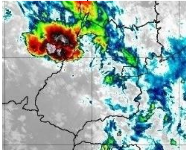
Figura 8 – Imagens realçadas do satélite GOES-16 das 05h00 do dia 03 de janeiro de 2020. FONTE: Cptec/INPE.
