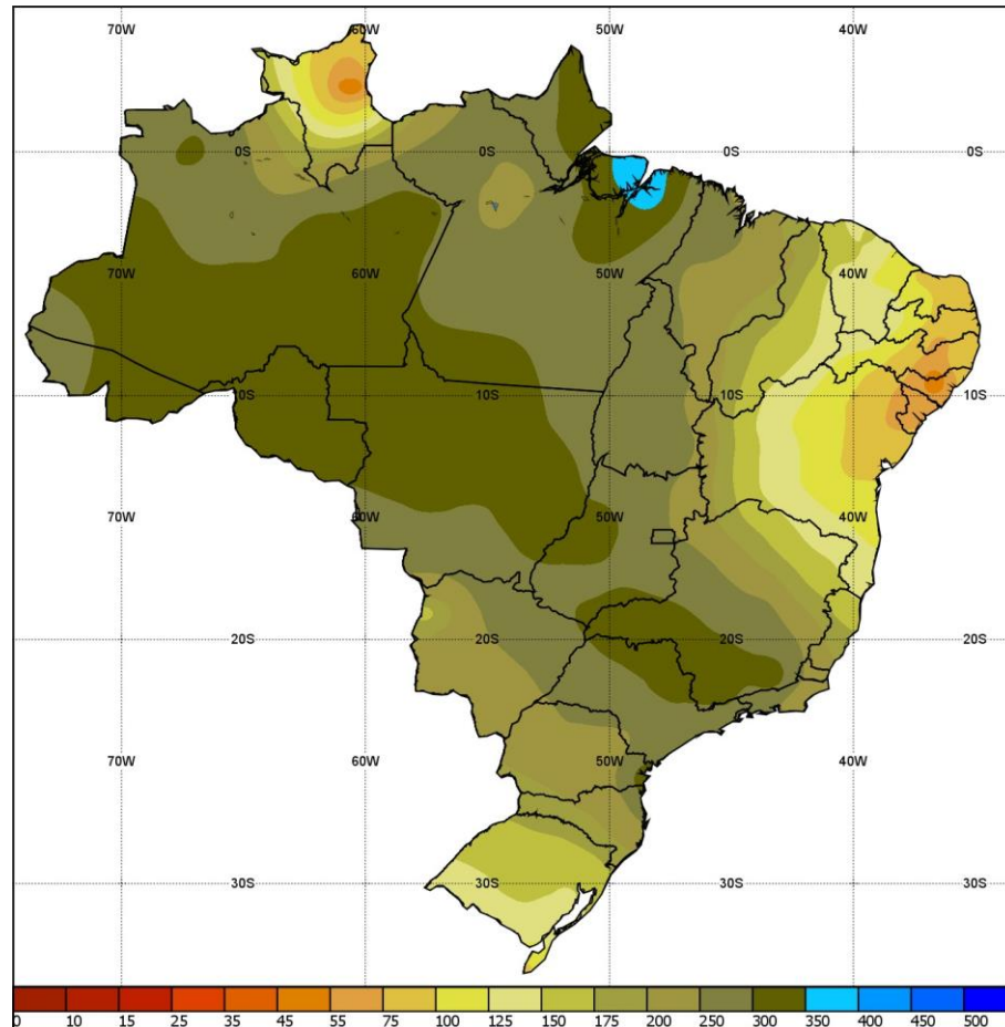
Figura A6 - Média climatológica de precipitação acumulada para o mês de janeiro. Fonte: INMET.
