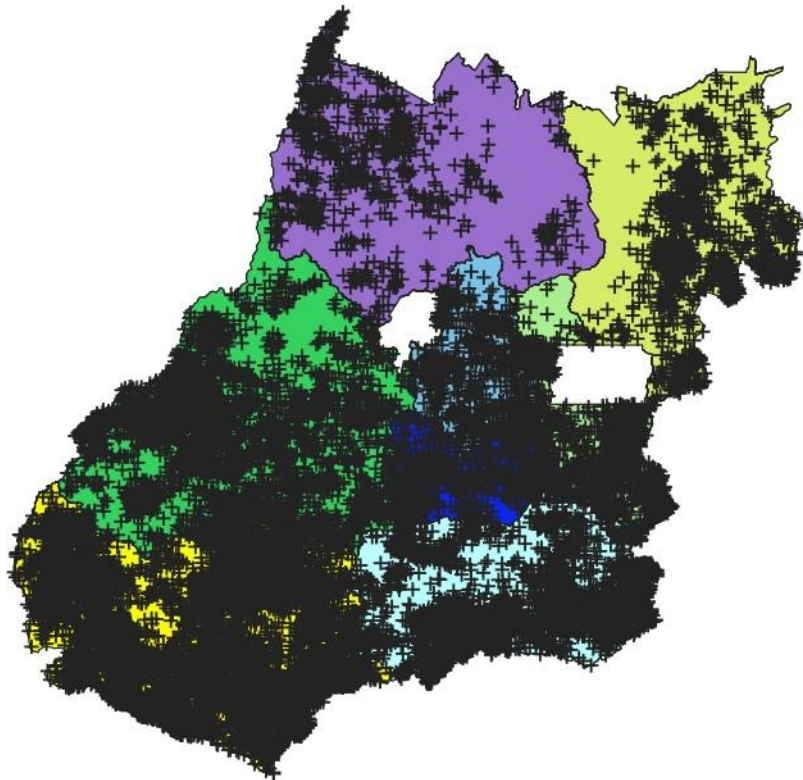
Figura 2 – Descargas atmosféricas nuvem-solo (em preto) detectadas pelo sistema Earth Networks entre 09h30 do dia 02 e 08h00 do dia 07 de janeiro de 2020 sobre a área de concessão da CELG Distribuição.
