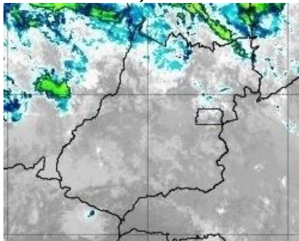
Figura 27 – Imagens realçadas do satélite GOES-16 das 09h00 do dia 06 de janeiro de 2020. FONTE: Cptec/INPE.
