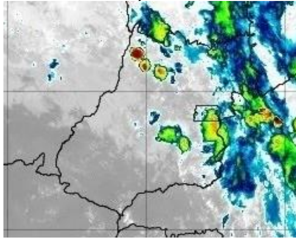
Figura 20 – Imagens realçadas do satélite GOES-16 das 05h00 do dia 05 de janeiro de 2020. FONTE: Cptec/INPE.
