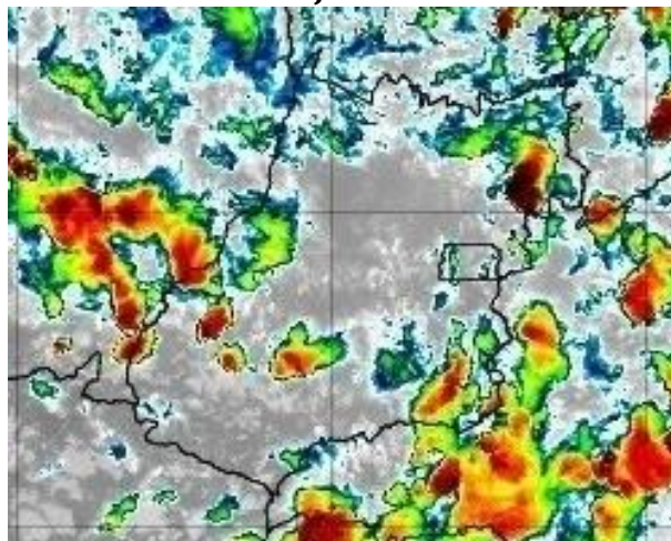
Figura 11 – Imagens realçadas do satélite GOES-16 das 17h00 do dia 03 de janeiro de 2020. FONTE: Cptec/INPE.
