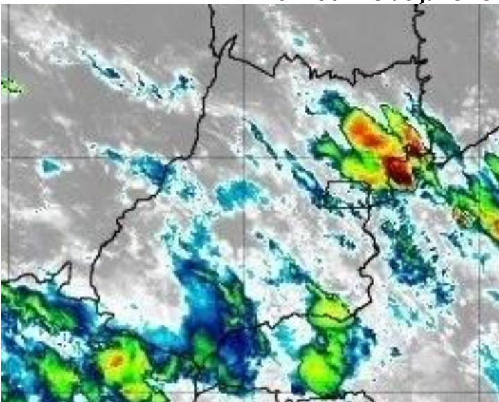
Figura 21 – Imagens realçadas do satélite GOES-16 das 01h00 do dia 18 de janeiro de 2020. FONTE: Cptec/INPE.
