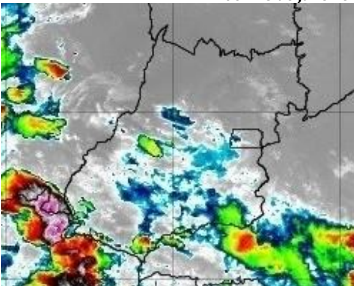
Figura 7 – Imagens realçadas do satélite GOES-16 das 21h00 do dia 16 de janeiro de 2020. FONTE: Cptec/INPE.
