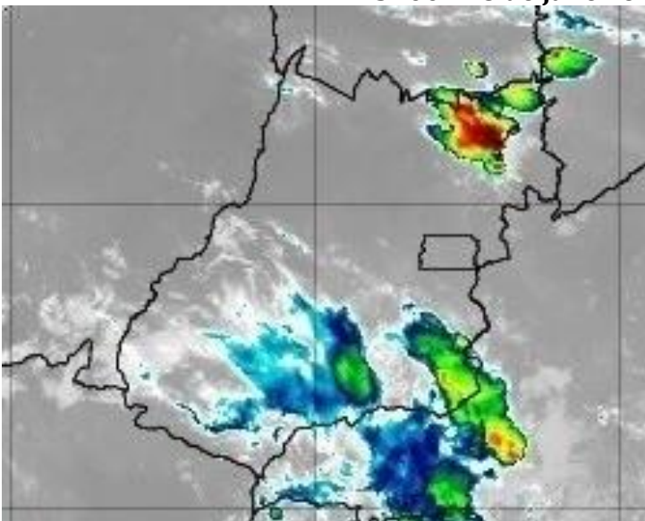
Figura 31 – Imagens realçadas do satélite GOES-16 das 23h00 do dia 18 de janeiro de 2020. FONTE: Cptec/INPE.
