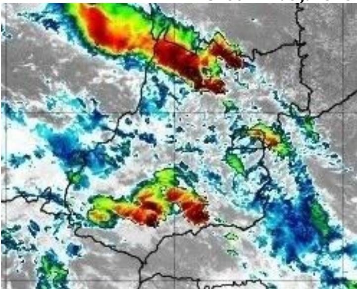
Figura 15 – Imagens realçadas do satélite GOES-16 das 13h00 do dia 17 de janeiro de 2020. FONTE: Cptec/INPE.
