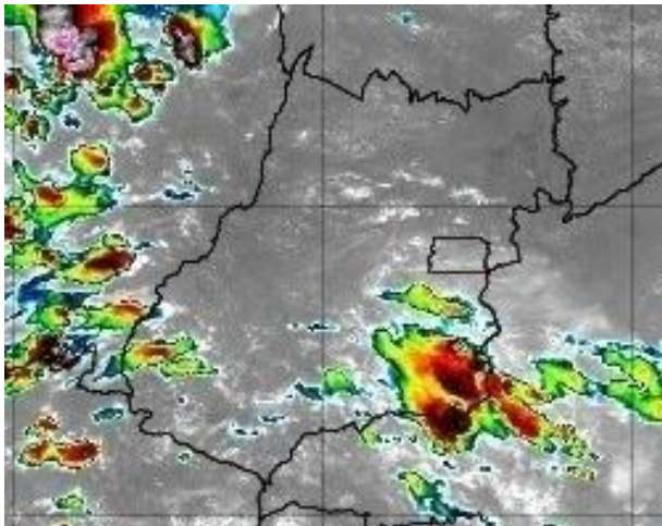
Figura 4 – Imagens realçadas do satélite GOES-16 das 15h00 do dia 16 de janeiro de 2020. FONTE: Cptec/INPE.
