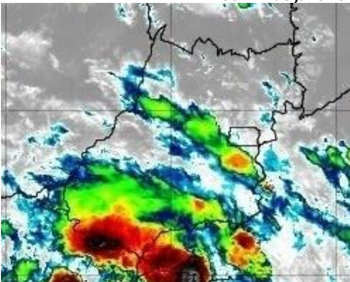
Figura 19 – Imagens realçadas do satélite GOES-16 das 21h00 do dia 17 de janeiro de 2020. FONTE: Cptec/INPE.
