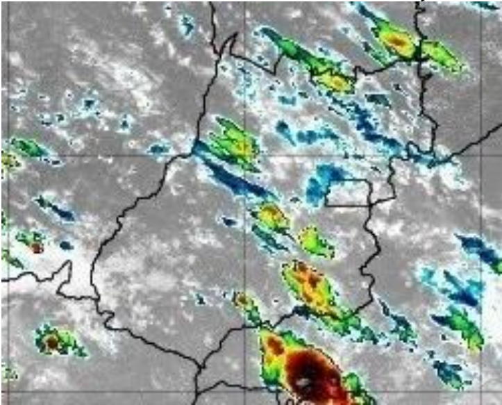
Figura 28 – Imagens realçadas do satélite GOES-16 das 15h00 do dia 18 de janeiro de 2020. FONTE: Cptec/INPE.
