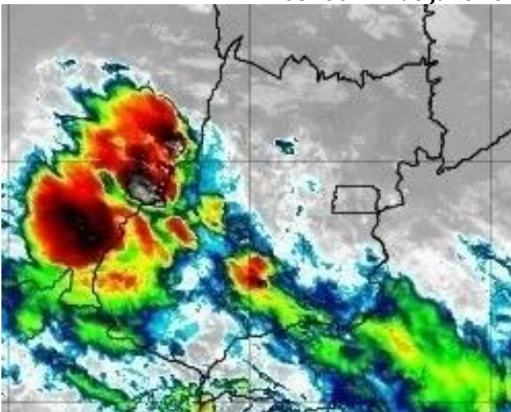
Figura 11 – Imagens realçadas do satélite GOES-16 das 05h00 do dia 17 de janeiro de 2020. FONTE: Cptec/INPE.
