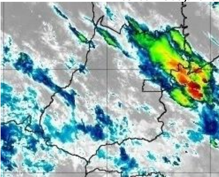
Figura 23 – Imagens realçadas do satélite GOES-16 das 05h00 do dia 18 de janeiro de 2020. FONTE: Cptec/INPE.
