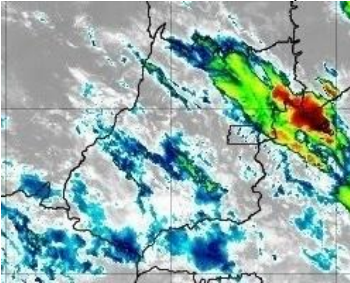
Figura 22 – Imagens realçadas do satélite GOES-16 das 03h00 do dia 18 de janeiro de 2020. FONTE: Cptec/INPE.
