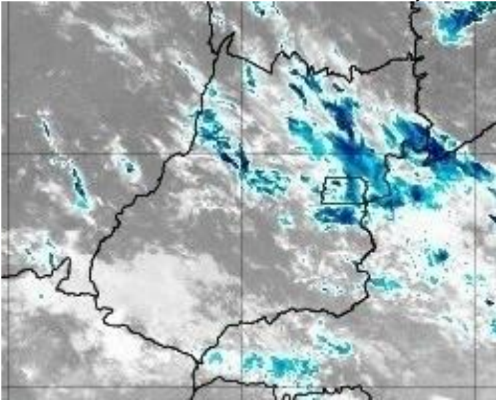
Figura 26 – Imagens realçadas do satélite GOES-16 das 11h00 do dia 18 de janeiro de 2020. FONTE: Cptec/INPE.
