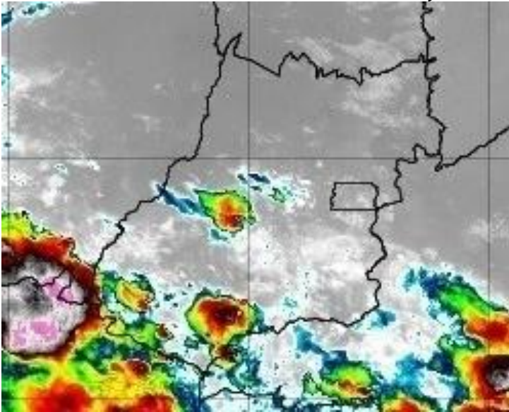
Figura 8 – Imagens realçadas do satélite GOES-16 das 23h00 do dia 16 de janeiro de 2020. FONTE: Cptec/INPE.
