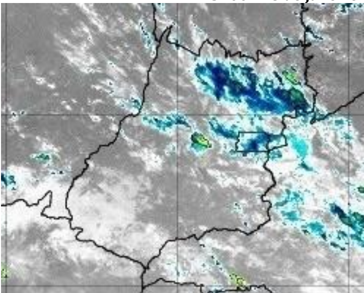
Figura 27 – Imagens realçadas do satélite GOES-16 das 13h00 do dia 18 de janeiro de 2020. FONTE: Cptec/INPE.
