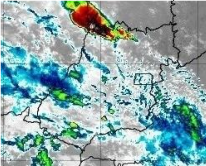
Figura 14 – Imagens realçadas do satélite GOES-16 das 11h00 do dia 17 de janeiro de 2020. FONTE: Cptec/INPE.
