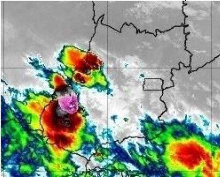
Figura 10 – Imagens realçadas do satélite GOES-16 das 03h00 do dia 17 de janeiro de 2020. FONTE: Cptec/INPE.
