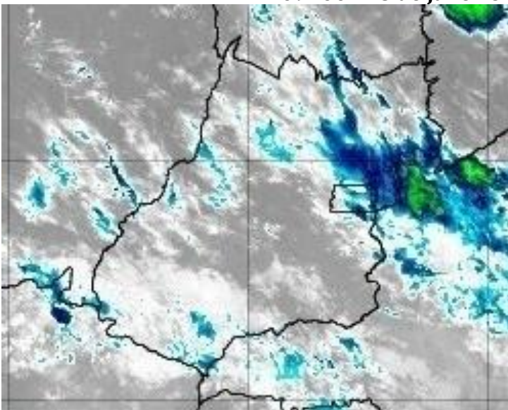
Figura 25 – Imagens realçadas do satélite GOES-16 das 09h00 do dia 18 de janeiro de 2020. FONTE: Cptec/INPE.
