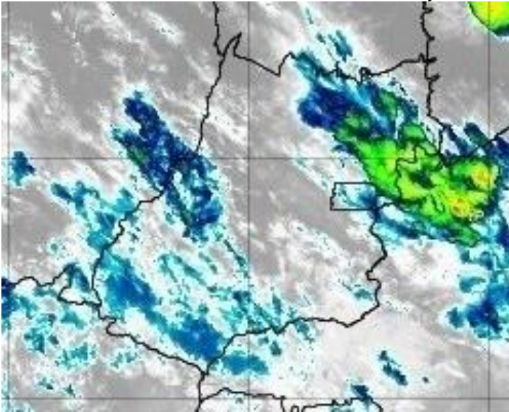
Figura 24 – Imagens realçadas do satélite GOES-16 das 07h00 do dia 18 de janeiro de 2020. FONTE: Cptec/INPE.
