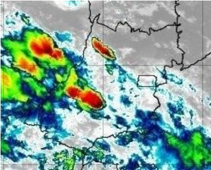
Figura 12 – Imagens realçadas do satélite GOES-16 das 07h00 do dia 17 de janeiro de 2020. FONTE: Cptec/INPE.
