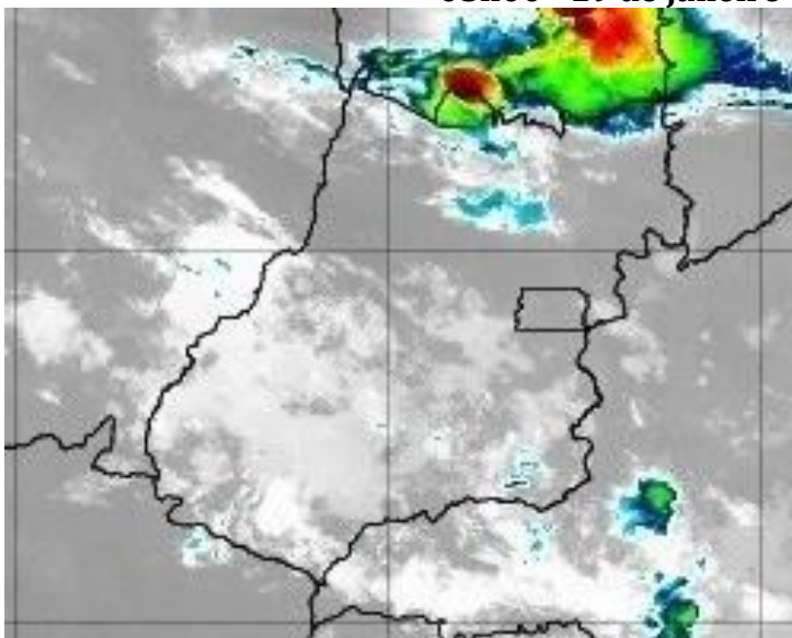
Figura 34 – Imagens realçadas do satélite GOES-16 das 05h00 do dia 19 de janeiro de 2020. FONTE: Cptec/INPE.
