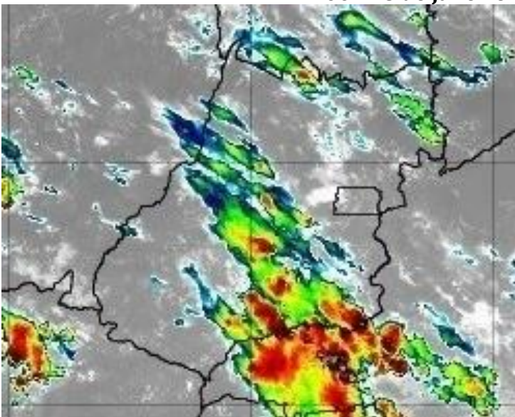
Figura 29 – Imagens realçadas do satélite GOES-16 das 17h00 do dia 18 de janeiro de 2020. FONTE: Cptec/INPE.
