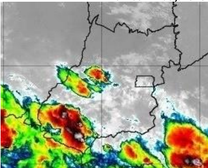
Figura 9 – Imagens realçadas do satélite GOES-16 das 01h00 do dia 17 de janeiro de 2020. FONTE: Cptec/INPE.
