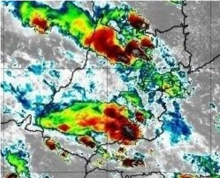
Figura 16 – Imagens realçadas do satélite GOES-16 das 15h00 do dia 17 de janeiro de 2020. FONTE: Cptec/INPE.
