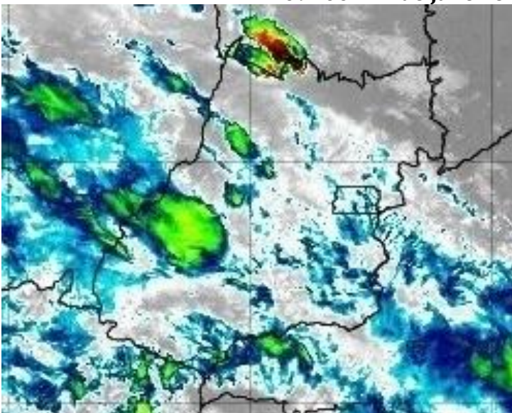
Figura 13 – Imagens realçadas do satélite GOES-16 das 09h00 do dia 17 de janeiro de 2020. FONTE: Cptec/INPE.
