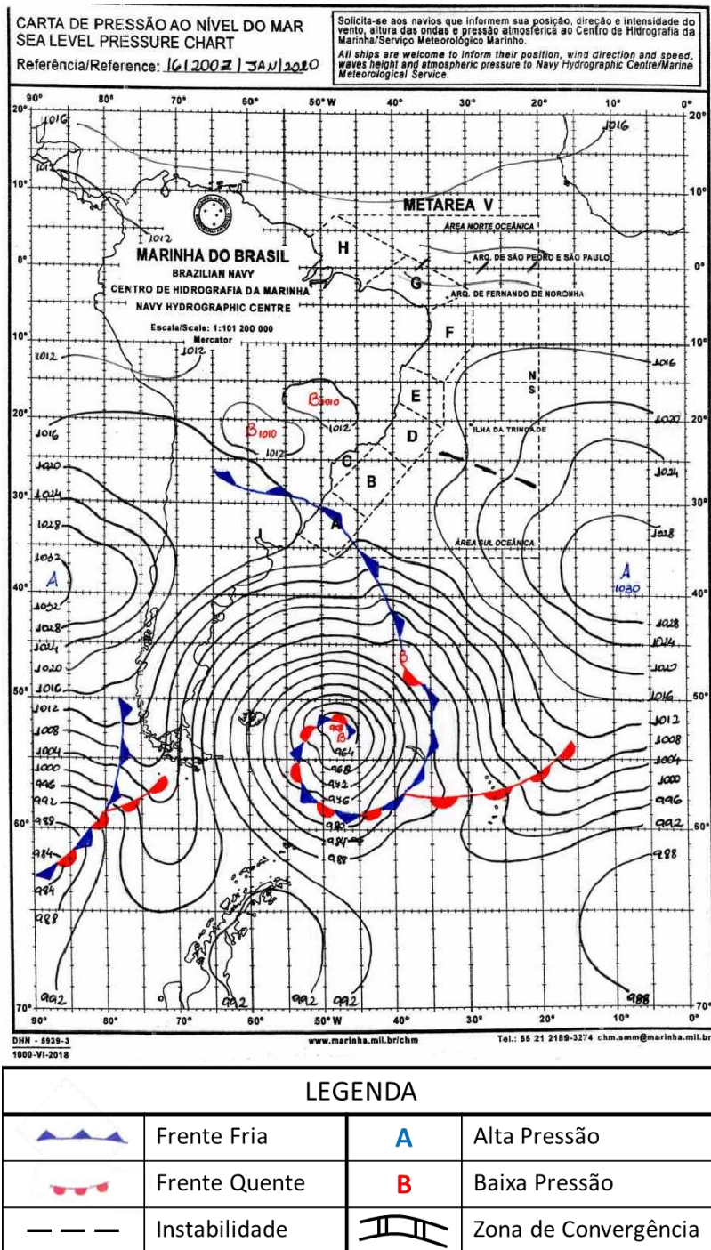
Figura A1 - Carta sinótica para as 1200Z do dia 16 de janeiro de 2020 (09h00 do dia 16 de janeiro de 2020 hora local. FONTE: Marinha do Brasil).
