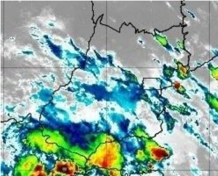
Figura 20 – Imagens realçadas do satélite GOES-16 das 23h00 do dia 17 de janeiro de 2020. FONTE: Cptec/INPE.
