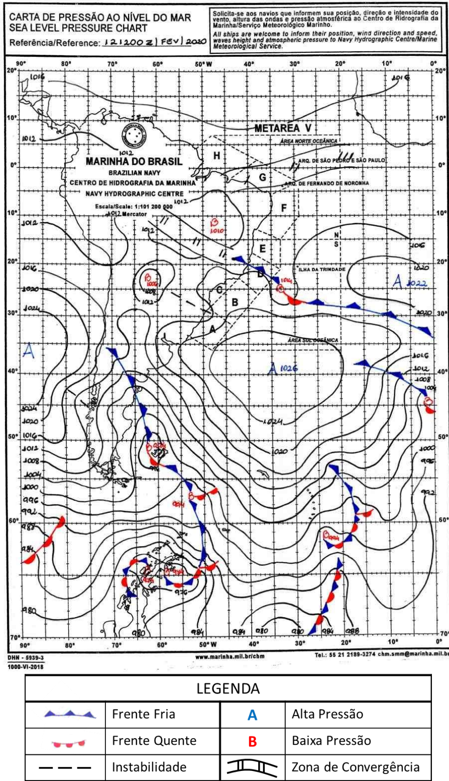
Figura A2 - Carta sinótica para as 1200Z do dia 12 de fevereiro de 2020 (09h00 do dia 12 de fevereiro de 2020 hora local. FONTE: Marinha do Brasil).
