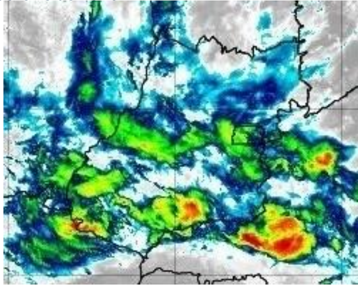
Figura 16 – Imagens realçadas do satélite GOES-16 das 3h00 do dia 13 de Fevereiro de 2020. FONTE: Cptec/INPE.
