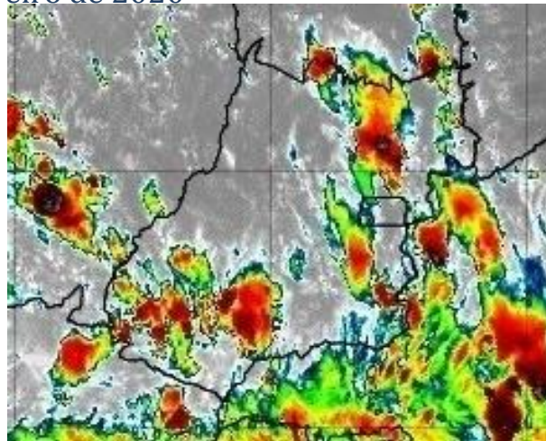
Figura 4 – Imagens realçadas do satélite GOES-16 das 15h00 do dia 11 de Fevereiro de 2020. FONTE: Cptec/INPE.
