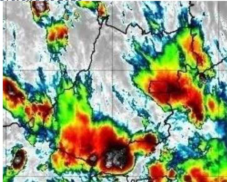
Figura 6 – Imagens realçadas do satélite GOES-16 das 21h00 do dia 11 de Fevereiro de 2020. FONTE: Cptec/INPE.
