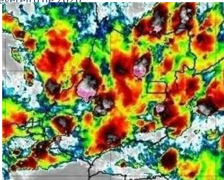
Figura 13 – Imagens realçadas do satélite GOES-16 das 18h00 do dia 12 de Fevereiro de 2020. FONTE: Cptec/INPE.
