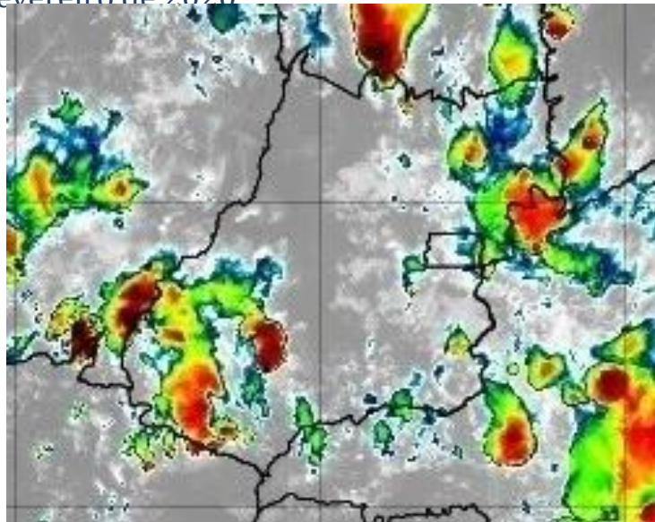
Figura 21 – Imagens realçadas do satélite GOES-16 das 18h00 do dia 13 de Fevereiro de 2020. FONTE: Cptec/INPE.
