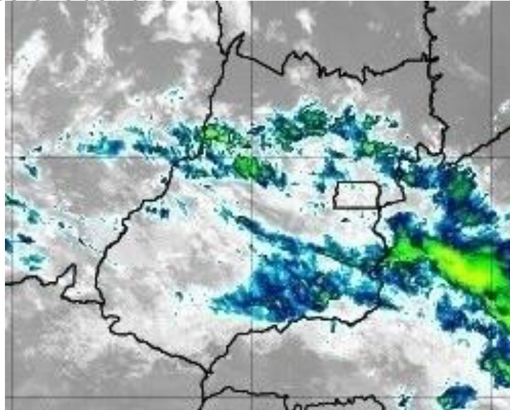
Figura 18 – Imagens realçadas do satélite GOES-16 das 9h00 do dia 13 de Fevereiro de 2020. FONTE: Cptec/INPE.
