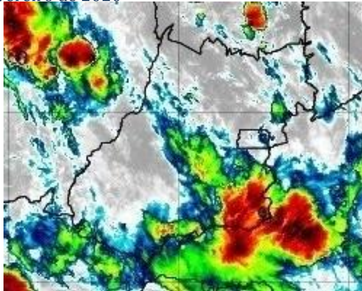
Figura 8 – Imagens realçadas do satélite GOES-16 das 3h00 do dia 12 de Fevereiro de 2020. FONTE: Cptec/INPE.
