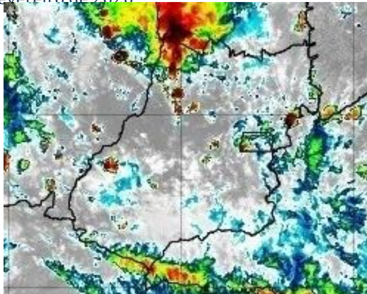
Figura 11 – Imagens realçadas do satélite GOES-16 das 12h00 do dia 12 de Fevereiro de 2020. FONTE: Cptec/INPE.
