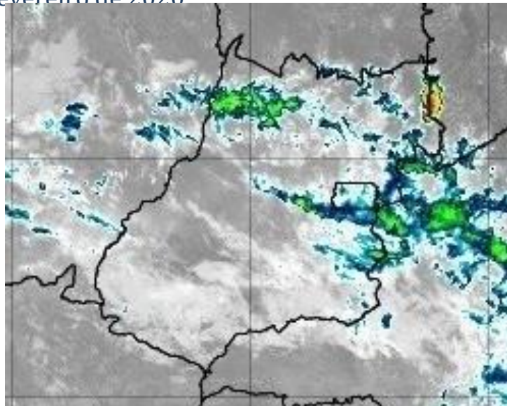
Figura 19 – Imagens realçadas do satélite GOES-16 das 12h00 do dia 13 de Fevereiro de 2020. FONTE: Cptec/INPE.
