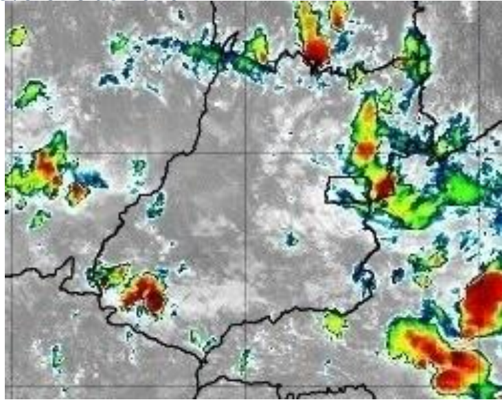
Figura 20 – Imagens realçadas do satélite GOES-16 das 15h00 do dia 13 de Fevereiro de 2020. FONTE: Cptec/INPE.
