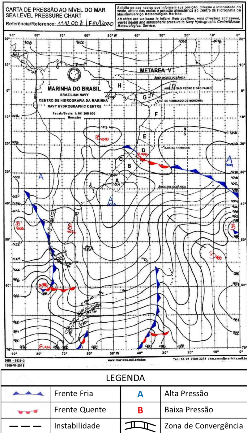
Figura A1 - Carta sinótica para as 1200Z do dia 11 de fevereiro de 2020 (09h00 do dia 11 de fevereiro de 2020 hora local. FONTE: Marinha do Brasil).
