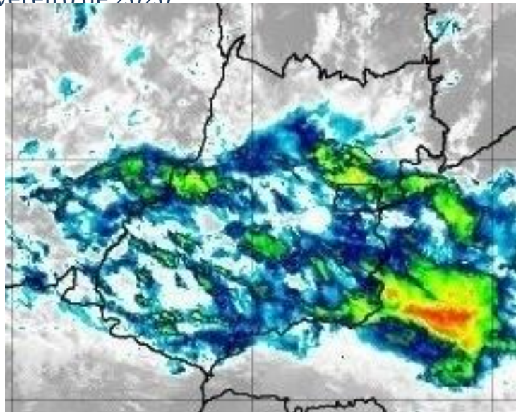
Figura 17 – Imagens realçadas do satélite GOES-16 das 6h00 do dia 13 de Fevereiro de 2020. FONTE: Cptec/INPE.
