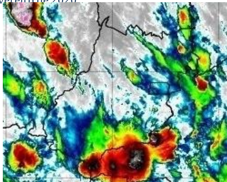
Figura 7 – Imagens realçadas do satélite GOES-16 das 0h00 do dia 12 de Fevereiro de 2020. FONTE: Cptec/INPE.
