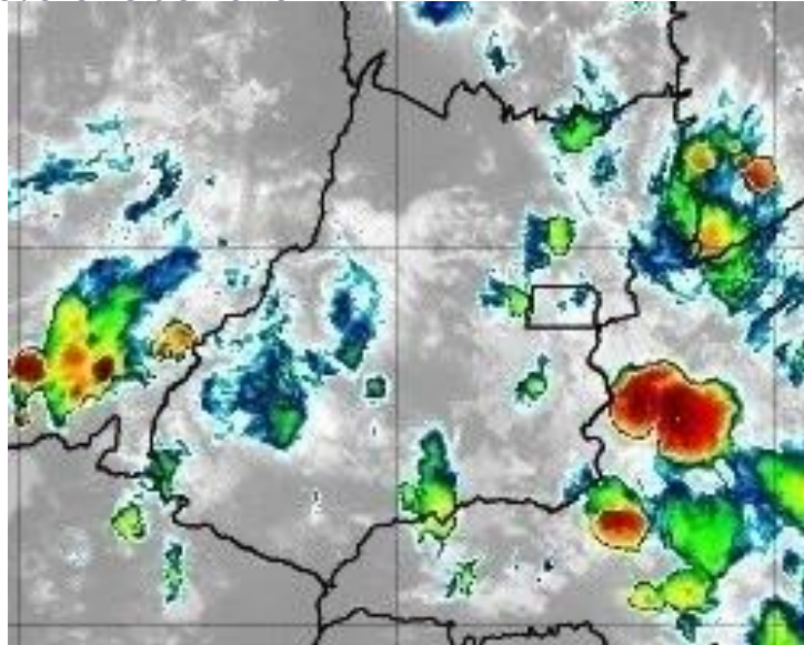
Figura 22 – Imagens realçadas do satélite GOES-16 das 21h00 do dia 13 de Fevereiro de 2020. FONTE: Cptec/INPE.
