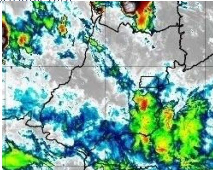
Figura 9 – Imagens realçadas do satélite GOES-16 das 6h00 do dia 12 de Fevereiro de 2020. FONTE: Cptec/INPE.
