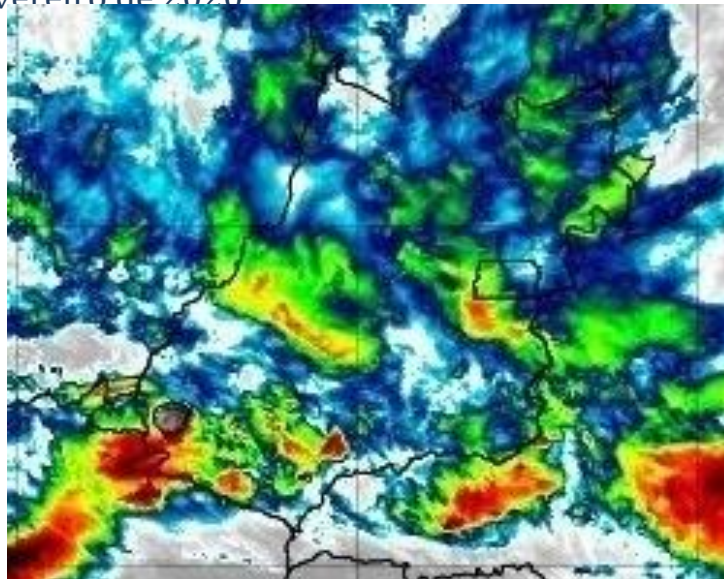
Figura 15 – Imagens realçadas do satélite GOES-16 das 0h00 do dia 13 de Fevereiro de 2020. FONTE: Cptec/INPE.
