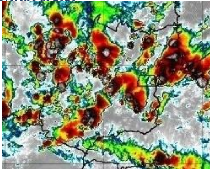
Figura 12 – Imagens realçadas do satélite GOES-16 das 15h00 do dia 12 de Fevereiro de 2020. FONTE: Cptec/INPE.
