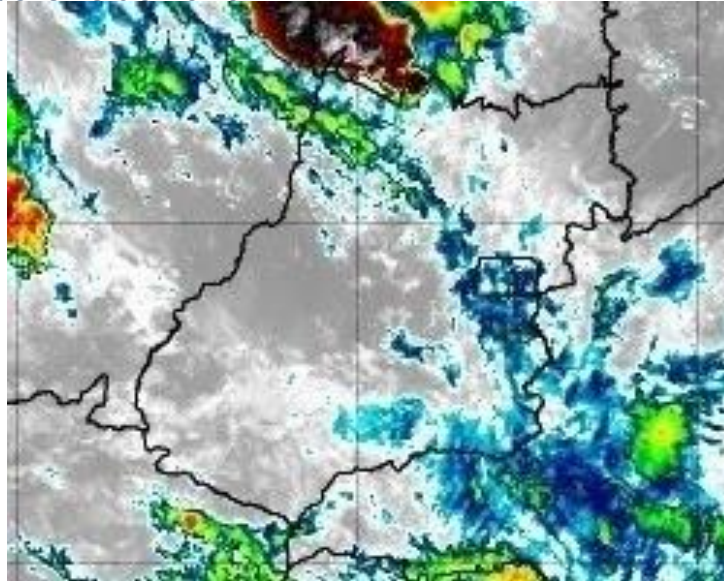
Figura 10 – Imagens realçadas do satélite GOES-16 das 9h00 do dia 12 de Fevereiro de 2020. FONTE: Cptec/INPE.
