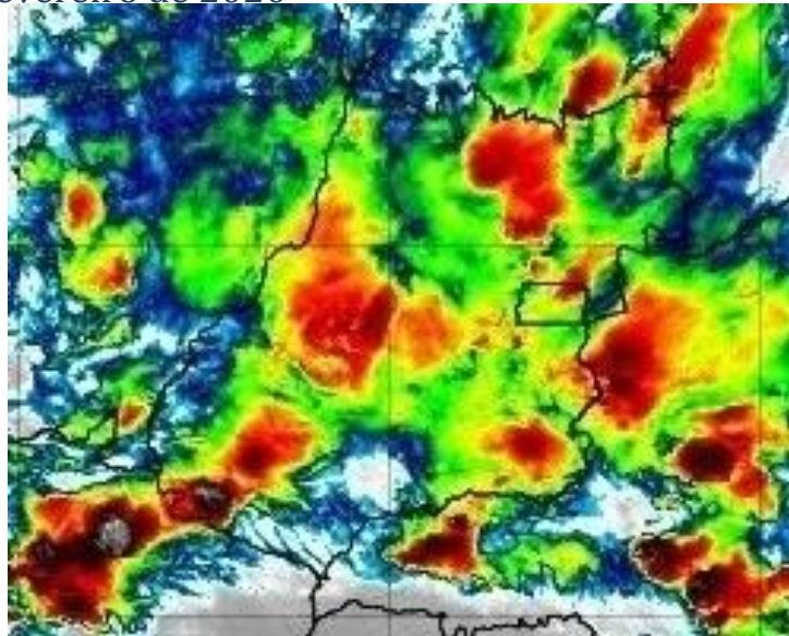
Figura 14 – Imagens realçadas do satélite GOES-16 das 21h00 do dia 12 de Fevereiro de 2020. FONTE: Cptec/INPE.
