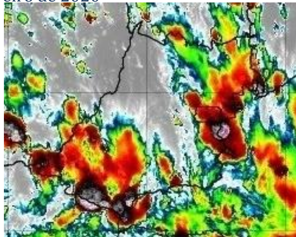
Figura 5 – Imagens realçadas do satélite GOES-16 das 18h00 do dia 11 de Fevereiro de 2020. FONTE: Cptec/INPE.
