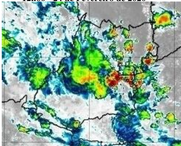
Figura 19 – Imagens realçadas do satélite GOES-16 das 12h00 do dia 24 de Fevereiro de 2020. FONTE: Cptec/INPE.
