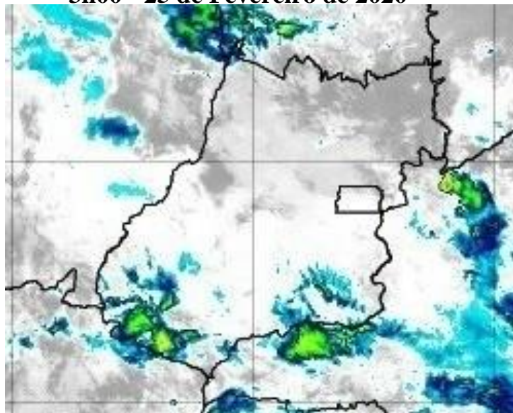
Figura 23 – Imagens realçadas do satélite GOES-16 das 3h00 do dia 25 de Fevereiro de 2020. FONTE: Cptec/INPE.
