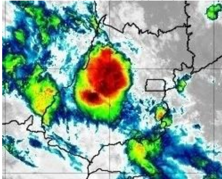
Figura 18 – Imagens realçadas do satélite GOES-16 das 9h00 do dia 24 de Fevereiro de 2020. FONTE: Cptec/INPE.
