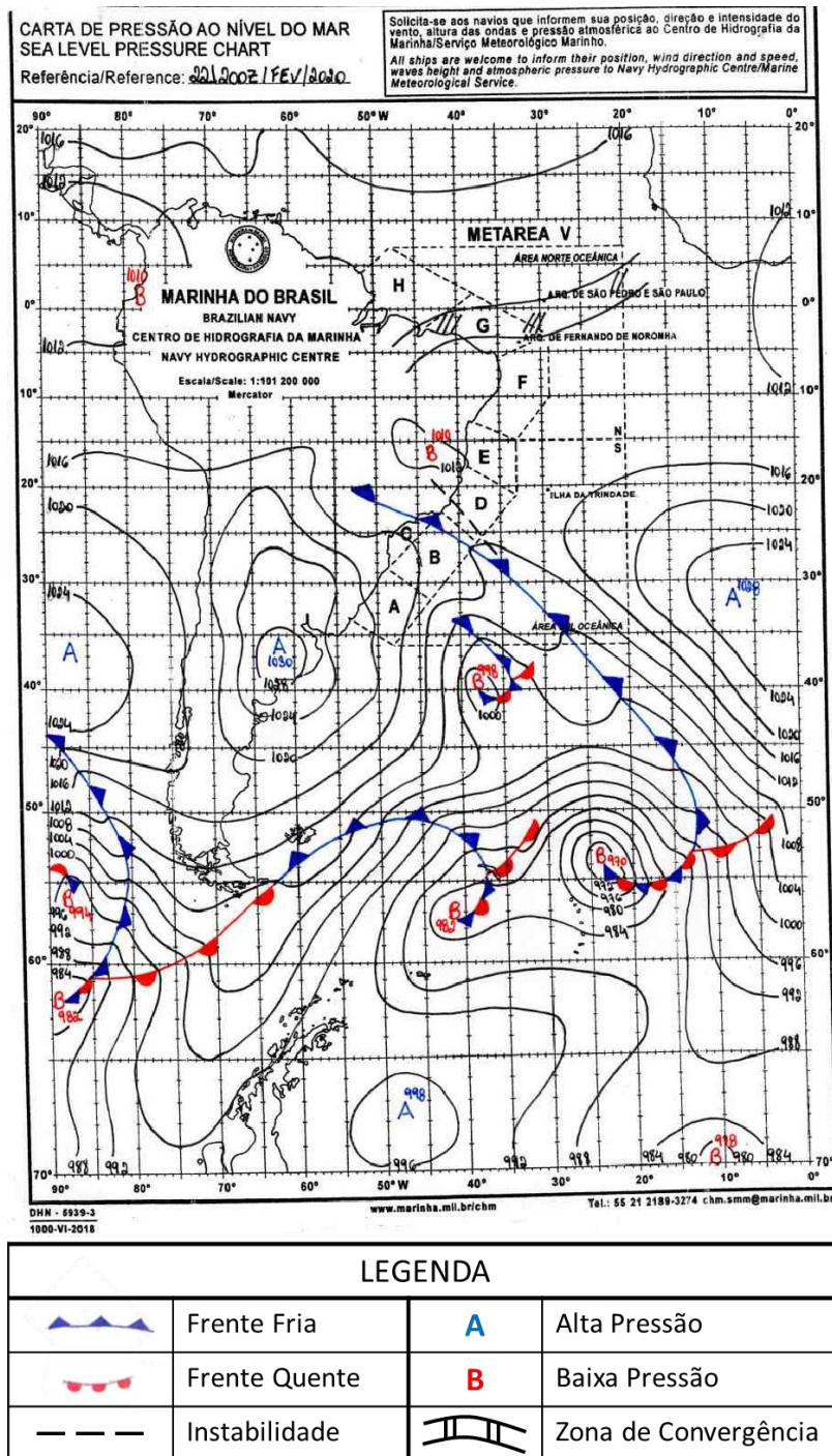
Figura A1 - Carta sinótica para as 1200Z do dia 22 de fevereiro de 2020 (0900 do dia 22 de fevereiro de 2020 hora local). FONTE: Marinha do Brasil).
