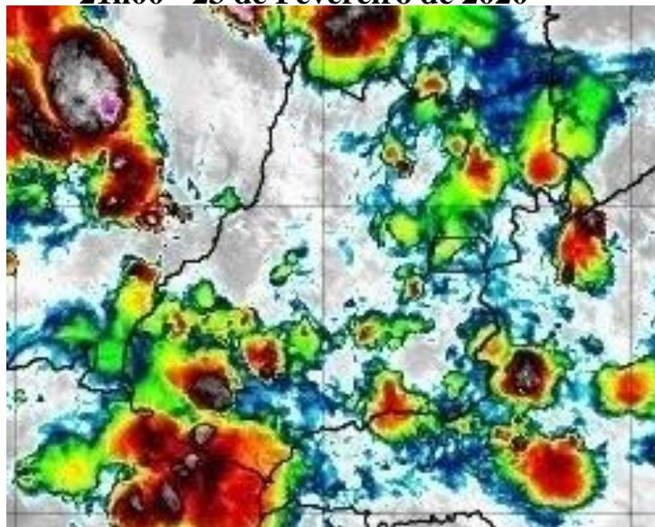
Figura 15 – Imagens realçadas do satélite GOES-16 das 21h00 do dia 23 de Fevereiro de 2020. FONTE: Cptec/INPE.
