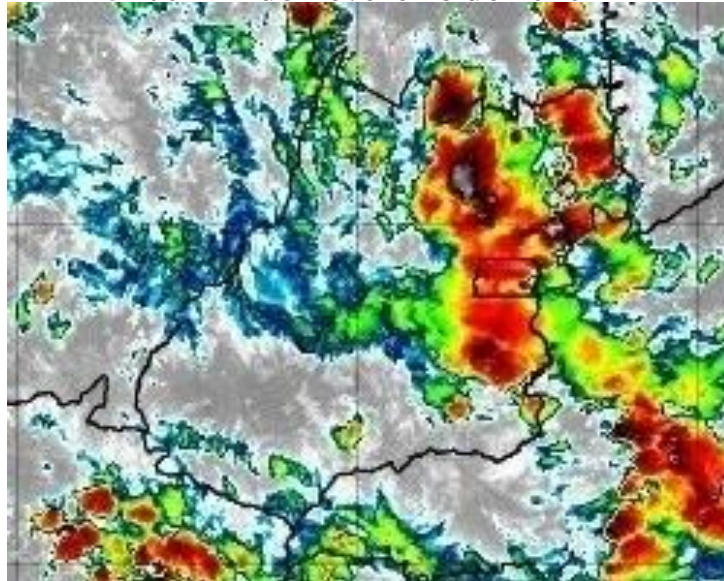
Figura 20 – Imagens realçadas do satélite GOES-16 das 15h00 do dia 24 de Fevereiro de 2020. FONTE: Cptec/INPE.
