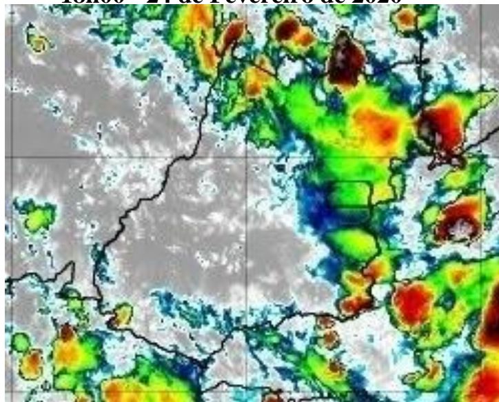
Figura 21 – Imagens realçadas do satélite GOES-16 das 18h00 do dia 24 de Fevereiro de 2020. FONTE: Cptec/INPE.
