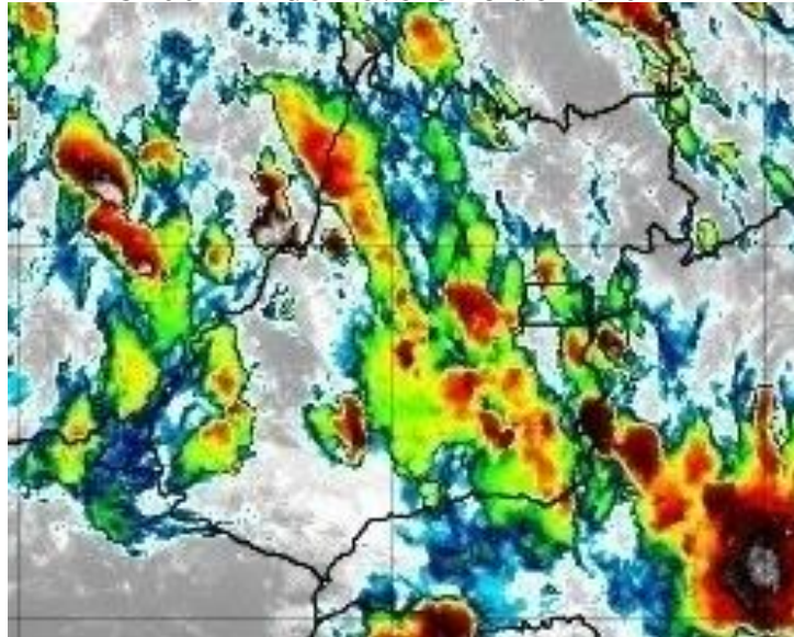
Figura 6 – Imagens realçadas do satélite GOES-16 das 18h00 do dia 22 de Fevereiro de 2020. FONTE: Cptec/INPE.
