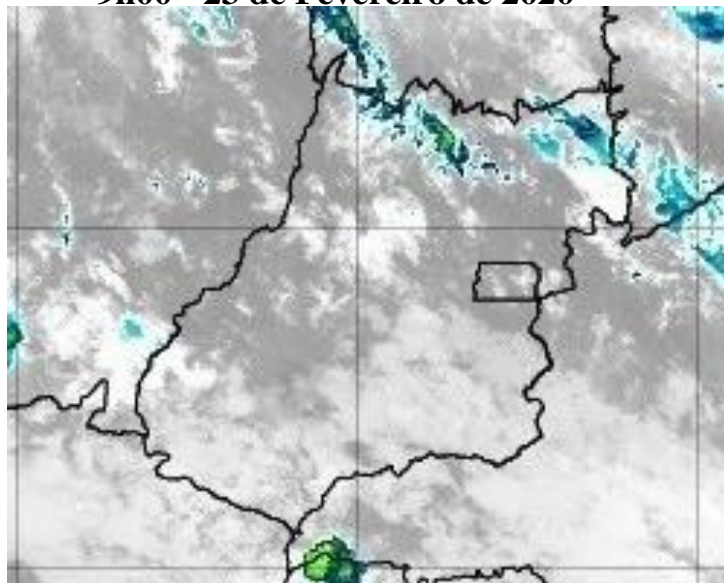
Figura 11 – Imagens realçadas do satélite GOES-16 das 9h00 do dia 23 de Fevereiro de 2020. FONTE: Cptec/INPE.
