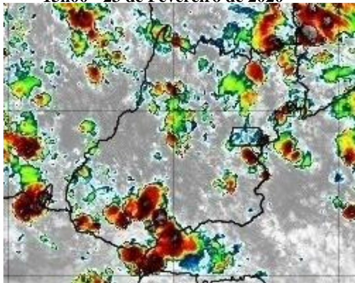
Figura 13 – Imagens realçadas do satélite GOES-16 das 15h00 do dia 23 de Fevereiro de 2020. FONTE: Cptec/INPE.
