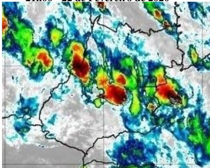
Figura 7 – Imagens realçadas do satélite GOES-16 das 21h00 do dia 22 de Fevereiro de 2020. FONTE: Cptec/INPE.
