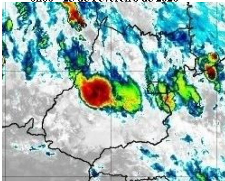
Figura 8 – Imagens realçadas do satélite GOES-16 das 0h00 do dia 23 de Fevereiro de 2020. FONTE: Cptec/INPE.
