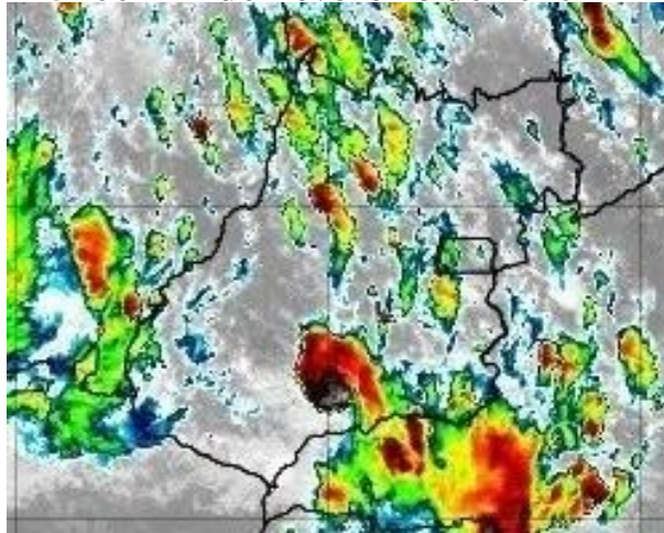
Figura 5 – Imagens realçadas do satélite GOES-16 das 15h00 do dia 22 de Fevereiro de 2020. FONTE: Cptec/INPE.
