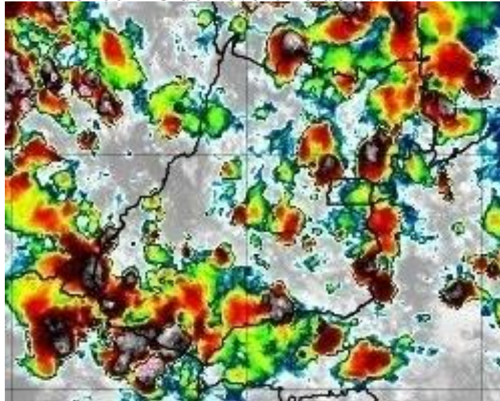
Figura 14 – Imagens realçadas do satélite GOES-16 das 18h00 do dia 23 de Fevereiro de 2020. FONTE: Cptec/INPE.
