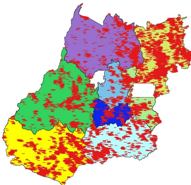
Figura 3 – Descargas atmosféricas nuvem-nuvem (em vermelho) detectadas pelo sistema Earth Networks entre 09h40 do dia 22 e 23h40 do dia 24 de fevereiro de 2020 sobre a área de concessão da CELG Distribuição.
