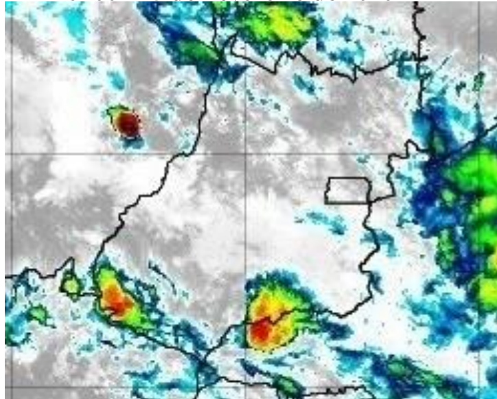
Figura 22 – Imagens realçadas do satélite GOES-16 das 0h00 do dia 25 de Fevereiro de 2020. FONTE: Cptec/INPE.
