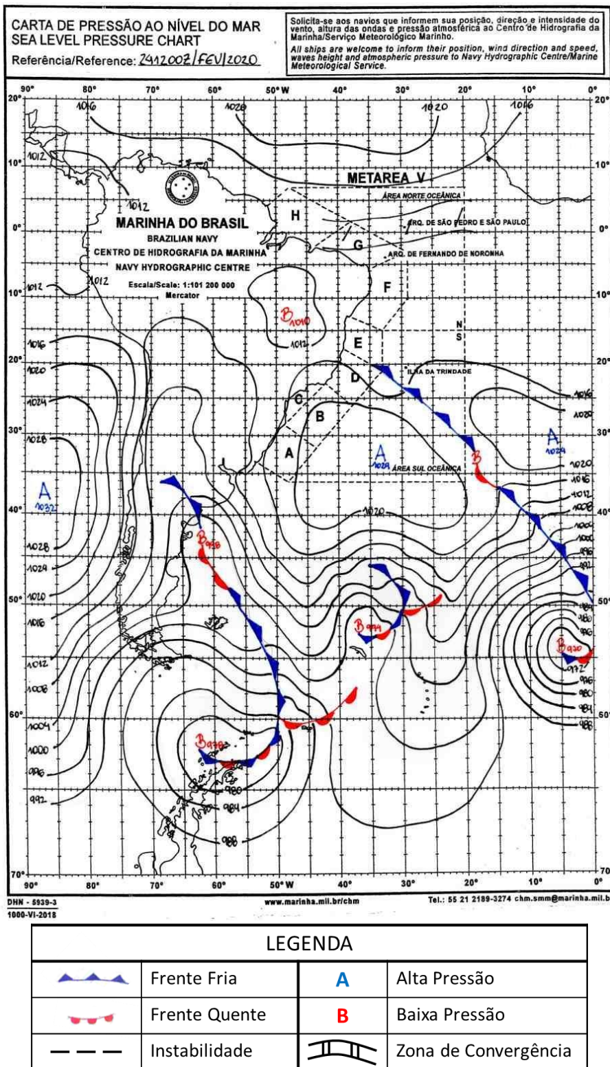
Figura A3 - Carta sinótica para as 1200Z do dia 24 de fevereiro de 2020 (09h00 do dia 24 de fevereiro de 2020 hora local). FONTE: Marinha do Brasil).
