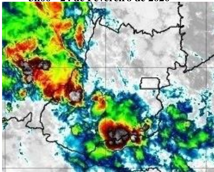
Figura 17 – Imagens realçadas do satélite GOES-16 das 3h00 do dia 24 de Fevereiro de 2020. FONTE: Cptec/INPE.
