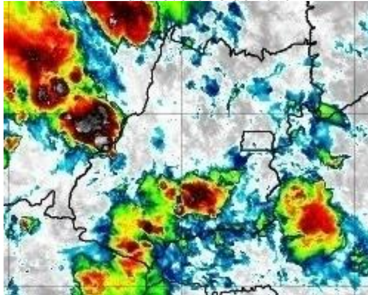
Figura 16 – Imagens realçadas do satélite GOES-16 das 0h00 do dia 24 de Fevereiro de 2020. FONTE: Cptec/INPE.
