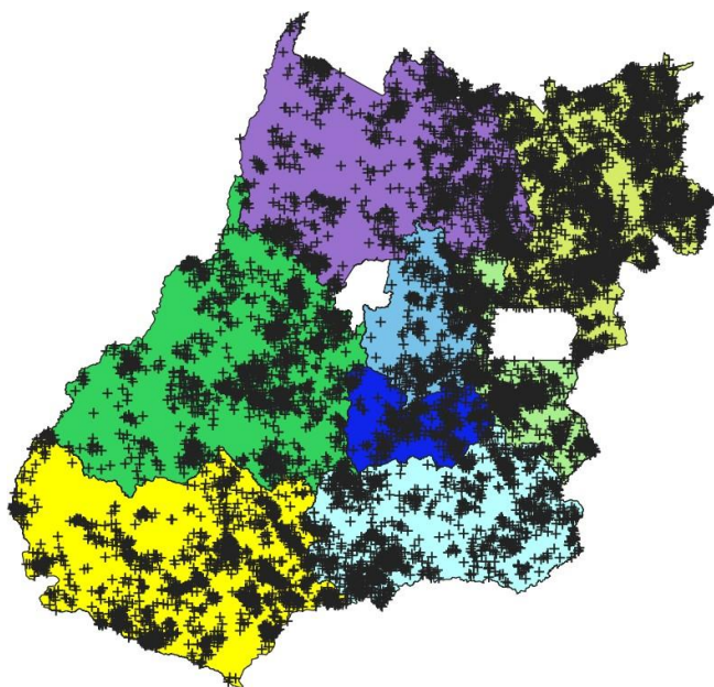
Figura 2 – Descargas atmosféricas nuvem-solo (em preto) detectadas pelo sistema Earth Networks entre 09h40 do dia 22 e 23h40 do dia 24 de fevereiro de 2020 sobre a área de concessão da CELG Distribuição.
