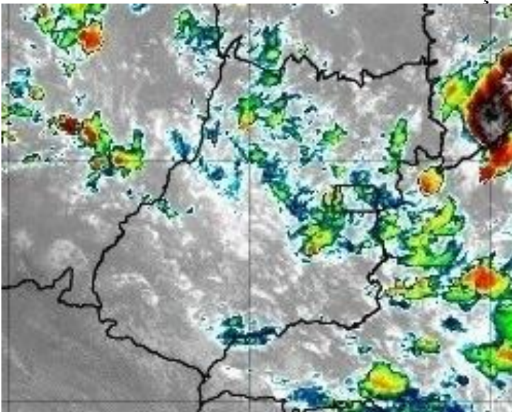
Figura 16 – Imagens realçadas do satélite GOES-16 das 15h00 do dia 01 de Março de 2020. FONTE: Cptec/INPE.
