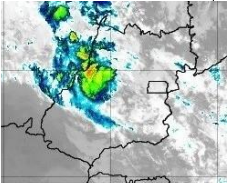
Figura 15 – Imagens realçadas do satélite GOES-16 das 9h00 do dia 01 de Março de 2020. FONTE: Cptec/INPE.
