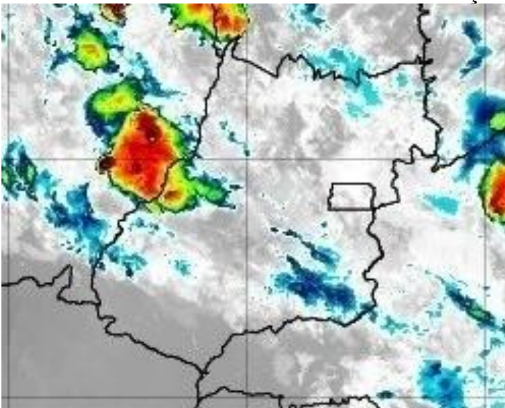
Figura 14 – Imagens realçadas do satélite GOES-16 das 3h00 do dia 01 de Março de 2020. FONTE: Cptec/INPE.
