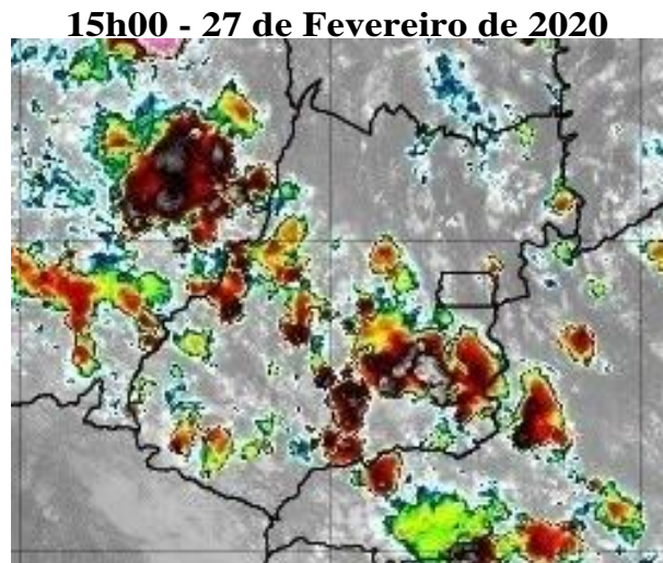
Figura 5 – Imagens realçadas do satélite GOES-16 das 15h00 do dia 27 de Fevereiro de 2020. FONTE: Cptec/INPE.
