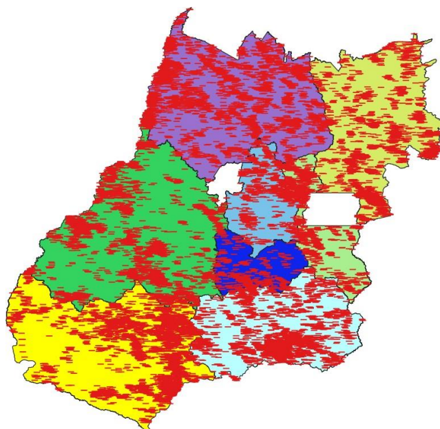
Figura 3 – Descargas atmosféricas nuvem-nuvem (em vermelho) detectadas pelo sistema Earth Networks entre 11h30 do dia 27 de fevereiro e 21h00 do dia 09 de março de 2020 sobre a área de concessão da CELG Distribuição.
