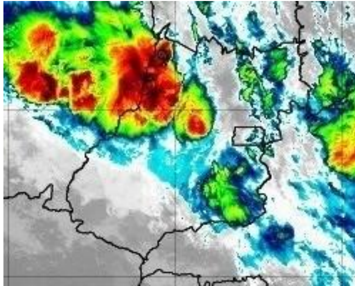
Figura 11 – Imagens realçadas do satélite GOES-16 das 9h00 do dia 29 de Fevereiro de 2020. FONTE: Cptec/INPE.
