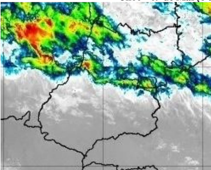
Figura 44 – Imagens realçadas do satélite GOES-16 das 3h00 do dia 09 de Março de 2020. FONTE: Cptec/INPE.
