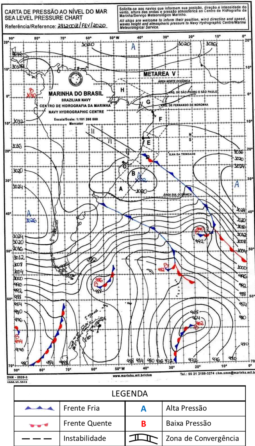
Figura A2 - Carta sinótica para as 1200Z do dia 28 de fevereiro de 2020 (09h00 do dia 28 de fevereiro de 2020 hora local. FONTE: Marinha do Brasil).
