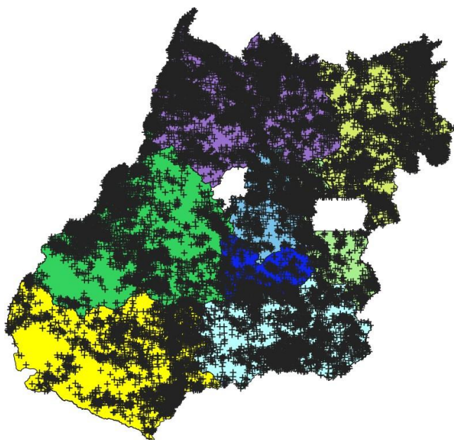
Figura 2 – Descargas atmosféricas nuvem-solo (em preto) detectadas pelo sistema Earth Networks entre 11h30 do dia 27 de fevereiro e 21h00 do dia 09 de março de 2020 sobre a área de concessão da CELG Distribuição.
