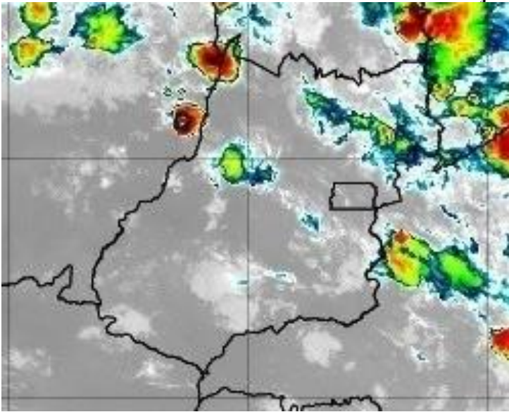
Figura 25 – Imagens realçadas do satélite GOES-16 das 21h00 do dia 03 de Março de 2020. FONTE: Cptec/INPE.
