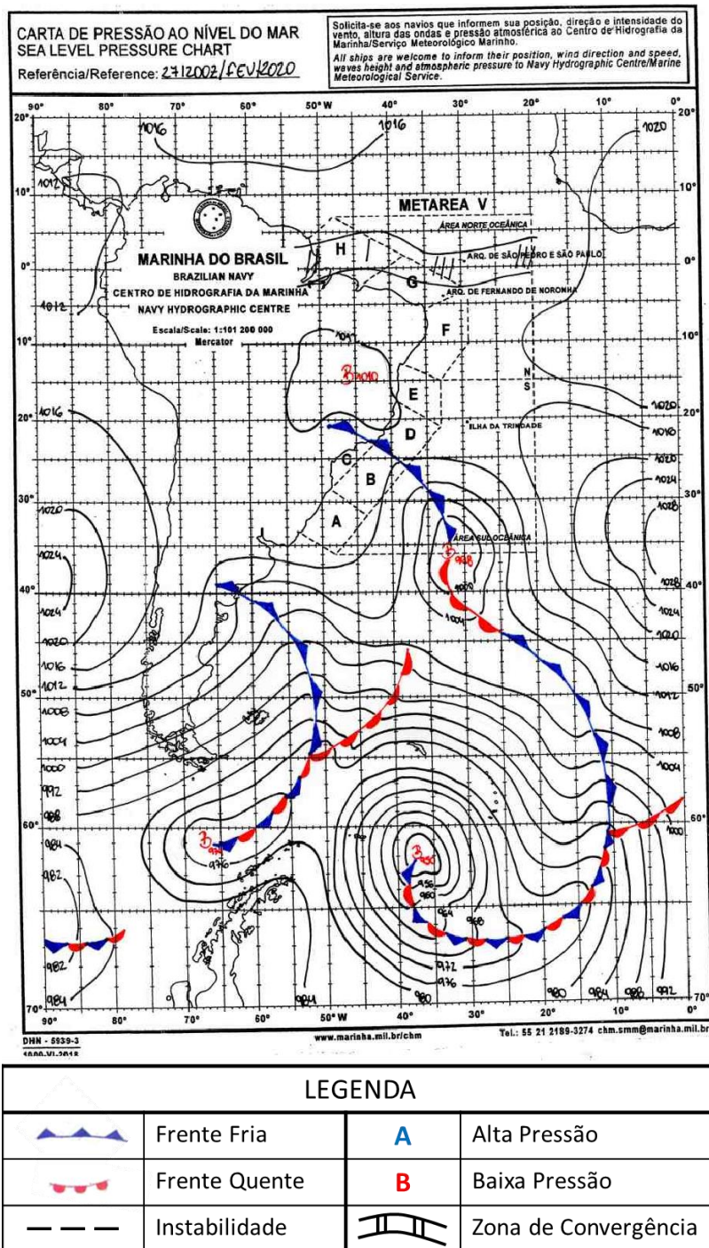
Figura A1 - Carta sinótica para as 1200Z do dia 27 de fevereiro de 2020 (0900 do dia 27 de fevereiro de 2020 hora local. FONTE: Marinha do Brasil).
