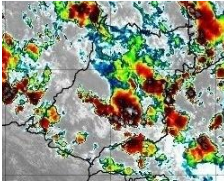
Figura 9 – Imagens realçadas do satélite GOES-16 das 15h00 do dia 28 de Fevereiro de 2020. FONTE: Cptec/INPE.
