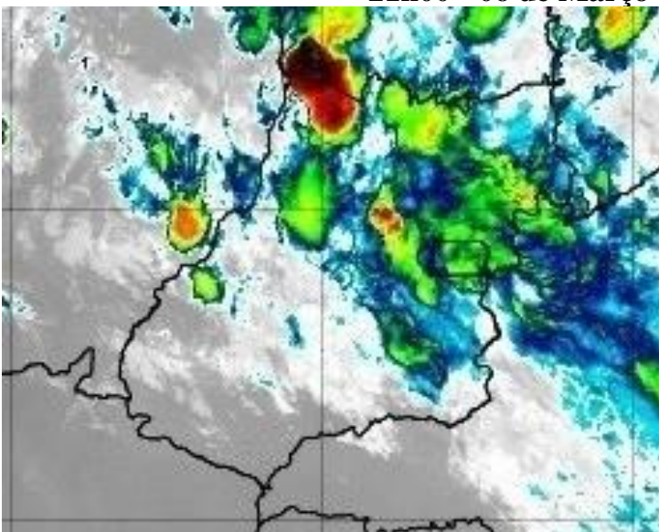
Figura 36 – Imagens realçadas do satélite GOES-16 das 21h00 do dia 06 de Março de 2020. FONTE: Cptec/INPE.
