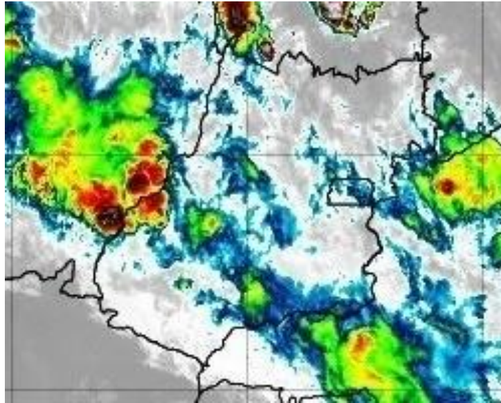
Figura 7 – Imagens realçadas do satélite GOES-16 das 3h00 do dia 28 de Fevereiro de 2020. FONTE: Cptec/INPE.
