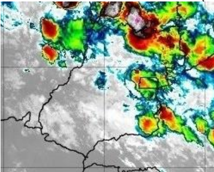
Figura 32 – Imagens realçadas do satélite GOES-16 das 21h00 do dia 05 de Março de 2020. FONTE: Cptec/INPE.
