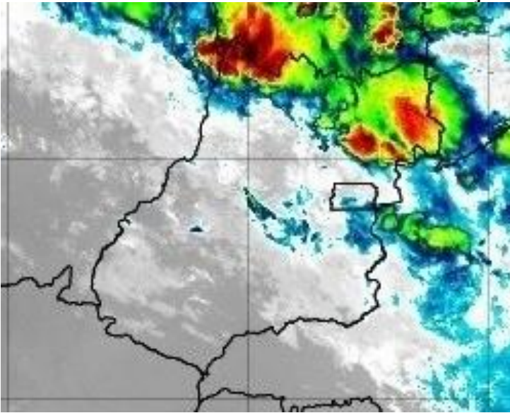
Figura 33 – Imagens realçadas do satélite GOES-16 das 3h00 do dia 06 de Março de 2020. FONTE: Cptec/INPE.
