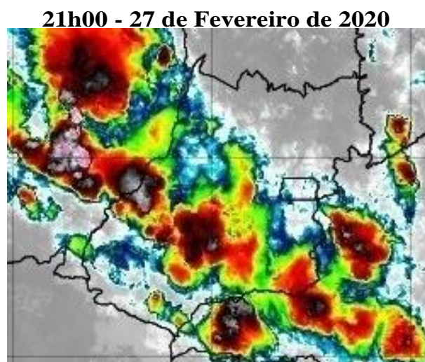
Figura 6 – Imagens realçadas do satélite GOES-16 das 21h00 do dia 27 de Fevereiro de 2020. FONTE: Cptec/INPE.
