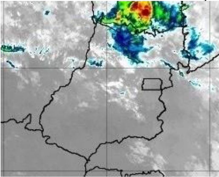
Figura 27 – Imagens realçadas do satélite GOES-16 das 9h00 do dia 04 de Março de 2020. FONTE: Cptec/INPE.
