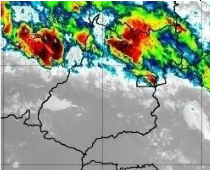
Figura 43 – Imagens realçadas do satélite GOES-16 das 21h00 do dia 08 de Março de 2020. FONTE: Cptec/INPE.
