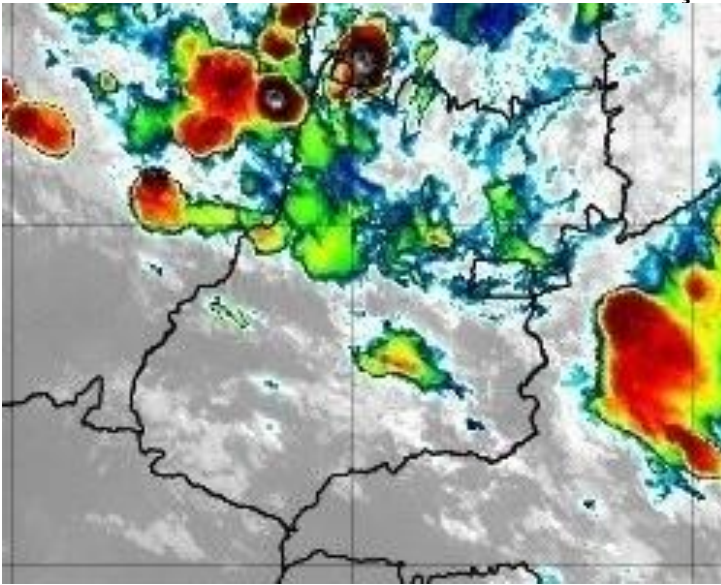
Figura 29 – Imagens realçadas do satélite GOES-16 das 21h00 do dia 04 de Março de 2020. FONTE: Cptec/INPE.
