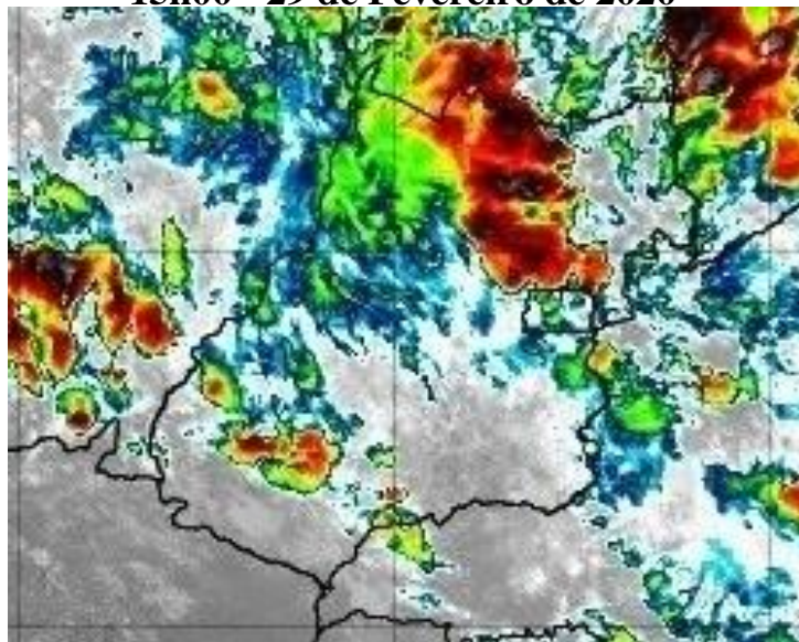
Figura 12 – Imagens realçadas do satélite GOES-16 das 15h00 do dia 29 de Fevereiro de 2020. FONTE: Cptec/INPE.
