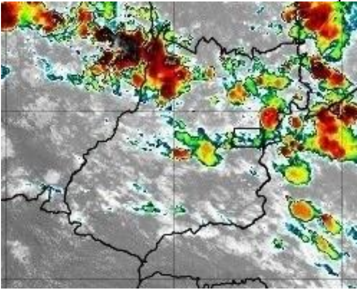
Figura 31 – Imagens realçadas do satélite GOES-16 das 15h00 do dia 05 de Março de 2020. FONTE: Cptec/INPE.
