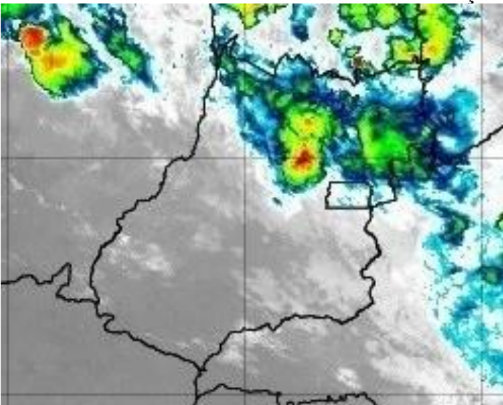
Figura 34 – Imagens realçadas do satélite GOES-16 das 9h00 do dia 06 de Março de 2020. FONTE: Cptec/INPE.
