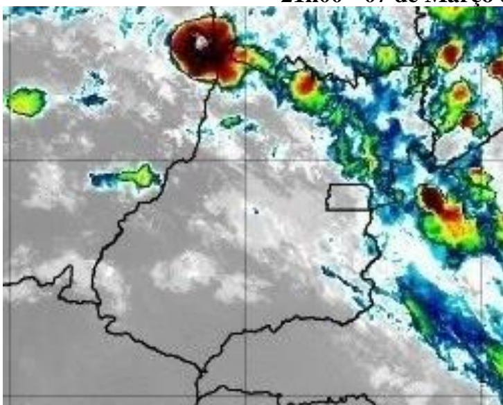
Figura 40 – Imagens realçadas do satélite GOES-16 das 21h00 do dia 07 de Março de 2020. FONTE: Cptec/INPE.
