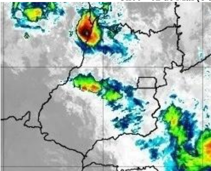
Figura 18 – Imagens realçadas do satélite GOES-16 das 3h00 do dia 02 de Março de 2020. FONTE: Cptec/INPE.
