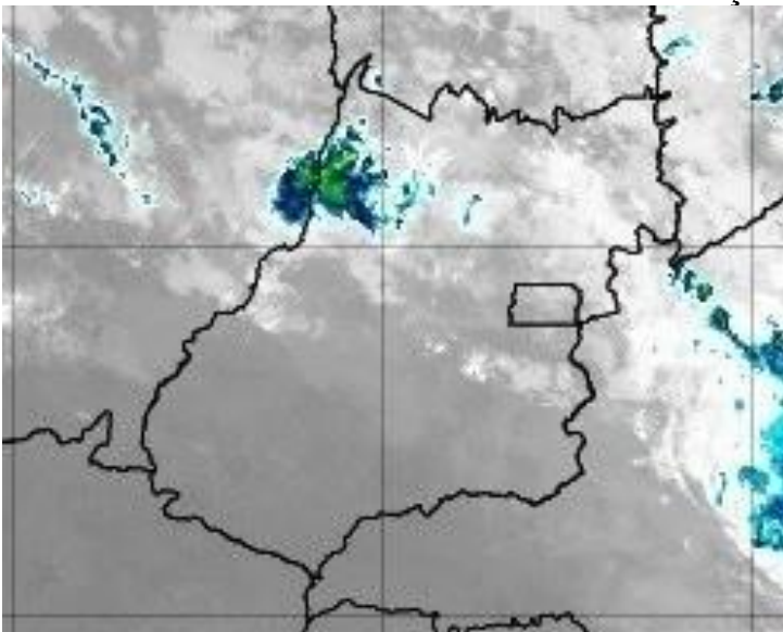
Figura 38 – Imagens realçadas do satélite GOES-16 das 9h00 do dia 07 de Março de 2020. FONTE: Cptec/INPE.
