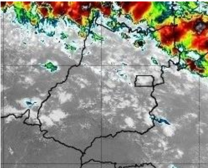
Figura 42 – Imagens realçadas do satélite GOES-16 das 15h00 do dia 08 de Março de 2020. FONTE: Cptec/INPE.
