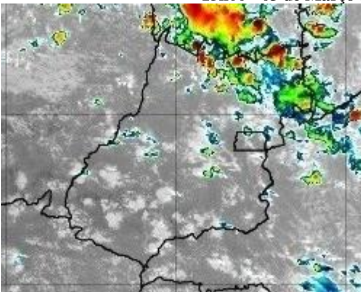
Figura 24 – Imagens realçadas do satélite GOES-16 das 15h00 do dia 03 de Março de 2020. FONTE: Cptec/INPE.
