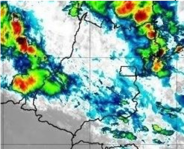
Figura 13 – Imagens realçadas do satélite GOES-16 das 21h00 do dia 00 de Março de 2020. FONTE: Cptec/INPE.
