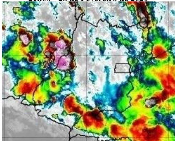
Figura 10 – Imagens realçadas do satélite GOES-16 das 21h00 do dia 28 de Fevereiro de 2020. FONTE: Cptec/INPE.
