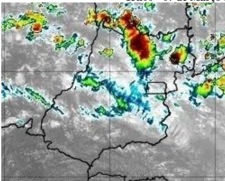
Figura 39 – Imagens realçadas do satélite GOES-16 das 15h00 do dia 07 de Março de 2020. FONTE: Cptec/INPE.
