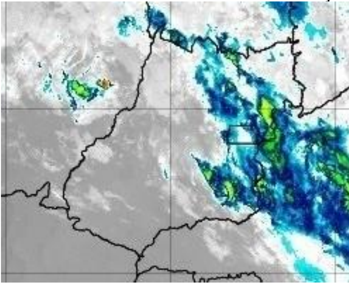
Figura 37 – Imagens realçadas do satélite GOES-16 das 3h00 do dia 07 de Março de 2020. FONTE: Cptec/INPE.
