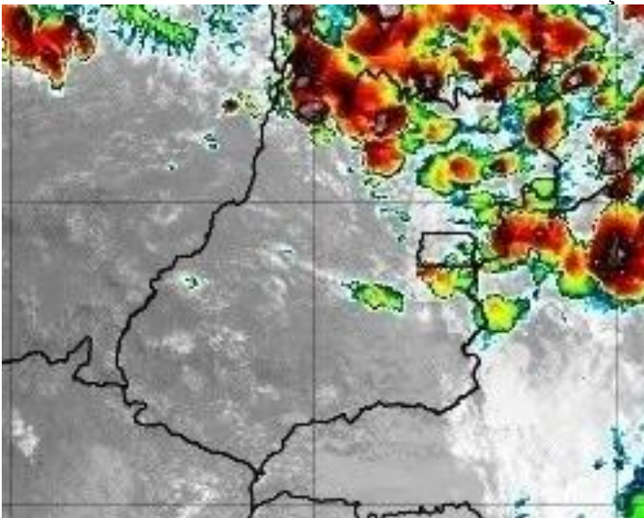
Figura 20 – Imagens realçadas do satélite GOES-16 das 15h00 do dia 02 de Março de 2020. FONTE: Cptec/INPE.
