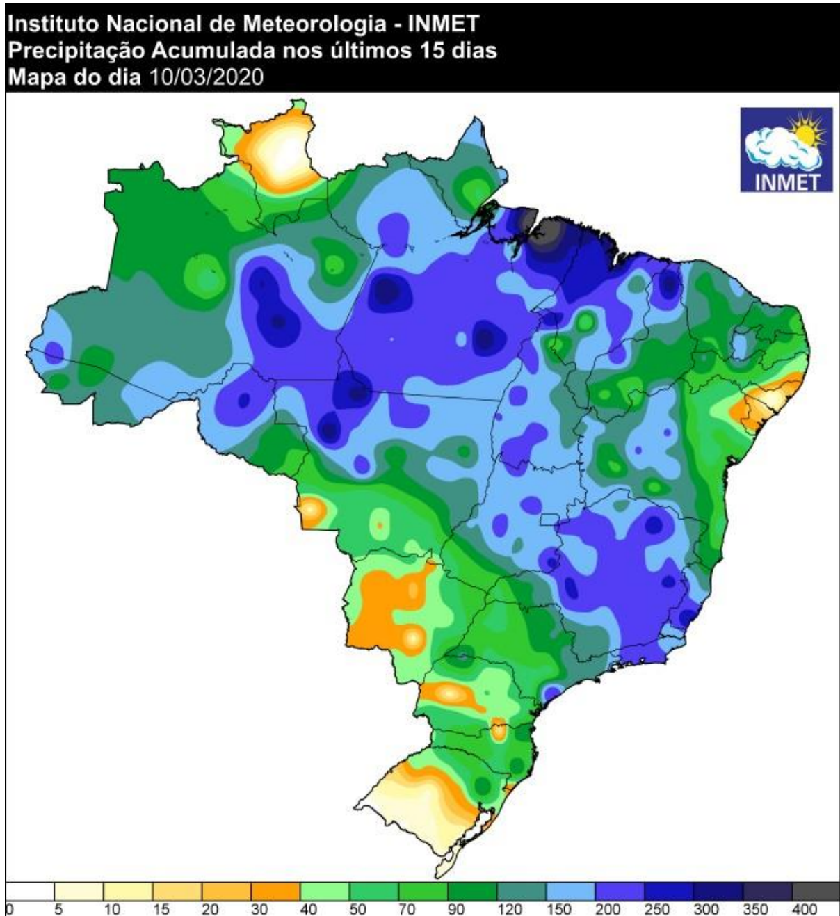
Figura 4 – Mapa de precipitação acumulada entre as 09h do dia 25 de fevereiro e 09h do dia 10 de março de 2020. FONTE: Cptec/INPE.
