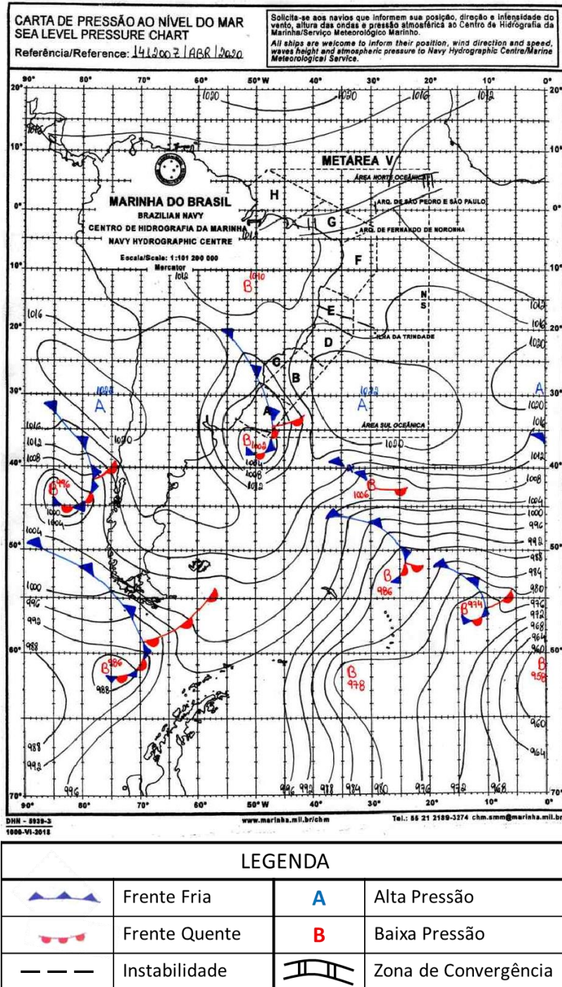
Figura A1 - Carta sinótica para as 1200Z do dia 14 de abril de 2020 (09h00 do dia 14 de abril de 2020 hora local. FONTE: Marinha do Brasil).
