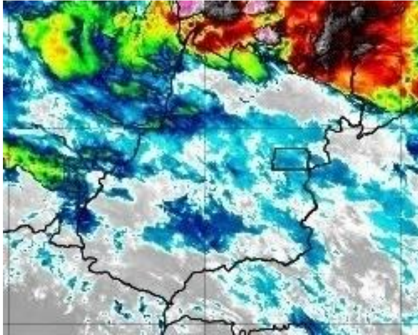
Figura 10 – Imagens realçadas do satélite GOES-16 das 0h00 do dia 15 de Abril de 2020. FONTE: Cptec/INPE.
