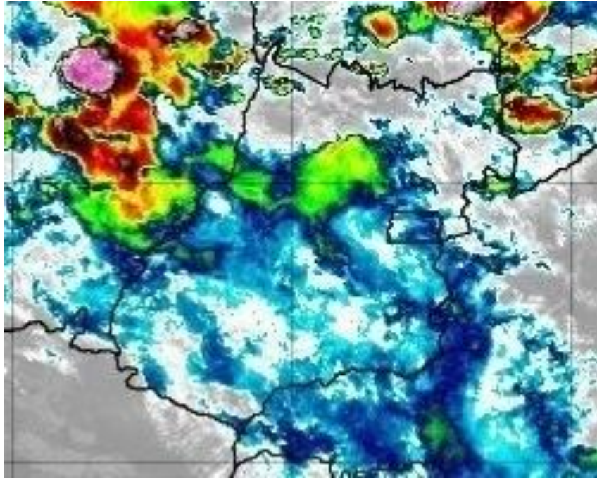
Figura 8 – Imagens realçadas do satélite GOES-16 das 18h00 do dia 14 de Abril de 2020. FONTE: Cptec/INPE.
