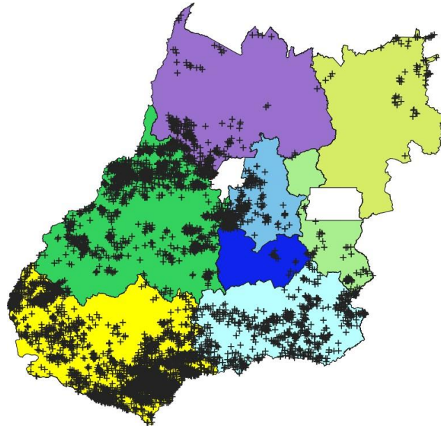
Figura 2 – Descargas atmosféricas nuvem-solo (em preto) detectadas pelo sistema Earth Networks entre 03h20 e 23h00 do dia 14 de abril de 2020 sobre a área de concessão da CELG Distribuição.
