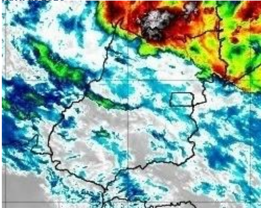
Figura 11 – Imagens realçadas do satélite GOES-16 das 3h00 do dia 15 de Abril de 2020. FONTE: Cptec/INPE.
