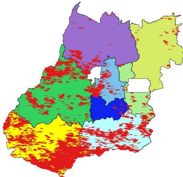
Figura 3 – Descargas atmosféricas nuvem-nuvem (em vermelho) detectadas pelo sistema Earth Networks entre 03h20 e 23h00 do dia 14 de abril de 2020 sobre a área de concessão da CELG Distribuição.
