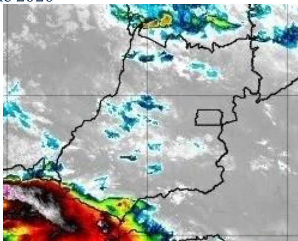
Figura 4 – Imagens realçadas do satélite GOES-16 das 06h00 do dia 14 de Abril de 2020. FONTE: Cptec/INPE.
