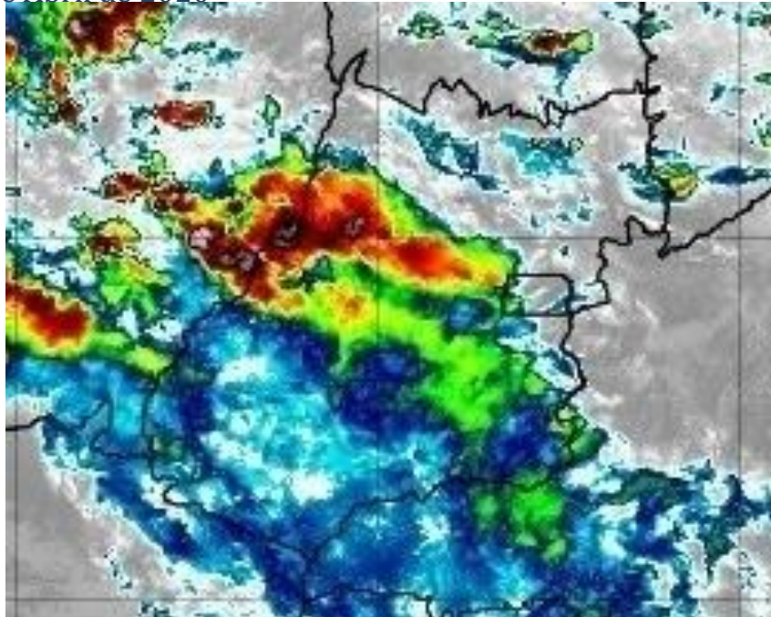
Figura 7 – Imagens realçadas do satélite GOES-16 das 15h00 do dia 14 de Abril de 2020. FONTE: Cptec/INPE.
