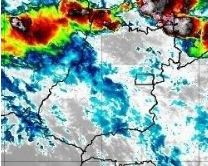
Figura 9 – Imagens realçadas do satélite GOES-16 das 21h00 do dia 14 de Abril de 2020. FONTE: Cptec/INPE.
