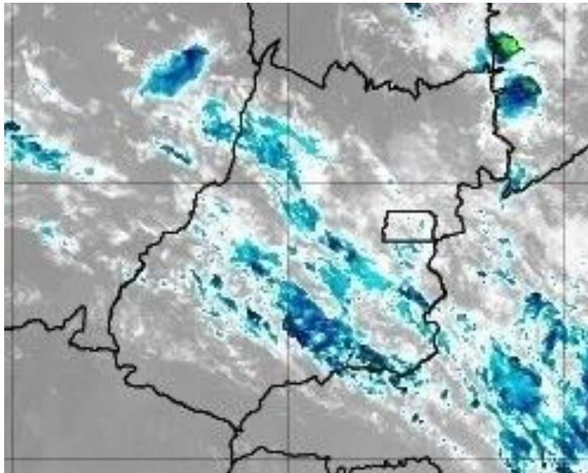
Figura 28 – Imagens realçadas do satélite GOES-16 das 23h00 do dia 23 de Setembro de 2020. FONTE: Cptec/INPE.
