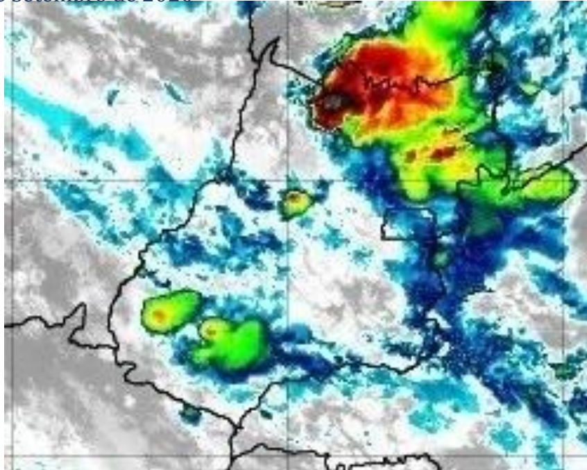
Figura 9 – Imagens realçadas do satélite GOES-16 das 21h00 do dia 21 de Setembro de 2020. FONTE: Cptec/INPE.
