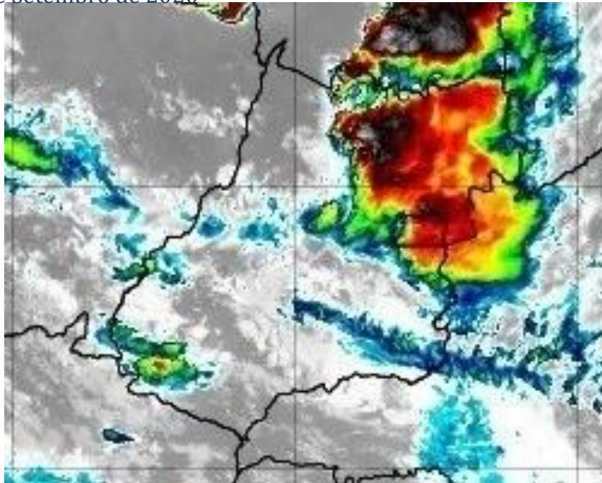
Figura 7 – Imagens realçadas do satélite GOES-16 das 17h00 do dia 21 de Setembro de 2020. FONTE: Cptec/INPE.
