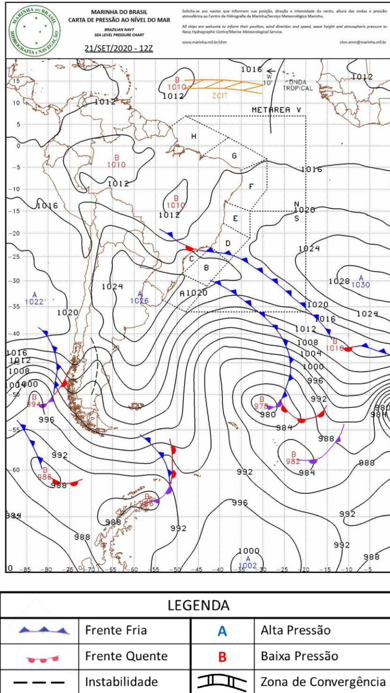
Figura A1 - Carta sinótica da Marinha do Brasil para as 1200Z do dia 21 de setembro de 2020 (09h00 do dia 21 de setembro de 2020, hora local).
