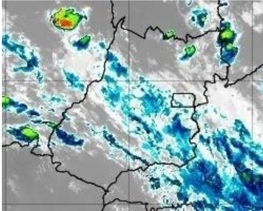
Figura 26 – Imagens realçadas do satélite GOES-16 das 19h00 do dia 23 de Setembro de 2020. FONTE: Cptec/INPE.
