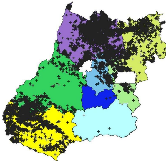
Figura 2 – Descargas atmosféricas nuvem-solo (em preto) detectadas pelo sistema Earth Networks entre 09h00 do dia 21 e 21h30 do dia 23 de setembro de 2020 sobre a área de concessão da ENEL DISTRIBUIÇÃO GOIÁS.
