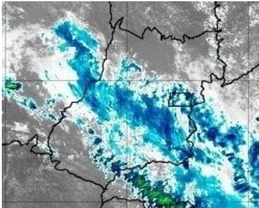
Figura 24 – Imagens realçadas do satélite GOES-16 das 15h00 do dia 23 de Setembro de 2020. FONTE: Cptec/INPE.
