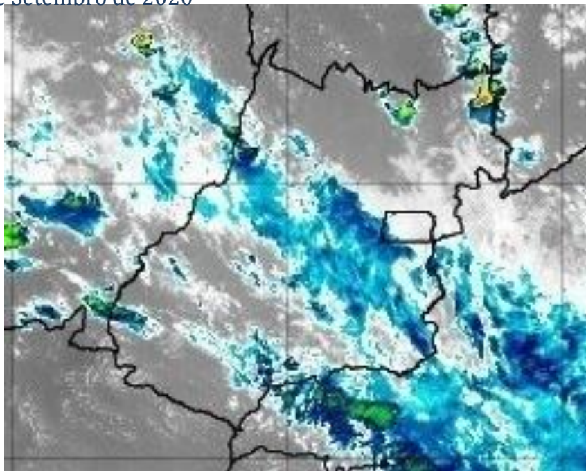
Figura 25 – Imagens realçadas do satélite GOES-16 das 17h00 do dia 23 de Setembro de 2020. FONTE: Cptec/INPE.
