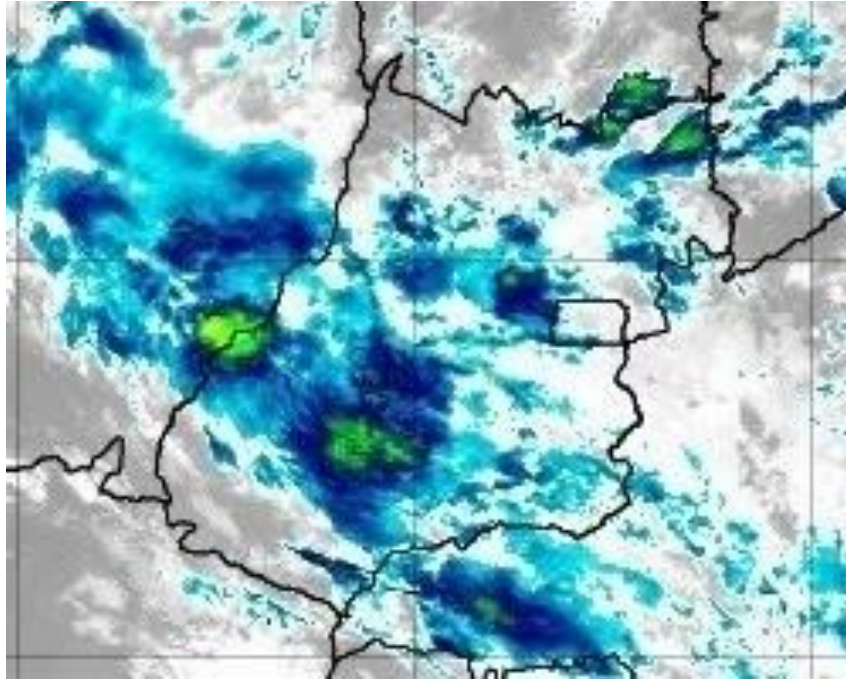
Figura 20 – Imagens realçadas do satélite GOES-16 das 1h00 do dia 23 de Setembro de 2020. FONTE: Cptec/INPE.
