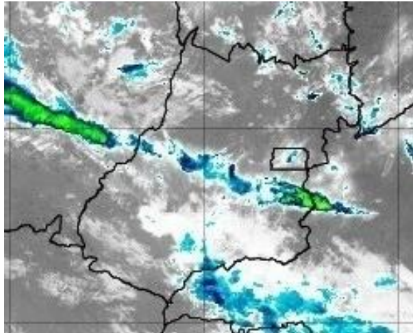
Figura 4 – Imagens realçadas do satélite GOES-16 das 11h00 do dia 21 de Setembro de 2020. FONTE: Cptec/INPE.
