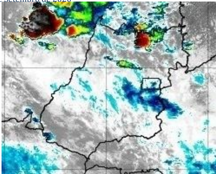
Figura 15 – Imagens realçadas do satélite GOES-16 das 15h00 do dia 22 de Setembro de 2020. FONTE: Cptec/INPE.
