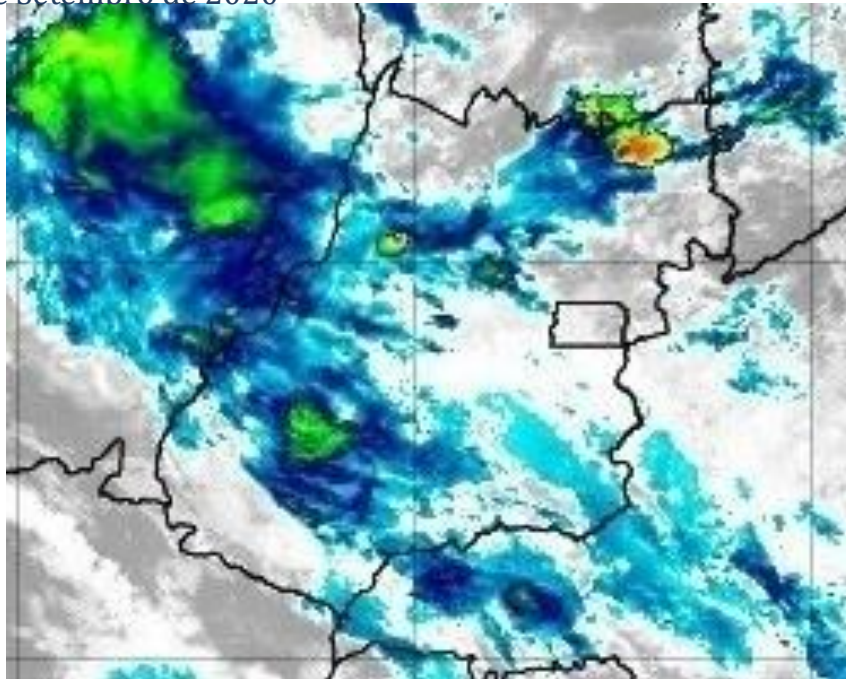
Figura 19 – Imagens realçadas do satélite GOES-16 das 23h00 do dia 22 de Setembro de 2020. FONTE: Cptec/INPE.
