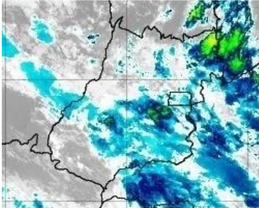
Figura 12 – Imagens realçadas do satélite GOES-16 das 3h00 do dia 22 de Setembro de 2020. FONTE: Cptec/INPE.
