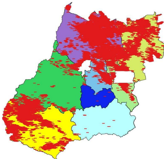
Figura 3 – Descargas atmosféricas nuvem-nuvem (em vermelho) detectadas pelo sistema Earth Networks entre 09h00 do dia 21 e 21h30 do dia 23 de setembro de 2020 sobre a área de concessão da ENEL DISTRIBUIÇÃO GOIÁS.
