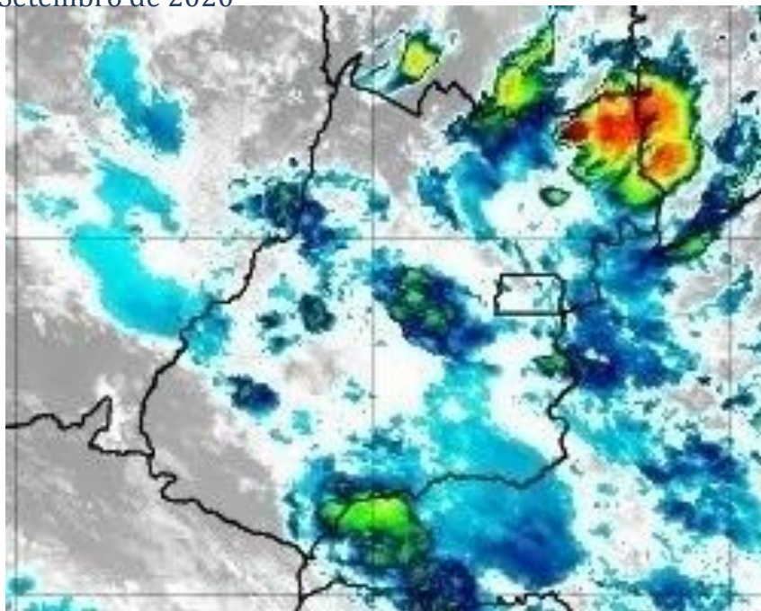
Figura 11 – Imagens realçadas do satélite GOES-16 das 1h00 do dia 22 de Setembro de 2020. FONTE: Cptec/INPE.
