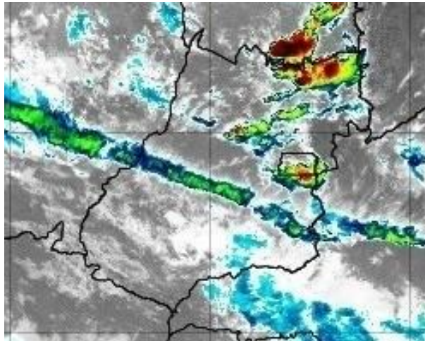
Figura 5 – Imagens realçadas do satélite GOES-16 das 13h00 do dia 21 de Setembro de 2020. FONTE: Cptec/INPE.
