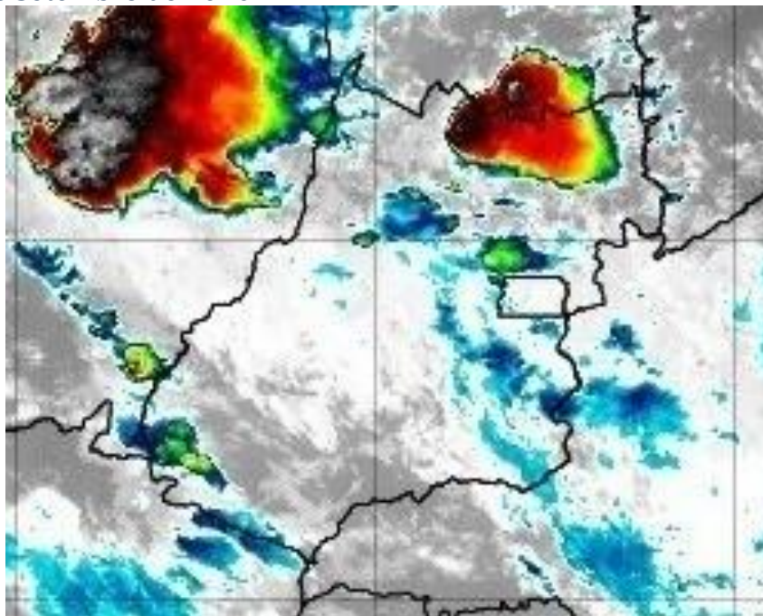
Figura 16 – Imagens realçadas do satélite GOES-16 das 17h00 do dia 22 de Setembro de 2020. FONTE: Cptec/INPE.
