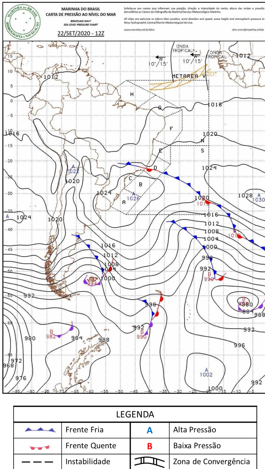
Figura A2 - Carta sinótica da Marinha do Brasil para as 1200Z do dia 22 de setembro de 2020 (09h00 do dia 22 de setembro de 2020, hora local).
