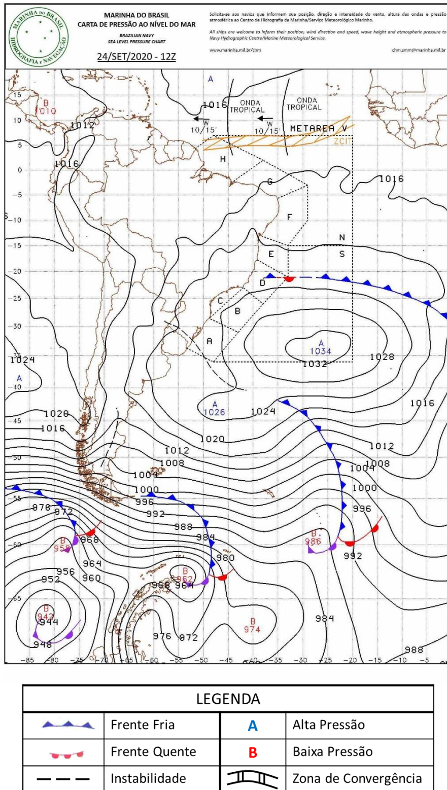
Figura A4 - Carta sinótica da Marinha do Brasil para as 1200Z do dia 23 de setembro de 2020 (09h00 do dia 23 de setembro de 2020, hora local).
