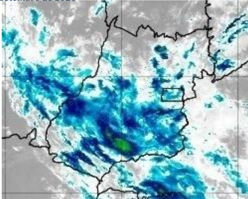
Figura 21 – Imagens realçadas do satélite GOES-16 das 3h00 do dia 23 de Setembro de 2020. FONTE: Cptec/INPE.
