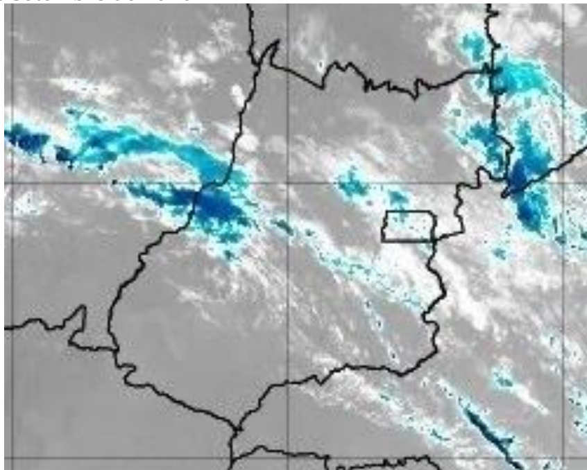
Figura 30 – Imagens realçadas do satélite GOES-16 das 03h00 do dia 24 de Setembro de 2020. FONTE: Cptec/INPE.
