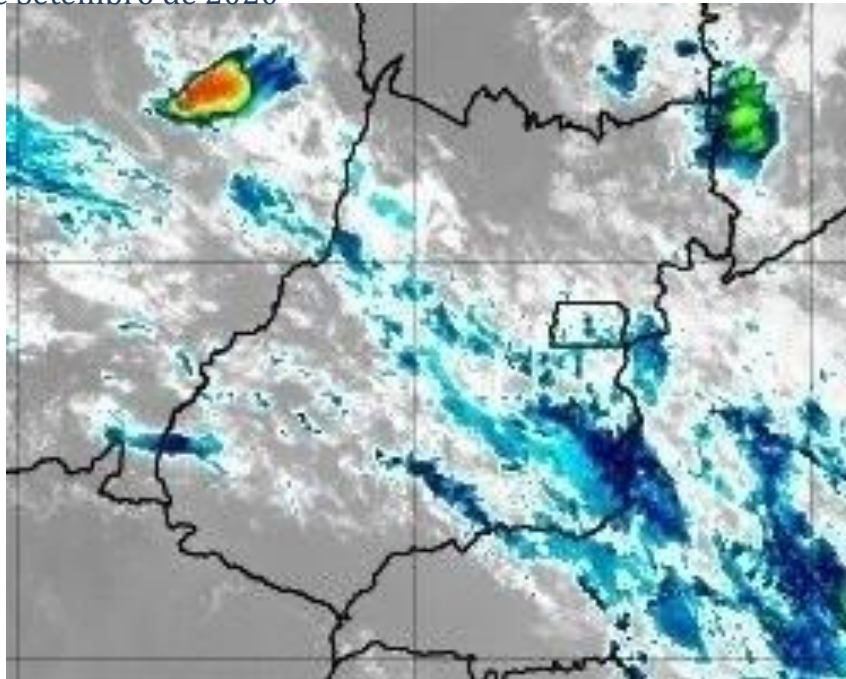
Figura 27 – Imagens realçadas do satélite GOES-16 das 21h00 do dia 23 de Setembro de 2020. FONTE: Cptec/INPE.
