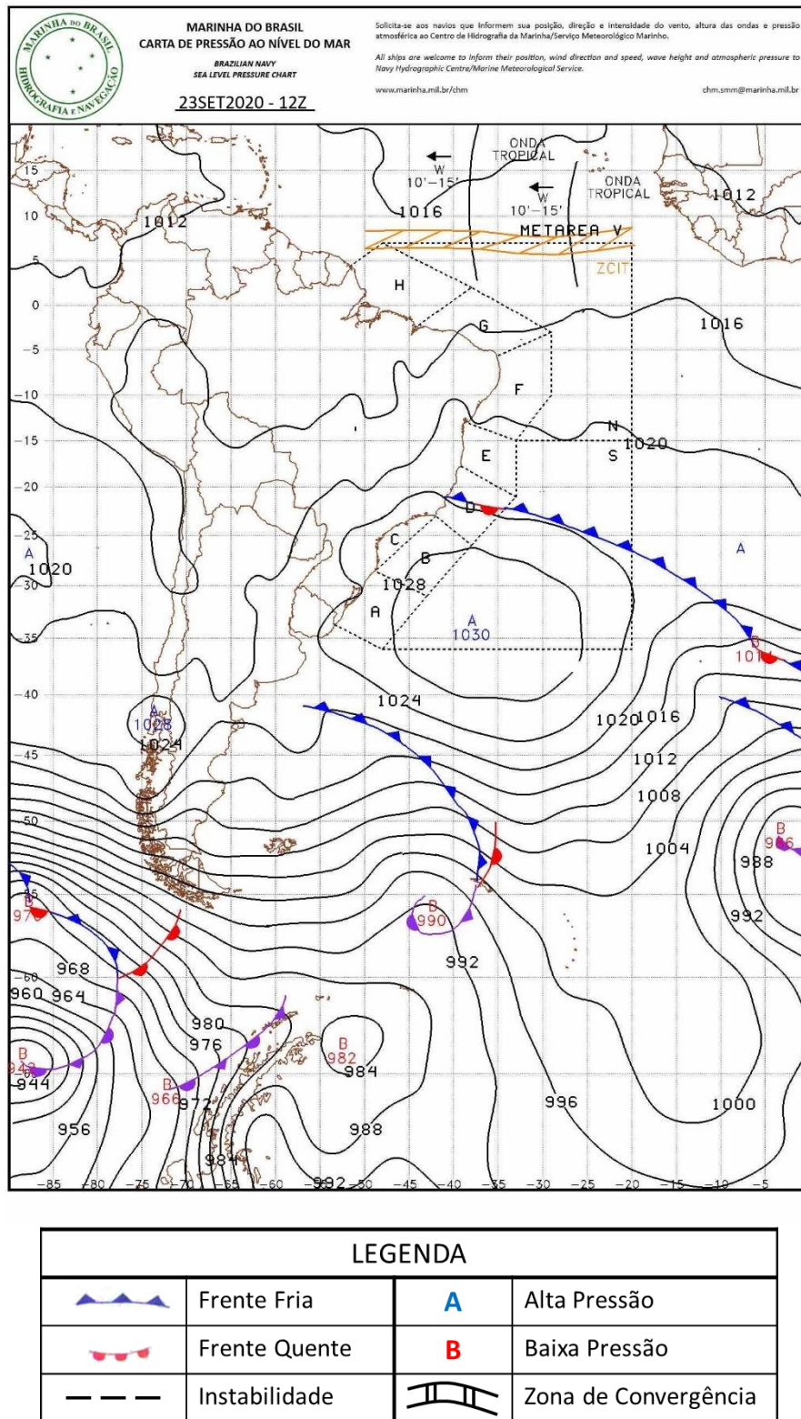
Figura A3 - Carta sinótica da Marinha do Brasil para as 1200Z do dia 23 de setembro de 2020 (09h00 do dia 23 de setembro de 2020, hora local).
