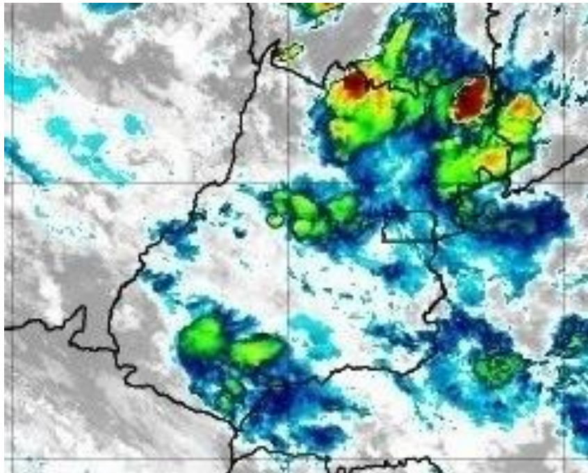
Figura 10 – Imagens realçadas do satélite GOES-16 das 23h00 do dia 21 de Setembro de 2020. FONTE: Cptec/INPE.
