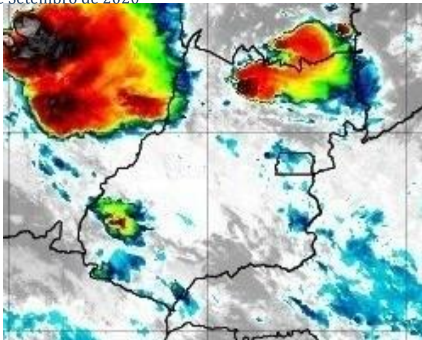
Figura 17 – Imagens realçadas do satélite GOES-16 das 19h00 do dia 22 de Setembro de 2020. FONTE: Cptec/INPE.
