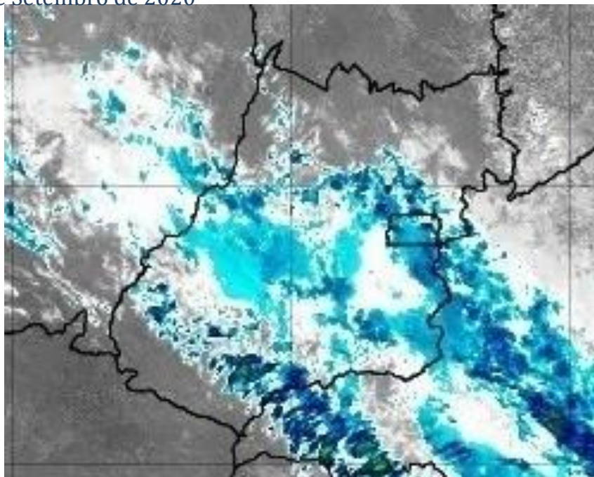
Figura 23 – Imagens realçadas do satélite GOES-16 das 13h00 do dia 23 de Setembro de 2020. FONTE: Cptec/INPE.
