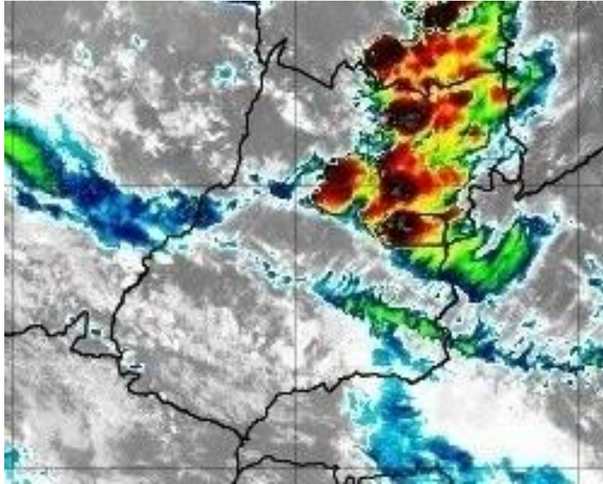
Figura 6 – Imagens realçadas do satélite GOES-16 das 15h00 do dia 21 de Setembro de 2020. FONTE: Cptec/INPE.
