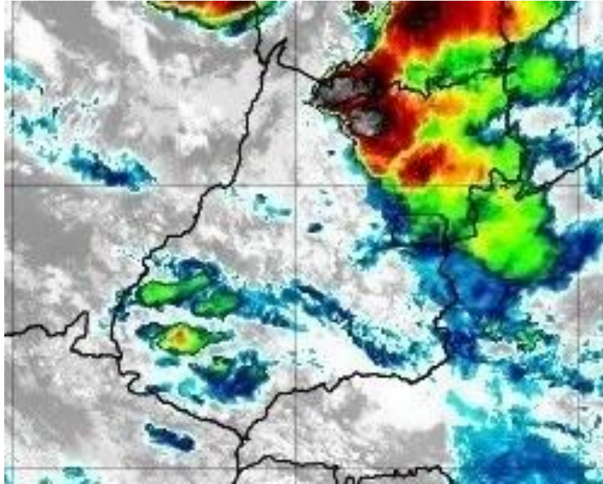
Figura 8 – Imagens realçadas do satélite GOES-16 das 19h00 do dia 21 de Setembro de 2020. FONTE: Cptec/INPE.
