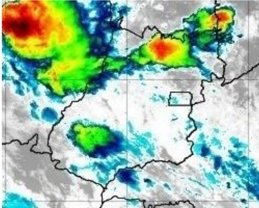
Figura 18 – Imagens realçadas do satélite GOES-16 das 21h00 do dia 22 de Setembro de 2020. FONTE: Cptec/INPE.
