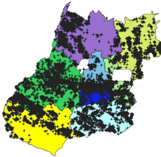
Figura 2 – Descargas atmosféricas nuvem-solo (em preto) detectadas pelo sistema Earth Networks entre 13h50 do dia 17 e 00h00 do dia 20 de outubro de 2020 sobre a área de concessão da ENEL DISTRIBUIÇÃO GOIÁS.
