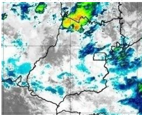
Figura 20 – Imagens realçadas do satélite GOES-16 das 12h00 do dia 19 de Outubro de 2020. FONTE: Cptec/INPE.
