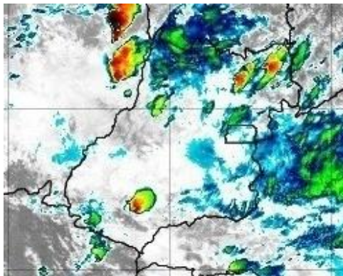
Figura 21 – Imagens realçadas do satélite GOES-16 das 15h00 do dia 19 de Outubro de 2020. FONTE: Cptec/INPE.
