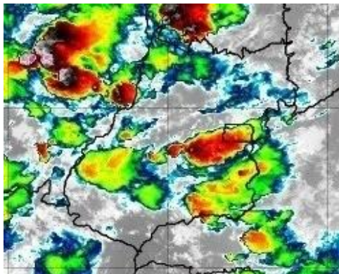
Figura 14 – Imagens realçadas do satélite GOES-16 das 18h00 do dia 18 de Outubro de 2020. FONTE: Cptec/INPE.
