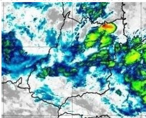
Figura 18 – Imagens realçadas do satélite GOES-16 das 6h00 do dia 19 de Outubro de 2020. FONTE: Cptec/INPE.
