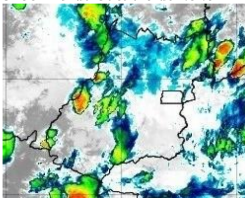
Figura 22 – Imagens realçadas do satélite GOES-16 das 18h00 do dia 19 de Outubro de 2020. FONTE: Cptec/INPE.
