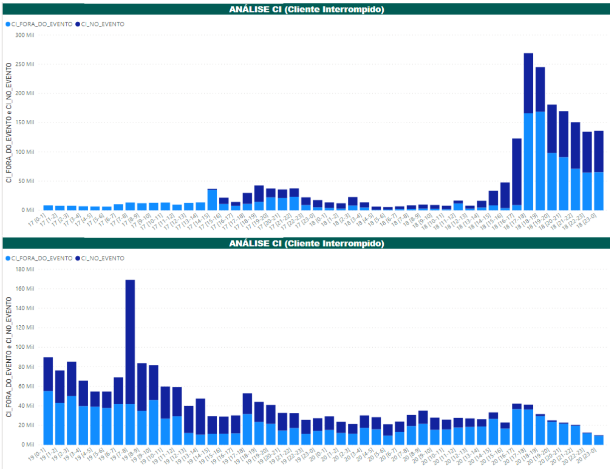
Figuras – Clientes Interrompidos em intervalos de horas
