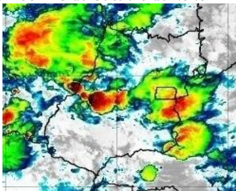
Figura 15 – Imagens realçadas do satélite GOES-16 das 21h00 do dia 18 de Outubro de 2020. FONTE: Cptec/INPE.
