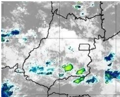
Figura 8 – Imagens realçadas do satélite GOES-16 das 0h00 do dia 18 de Outubro de 2020. FONTE: Cptec/INPE.
