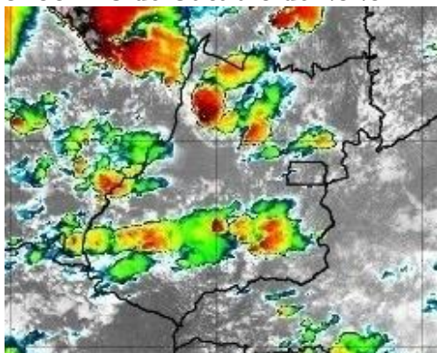
Figura 13 – Imagens realçadas do satélite GOES-16 das 15h00 do dia 18 de Outubro de 2020. FONTE: Cptec/INPE.
