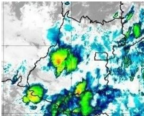
Figura 23 – Imagens realçadas do satélite GOES-16 das 21h00 do dia 19 de Outubro de 2020. FONTE: Cptec/INPE.
