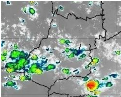
Figura 6 – Imagens realçadas do satélite GOES-16 das 18h00 do dia 17 de Outubro de 2020. FONTE: Cptec/INPE.
