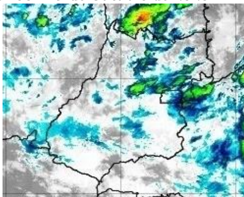
Figura 19 – Imagens realçadas do satélite GOES-16 das 9h00 do dia 19 de Outubro de 2020. FONTE: Cptec/INPE.
