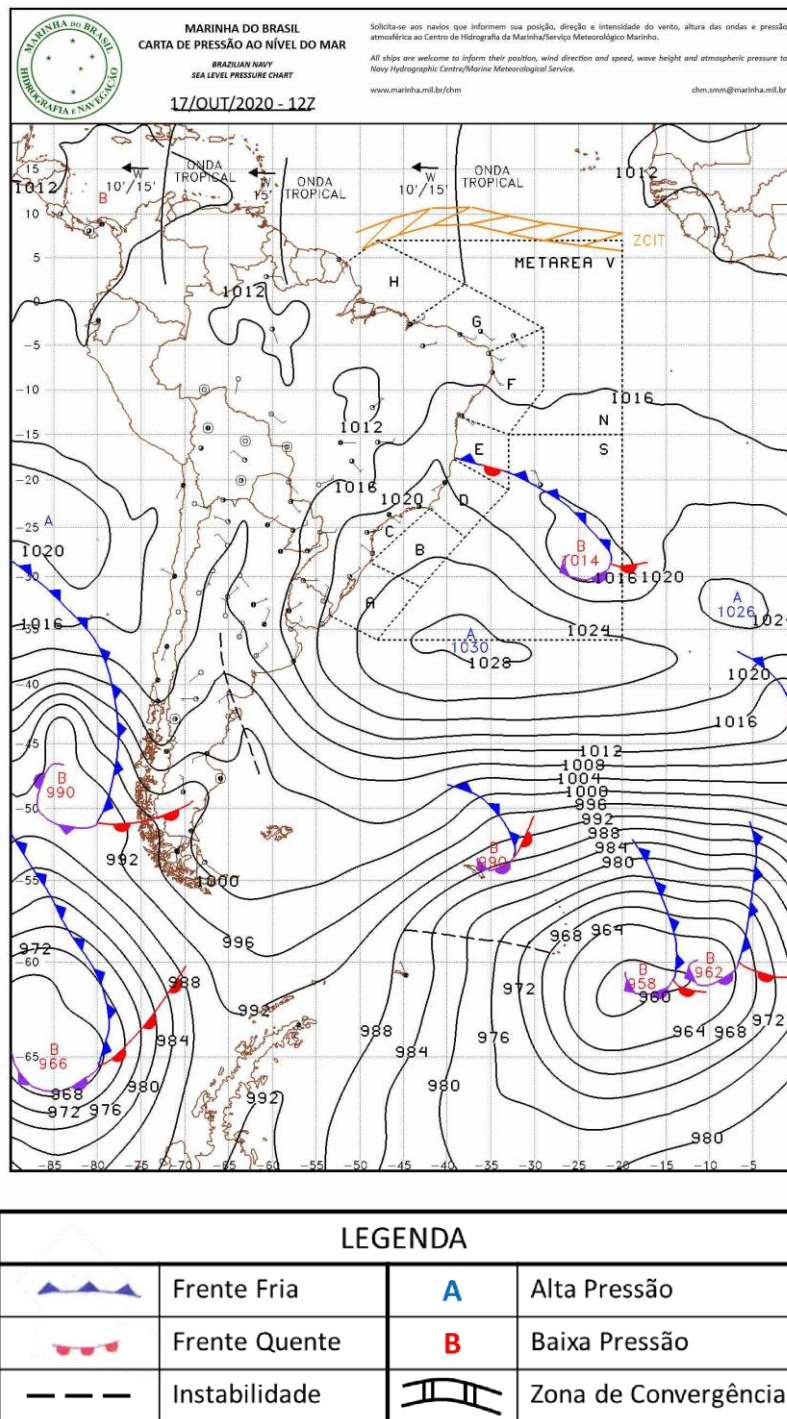
Figura A1 - Carta sinótica da Marinha do Brasil para as 1200Z do dia 17 de outubro de 2020 (09h00 do dia 17 de outubro de 2020, hora local).
