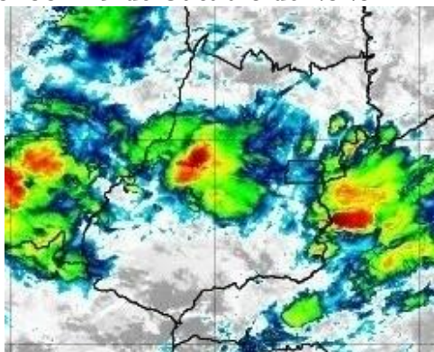
Figura 16 – Imagens realçadas do satélite GOES-16 das 0h00 do dia 19 de Outubro de 2020. FONTE: Cptec/INPE.
