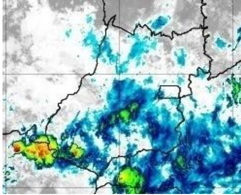
Figura 24 – Imagens realçadas do satélite GOES-16 das 0h00 do dia 20 de Outubro de 2020. FONTE: Cptec/INPE.
