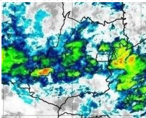
Figura 17 – Imagens realçadas do satélite GOES-16 das 3h00 do dia 19 de Outubro de 2020. FONTE: Cptec/INPE.
