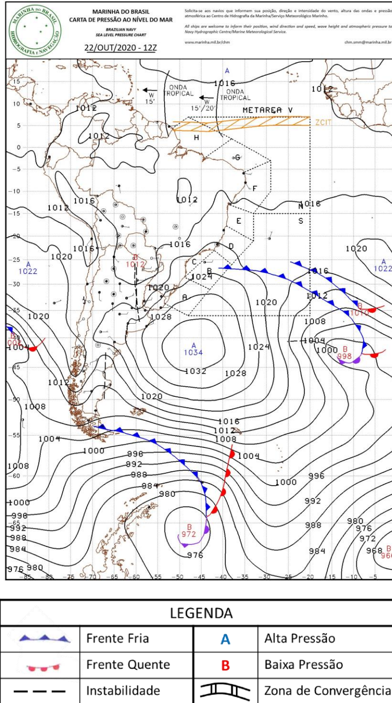
Figura A1 - Carta sinótica da Marinha do Brasil para as 1200Z do dia 22 de outubro de 2020 (09h00 do dia 22 de outubro de 2020, hora local).
