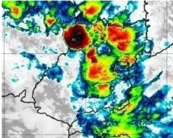
Figura 17 – Imagens realçadas do satélite GOES-16 das 3h00 do dia 24 de Outubro de 2020. FONTE: Cptec/INPE.
