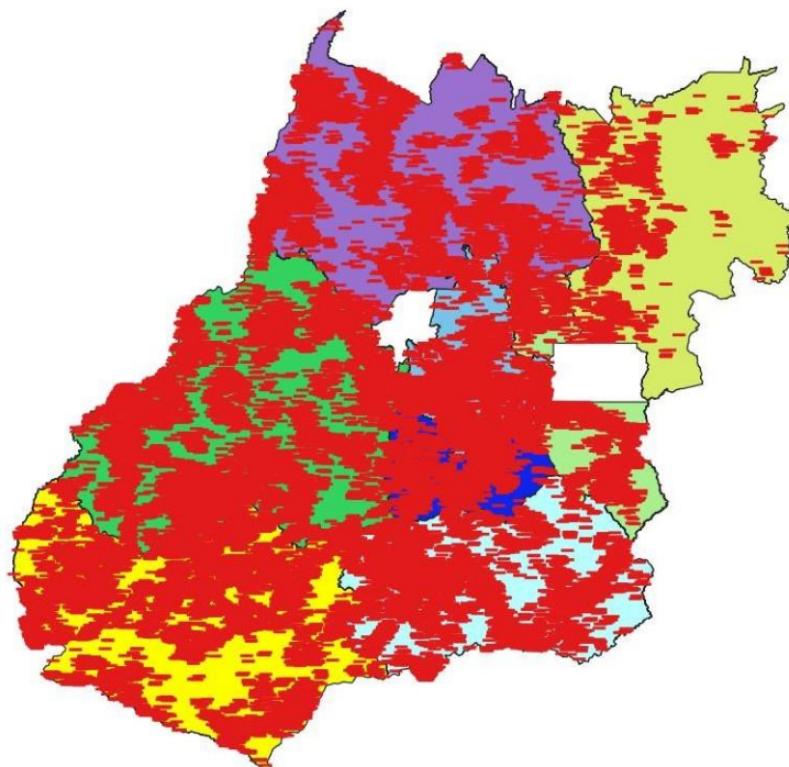
Figura 3 – Descargas atmosféricas nuvem-nuvem (em vermelho) detectadas pelo sistema Earth Networks entre 11h00 do dia 22 e as 09h40 do dia 24 de outubro de 2020 sobre a área de concessão da ENEL DISTRIBUIÇÃO GOIÁS.
