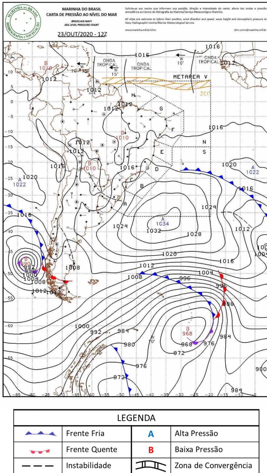
Figura A2 - Carta sinótica da Marinha do Brasil para as 1200Z do dia 23 de outubro de 2020 (09h00 do dia 23 de outubro de 2020, hora local).
