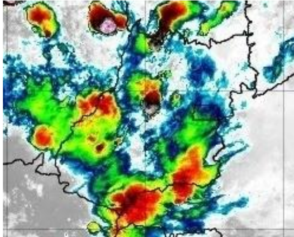
Figura 15 – Imagens realçadas do satélite GOES-16 das 21h00 do dia 23 de Outubro de 2020. FONTE: Cptec/INPE.
