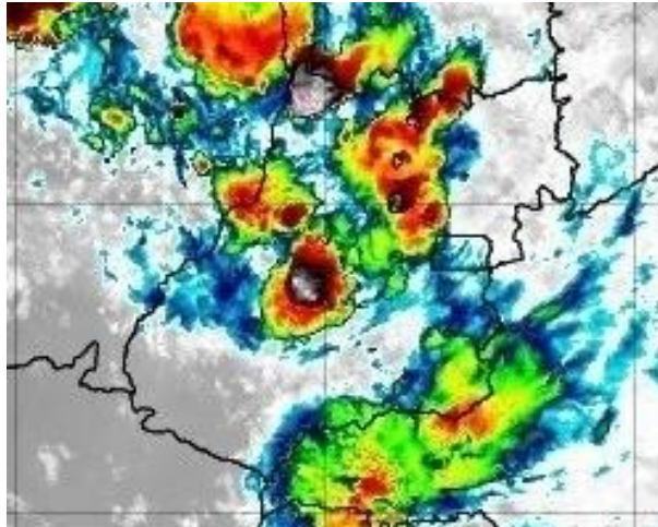
Figura 16 – Imagens realçadas do satélite GOES-16 das 0h00 do dia 24 de Outubro de 2020. FONTE: Cptec/INPE.
