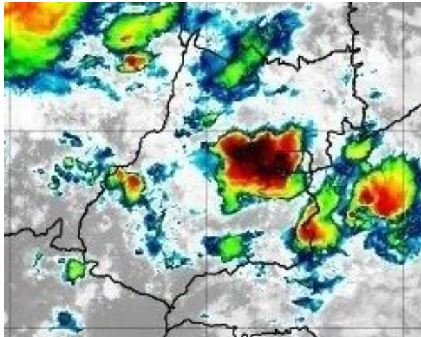
Figura 7 – Imagens realçadas do satélite GOES-16 das 21h00 do dia 22 de Outubro de 2020. FONTE: Cptec/INPE.
