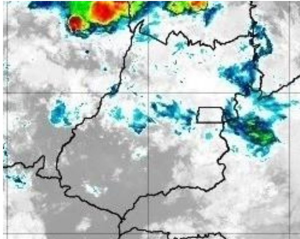
Figura 10 – Imagens realçadas do satélite GOES-16 das 6h00 do dia 23 de Outubro de 2020. FONTE: Cptec/INPE.
