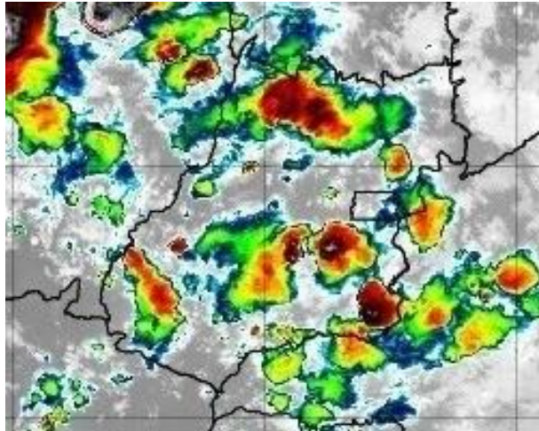
Figura 6 – Imagens realçadas do satélite GOES-16 das 18h00 do dia 22 de Outubro de 2020. FONTE: Cptec/INPE.
