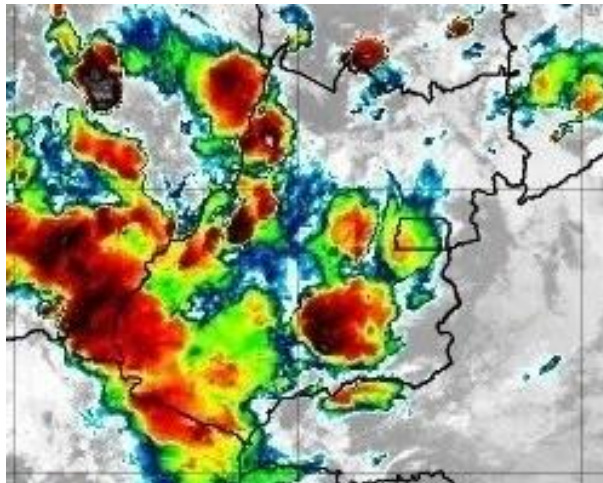
Figura 14 – Imagens realçadas do satélite GOES-16 das 18h00 do dia 23 de Outubro de 2020. FONTE: Cptec/INPE.
