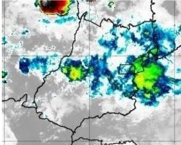
Figura 9 – Imagens realçadas do satélite GOES-16 das 3h00 do dia 23 de Outubro de 2020. FONTE: Cptec/INPE.
