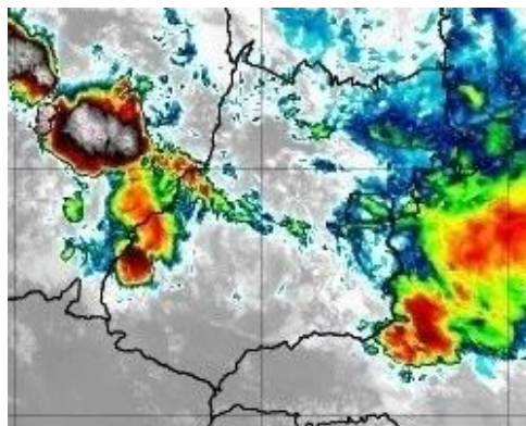
Figura 11 – Imagens realçadas do satélite GOES-16 das 19h00 do dia 31 de Outubro de 2020. FONTE: Cptec/INPE.
