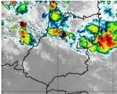
Figura 19 – Imagens realçadas do satélite GOES-16 das 18h00 do dia 02 de Novembro de 2020. FONTE: Cptec/INPE.
