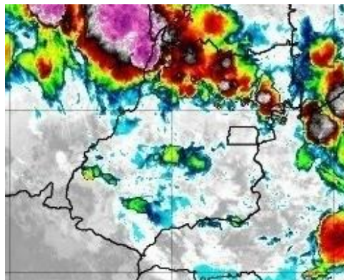
Figura 7 – Imagens realçadas do satélite GOES-16 das 23h00 do dia 30 de Outubro de 2020. FONTE: Cptec/INPE.
