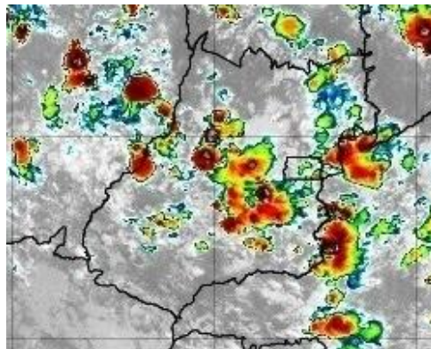
Figura 5 – Imagens realçadas do satélite GOES-16 das 15h00 do dia 30 de Outubro de 2020. FONTE: Cptec/INPE.
