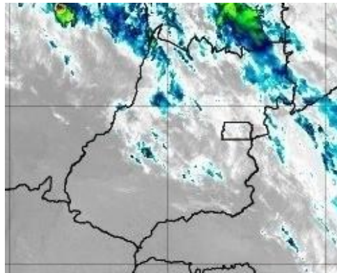
Figura 25 – Imagens realçadas do satélite GOES-16 das 6h00 do dia 04 de Novembro de 2020. FONTE: Cptec/INPE.
