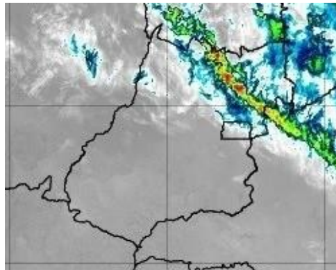
Figura 28 – Imagens realçadas do satélite GOES-16 das 0h00 do dia 05 de Novembro de 2020. FONTE: Cptec/INPE.
