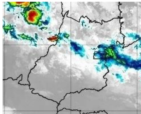
Figura 13 – Imagens realçadas do satélite GOES-16 das 6h00 do dia 01 de Novembro de 2020. FONTE: Cptec/INPE.
