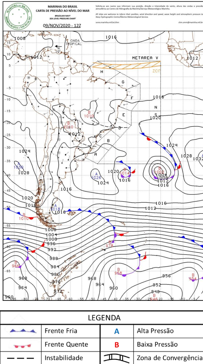
Figura A1 - Carta sinótica da Marinha do Brasil para as 1200Z do dia 09 de novembro de 2020 (09h00 do dia 09 de novembro de 2020, hora local).
