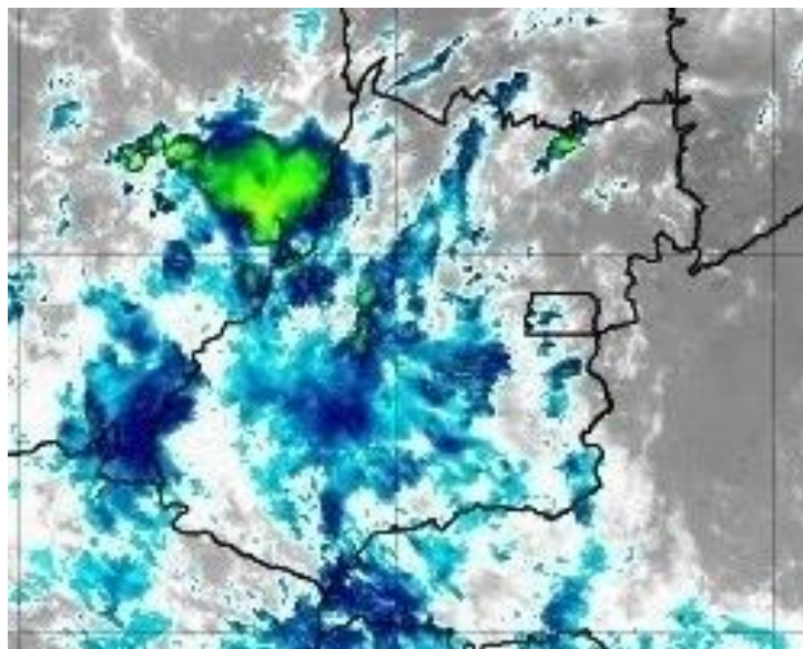
Figura 11 – Imagens realçadas do satélite GOES-16 das 9h00 do dia 10 de Novembro de 2020. FONTE: Cptec/INPE.
