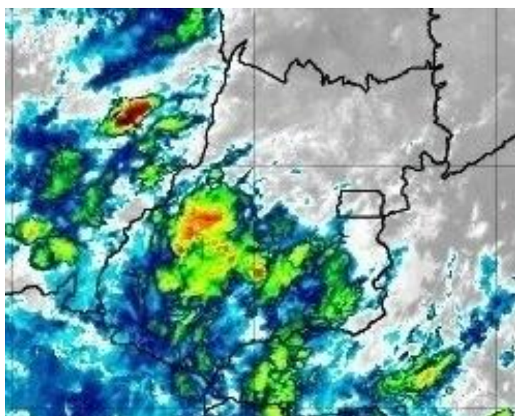
Figura 9 – Imagens realçadas do satélite GOES-16 das 3h00 do dia 10 de Novembro de 2020. FONTE: Cptec/INPE.
