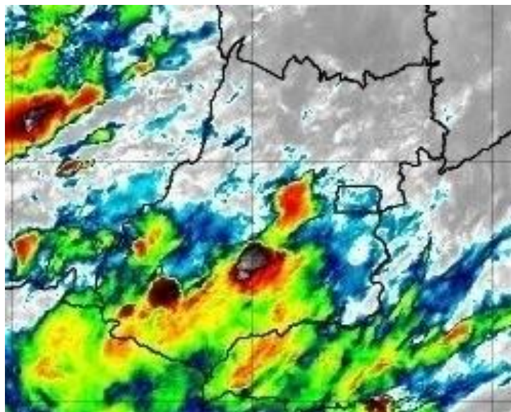
Figura 7 – Imagens realçadas do satélite GOES-16 das 21h00 do dia 9 de Novembro de 2020. FONTE: Cptec/INPE.
