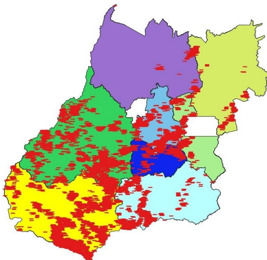
Figura 3 – Descargas atmosféricas nuvem-nuvem (em vermelho) detectadas pelo sistema Earth Networks entre 11h45 do dia 09 e 09h30 do dia 10 de novembro de 2020 sobre a área de concessão da ENEL DISTRIBUIÇÃO GOIÁS.
