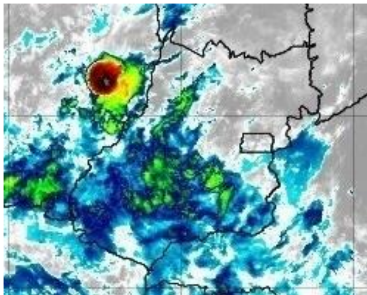
Figura 10 – Imagens realçadas do satélite GOES-16 das 6h00 do dia 10 de Novembro de 2020. FONTE: Cptec/INPE.
