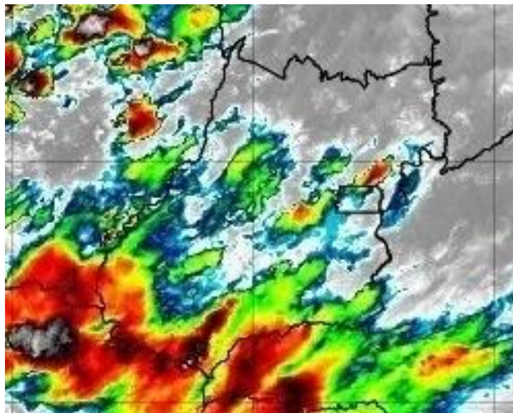
Figura 6 – Imagens realçadas do satélite GOES-16 das 18h00 do dia 09 de Novembro de 2020. FONTE: Cptec/INPE.
