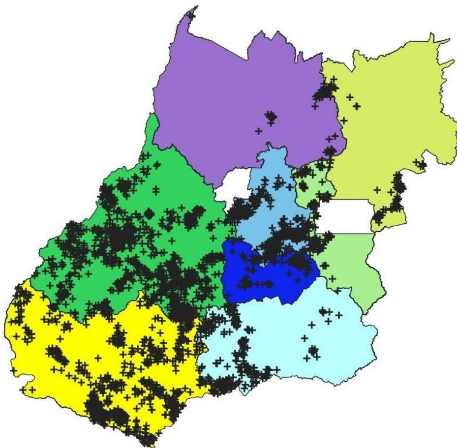
Figura 2 – Descargas atmosféricas nuvem-solo (em preto) detectadas pelo sistema Earth Networks entre 11h45 do dia 09 e 09h30 do dia 10 de novembro de 2020 sobre a área de concessão da ENEL DISTRIBUIÇÃO GOIÁS.
