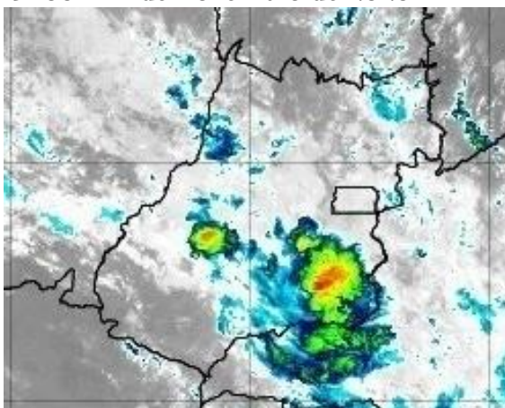
Figura 19 – Imagens realçadas do satélite GOES-16 das 9h00 do dia 14 de Novembro de 2020. FONTE: Cptec/INPE.
