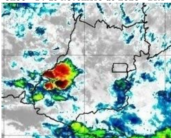
Figura 16 – Imagens realçadas do satélite GOES-16 das 0h00 do dia 14 de Novembro de 2020. FONTE: Cptec/INPE.
