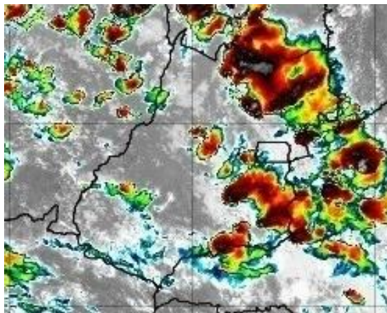
Figura 13 – Imagens realçadas do satélite GOES-16 das 15h00 do dia 13 de Novembro de 2020. FONTE: Cptec/INPE.
