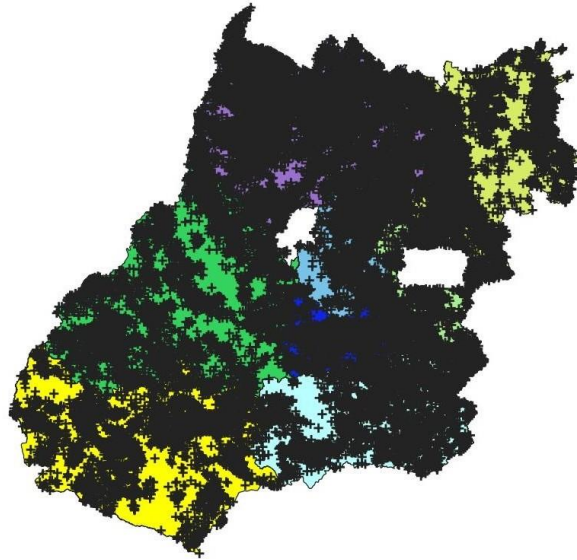
Figura 2 – Descargas atmosféricas nuvem-solo (em preto) detectadas pelo sistema Earth Networks entre 10h00 do dia 12 e 04h10 do dia 16 de novembro de 2020 sobre a área de concessão da ENEL DISTRIBUIÇÃO GOIÁS.
