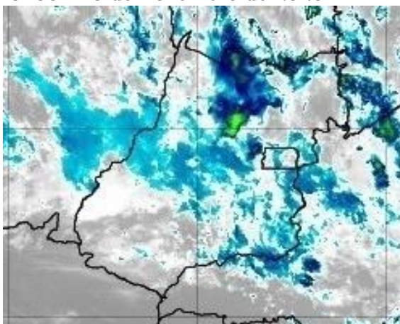
Figura 26 – Imagens realçadas do satélite GOES-16 das 6h00 do dia 15 de Novembro de 2020. FONTE: Cptec/INPE.
