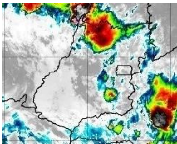
Figura 7 – Imagens realçadas do satélite GOES-16 das 21h00 do dia 12 de Novembro de 2020. FONTE: Cptec/INPE.
