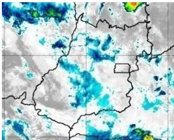
Figura 10 – Imagens realçadas do satélite GOES-16 das 6h00 do dia 13 de Novembro de 2020. FONTE: Cptec/INPE.
