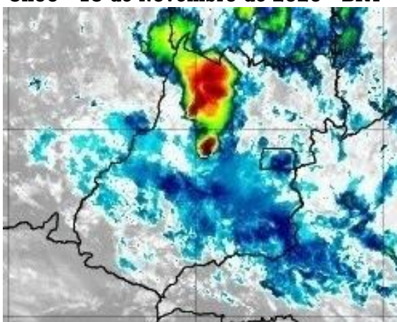
Figura 25 – Imagens realçadas do satélite GOES-16 das 3h00 do dia 15 de Novembro de 2020. FONTE: Cptec/INPE.
