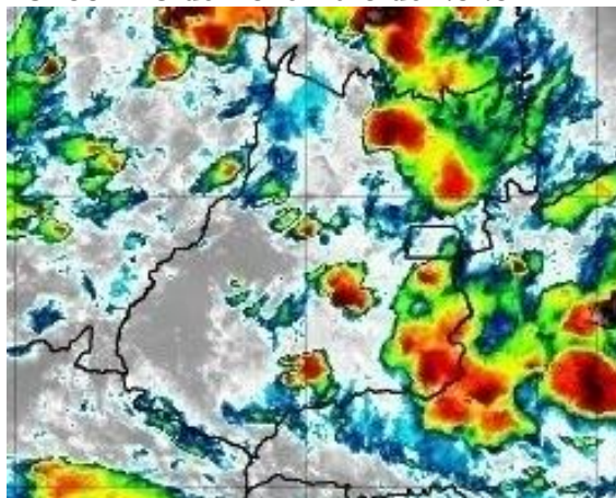
Figura 14 – Imagens realçadas do satélite GOES-16 das 18h00 do dia 13 de Novembro de 2020. FONTE: Cptec/INPE.
