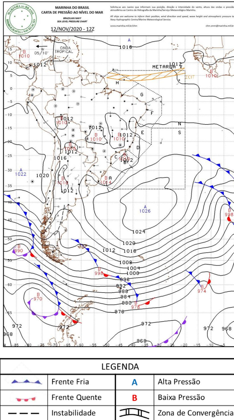
Figura A1 - Carta sinótica da Marinha do Brasil para as 1200Z do dia 12 de novembro de 2020 (09h00 do dia 12 de novembro de 2020, hora local).
