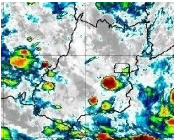
Figura 15 – Imagens realçadas do satélite GOES-16 das 21h00 do dia 13 de Novembro de 2020. FONTE: Cptec/INPE.
