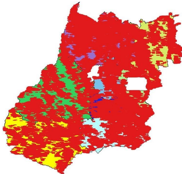
Figura 3 – Descargas atmosféricas nuvem-nuvem (em vermelho) detectadas pelo sistema Earth Networks entre 10h00 do dia 12 e 04h10 do dia 16 de novembro de 2020 sobre a área de concessão da ENEL DISTRIBUIÇÃO GOIÁS.
