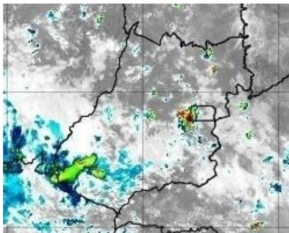
Figura 4 – Imagens realçadas do satélite GOES-16 das 12h00 do dia 12 de Novembro de 2020. FONTE: Cptec/INPE.
