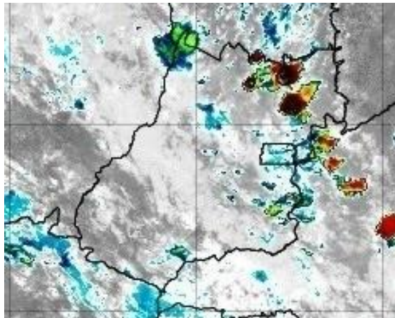
Figura 12 – Imagens realçadas do satélite GOES-16 das 12h00 do dia 13 de Novembro de 2020. FONTE: Cptec/INPE.
