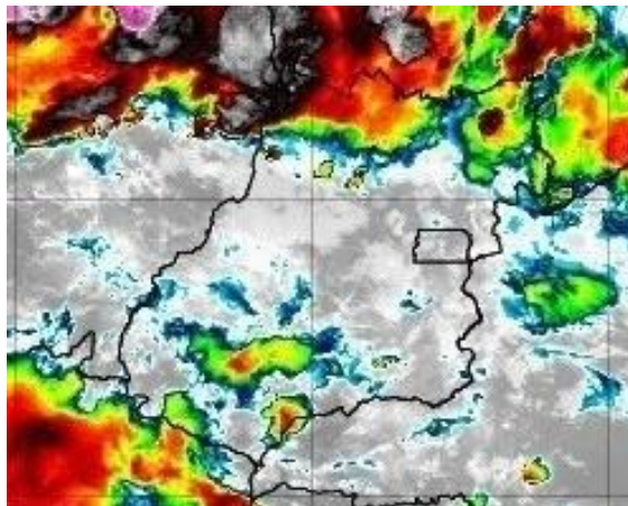
Figura 30 – Imagens realçadas do satélite GOES-16 das 18h00 do dia 15 de Novembro de 2020. FONTE: Cptec/INPE.
