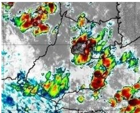
Figura 5 – Imagens realçadas do satélite GOES-16 das 15h00 do dia 12 de Novembro de 2020. FONTE: Cptec/INPE.
