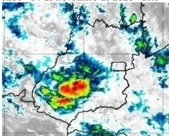
Figura 17 – Imagens realçadas do satélite GOES-16 das 3h00 do dia 14 de Novembro de 2020. FONTE: Cptec/INPE.
