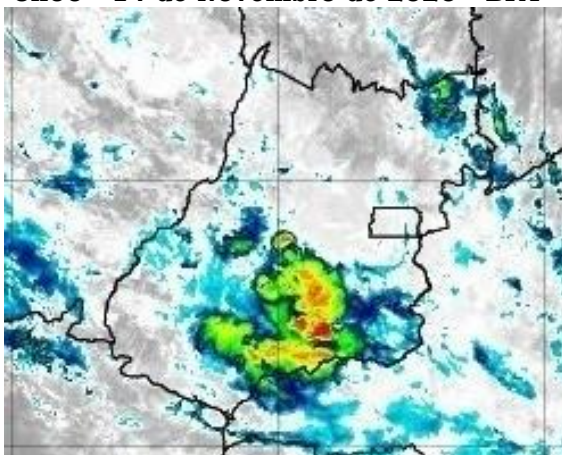
Figura 18 – Imagens realçadas do satélite GOES-16 das 6h00 do dia 14 de Novembro de 2020. FONTE: Cptec/INPE.
