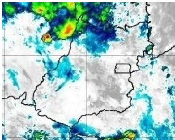
Figura 9 – Imagens realçadas do satélite GOES-16 das 3h00 do dia 13 de Novembro de 2020. FONTE: Cptec/INPE.
