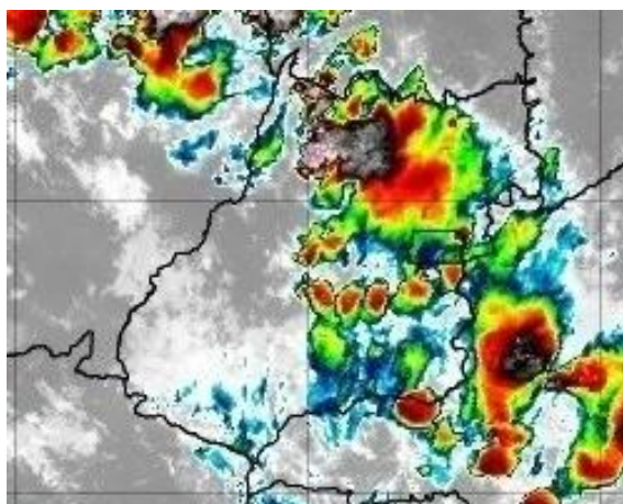
Figura 6 – Imagens realçadas do satélite GOES-16 das 18h00 do dia 12 de Novembro de 2020. FONTE: Cptec/INPE.
