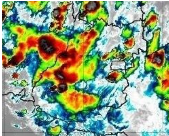
Figura 22 – Imagens realçadas do satélite GOES-16 das 18h00 do dia 14 de Novembro de 2020. FONTE: Cptec/INPE.
