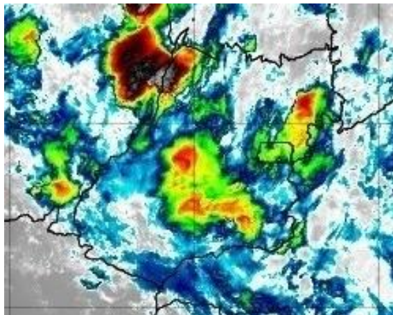
Figura 23 – Imagens realçadas do satélite GOES-16 das 21h00 do dia 14 de Novembro de 2020. FONTE: Cptec/INPE.
