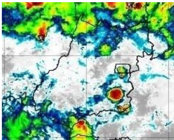
Figura 31 – Imagens realçadas do satélite GOES-16 das 21h00 do dia 15 de Novembro de 2020. FONTE: Cptec/INPE.
