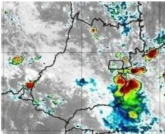
Figura 20 – Imagens realçadas do satélite GOES-16 das 12h00 do dia 14 de Novembro de 2020. FONTE: Cptec/INPE.
