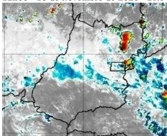
Figura 28 – Imagens realçadas do satélite GOES-16 das 12h00 do dia 15 de Novembro de 2020. FONTE: Cptec/INPE.
