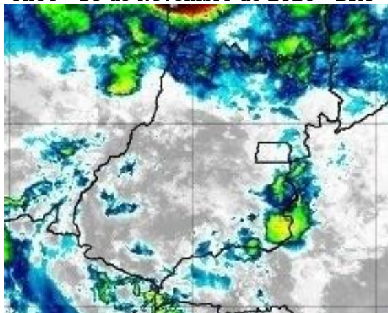
Figura 32 – Imagens realçadas do satélite GOES-16 das 0h00 do dia 16 de Novembro de 2020. FONTE: Cptec/INPE.
