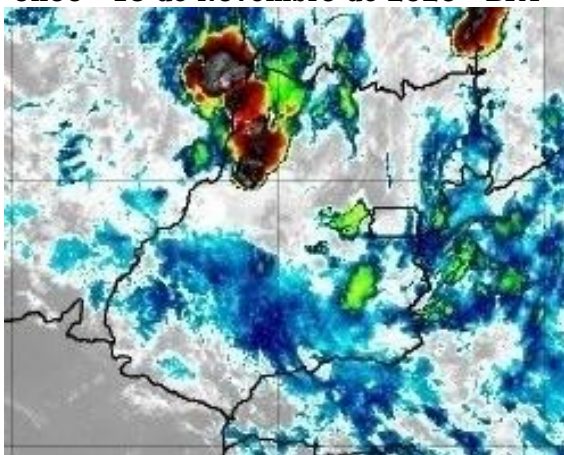
Figura 24 – Imagens realçadas do satélite GOES-16 das 0h00 do dia 15 de Novembro de 2020. FONTE: Cptec/INPE.
