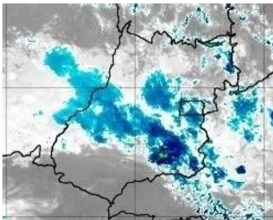
Figura 27 – Imagens realçadas do satélite GOES-16 das 9h00 do dia 15 de Novembro de 2020. FONTE: Cptec/INPE.
