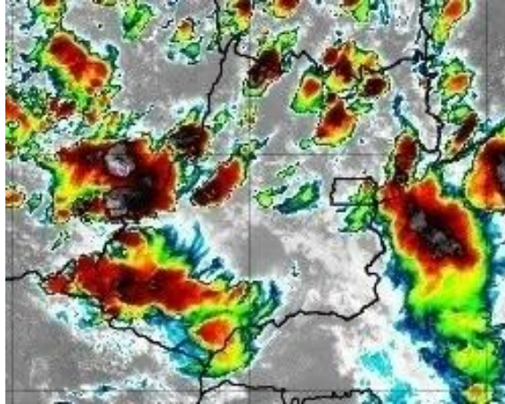
Figura 21 – Imagens realçadas do satélite GOES-16 das 15h00 do dia 14 de Novembro de 2020. FONTE: Cptec/INPE.
