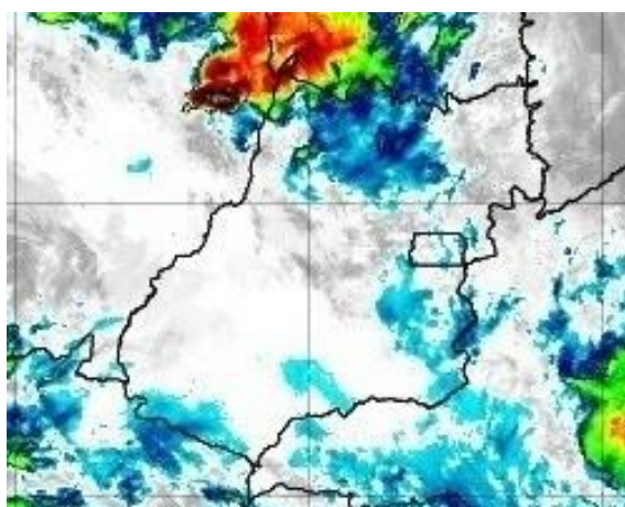
Figura 8 – Imagens realçadas do satélite GOES-16 das 0h00 do dia 13 de Novembro de 2020. FONTE: Cptec/INPE.
