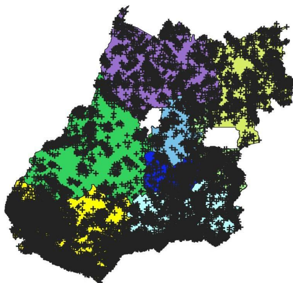
Figura 2 – Descargas atmosféricas nuvem-solo (em preto) detectadas pelo sistema Earth Networks entre 08h30 do dia 05 e 07h15 do dia 06 de dezembro de 2020 sobre a área de concessão da ENEL DISTRIBUIÇÃO GOIÁS.
