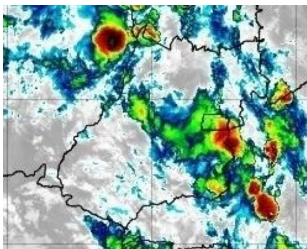
Figura 10 – Imagens realçadas do satélite GOES-16 das 6h00 do dia 06 de Dezembro de 2020. FONTE: Cptec/INPE.
