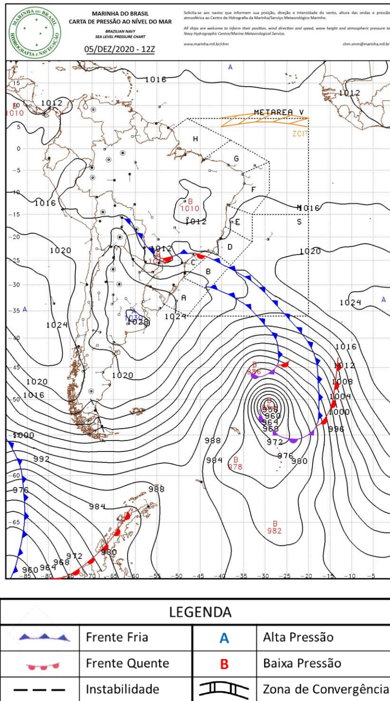
Figura A1 - Carta sinótica da Marinha do Brasil para as 1200Z do dia 05 de dezembro de 2020 (09h00 do dia 05 de dezembro de 2020, hora local).
