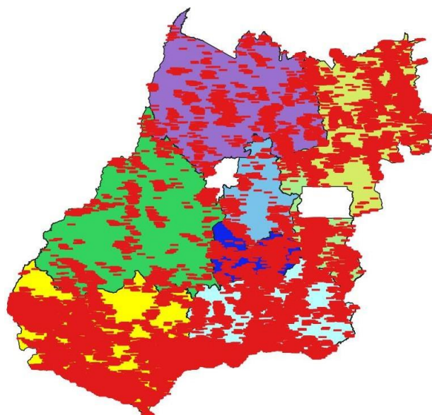
Figura 3 – Descargas atmosféricas nuvem-nuvem (em vermelho) detectadas pelo sistema Earth Networks entre 08h30 do dia 05 e 07h15 do dia 06 de dezembro de 2020 sobre a área de concessão da ENEL DISTRIBUIÇÃO GOIÁS.
