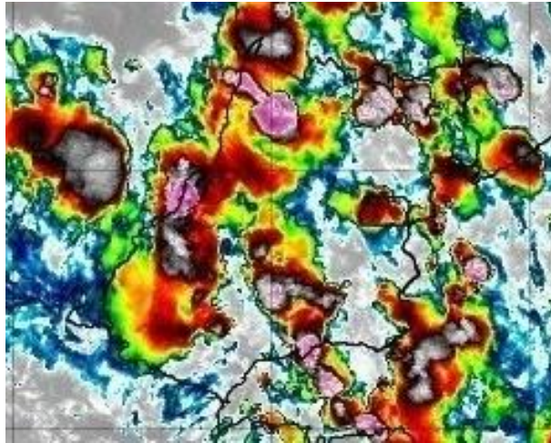
Figura 6 – Imagens realçadas do satélite GOES-16 das 18h00 do dia 05 de Dezembro de 2020. FONTE: Cptec/INPE.
