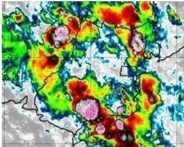
Figura 7 – Imagens realçadas do satélite GOES-16 das 21h00 do dia 05 de Dezembro de 2020. FONTE: Cptec/INPE.
