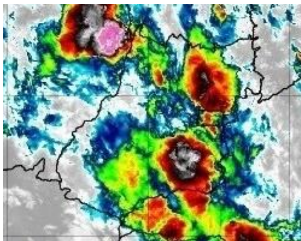
Figura 8 – Imagens realçadas do satélite GOES-16 das 0h00 do dia 06 de Dezembro de 2020. FONTE: Cptec/INPE.
