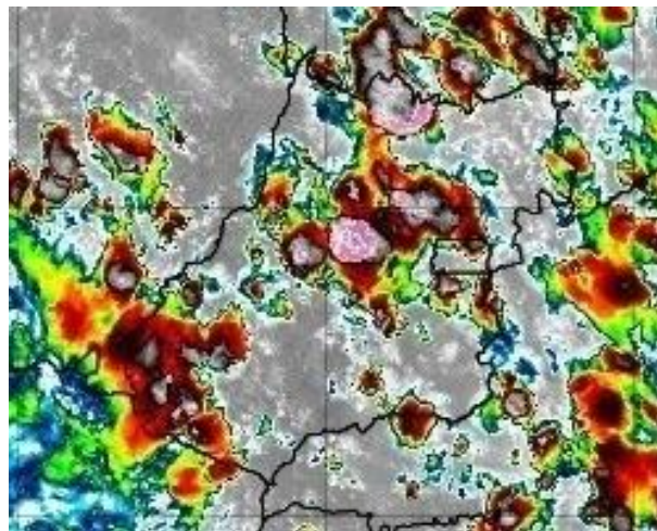
Figura 5 – Imagens realçadas do satélite GOES-16 das 15h00 do dia 05 de Dezembro de 2020. FONTE: Cptec/INPE.
