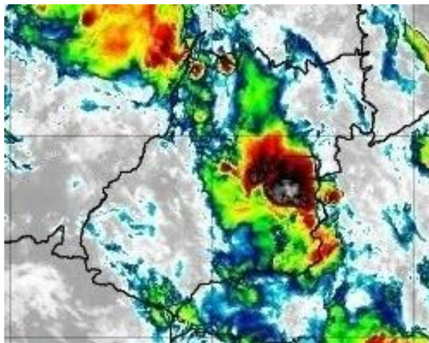
Figura 9 – Imagens realçadas do satélite GOES-16 das 3h00 do dia 06 de Dezembro de 2020. FONTE: Cptec/INPE.
