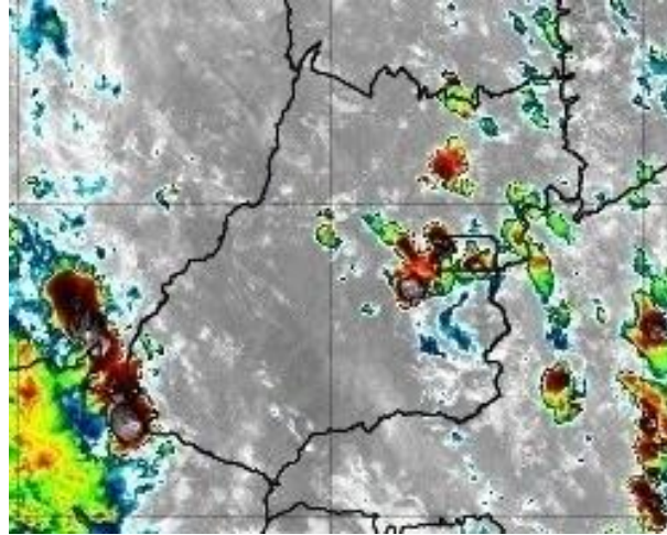
Figura 4 – Imagens realçadas do satélite GOES-16 das 12h00 do dia 05 de Dezembro de 2020. FONTE: Cptec/INPE.
