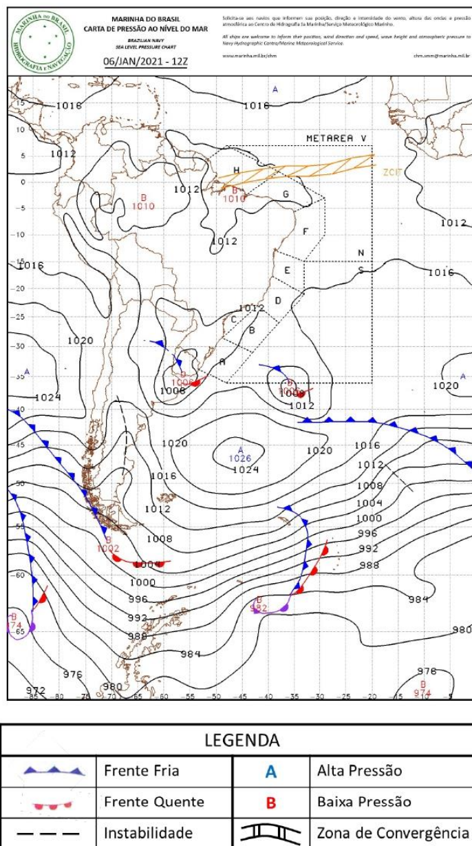
Figura A1 - Carta sinótica da Marinha do Brasil para as 1200Z do dia 06 de janeiro de 2021 (09h00 do dia 06 de janeiro de 2021, hora local).
