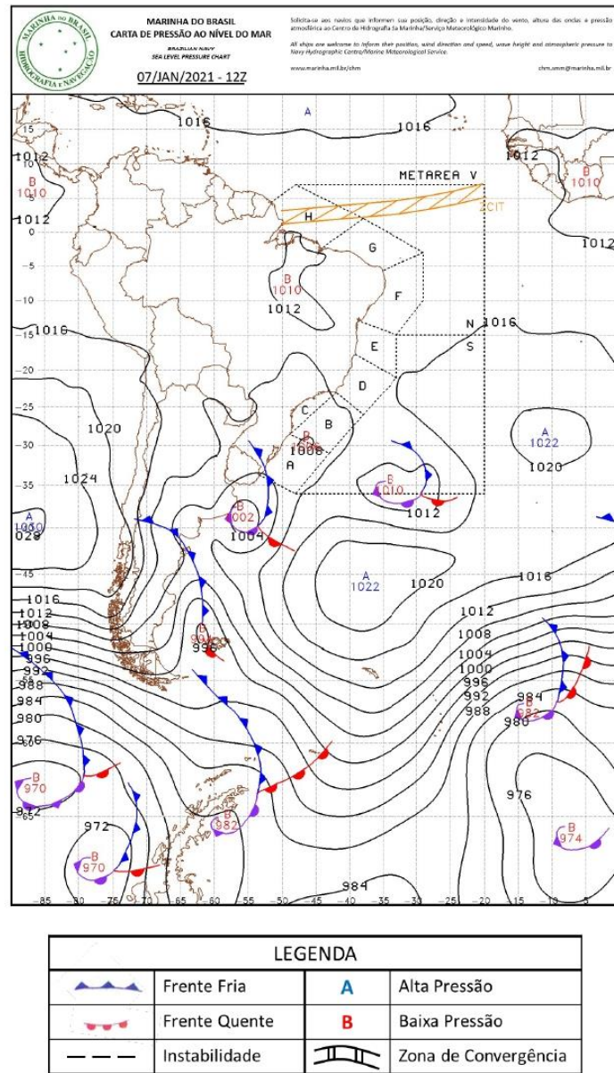
Figura A2 - Carta sinótica da Marinha do Brasil para as 1200Z do dia 07 de janeiro de 2021 (09h00 do dia 07 de janeiro de 2021, hora local).
