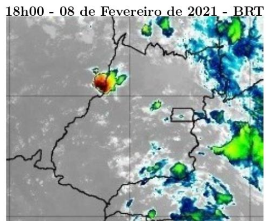
Figura 30 – Imagens realçadas do satélite GOES-16 das 18h00 do dia 08 de Fevereiro de 2021. FONTE: Cptec/INPE.
