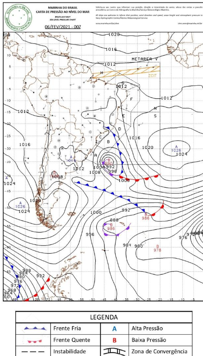
Figura A1 - Carta sinótica da Marinha do Brasil para as 0000Z do dia 06 de fevereiro de 2021 (21h00 do dia 05 de fevereiro de 2021, hora local).
