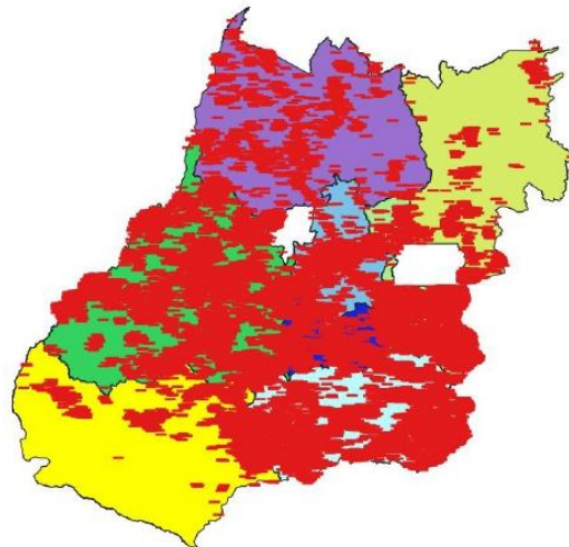
Figura 3 – Descargas atmosféricas nuvem-nuvem (em vermelho) detectadas pelo sistema Earth Networks entre 10h15 do dia 05 e 01h05 do dia 09 de fevereiro de 2021 sobre a área de concessão da ENEL DISTRIBUIÇÃO GOIÁS.
