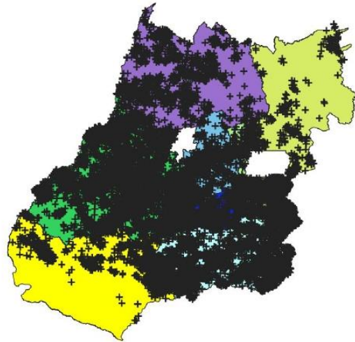
Figura 2 – Descargas atmosféricas nuvem-solo (em preto) detectadas pelo sistema Earth Networks entre 10h15 do dia 05 e 01h05 do dia 09 de fevereiro de 2021 sobre a área de concessão da ENEL DISTRIBUIÇÃO GOIÁS.
