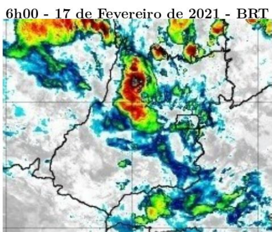
Figura 26 – Imagens realçadas do satélite GOES-16 das 6h00 do dia 17 de Fevereiro de 2021. FONTE: Cptec/INPE.
