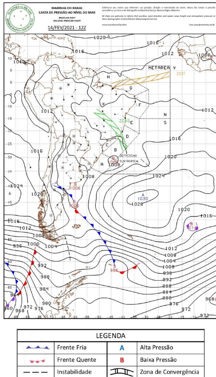
Figura A1 - Carta sinótica da Marinha do Brasil para as 1200Z do dia 14 de fevereiro de 2021 (09h00 do dia 14 de fevereiro de 2021, hora local).
