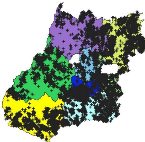
Figura 2 – Descargas atmosféricas nuvem-solo (em preto) detectadas pelo sistema Earth Networks entre 10h30 do dia 14 e 06h35 do dia 17 de fevereiro de 2021 sobre a área de concessão da ENEL DISTRIBUIÇÃO GOIÁS.
