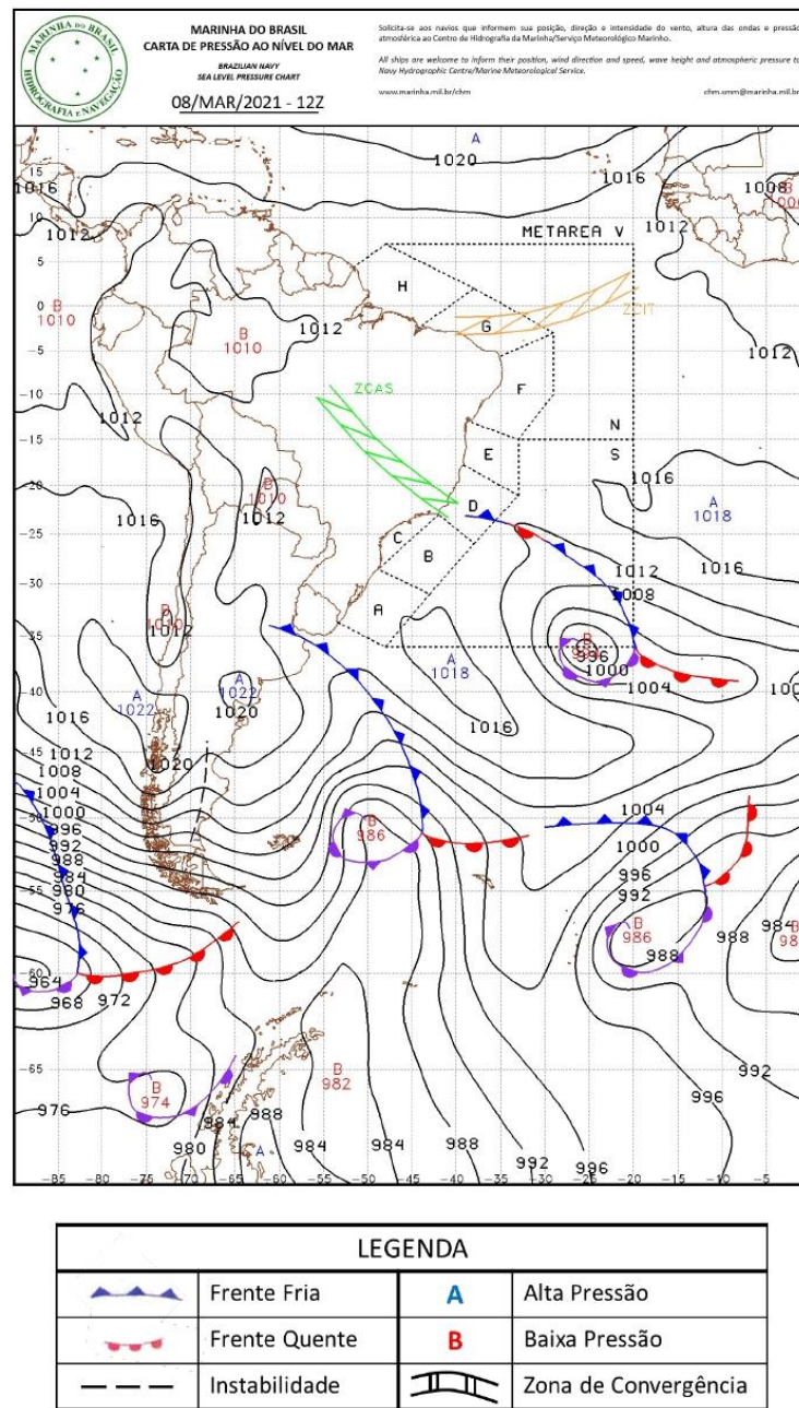
Figura A2 - Carta sinótica da Marinha do Brasil para as 1200Z do dia 08 de março de 2021 (09h00 do dia 08 de março de 2021, hora local).
