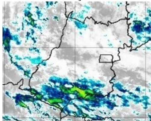
Figura 28 – Imagens realçadas do satélite GOES-16 das 0h00 do dia 12 de Março de 2021. FONTE: Cptec/INPE.
