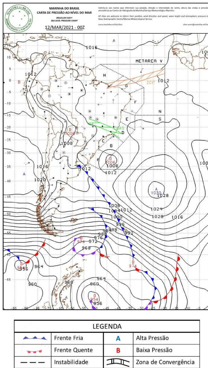
Figura A5 - Carta sinótica da Marinha do Brasil para as 0000Z do dia 12 de março de 2021 (21h00 do dia 11 de março de 2021, hora local).
