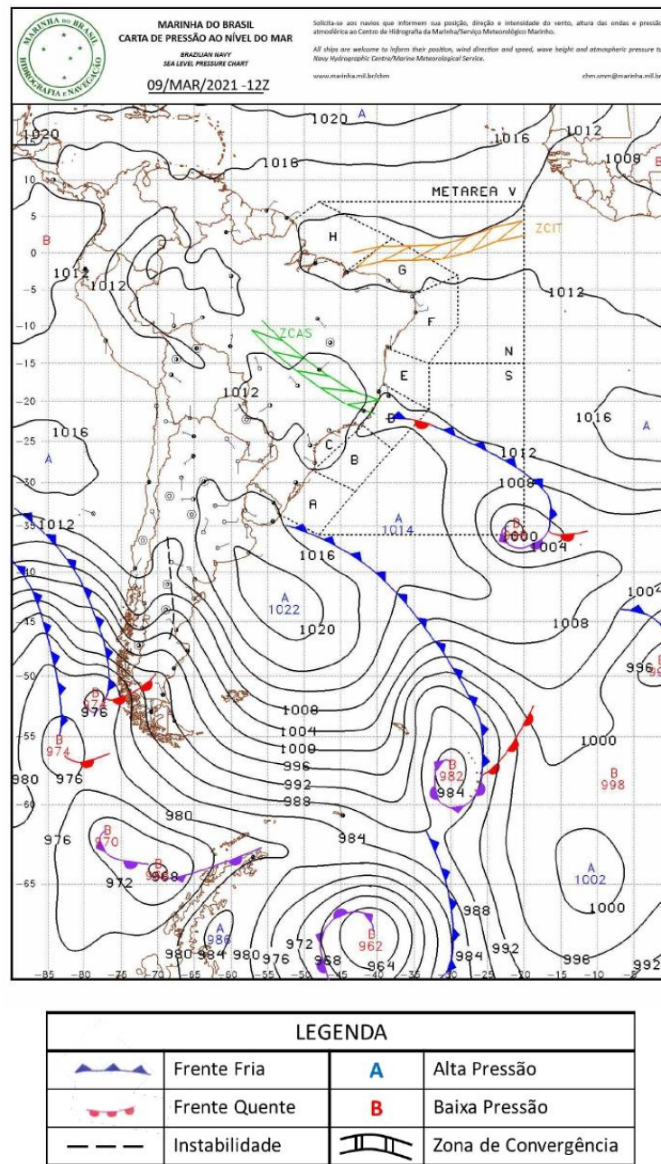
Figura A3 - Carta sinótica da Marinha do Brasil para as 1200Z do dia 09 de março de 2021 (09h00 do dia 09 de março de 2021, hora local).
