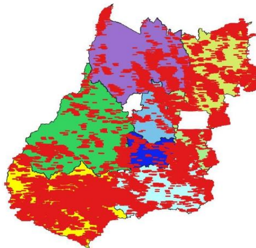
Figura 3 – Descargas atmosféricas nuvem-nuvem (em vermelho) detectadas pelo sistema Earth Networks entre 11h40 do dia 07 e 06h50 do dia 12 de março de 2021 sobre a área de concessão da ENEL DISTRIBUIÇÃO GOIÁS.
