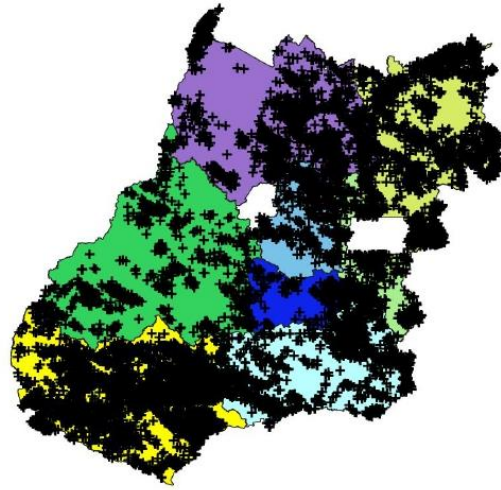
Figura 2 – Descargas atmosféricas nuvem-solo (em preto) detectadas pelo sistema Earth Networks entre 11h40 do dia 07 e 06h50 do dia 12 de março de 2021 sobre a área de concessão da ENEL DISTRIBUIÇÃO GOIÁS.
