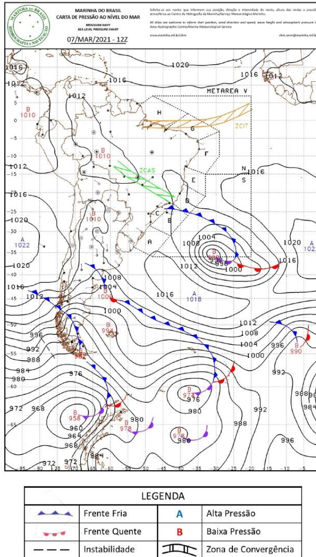
Figura A1 - Carta sinótica da Marinha do Brasil para as 1200Z do dia 07 de março de 2021 (09h00 do dia 07 de março de 2021, hora local).
