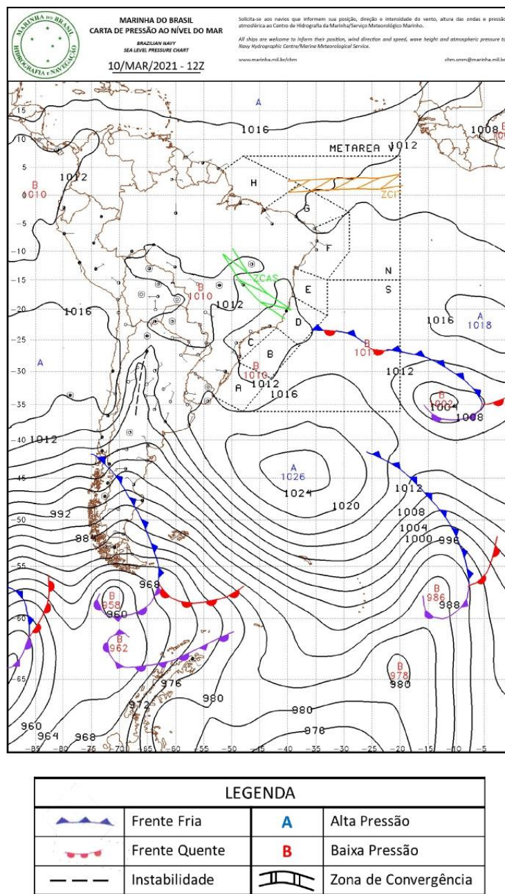
Figura A4 - Carta sinótica da Marinha do Brasil para as 1200Z do dia 10 de março de 2021 (09h00 do dia 10 de março de 2021, hora local).
