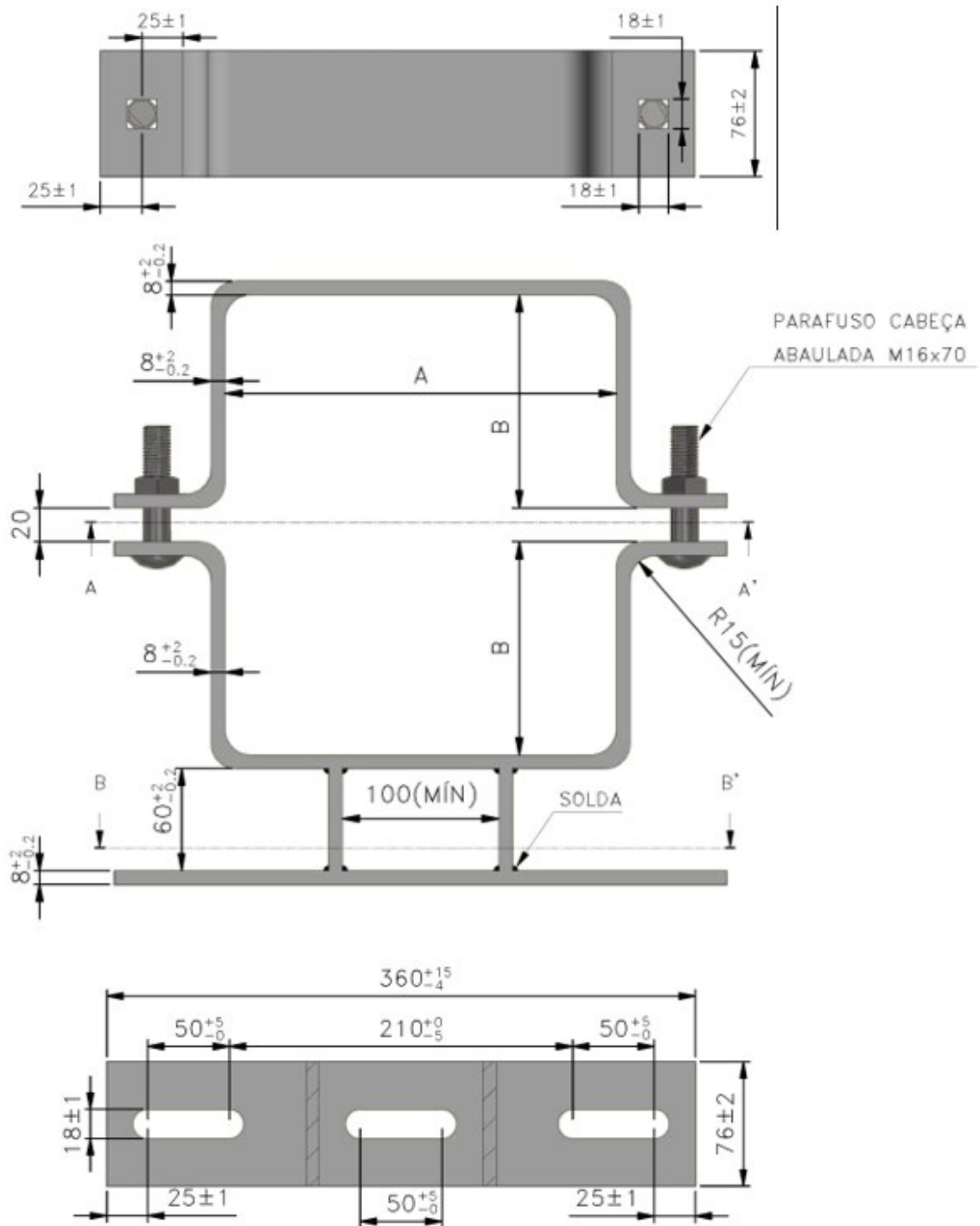
Figura 1 - Suporte para transformador em poste duplo T
