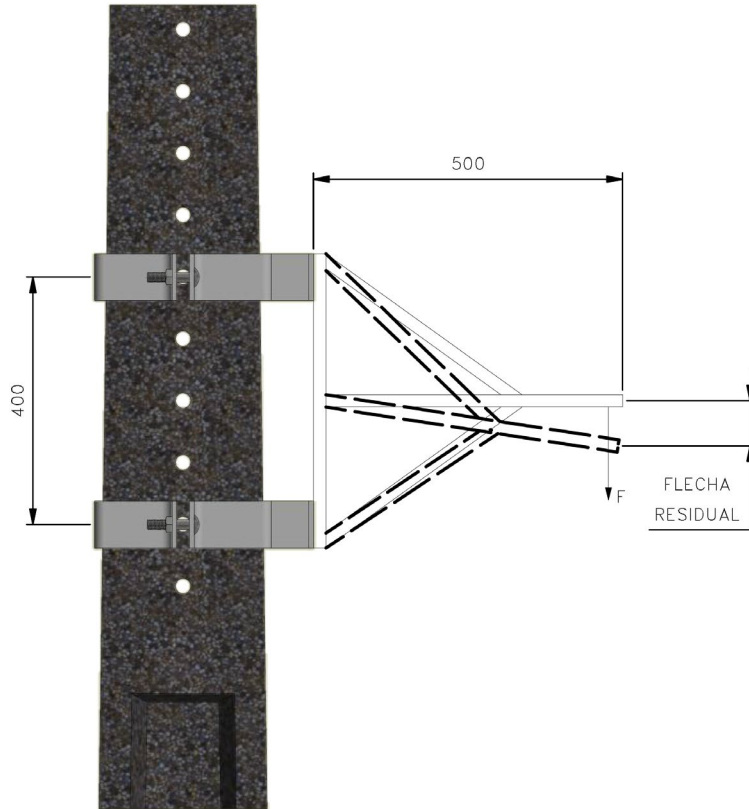
Figura 2 - Detalhe para ensaio
