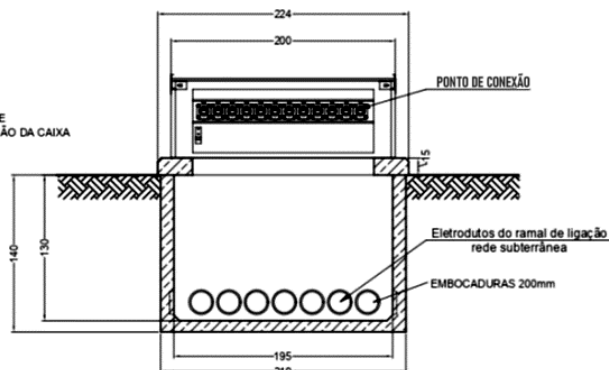
CORTE B-B
