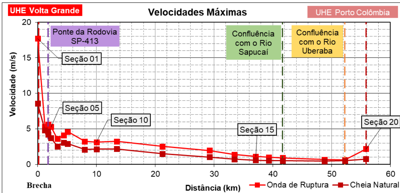
Figura 17 – Cenário 3: Velocidades Máximas na Passagem da Onda
