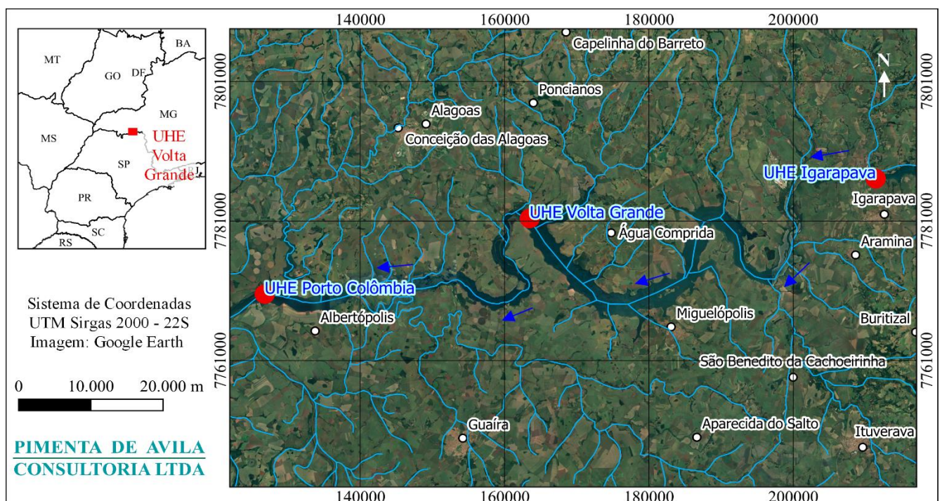
Figura 1 – Localização da UHE Volta Grande
