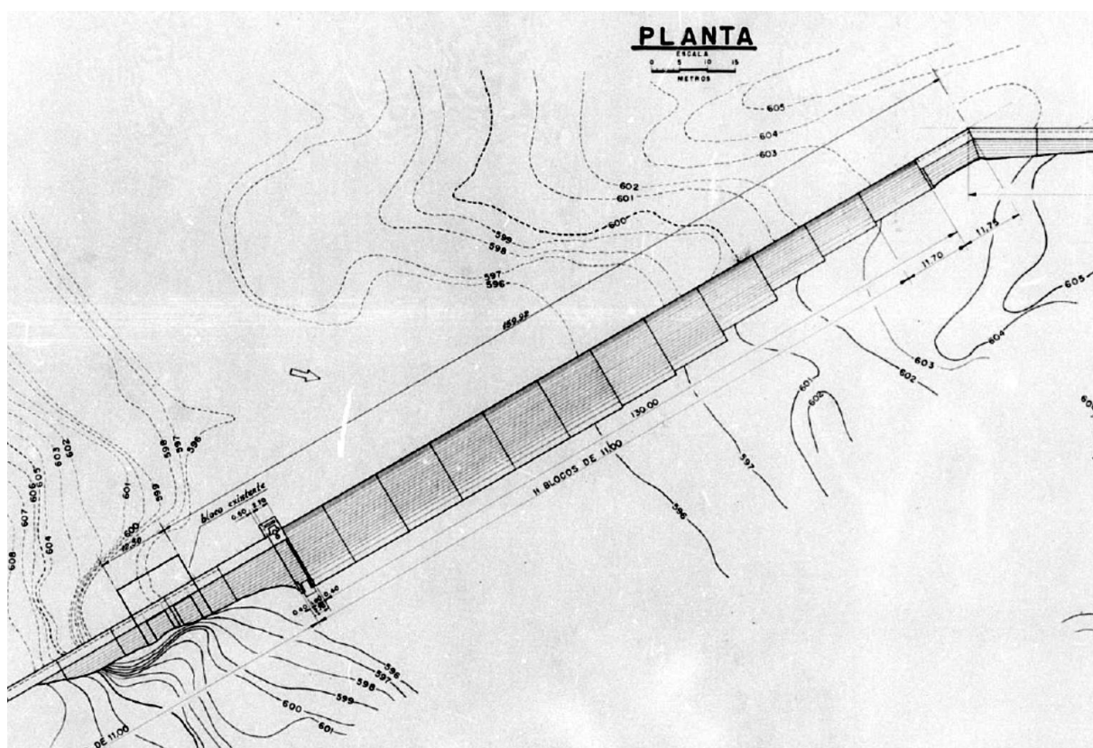
Figura 4 - Vertedouro e barragem da margem direita
