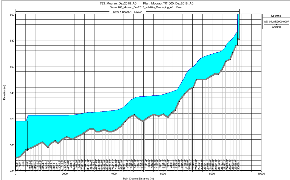
Figura 11– Cenário 2 - Chegada da onda de ruptura da barragem na última seção de jusante, na barragem da PCH Salto Natal
