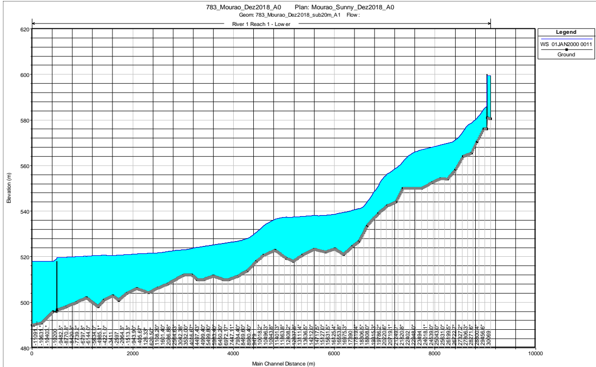
Figura 7 – Cenário 1- Chegada da onda de ruptura da barragem na última seção a jusante (barragem da PCH Salto Natal)
